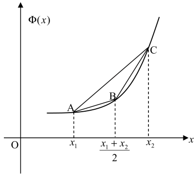
Şekil 1.1. Konveks Fonksiyon
