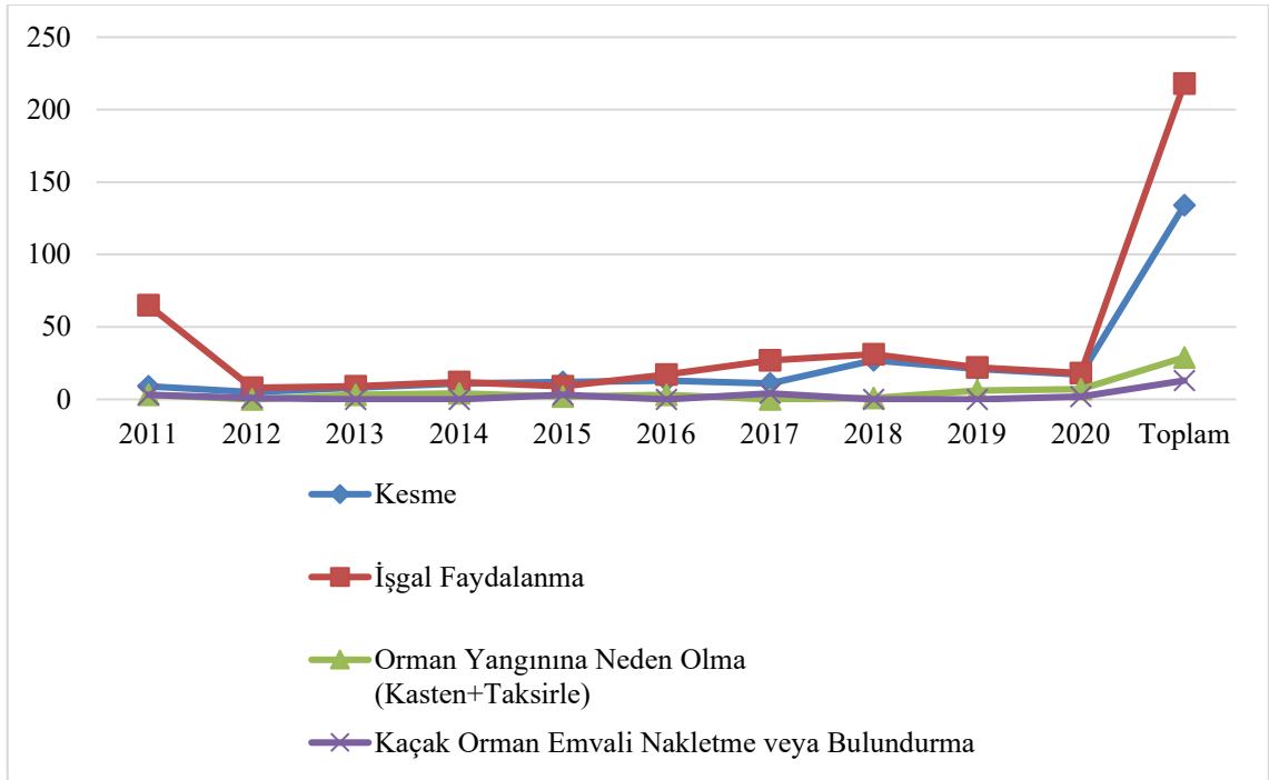
Şekil 3. YOİM’de 2011-2020 yılları arasında işlenen orman suçlarının yıllara göre artış ve azalış grafiği.
