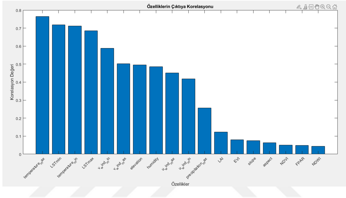
Şekil 4.2. Özellik önem grafiği
