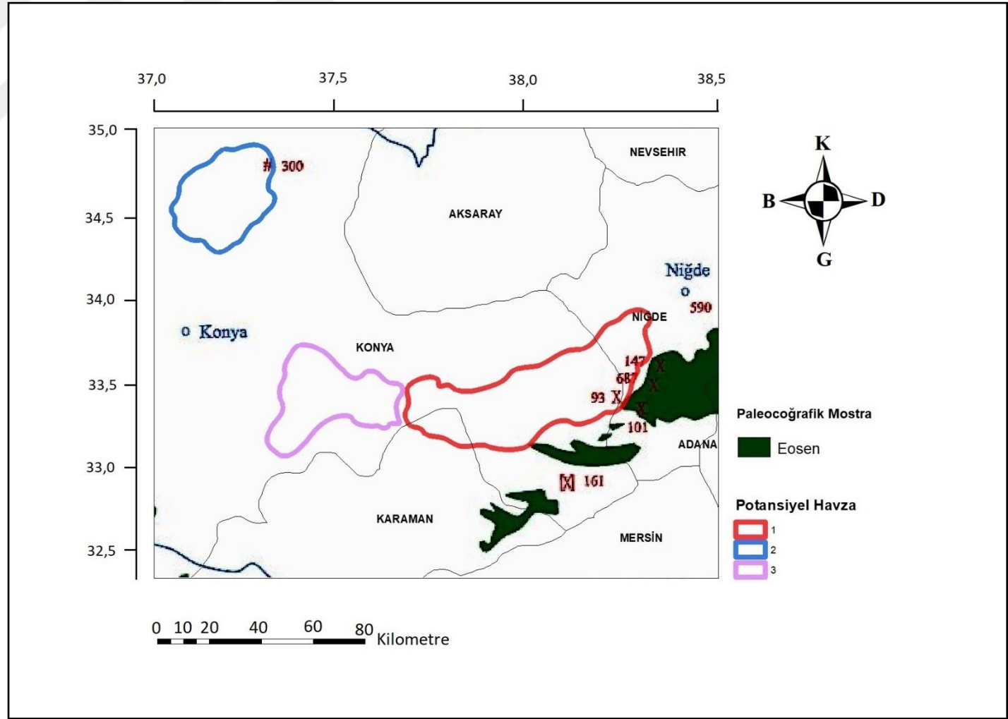
Şekil 4.3. Eosen mostra paleocoğrafya haritası (Görür vd. 1998) ile potansiyel kömür havzasının gösterimi
