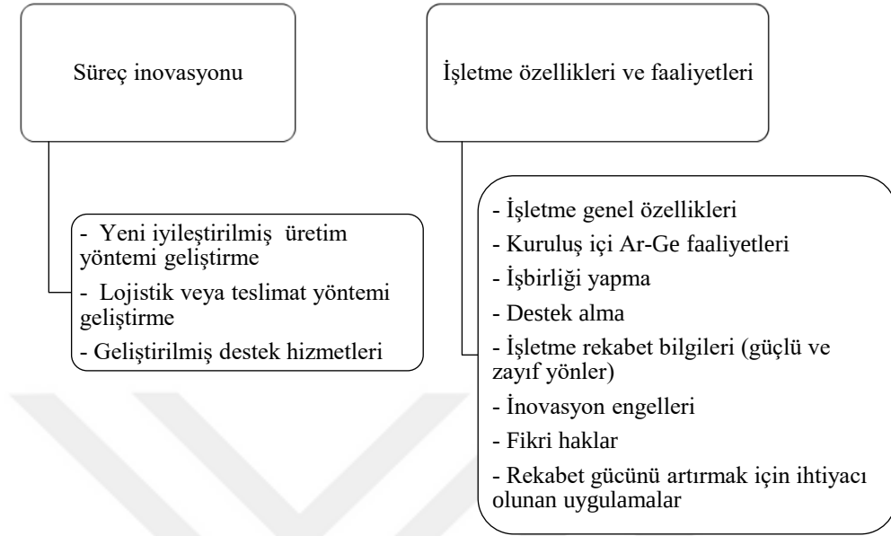
Şekil 3.2: Süreç inovasyonu hipotez alt modeli.
