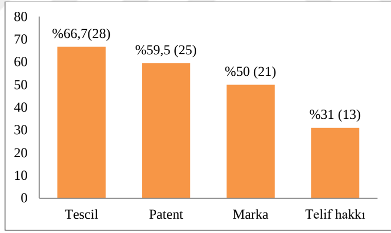
Şekil 4.7: Fikri haklar (Birden fazla cevap vardır).
