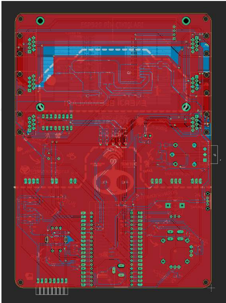
Şekil 5.16. Tasarlanan kartın ve üst bakır katmanının görüntüsü.
