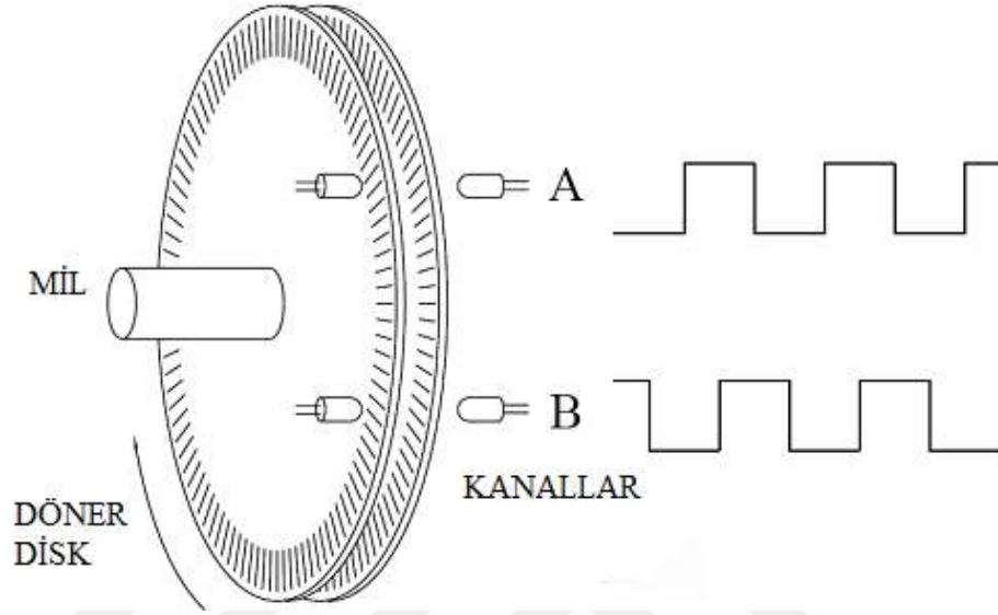
Şekil 5.4. Encoder'ın çalışma prensibi.
