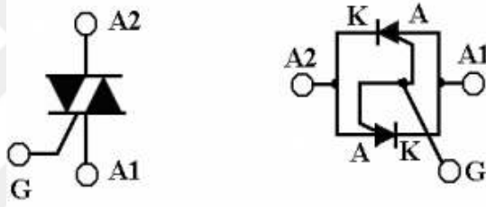
Şekil 3.9. Triyak'ın simgesi.
