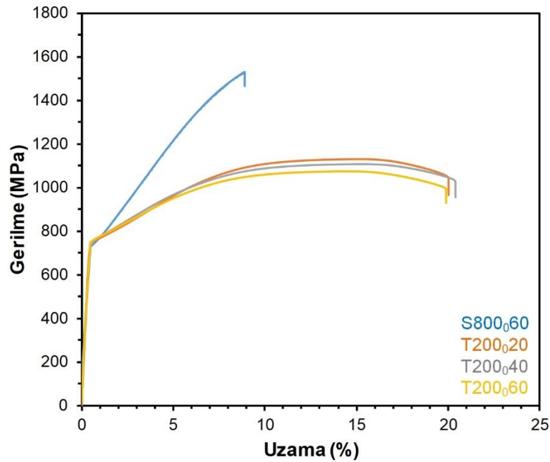
Şekil 5.158. S800 0 60, T200 0 20, T200 0 40 ve T200 0 60 numunelerinin gerilme-uzama grafikleri
