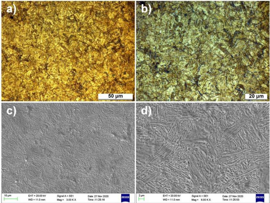
Şekil 5.59. %0.4 Cr ilaveli S650 0 .430 numunesine ait OM ve SEM görüntüleri
