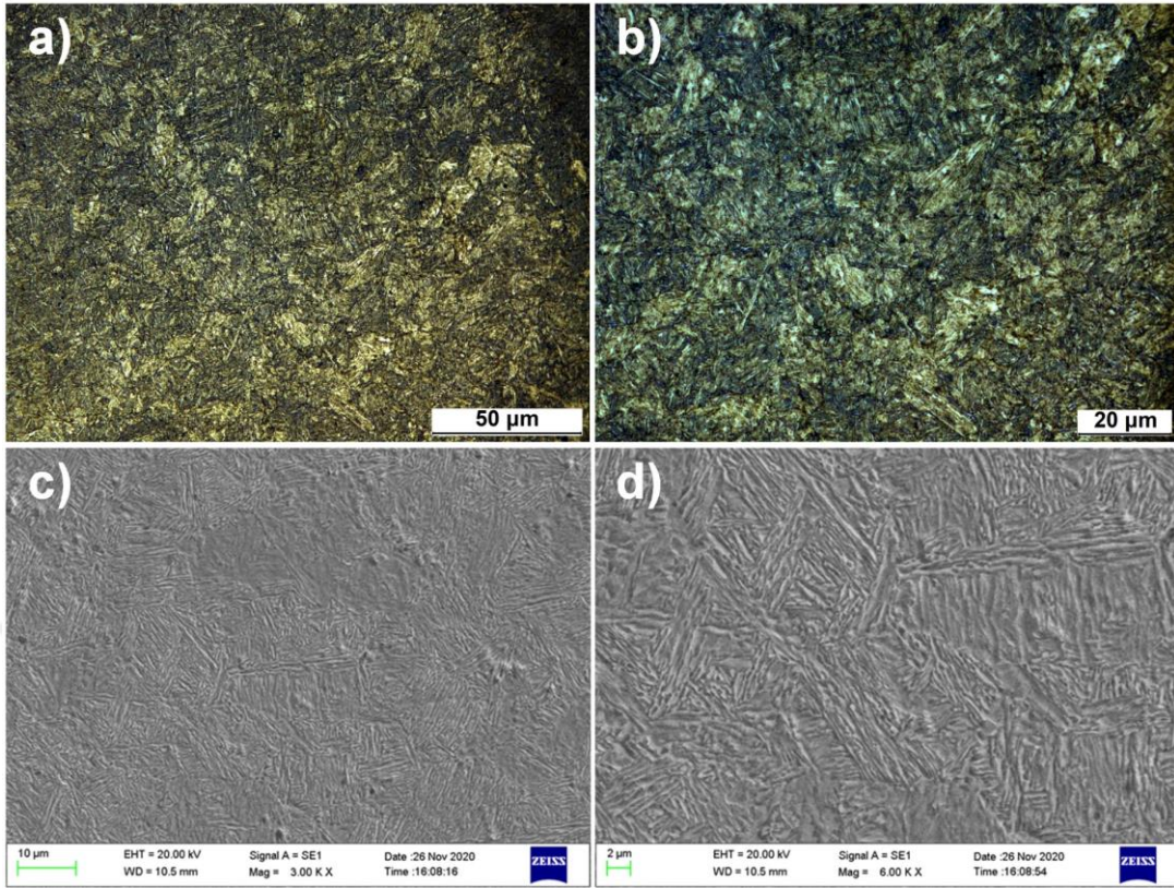
Şekil 5.53. %0.4 Cr ilaveli H650 0,430 numunesine ait OM ve SEM görüntüleri
