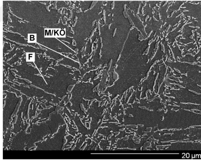
Őekil 2.7. Tipik bir TRIP eliēi mikroyapısının SEM grntē (F: Ferrit, B: Beynit, M: Martenzit ve K: Kalıntı stenit) [54]
