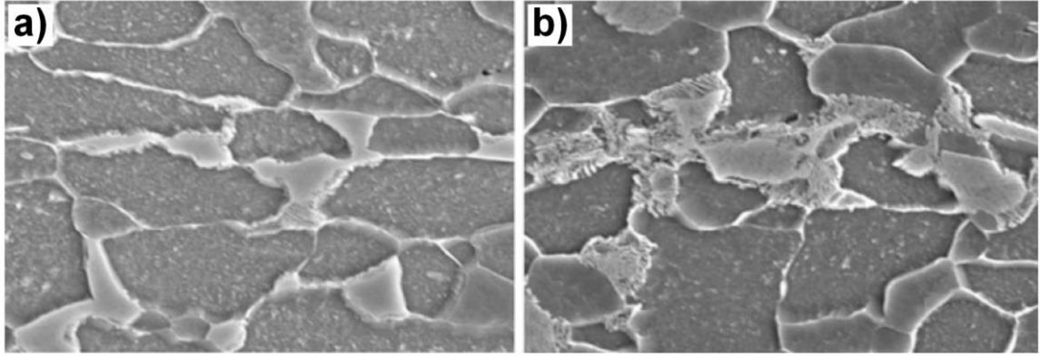
Şekil 2.23. (a) 740°C ve (b) 760°C’de tavlanmış 0.1C-0.5Mn çeliğinin mikroyapı görüntüsü [114]
