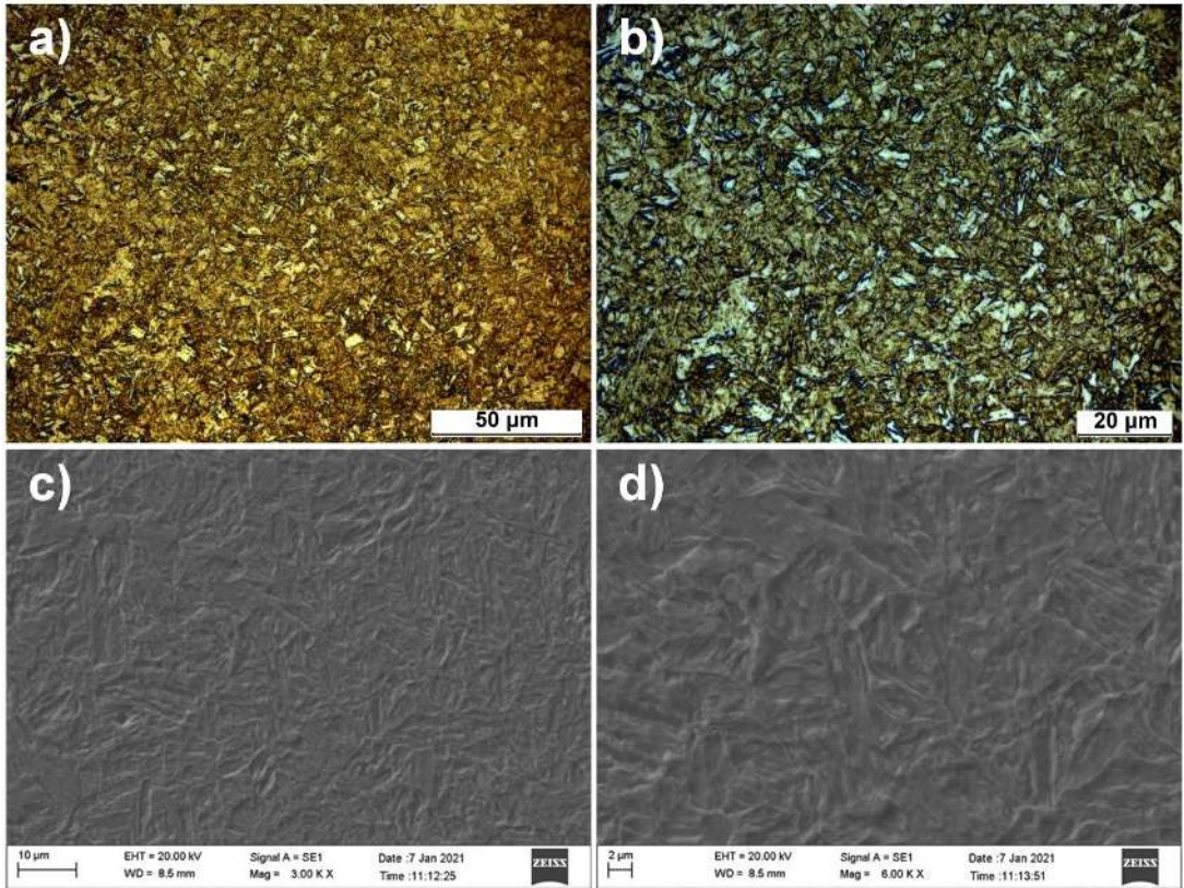
Şekil 5.40. S800 1,230 numunesine ait OM ve SEM görüntüleri
