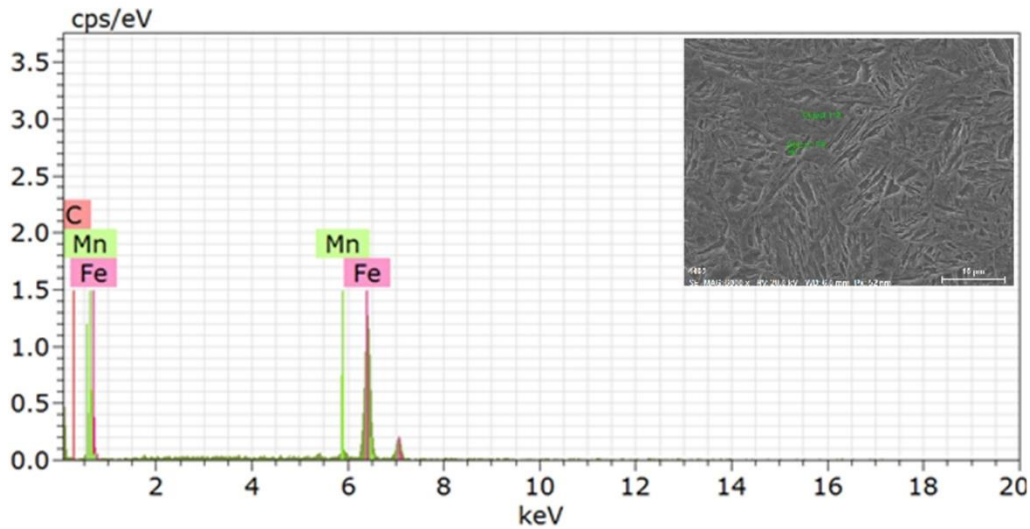
Şekil 5.75. N_0 numunesine ait EDS analizi grafiğı
