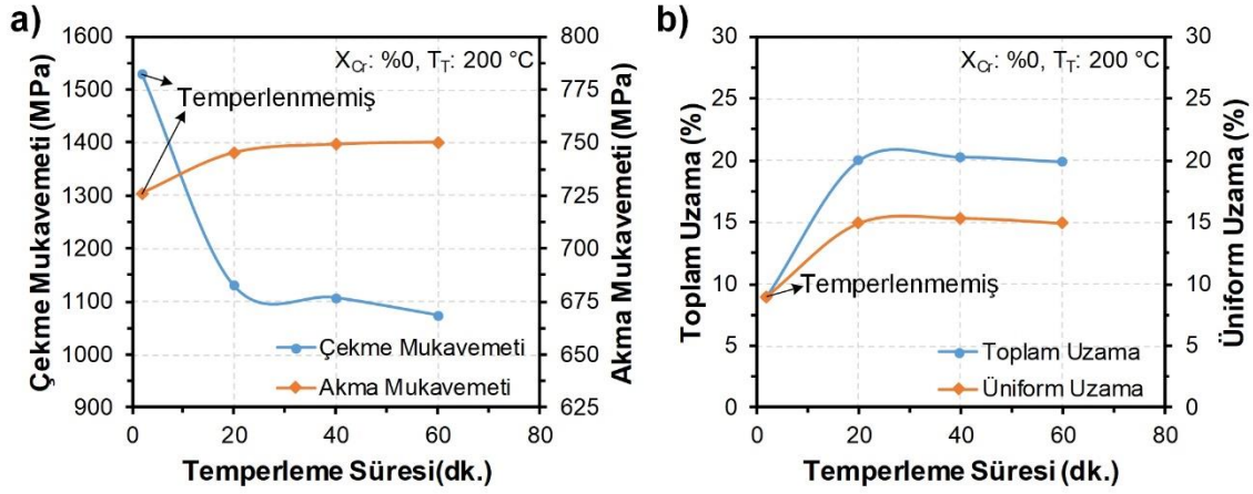
Şekil 5.160. Temperleme süresinin 0.16C-5.5Mn çeliğinin mekanik özellikleri üzerindeki etkisi, a) Çekme ve akma mukavemeti; b) Üniform ve toplam uzama miktarı
