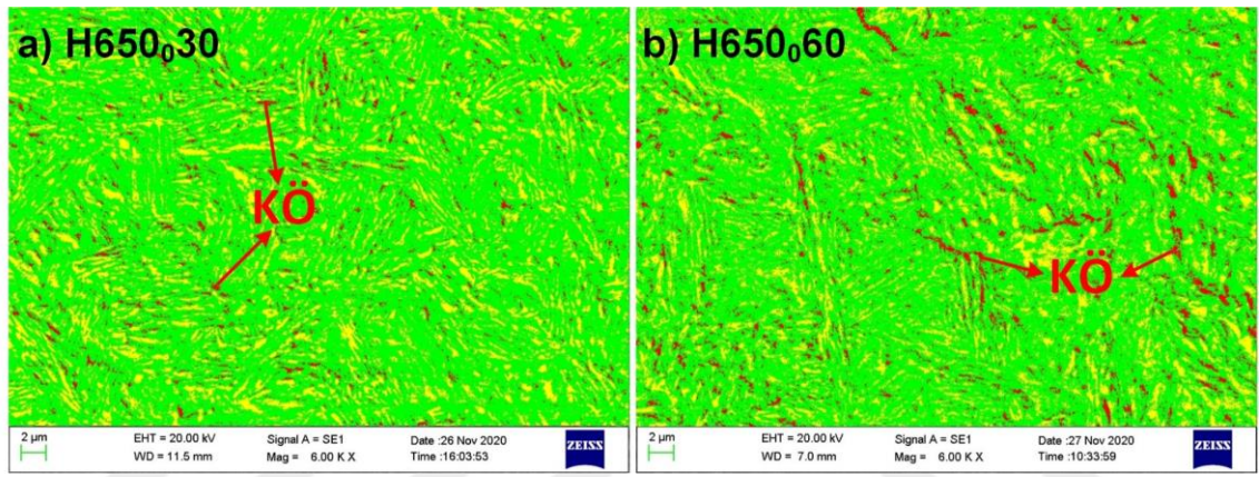
Şekil 5.47. Farklı sürelerde tavllanmış numunelere ait renklendirilmiş SEM görüntüleri; a) H650 0 30, b) H650 0 60
