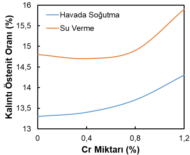
Şekil 5.112. 0.16C-5.5Mn çeliğine ilave edilen Cr'nin kalıntı östenit oranı üzerindeki etkisi
