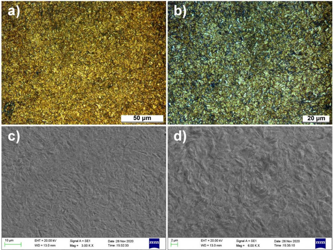
Şekil 5.49. S800 060 ( t_A : 60 dk.) numunesine ait OM ve SEM görüntüleri
