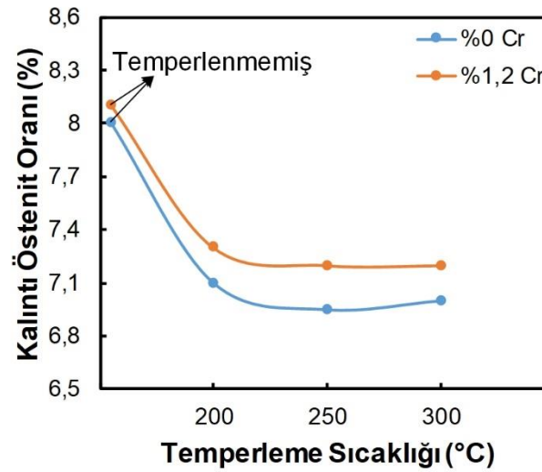
Şekil 5.124. Temperleme sıcaklığının kalıntı östenit oranı üzerindeki etkisi
