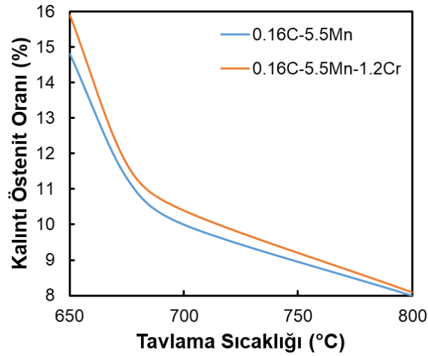
Şekil 5.86. Tavlama sıcaklığındaki değişimin kalıntı östenit oranı üzerindeki etkisi
