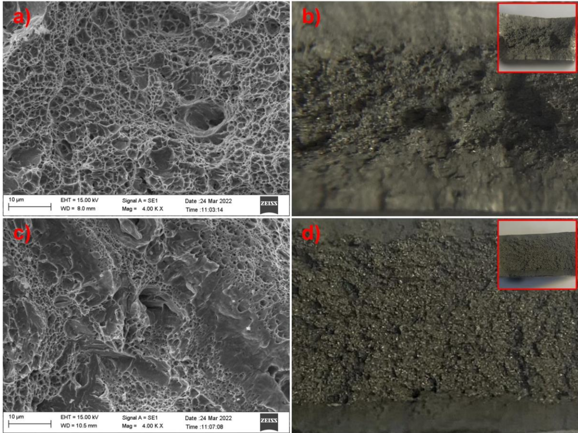
Şekil 5.146. Kopma yüzeylerinin SEM görüntüleri; a) H650 0 60, c) H650 1.2 60 ile makro görüntüleri; b) H650 0 60, d) H650 1.2 60
