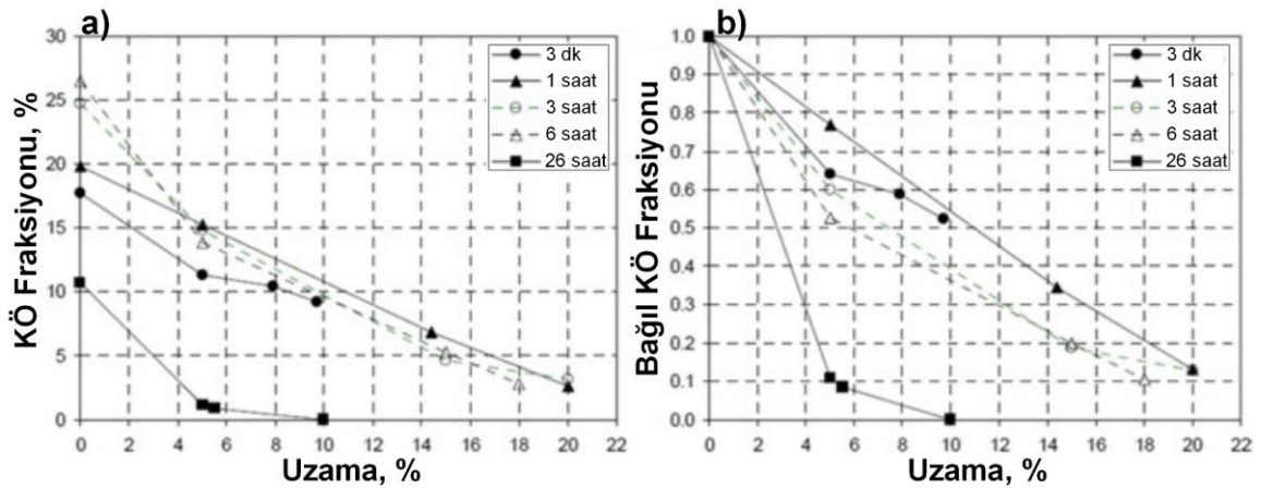
Şekil 3.20. Deformasyon miktarının bir fonksiyonu olarak kalıntı östenitin hacim fraksiyonunda (a) ve kalan kalıntı östenitin bağıl fraksiyonunda meydana gelen değişim (b) [5]
