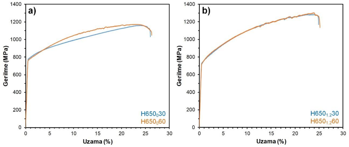
Şekil 5.145. 650 °C’de farklı sürelerde tavlanan Cr ilavesiz (a) ve %1.2 Cr ilaveli (b) numunelerin gerilme-uzama grafikleri
