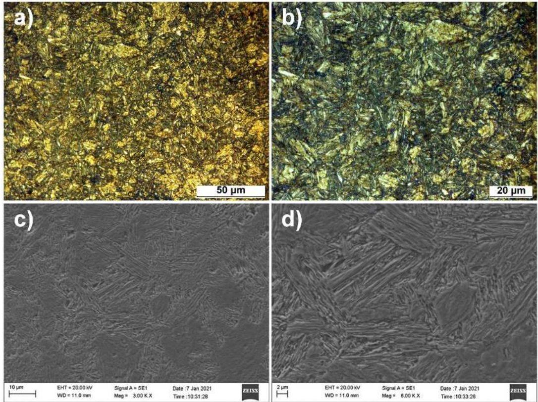
Şekil 5.61. %1.2 Cr ilaveli S650 1.2 30 numunesine ait OM ve SEM görüntüleri
