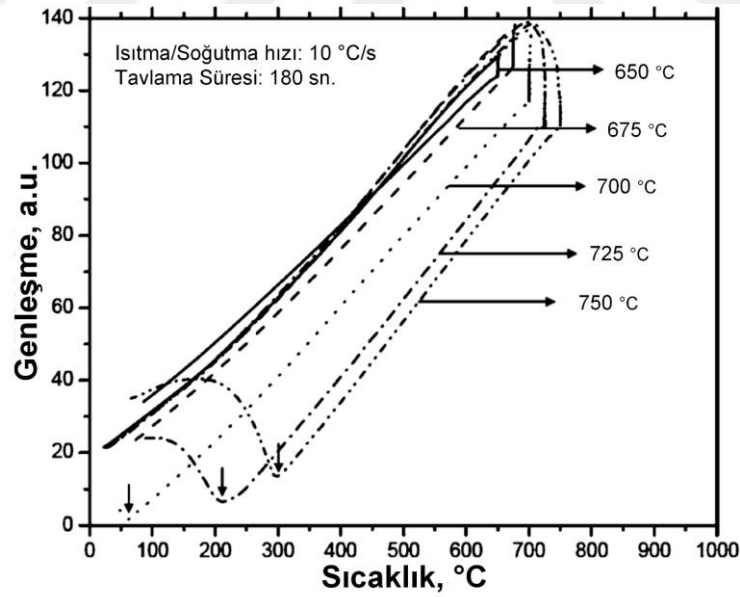
Şekil 3.3. Tavlama sıcaklığının genleşme eğrileri üzerindeki etkisi; T_A = 650 ve 675 °C’de hiçbir martenzit dönüşümü gözlenmemiştir, T_A = 700, 725, 750 °C’de soğutma sırasında martenzit dönüşümü gerçekleşmiştir [5]
