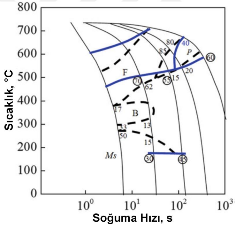
Şekil 2.27. 0.14C-1.0Mn-0.5Cr-0.003B çeliğinin kritik sıcaklık aralığından (mavi çizgiler) ve östenit bölgesinden (kesikli çizgiler) soğutulması sonrası CCT diyagramları [94]
