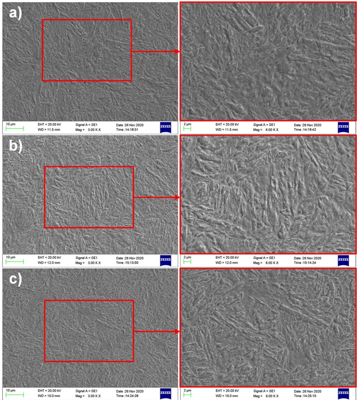
Şekil 5.74. T200 1,2 60, T250 1,2 60 ve T300 1,2 60 numunelerinin SEM görüntüleri; a) T200 1,2 60, b) T250 1,2 60, c) T300 1,2 60
