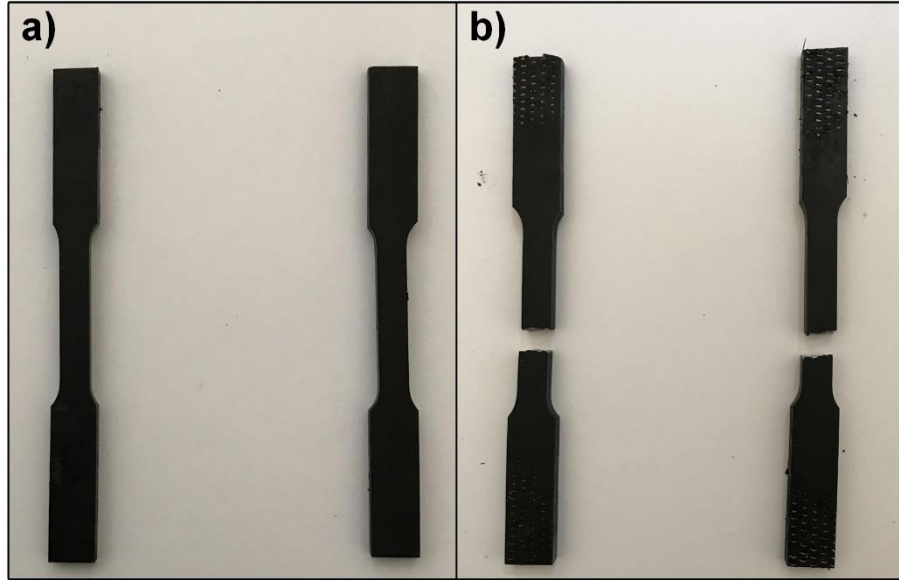
Şekil 4.19. Çekme testi numuneleri; a) Test öncesi, b) Test sonrası
