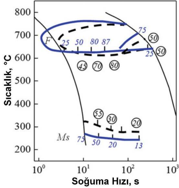
Şekil 2.31. İki fazlı bölgede bekleme süresinin östenit kararlılığı üzerindeki etkisini gösteren CCT diyagramı; 1 dakika (mavi çizgiler) ve 10 dakika (kesikli siyah çizgiler) [94]
