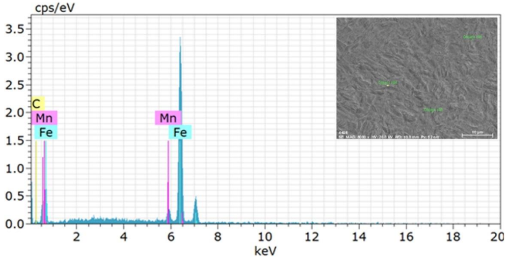
Şekil 5.98. S800 0 60 numunesine ait EDS analizi grafiği
