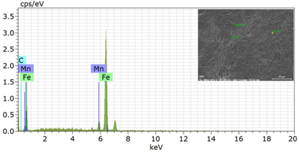
Şekil 5.107. S650 0,830 numunesine ait EDS analizi grafiği
