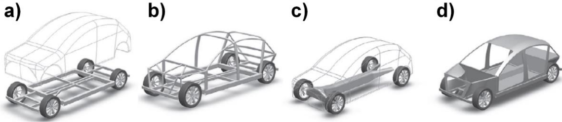
Şekil 2.33. Farklı otomobil gövde tasarımları; a) Şasi üzerine gövde, b) Uzak kafes gövde, c) Merkezi tünel yapısı ve d) Monokok yapı [131]
