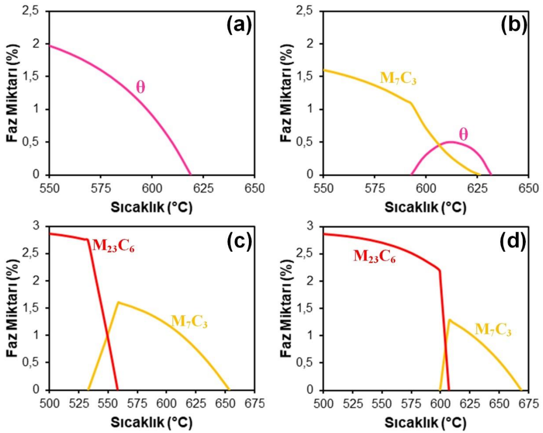
Şekil 5.12. Farklı oranlardaki Cr ilavesinin karbür oluşumları üzerindeki etkisi; a) %0 Cr, b) %0,4 Cr, c) %0,8 Cr, d) %1,2 Cr
