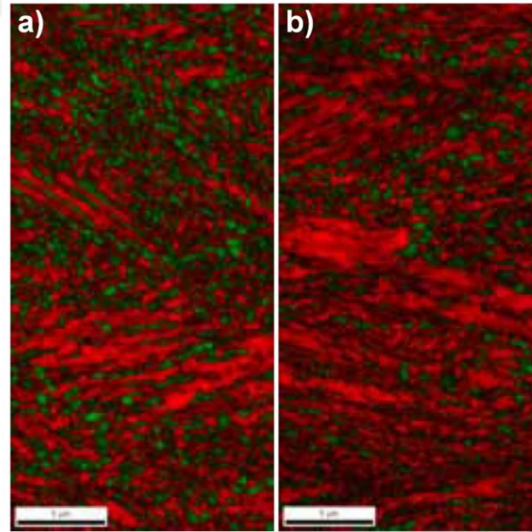
Şekil 3.13. %6.7 Mn çeliğinin EBSD faz haritaları; a) sıcak haddelenmiş, b) yığın halinde 550 °C'de toplu tavllanmış (kırmızı: HMK yapılı fazlar, yeşil: YMK yapılı östenit) [156]
