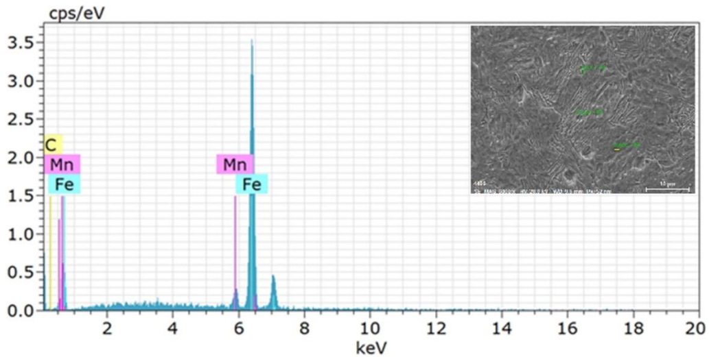
Şekil 5.97. H650 1,2 60 numunesine ait EDS analizi grafiği
