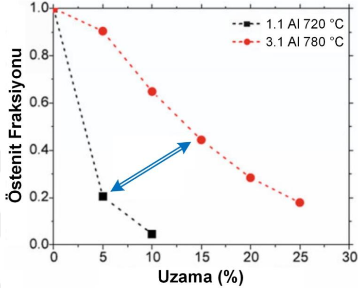
Şekil 3.14. %1.1 Al ve %3.1 Al içeren 0.12C-Mn çelikleri için normalize edilmiş östenit fraksiyonunun yüzde uzamaya göre değişimi [5]
