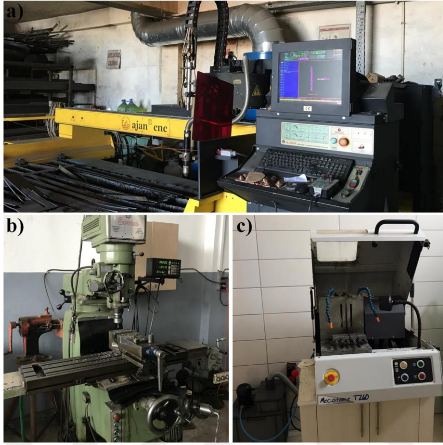
Şekil 4.6. Numune hazırlama işlemleri sırasında kullanılan cihazlar; a) Plazma kesim makinesi, b) Freze tezgâhı, c) Numune kesme cihazı
