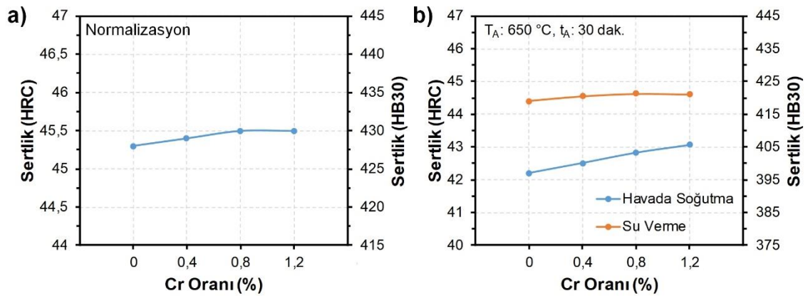
Şekil 5.127. Farklı oranlarda Cr içeren numunelerin sertlik grafiği; a) Normalizasyon, b) Kritik Tavlama
