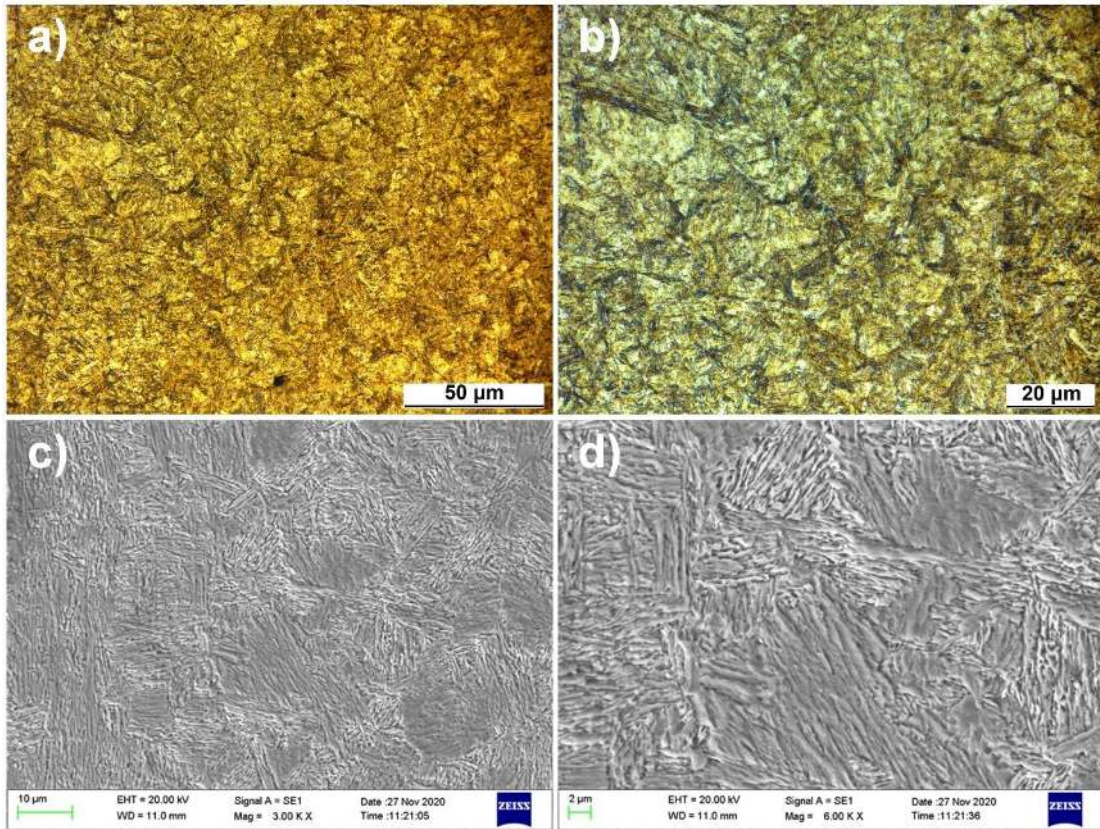
Şekil 5.33. S650030 numunesine ait OM ve SEM görüntüleri
