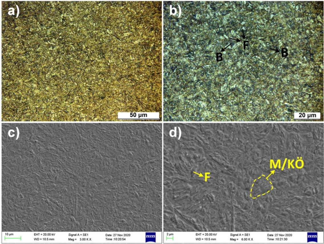
Şekil 5.27. H800 0 30 numunesine ait OM ve SEM görüntüleri
