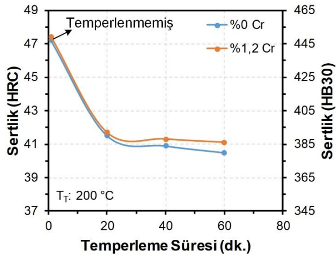
Şekil 5.130. Farklı sürelerde temperlenen numunelerin sertlik grafiği
