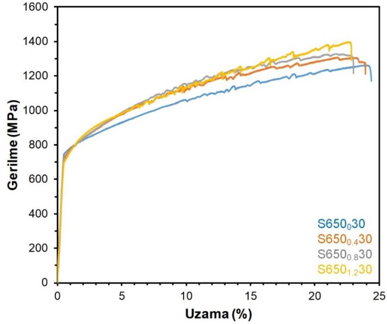
Şekil 5.149. S650 0.30 , S650 0.430 , S650 0.830 ve S650 1.230 numunelerinin gerilme-uzama grafikleri
