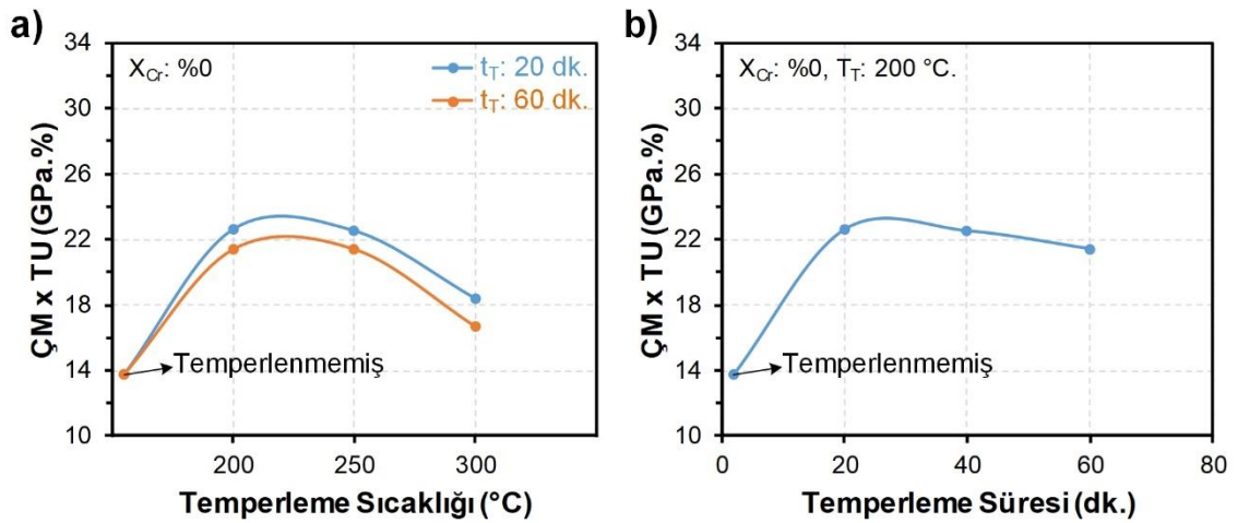
Şekil 5.168. Temperleme parametrelerinin 0.16C-5.5Mn çeliğinin \text{ÇM} - \text{TU} kombinasyonu üzerindeki etkisi; a) Temperleme Sıcaklığı, b) Temperleme Süresi
