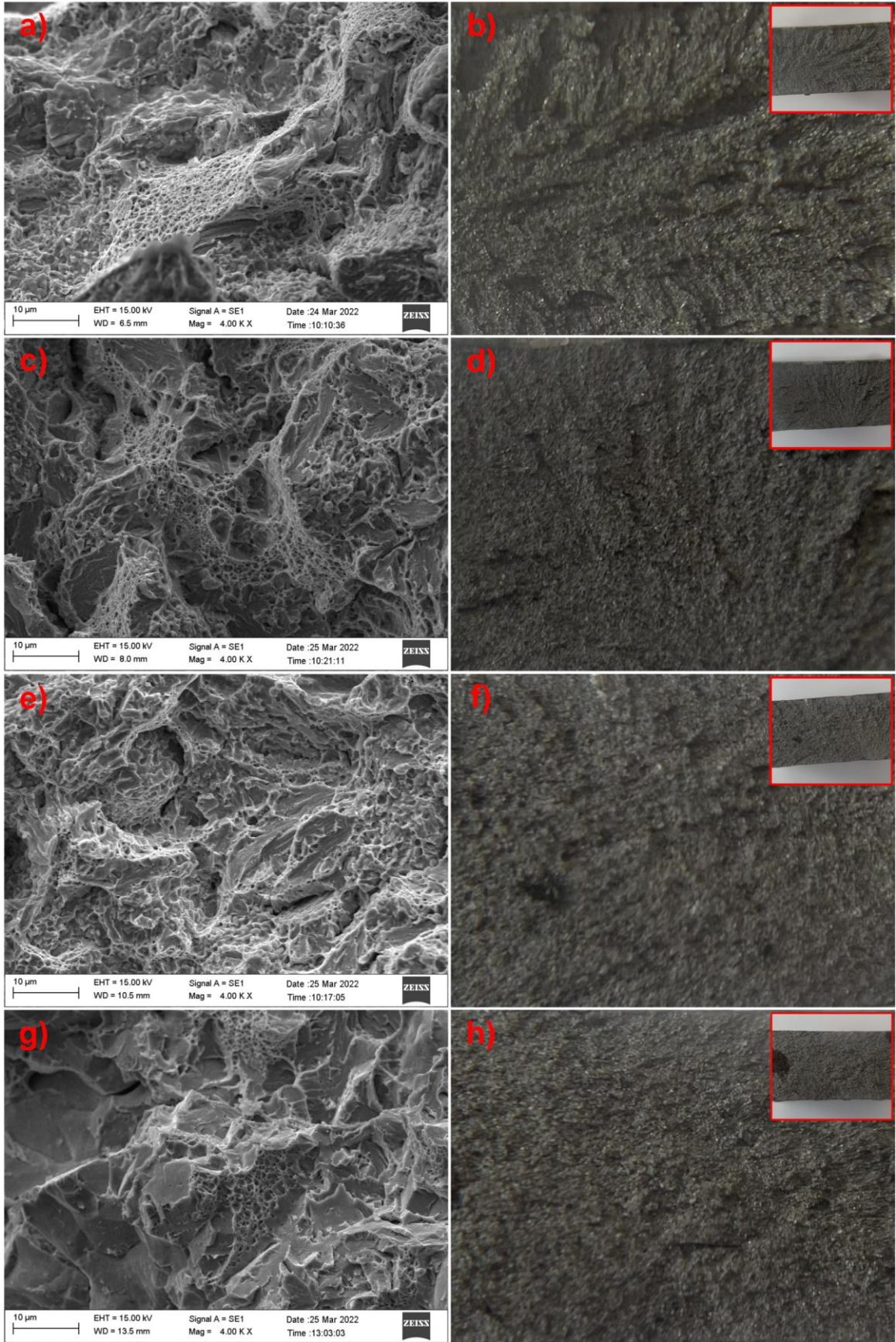
Şekil 5.136. Kopma yüzeylerinin SEM görüntüleri; a) S650 1,230 , c) S675 1,230 , e) S700 1,230 , g) S800 1,230 ile makro görüntüleri; b) S650 1,230 , d) S675 1,230 , f) S700 1,230 , h) S800 1,230
