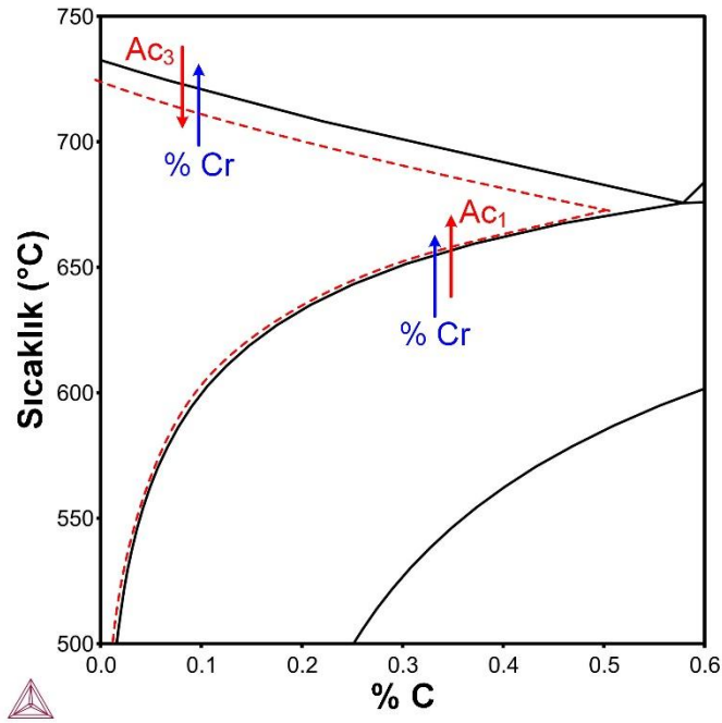
Şekil 5.4. Cr ilavesinin kritik sıcaklık aralığını üzerindeki etkisi
