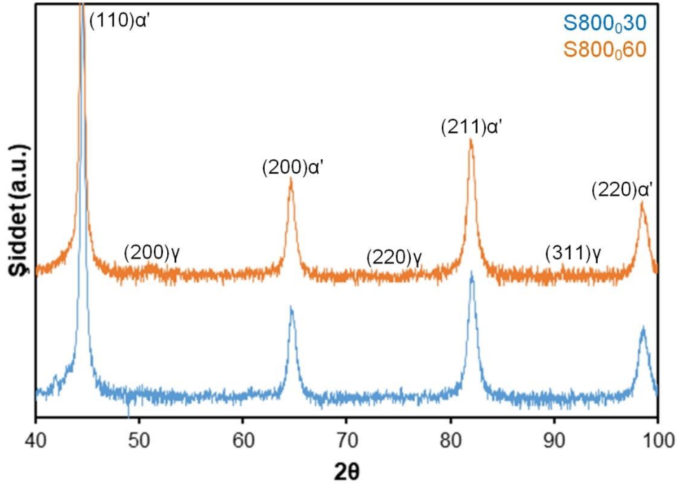
Şekil 5.103. S800 0 30 ve S800 0 60 numunelerine ait XRD analizi grafiği
