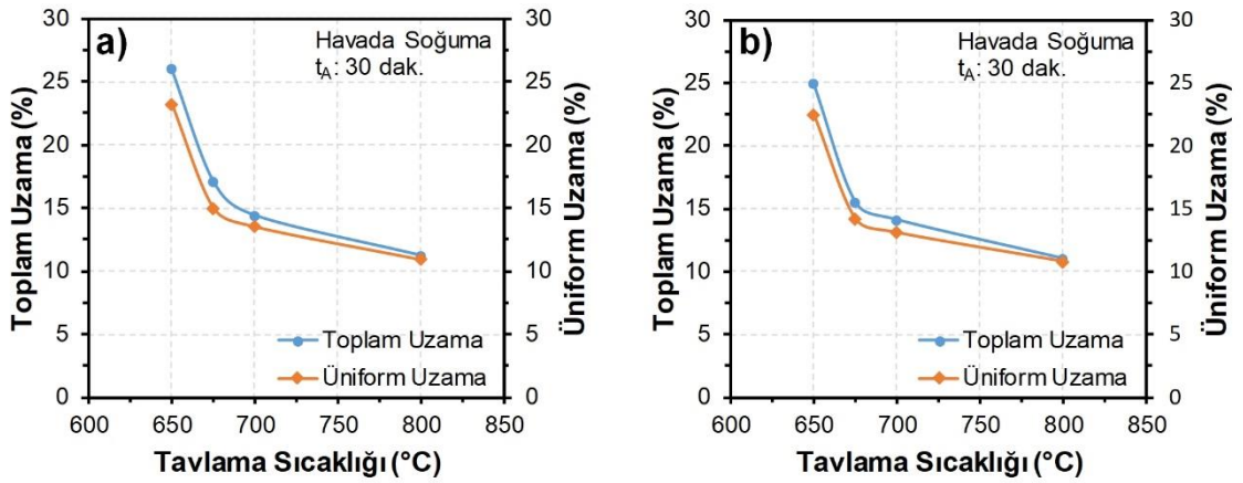
Şekil 5.144. Hava ortamında soğutulan Cr ilavesiz ve %1.2 Cr ilaveli numunelerin üniform ve toplam uzama miktarları; a) %0 Cr, b) %1.2 Cr
