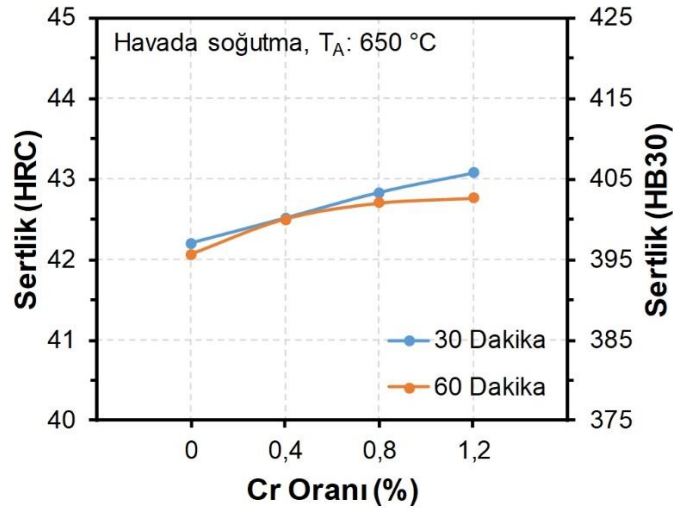
Şekil 5.128. 30 ve 60 dakika tavlama süresinin 0.16C-5.5Mn çeliğinin sertliği üzerindeki etkisi
