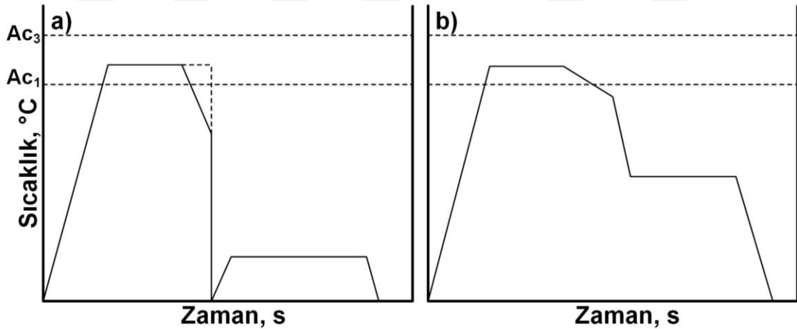
Şekil 2.18. Sürekli tavlama proseslerinin ana termal profilleri; (a) su verme, (b) doğrudan soğutma [94]
