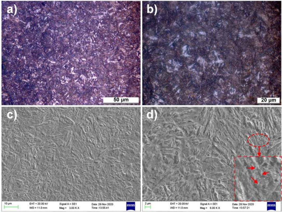
Şekil 5.63. T200 0 20 numunesine ait OM ve SEM görüntüleri
