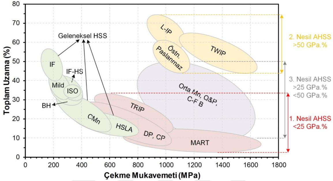
Şekil 2.1. Geleneksel HSS ve AHSS türleri için mukavemet-uzama ilişkisi [35, 36]
