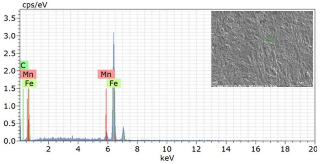
Şekil 5.117. T250 1,220 numunesine ait EDS analizi grafiği
