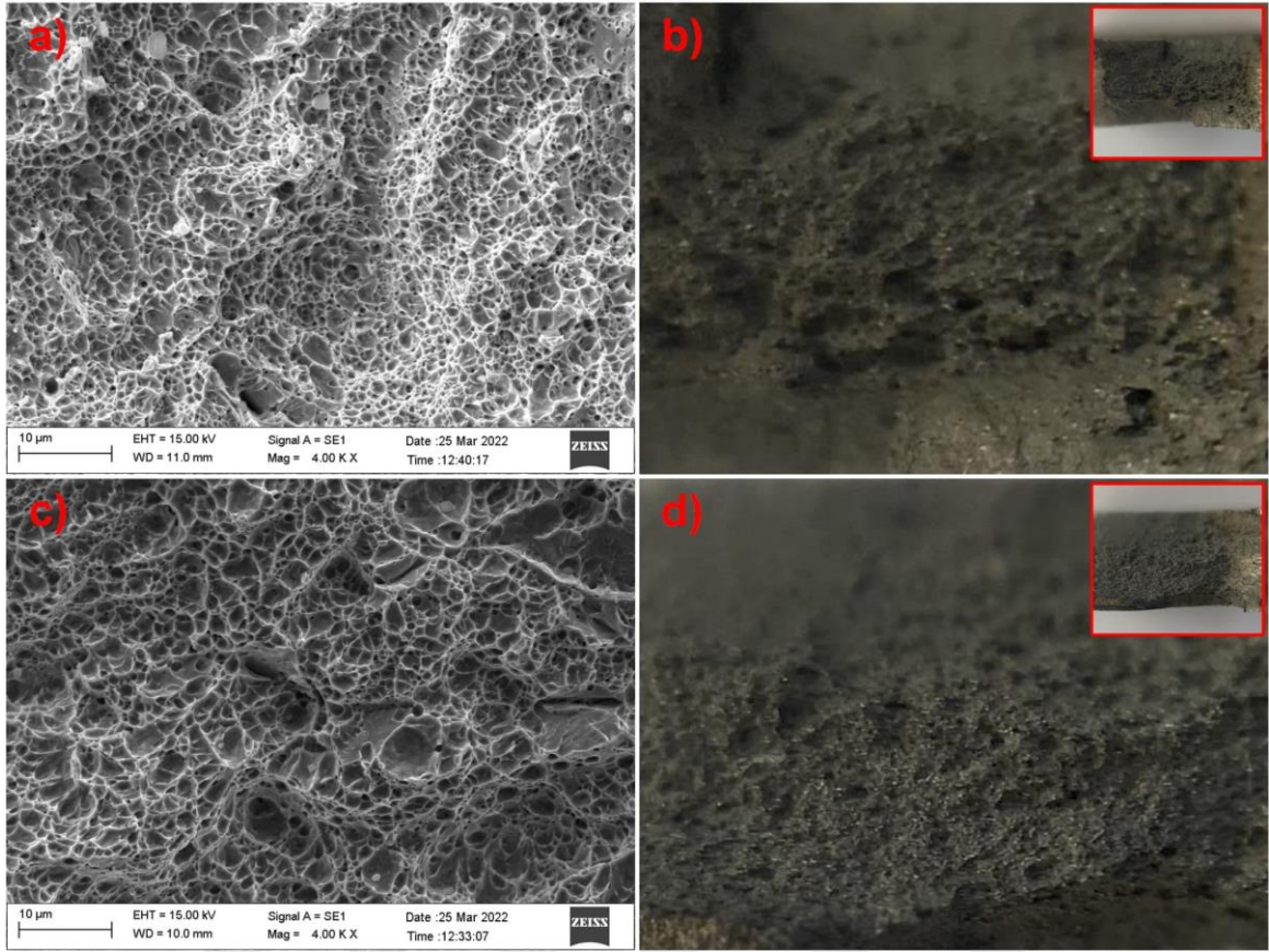
Şekil 5.159. Kopma yüzeylerinin SEM görüntüleri; a) T200 40 , c) T200 60 ile makro görüntüleri; b) T200 40 , d) T200 60
