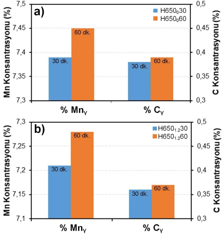
Şekil 5.100. Tavlama süresine bağlı olarak kalıntı östenit bileşiminde meydana gelen değişimi; a) 0.16C-5.5Mn, b) 0.16C-5.5Mn-1.2Cr
