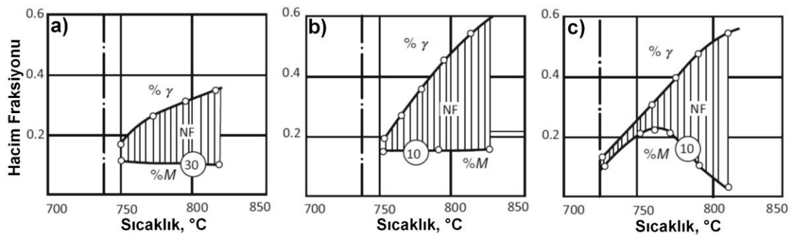
Şekil 2.32. Soğutma hızına bağlı olarak tavlama sıcaklığının oluşan östenit ve martenzit fraksiyonu üzerindeki etkisi; a) 0.08\text{C}-1.35\text{Mn}-0.35\text{Si}-0.08\text{V} çeliği, soğutma hızı 30^{\circ}\text{C/s} ; b) 0.065\text{C}-1.21\text{Mn}-0.6\text{Si}-0.003\text{B} çeliği, soğutma hızı 10^{\circ}\text{C/s} ; c) 0.065\text{C}-1.2\text{Mn}-0.2\text{Cr}-0.1\text{Mo} çeliği, soğutma hızı 10^{\circ}\text{C/s} [94]
