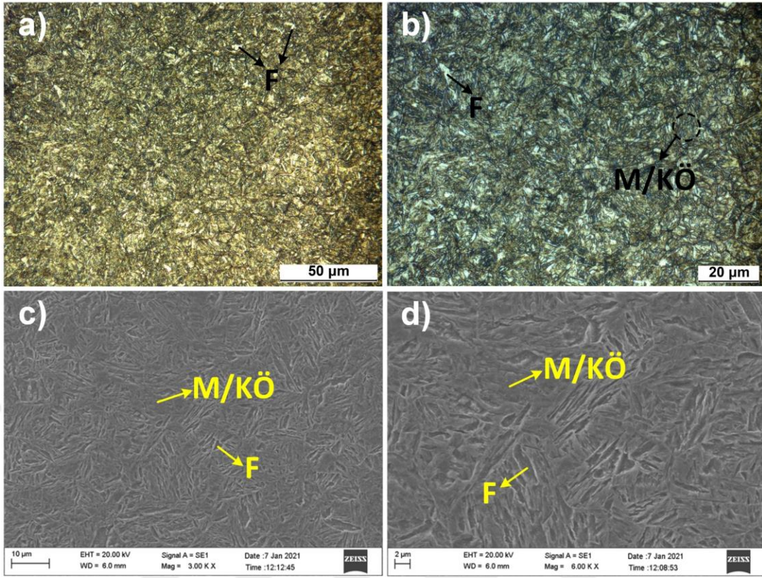
Şekil 5.20. N_0 numunesine ait OM ve SEM görüntüleri
