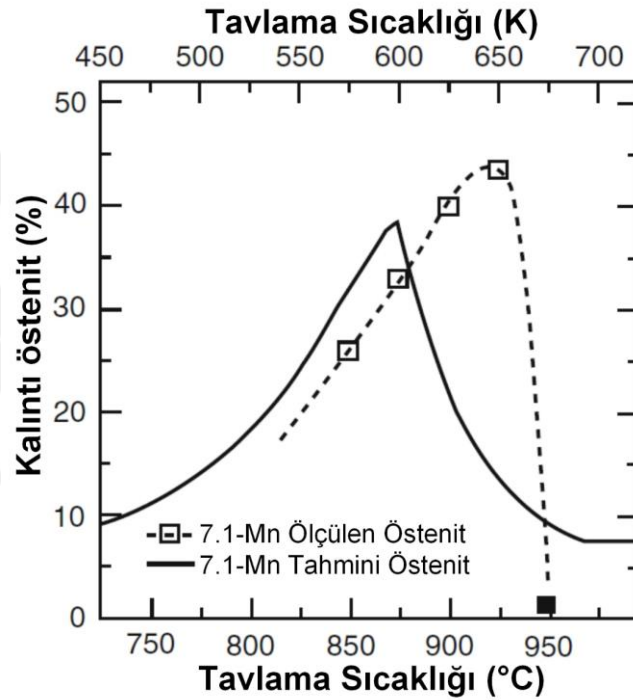
Şekil 3.4. 0.1C-7.1Mn-0.12Si çeliğinde tavlama sıcaklığına bağlı olarak östenit hacim fraksiyonunda meydana gelen değişim [75]
