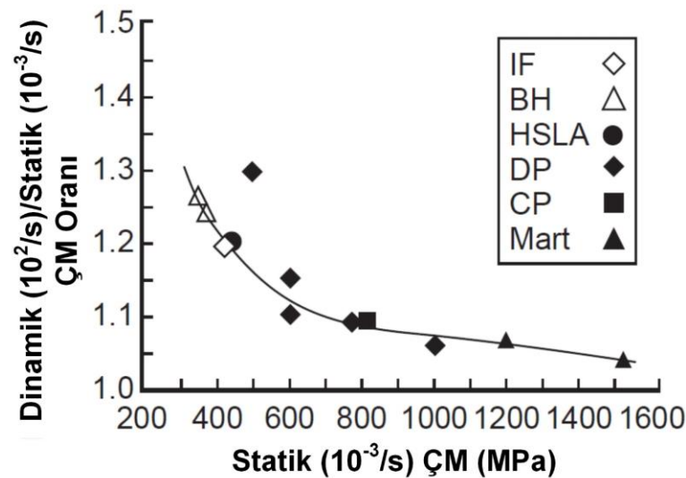
Şekil 2.35. Bir dizi farklı çelik için artan çekme mukavemeti ile gerinme hızındaki artışın bir sonucu olarak gerilme mukavemetindeki artışın azalması [45]
