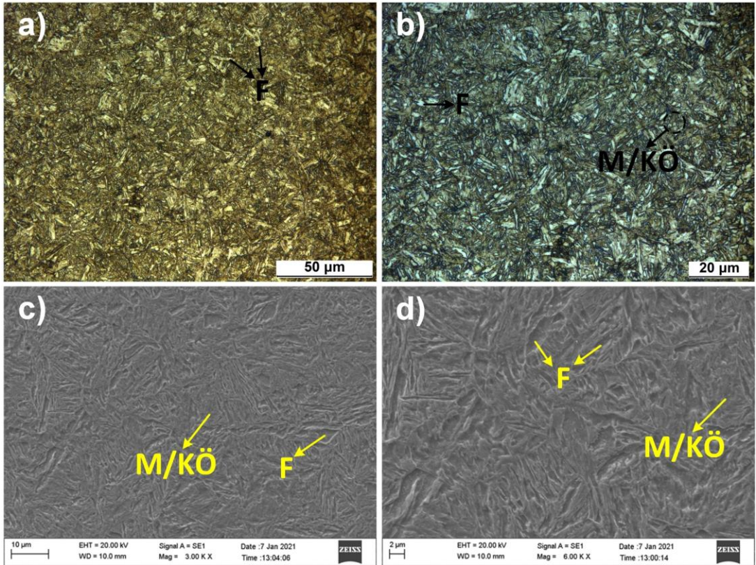
Şekil 5.23. N_{1.2} numunesine ait OM ve SEM görüntüleri
