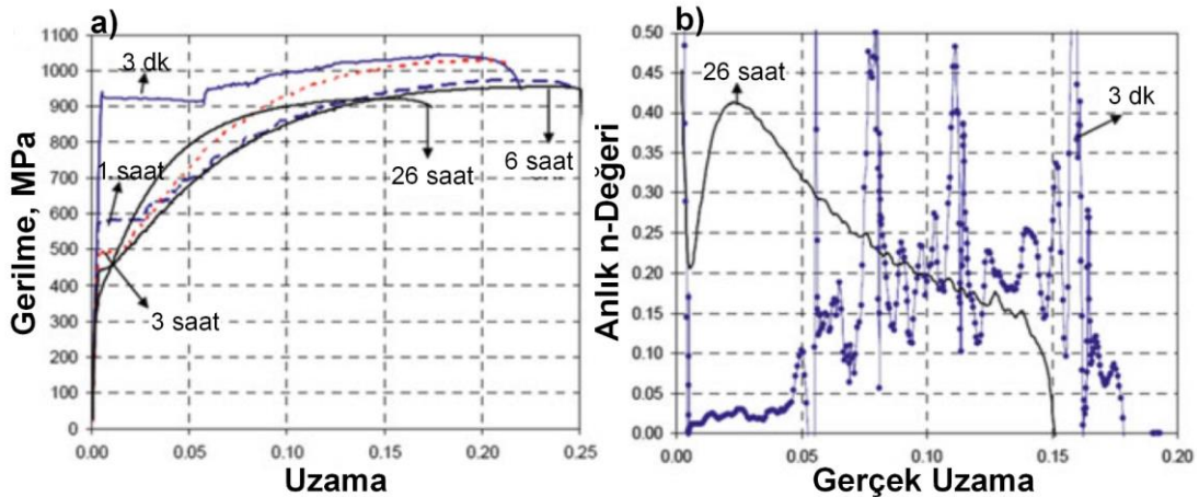
Şekil 3.19. Farklı tavlama sürelerine ait gerilme-uzama eğrileri (a) ve anlık n değerleri (b) [5]
