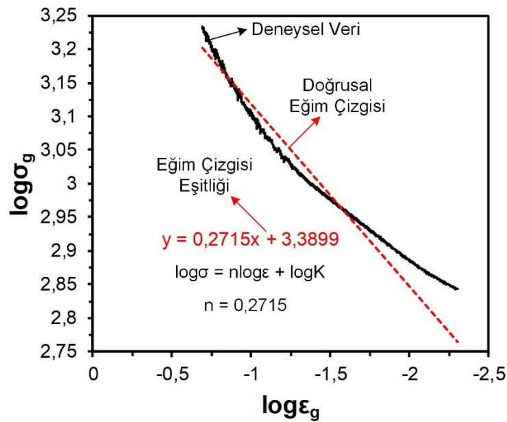
Şekil 4.20. Pekleşme üssünün ( n değeri) tespiti
