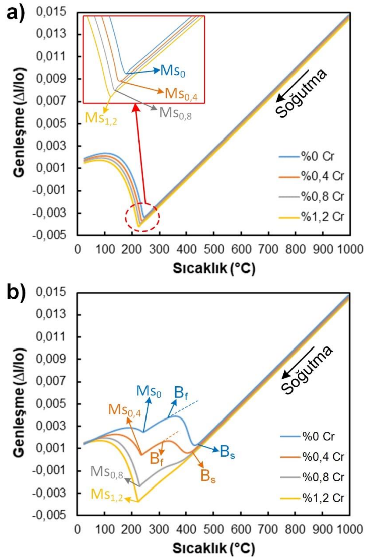
Şekil 5.111. Farklı oranlarda Cr içeren 0.16C-5.5Mn çeliklerine ait genleşme eğrileri; a) Su verme, b) Havada soğutma
