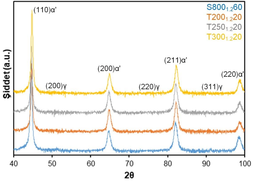
Şekil 5.122. S800 1,2 60, T200 1,2 20, T250 1,2 20, T300 1,2 20 numunelerine ait XRD analizi grafiği
