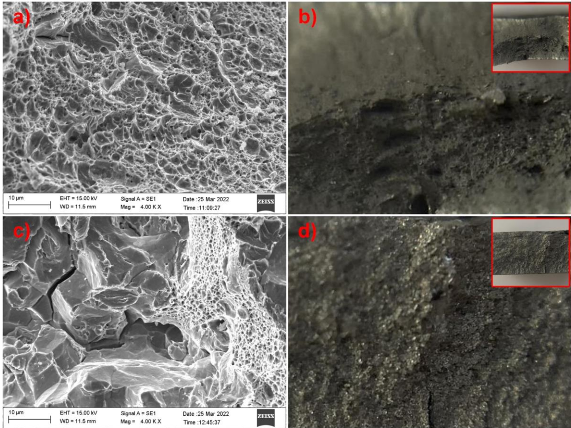
Şekil 5.162. Kopma yüzeylerinin SEM görüntüleri; a) T250 60 , c) T300 60 ile makro görüntüleri; b) T250 60 , d) T300 60
