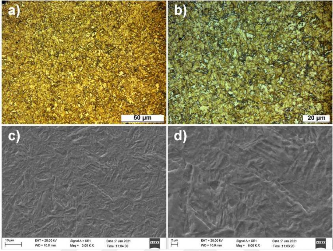
Şekil 5.48. S800 030 ( t_A : 30 dk.) numunesine ait OM ve SEM görüntüleri
