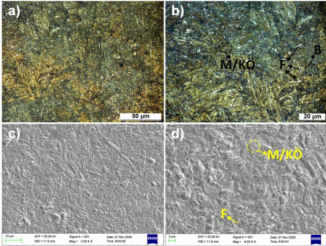
Şekil 5.29. H650 1,2 30 numunesine ait OM ve SEM görüntüleri
