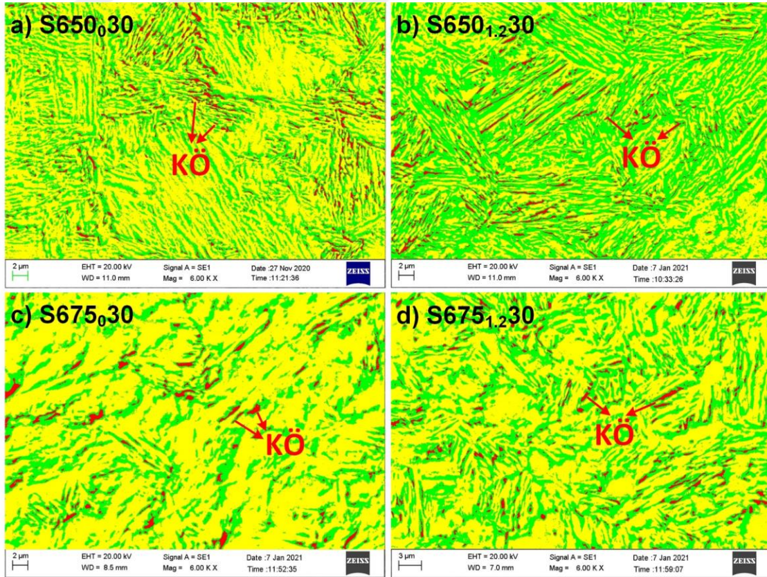
Şekil 5.41. Renklendirilmiş SEM görüntüleri üzerinde kalıntı östenit fazının (kırmızı) gösterimi
