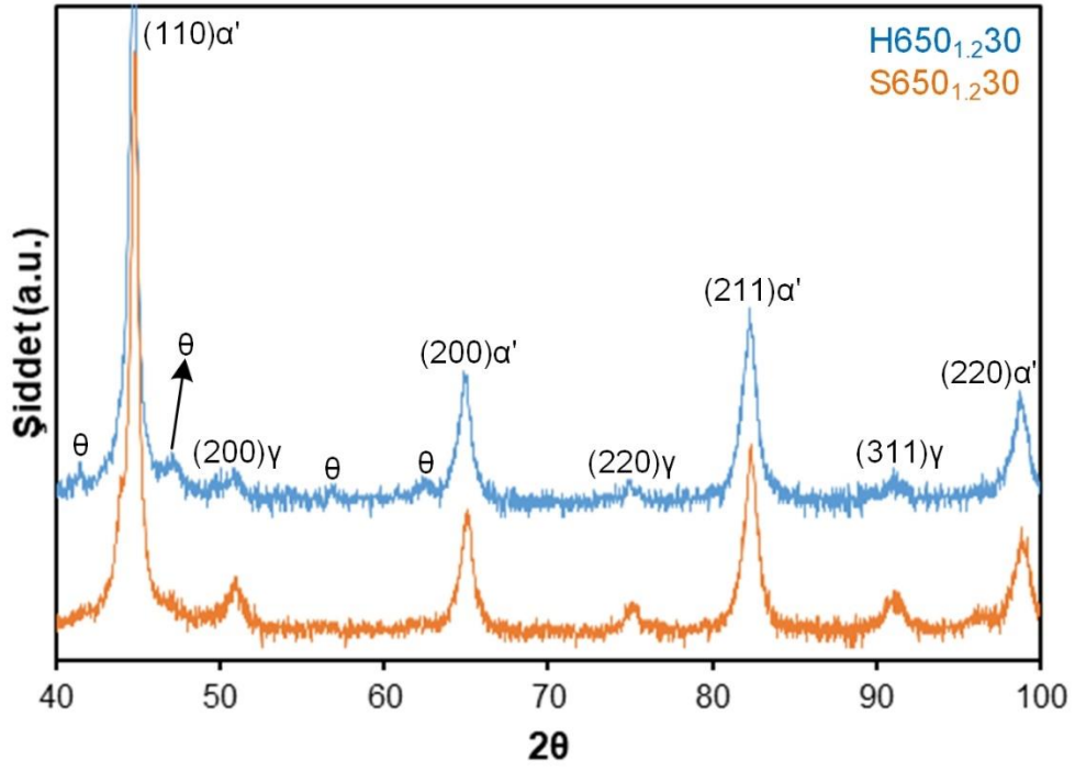
Şekil 5.93. S650 1,230 ve H650 1,230 numunelerine ait XRD analizi grafiği
