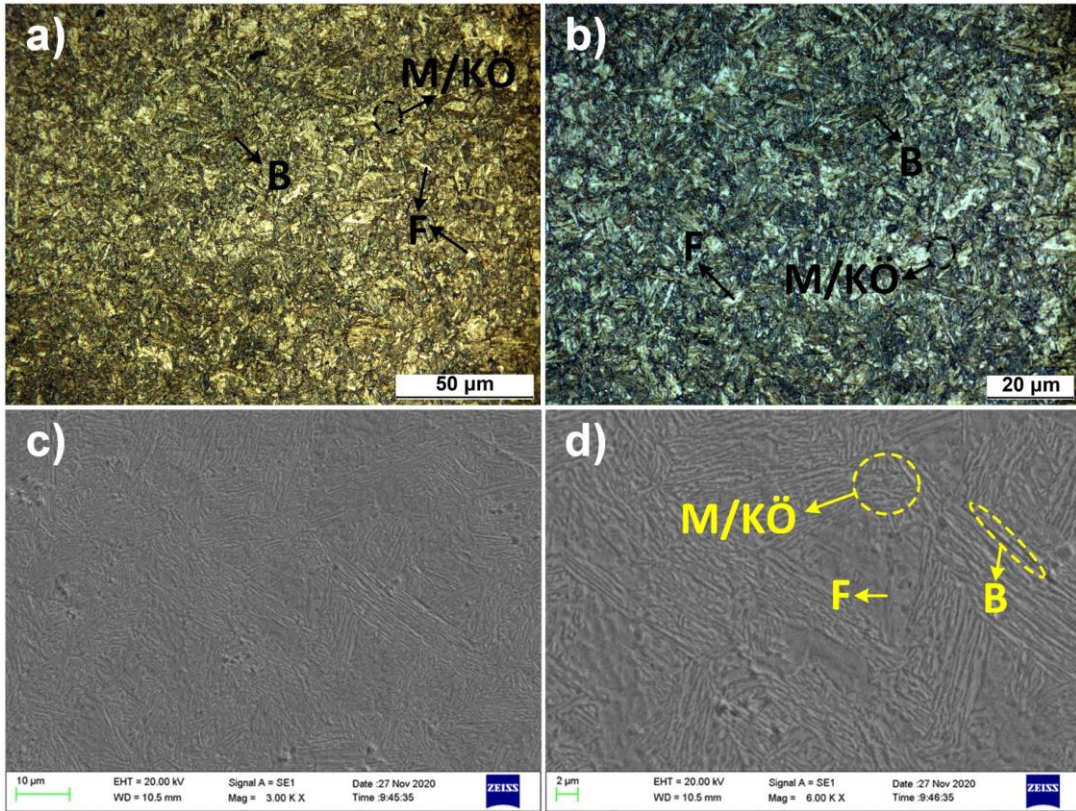
Şekil 5.54. %0.8 Cr ilaveli H650 0,830 numunesine ait OM ve SEM görüntüleri
