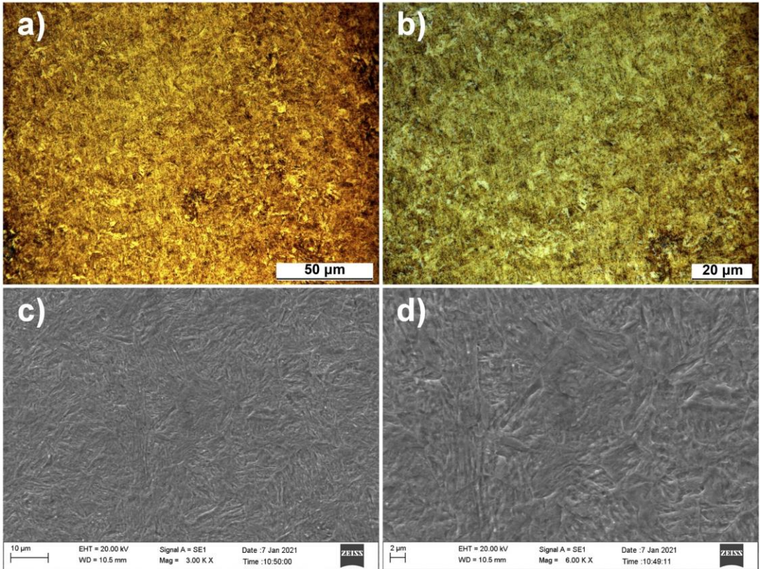
Şekil 5.35. S700 0 30 numunesine ait OM ve SEM görüntüleri
