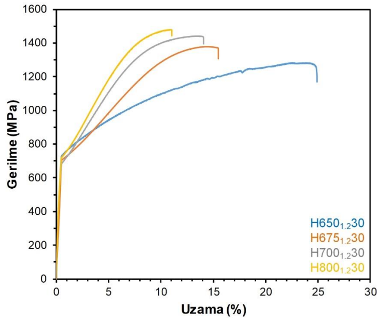
Şekil 5.140. H650 1,2 30, H675 1,2 30, H700 1,2 30 ve H800 1,2 30 numunelerinin gerilme-uzama grafikleri
