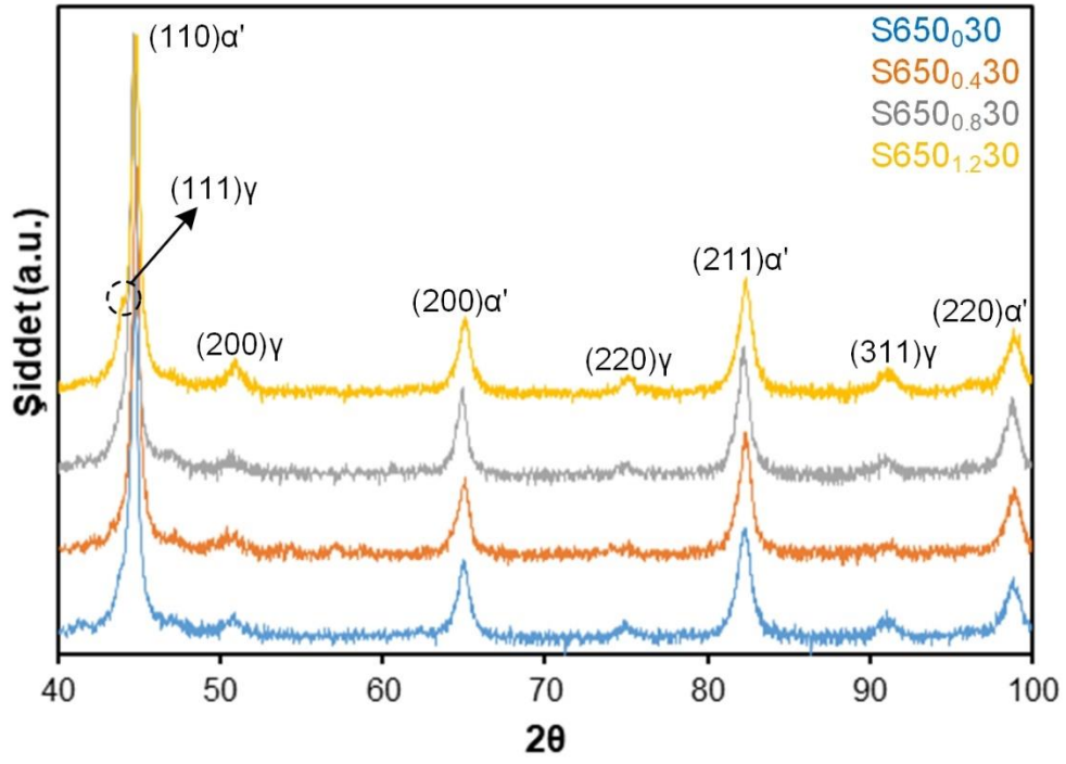
Şekil 5.109. S650 0.30 , S650 0.430 , S650 0.830 ve S650 1.230 numunelerine ait XRD analizi grafiği
