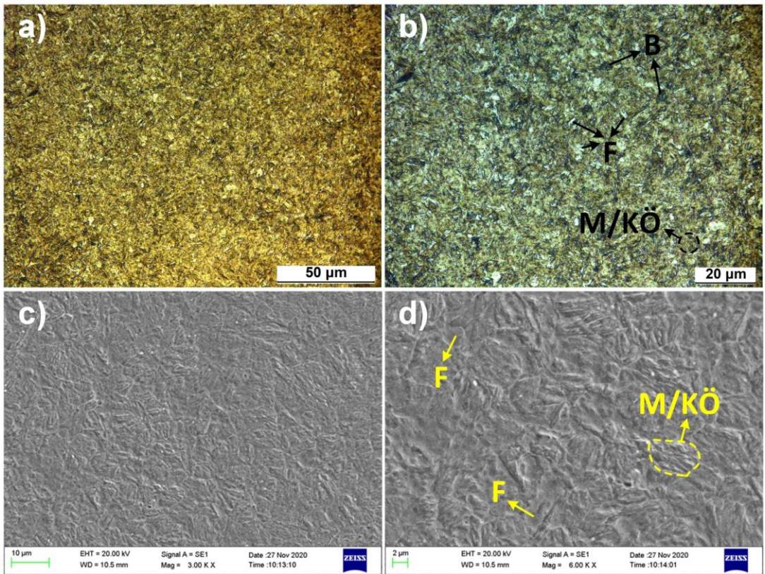
Şekil 5.26. H700 0 30 numunesine ait OM ve SEM görüntüleri
