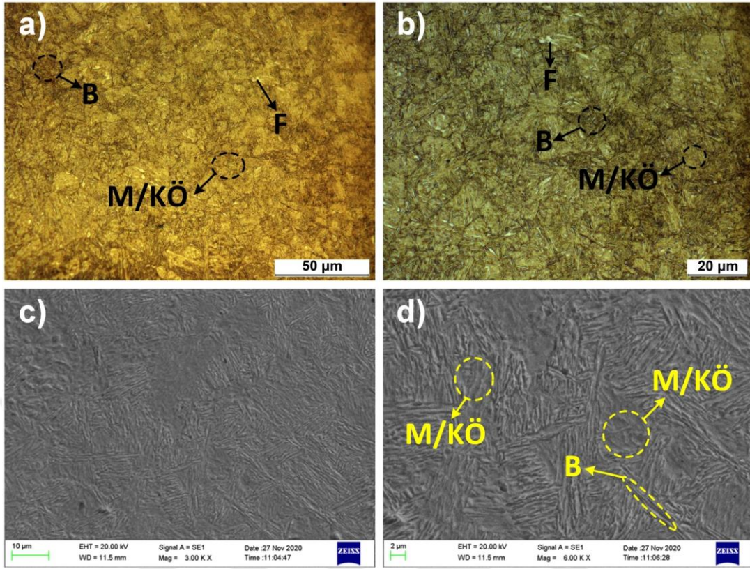
Şekil 5.44. H650 0,4 60 numunesine ait OM ve SEM görüntüleri
