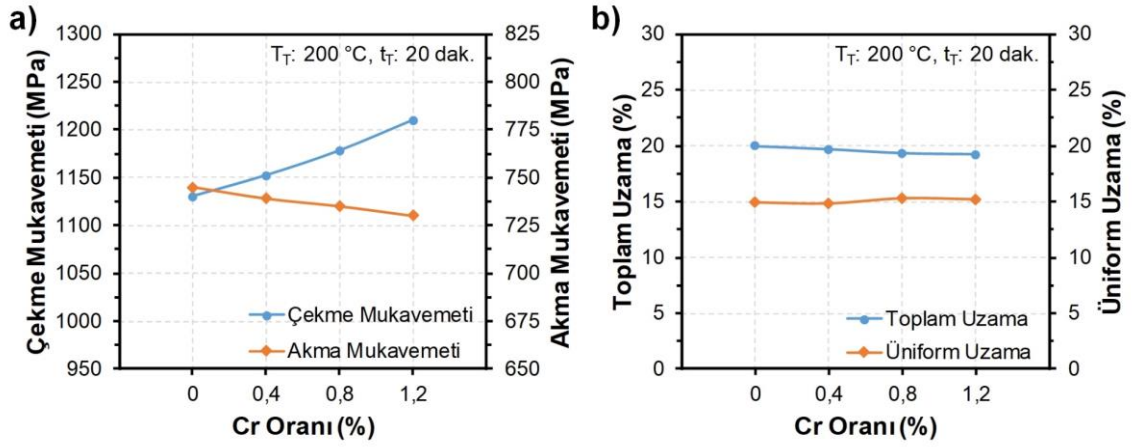
Şekil 5.164. Temperlenen numunelerde Cr oranının 0.16C-5.5Mn çeliğinin mekanik özellikleri üzerindeki etkisi; a) Çekme ve akma mukavemeti, b) Üniform ve toplam uzama miktarı
