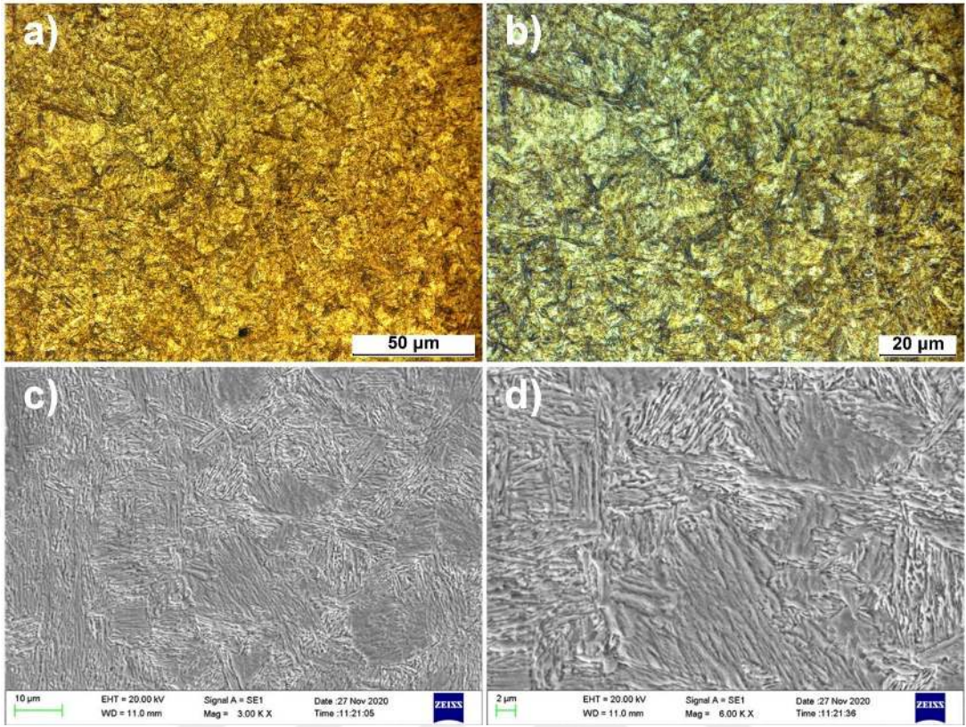
Şekil 5.58. Cr ilavesiz S650 0 30 numunesine ait OM ve SEM görüntüleri
