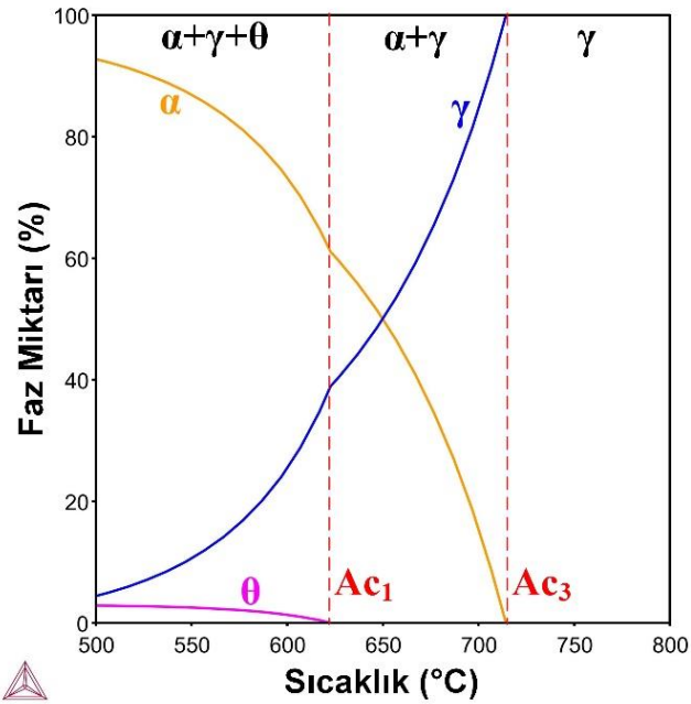
Şekil 5.10. Fe-0.16C-5.5Mn çeliği için faz miktarlarının sıcaklığa göre değişimi
