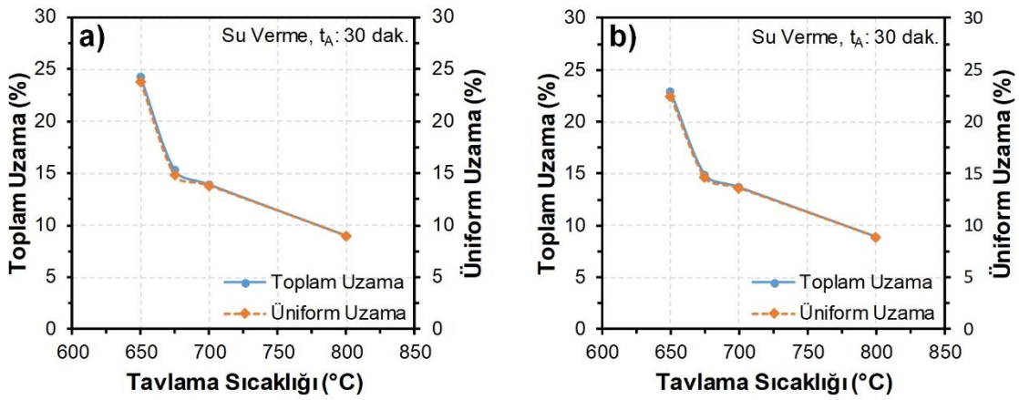
Şekil 5.138. Tavlama sıcaklığına bağlı olarak Cr ilavesiz ve %1.2 Cr ilaveli numunelerin üniform ve toplam uzama miktarlarında meydana gelen değişimler; a) %0 Cr, b) %1.2 Cr
