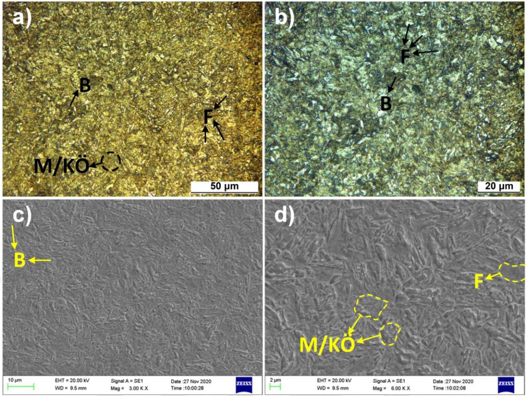
Şekil 5.25. H675 0 30 numunesine ait OM ve SEM görüntüleri
