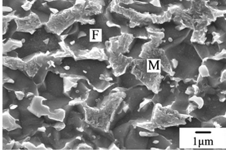
Şekil 2.3. Tipik bir DP çeliği mikroyapısının SEM görüntüsü (F: Ferrit, M: Martenzit) [46]
