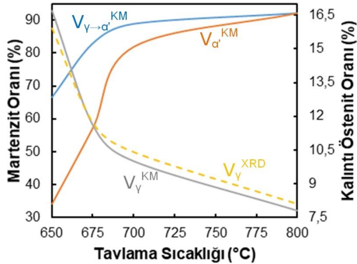
Şekil 5.87. Koistinen – Marburger eşitliğine göre tavlama sıcaklığına bağlı olarak östenit – martenzit dönüşümünde meydana gelen değişim
