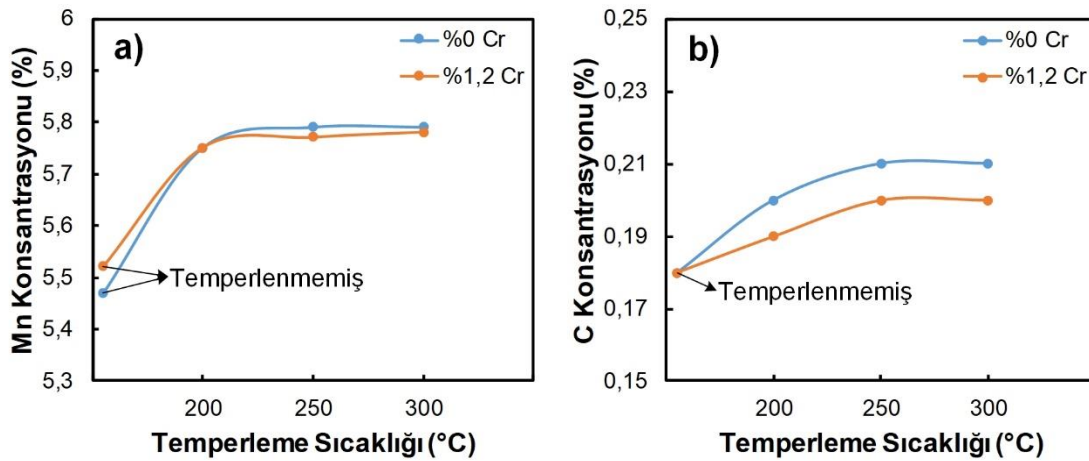
Şekil 5.120. Temperleme sıcaklığına bağlı olarak kalıntı östenitin Mn ve C içeriğinde meydana gelen değişimler; a) % Mn, b) % C
