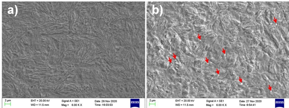
Şekil 5.56. Cr ilavesi ile karbür oluşumunda meydana gelen artış; a) H650 030 , b) H650 1,230
