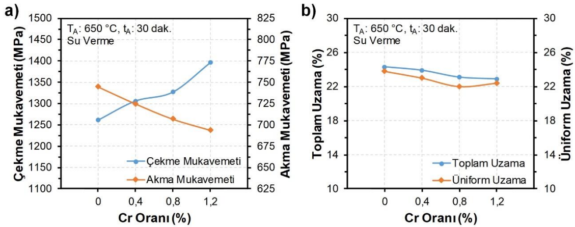
Şekil 5.151. Cr oranının 0.16C-5.5Mn çeliğinin mekanik özellikleri üzerindeki etkisi, a) Çekme ve akma mukavemeti; b) Üniform ve toplam uzama miktarı
