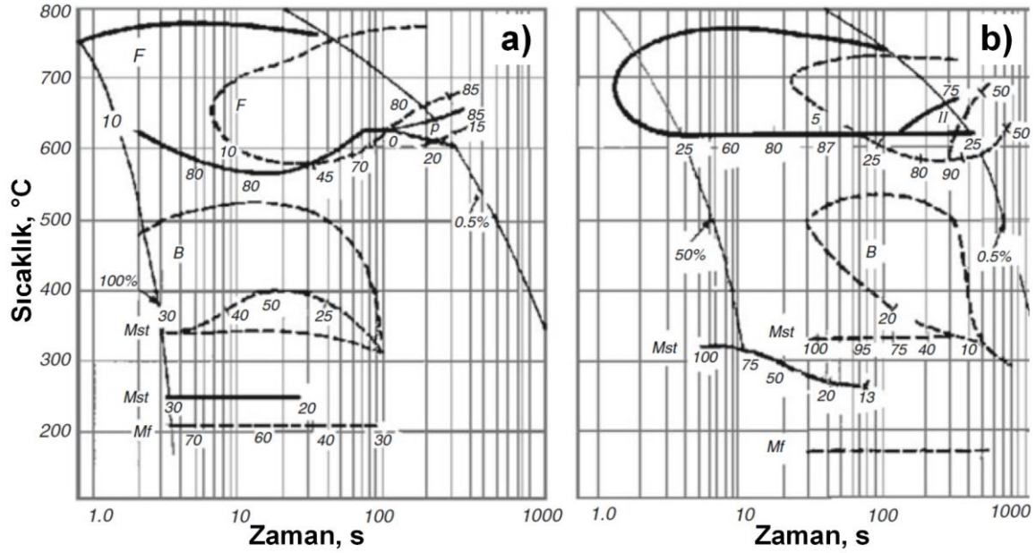
Şekil 2.29. 800 °C (a) ve 780 °C (b) 'den soğutulmuş 0.06C-1.2Mn-0.5Si-0.5Cr çeliği (düz çizgiler) ile tamamen östenitlenmiş %0.18 (a) ve %0.3 (b) C'li Mn-Cr-Si çeliklerinin (kesikli çizgiler) CCT diyagramları [94]
