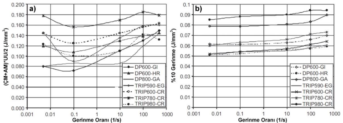
Şekil 2.36. TRIP ve DP çelikleri için gerinme oranının boyun verme (a) ve %10 uzama miktarı (b) sırasında enerji emilimi üzerindeki etkisi [93]
