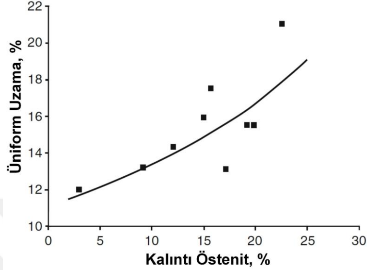
Şekil 3.5. Kalıntı östenit fraksiyonunun üniform uzama üzerindeki etkisi [6]
