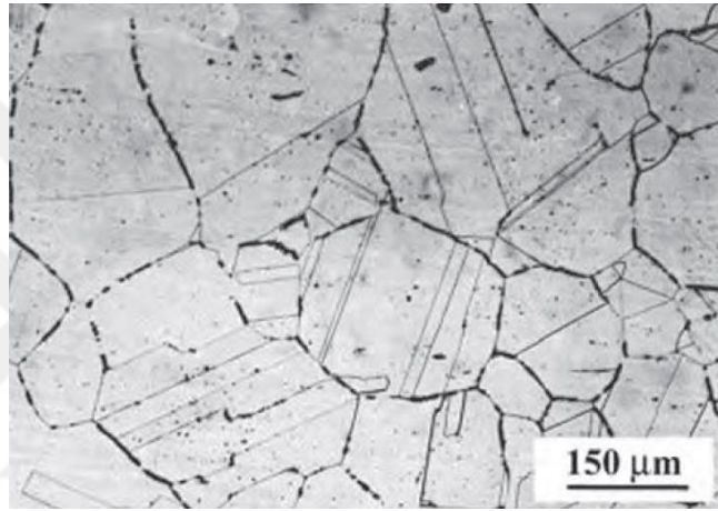
Şekil 2.10. Tavlanmış östenitik paslanmaz tip 302 çeliğine ait mikroyapı görüntüsü [61]
