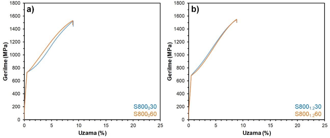
Şekil 5.147. 800 °C’de farklı sürelerde tavlanan Cr ilavesiz (a) ve %1.2 Cr ilaveli (b) numunelerin gerilme-uzama grafikleri
