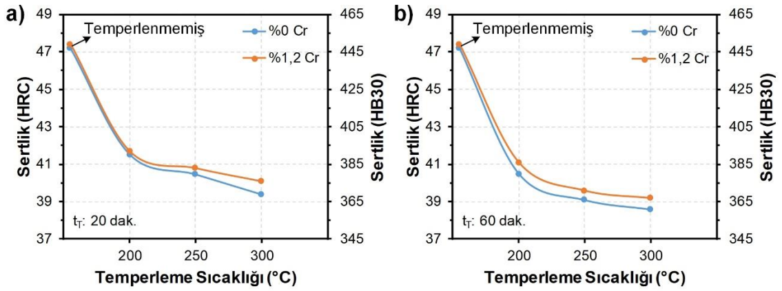
Şekil 5.129. Farklı sıcaklıklarda temperlenen numunelerin sertlik grafiği; a) 20 dk. temperleme, b) 60 dk. temperleme
