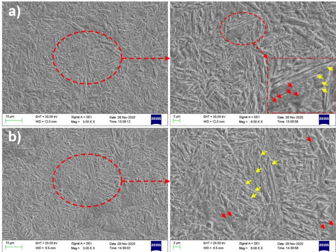
Şekil 5.68. T250 60 ve T300 60 numunelerine ait SEM görüntüleri; a) T250 60 , b) T300 60
