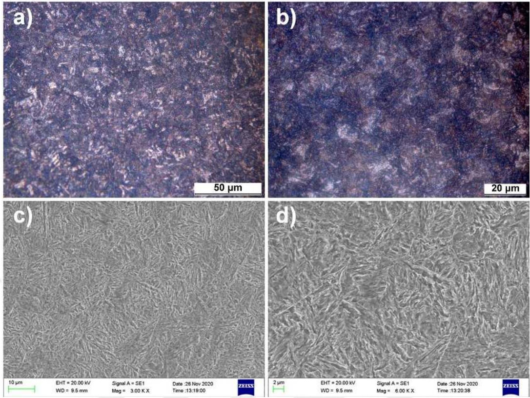
Şekil 5.71. %0.8 Cr ilaveli T200 0.8 20 numunesine ait OM ve SEM görüntüleri
