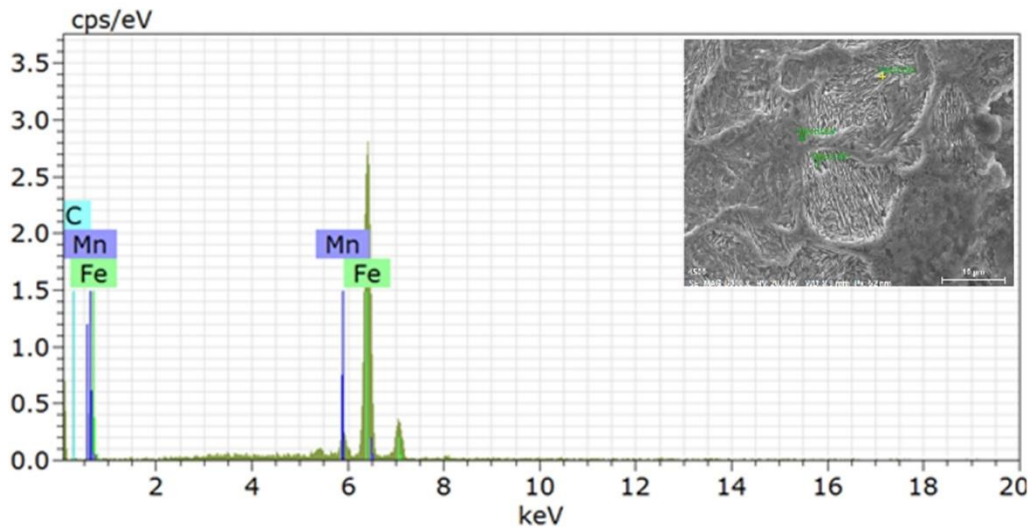
Şekil 5.89. H650 0 30 numunesine ait EDS analizi grafiği
