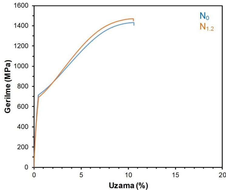
Şekil 5.132. Normalize edilmiş N_0 ve N_{1.2} numunelerinin gerilme-uzama grafikleri
