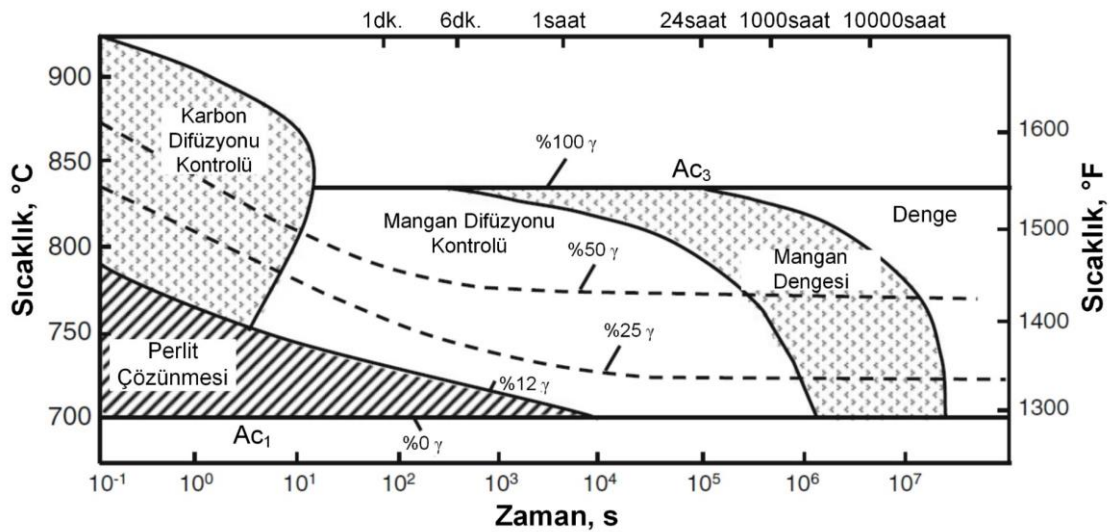
Şekil 2.19. 0.12C-1.5Mn çeliği için sıcaklığa ve zamana bağlı olarak östenitleşme evrelerini gösteren diyagram [96]
