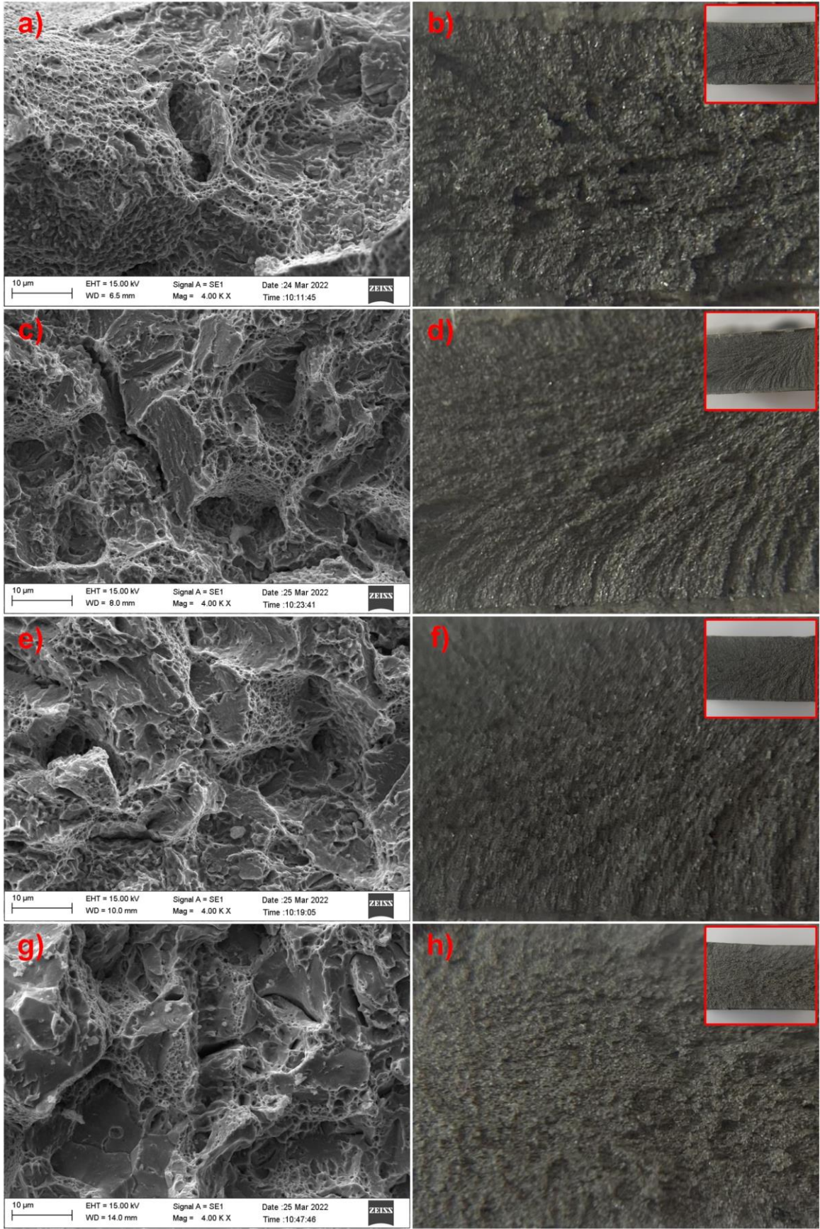
Şekil 5.135. Kopma yüzeylerinin SEM görüntüleri; a) S650 30 , c) S675 30 , e) S700 30 , g) S800 30 ile makro görüntüleri; b) S650 30 , d) S675 30 , f) S700 30 , h) S800 30
