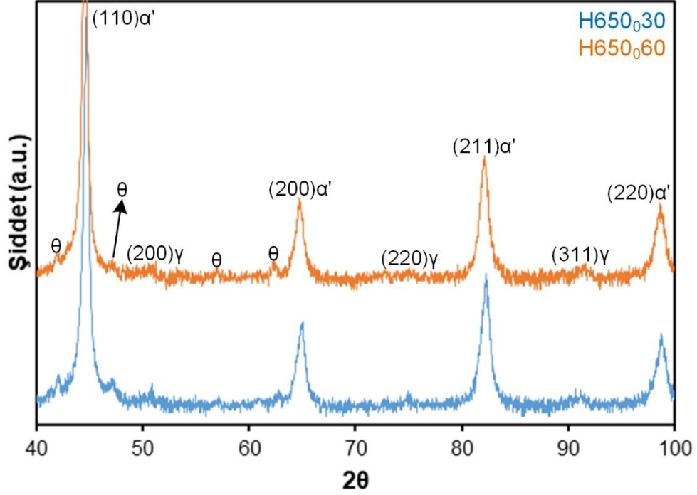
Şekil 5.101. H650 030 ve H650 060 numunelerine ait XRD analizi grafiği
