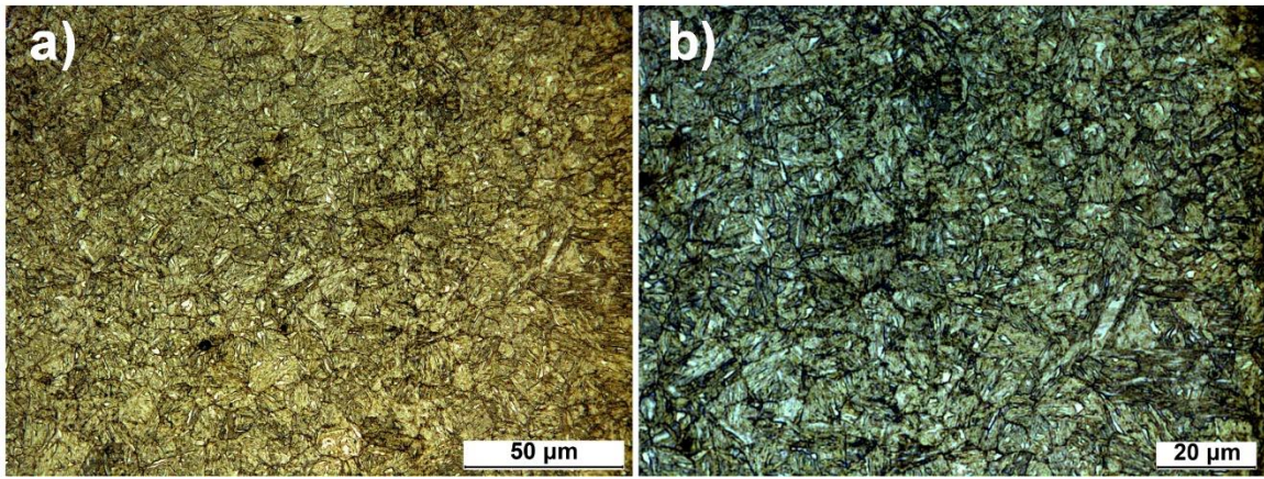
Şekil 5.42. 600 °C’ deki tavlama işlemi sonrası elde edilen OM görüntüleri; a) 40x, b) 63x
