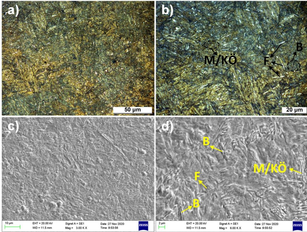
Şekil 5.55. %1.2 Cr ilaveli H650 1,230 numunesine ait OM ve SEM görüntüleri
