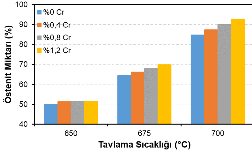
Şekil 5.14. Kritik bölgedeki tavlama sıcaklıkları için östenit fazı oranları
