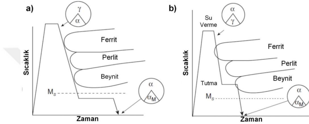
Şekil 2.2. DP ve TRIP çeliklerinin tipik üretim döngüleri; a) DP, b) TRIP ( \alpha : Ferrit, \alpha_M : Martenzit ve \gamma : östenit) [30]
