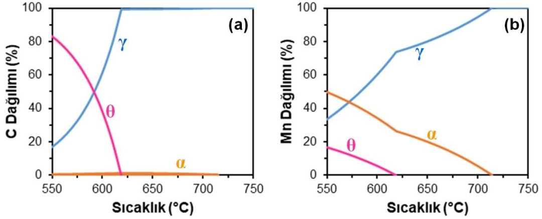
Şekil 5.17. Fe-0.16C-5.5Mn çeliğinde görülen fazlara ait C ve Mn dağılımları
