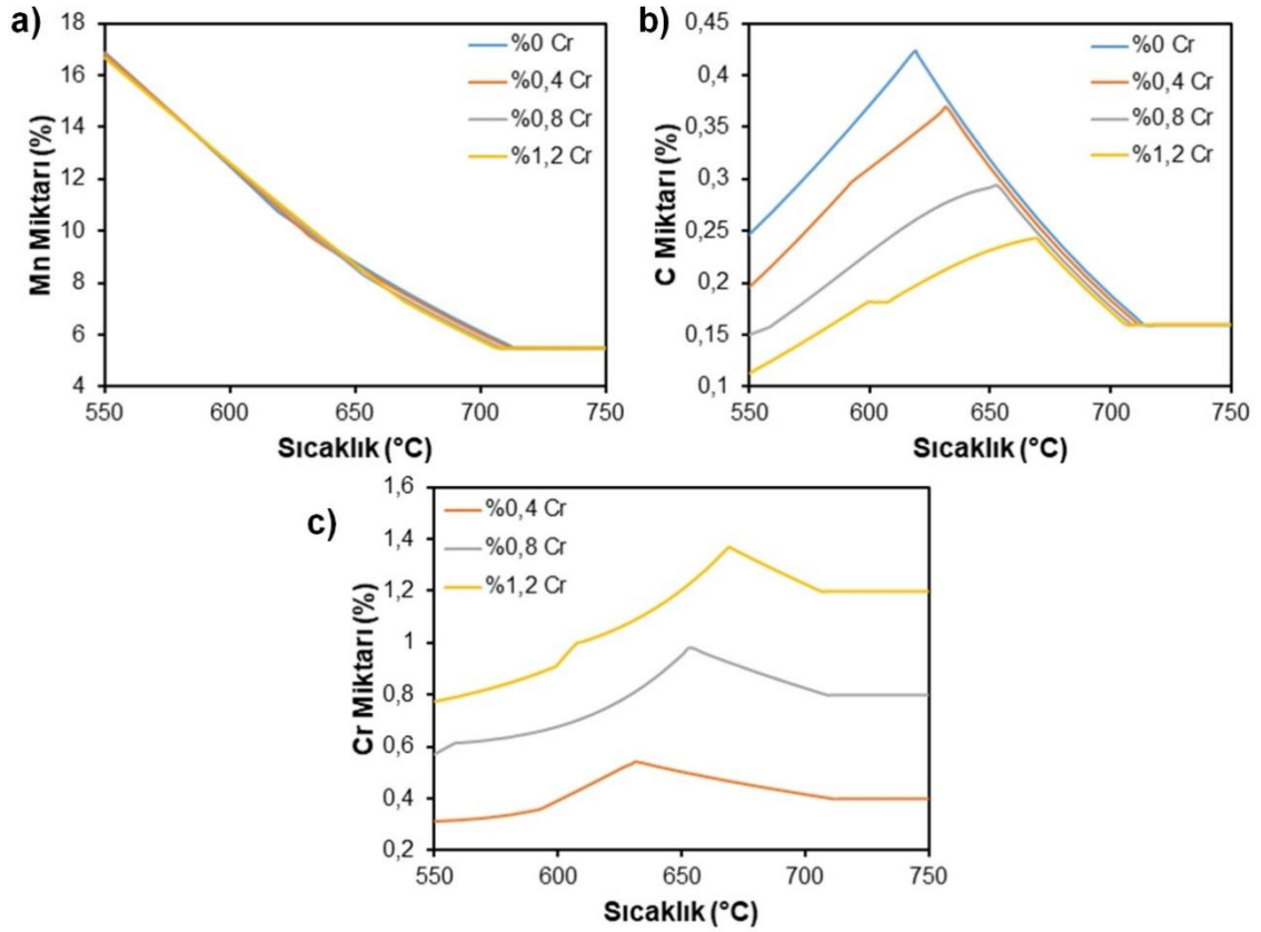
Şekil 5.16. Cr ilavesinin östenit fazı bileşimi üzerindeki etkisi
