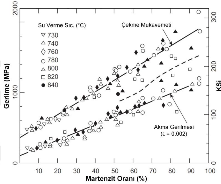
Şekil 2.5. Çift fazlı çeliklerde martenzit fazı hacim fraksiyonunun akma ve çekme mukavemeti üzerindeki etkisi [48]
