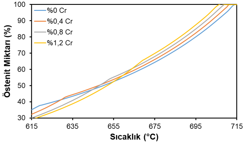
Şekil 5.13. Cr ilavesinin östenit fazı miktarı üzerindeki etkisi
