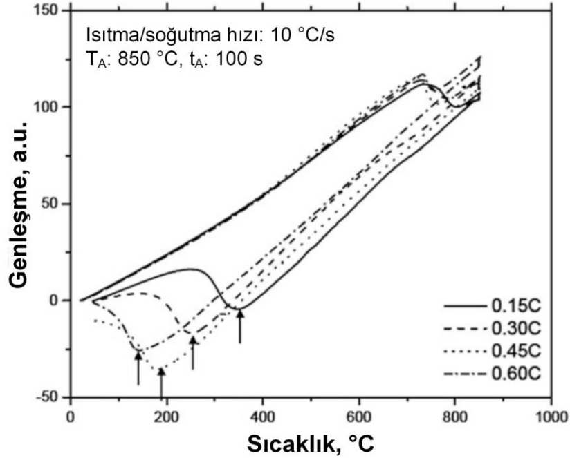
Şekil 3.16. (0.15-0.6)C-4Mn çeliği için tam östenizasyon sonrası soğutma sırasında (10 °C/s) martenzit dönüşümünü gösteren genleşme eğrileri [5]
