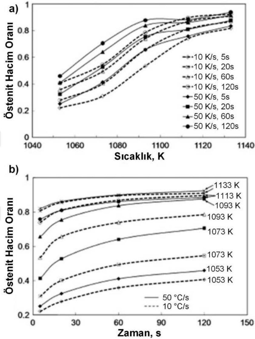
Şekil 2.26. Isıtma hızı ile kritik sıcaklığın, kritik tavlama sırasında zamana bağlı olarak oluşan östenit fazının fraksiyonu üzerindeki etkisi; a) Isıtma hızı, b) Kritik sıcaklık [121]
