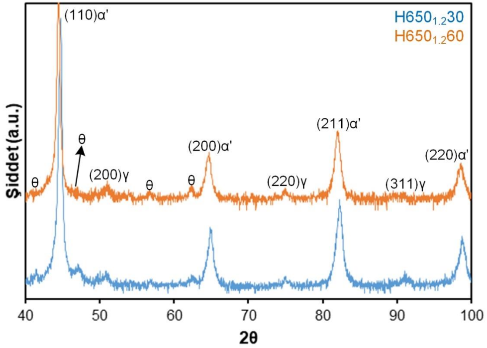
Şekil 5.102. H650 1.230 ve H650 1.260 numunelerine ait XRD analizi grafiği
