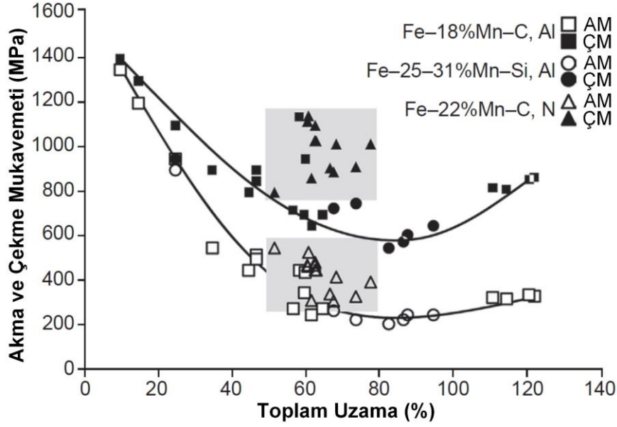
Şekil 2.11. TWIP çelikleri için mukavemet ve süneklik aralıkları (AM: Akma mukavemeti, ÇM: Çekme Mukavemeti) [64]
