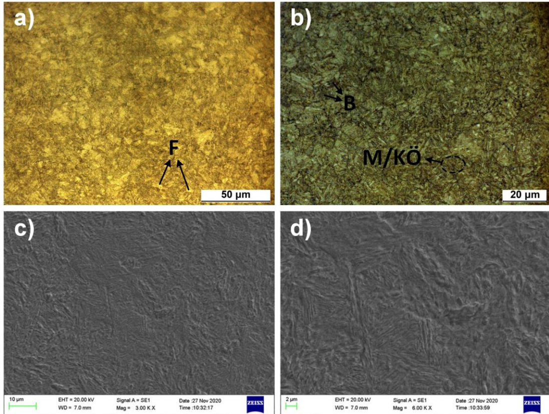
Şekil 5.43. H650 060 numunesine ait OM ve SEM görüntüleri
