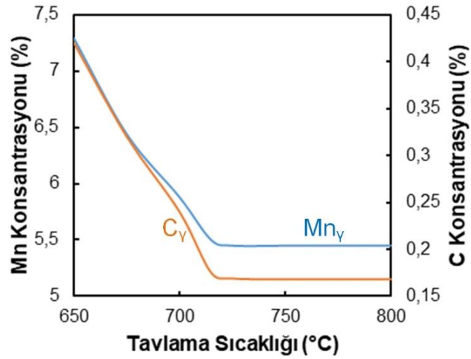
Şekil 5.82. Tavlama sıcaklığına bağlı olarak kalıntı östenitin Mn ve C içeriğinde meydana gelen değişim
