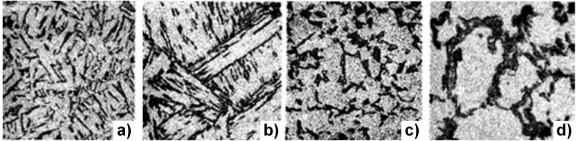
Şekil 2.25. Farklı birincil mikroyapıların büyüyen östenitin morfolojisi üzerindeki etkisini gösteren mikrograflar; a) 950 °C'den su verme sonrası birincil martenzit mikroyapısı, b) 1150 °C'den su verme sonrası birincil martenzit mikroyapısı, c) Birincil ferrit-perlit mikroyapısı, d) Küresel karbürlü ferrit mikroyapısı [94]
