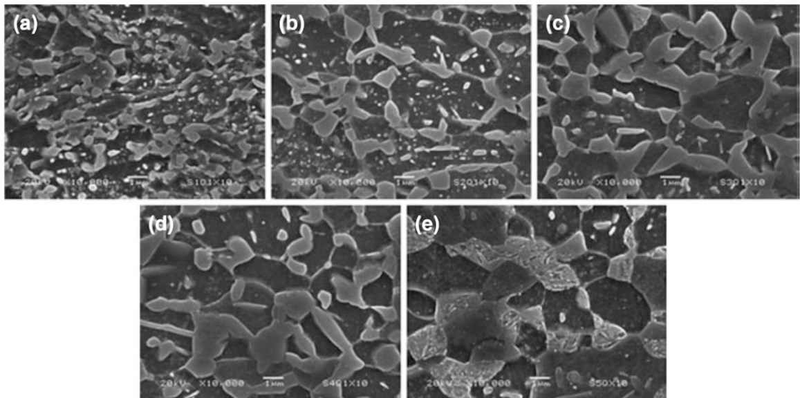
Şekil 3.17. 675°C’de farklı sürelerde tavlanan numunelerin SEM görüntüleri; a) 3 dakika, b) 1 saat, c) 3 saat, d) 6 saat, e) 26 saat [145]
