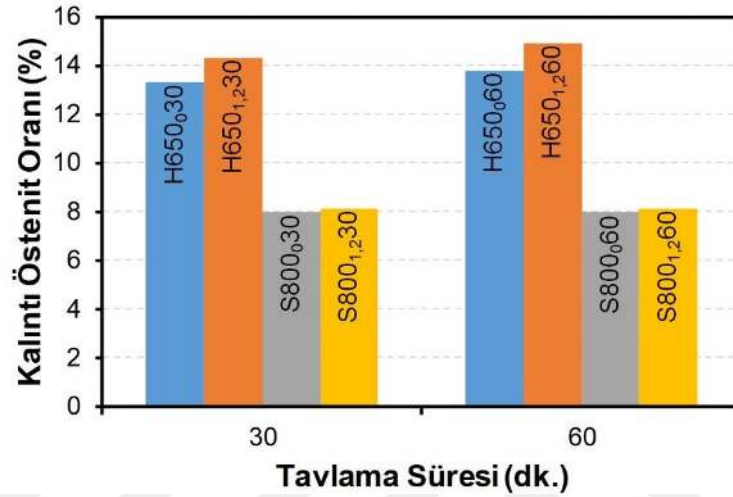
Şekil 5.105. Tavlama süresinin kalıntı östenit oranı üzerindeki etkisi
