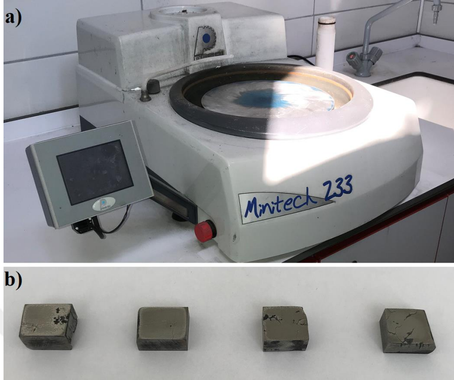
Şekil 4.12. Parlatma Cihazı (a) ve parlatma işleminden geçen numuneler (b)
