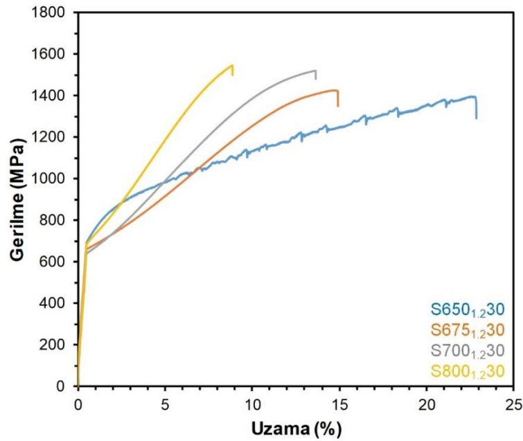
Şekil 5.134. S650 1,2 30, S675 1,2 30, S700 1,2 30 ve S800 1,2 30 numunelerinin gerilme-uzama grafikleri
