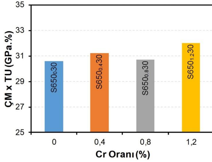
Şekil 5.153. S650 0,30 , S650 0,430 , S650 0,830 ve S650 1,230 numunelerine ait ÇM x TU değerleri
