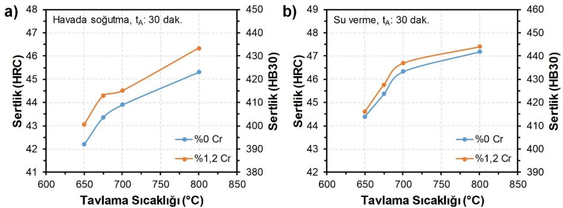
Şekil 5.126. Hava ve su ortamında soğutulan numunelerin sertlik grafiği; a) Havada soğutma, b) Su verme
