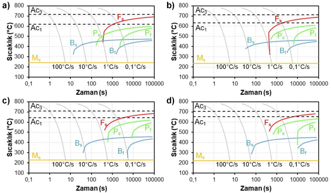
Şekil 5.7. Farklı oranlarda Cr içeren Fe-0.16C-5.5Mn çeliğine ait CCT diyagramları; a) %0 Cr, b) %0,4 Cr, c) %0,8 Cr, d) %1,2 Cr
