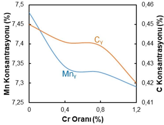
Şekil 5.108. Cr oranına bağlı olarak kalıntı östenitin Mn ve C içeriğinde meydana gelen değişim
