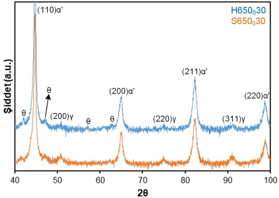
Şekil 5.92. S650 0 30 ve H650 0 30 numunelerine ait XRD analizi grafiği
