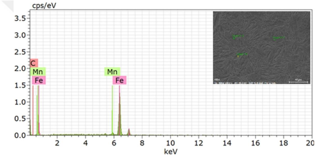
Şekil 5.88. S650 0 30 numunesine ait EDS analizi grafiği
