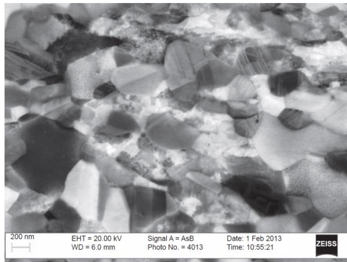
Şekil 2.12. 0.17C-6.5Mn orta manganlı çeliğine ait SEM görüntüsü [72]
