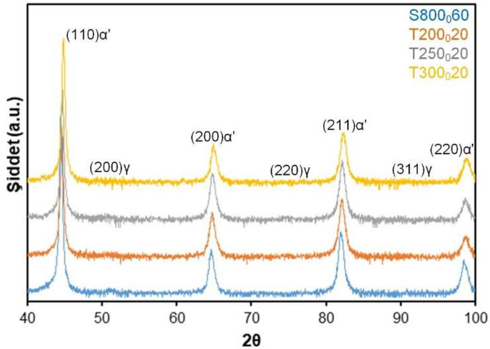
Şekil 5.121. S800 0 60, T200 0 20, T250 0 20 ve T300 0 20 numunelerine ait XRD analizi grafiği
