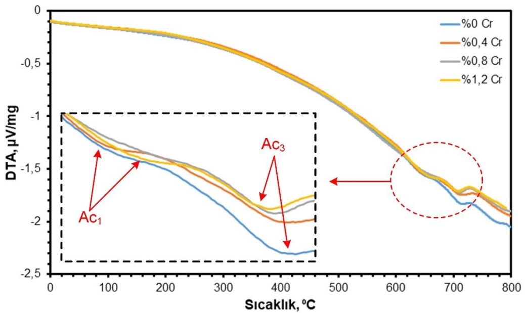
Şekil 5.3. DTA analiz sonuçları
