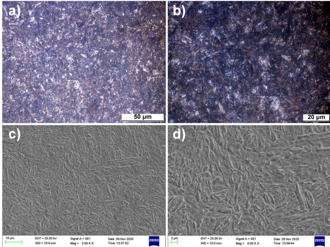
Şekil 5.66. T200 0 40 numunesine ait OM ve SEM görüntüleri
