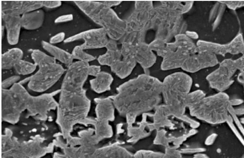
Şekil 2.24. Birincil östenit fazında mevcut olan çözünmeyen karbürler [94]
