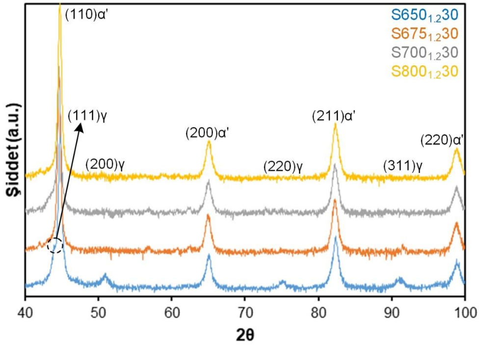
Şekil 5.85. S650 1.2 30, S675 1.2 30, S700 1.2 30 ve S800 1.2 30 numunelerine ait XRD analizi grafiği
