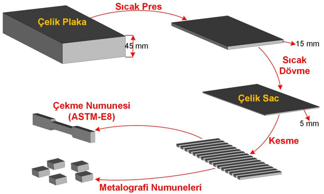
Şekil 4.7. Çelik sacların üretim aşamalarının ve numune hazırlama sürecinin şematik gösterimi
