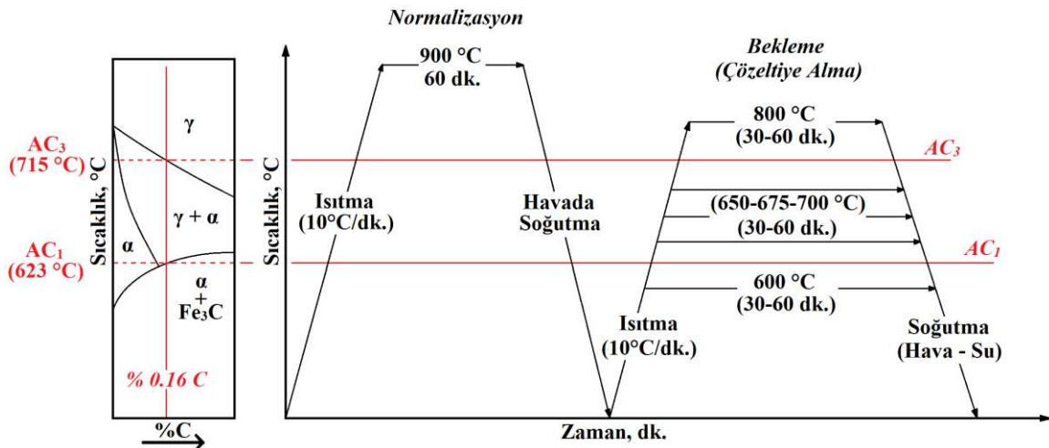
Şekil 4.8. Kritik tavlama işlemine ait termal döngülerin şematik gösterimi
