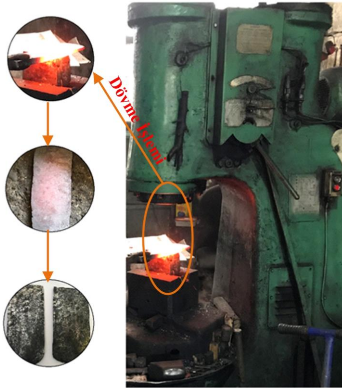
Şekil 4.3. Sıcak dövme işleminin uygulanması
