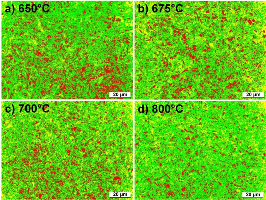
Şekil 5.28. H650 030 , H675 030 , H700 030 ve H800 030 numunelerine ait renklendirilmiş OM görüntüleri, Yeşil: Martenzit, Sarı: Beynit, Kırmızı: Ferrit
