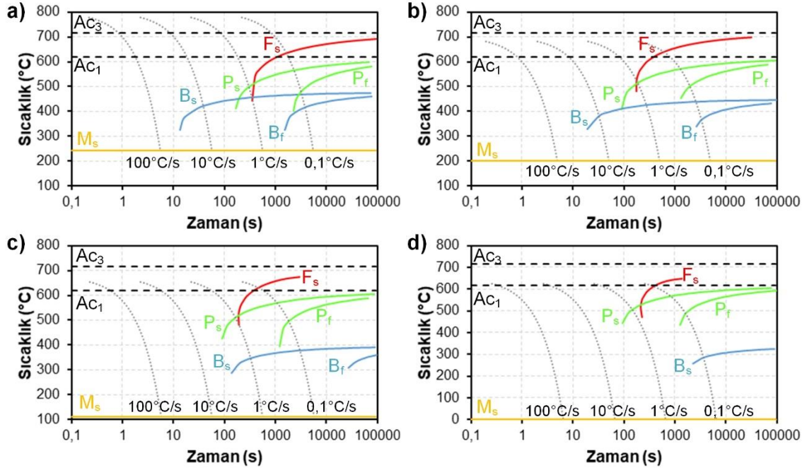
Şekil 5.5. Fe-0.16C-5.5Mn çeliğine ait CCT eğrileri; a) 800 °C, b) 700 °C, c) 675 °C, d) 650 °C
