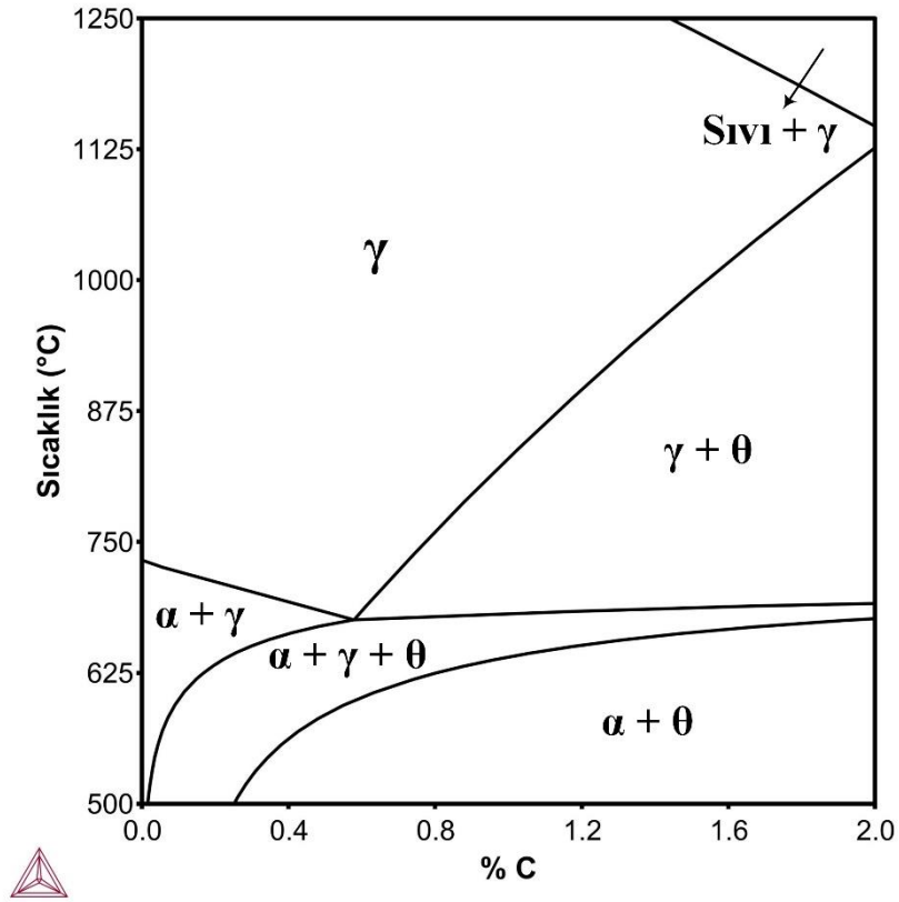
Şekil 5.1. Fe-Mn-C denge diyagramı
