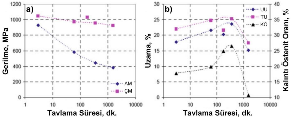
Şekil 3.18. Tavlama süresine bağlı olarak çekme özellikleri ve kalıntı östenitin hacim fraksiyonunda meydana gelen değişim [145]
