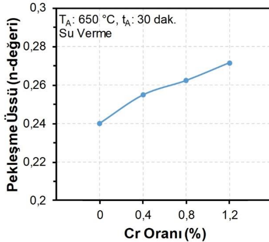
Şekil 5.152. Çelik bileşimindeki Cr oranına bağlı olarak pekleşme üssünde meydana gelen değişim
