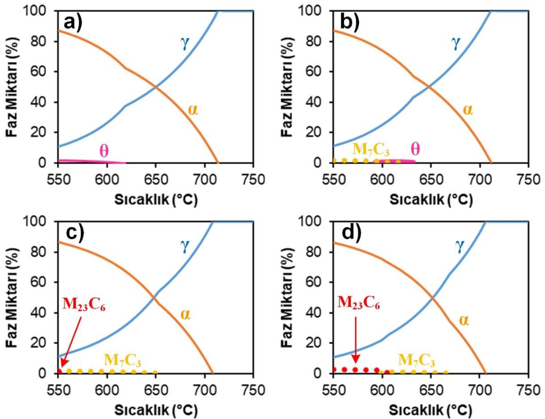
Şekil 5.11. Farklı oranlardaki Cr ilavesinin faz miktarları üzerindeki etkisi; a) %0 Cr, b) %0,4 Cr, c) %0,8 Cr, d) %1,2 Cr
