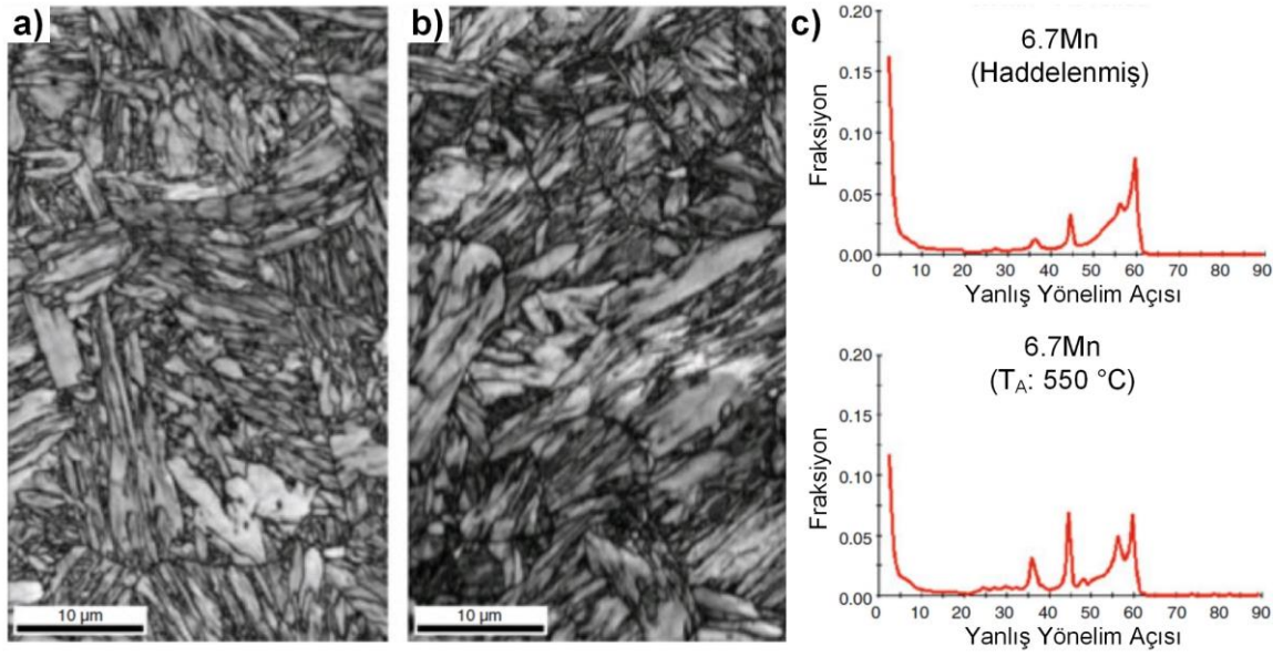
Şekil 3.9. %6.7 Mn’li çeliğin EBSD analizi; a) Haddelenmiş, b) 550 °C’de yığın halinde tavllanmış, c) Aynı numunelerde mikroyapı elemanlarının yanlış yönelim dağılımı [5]
