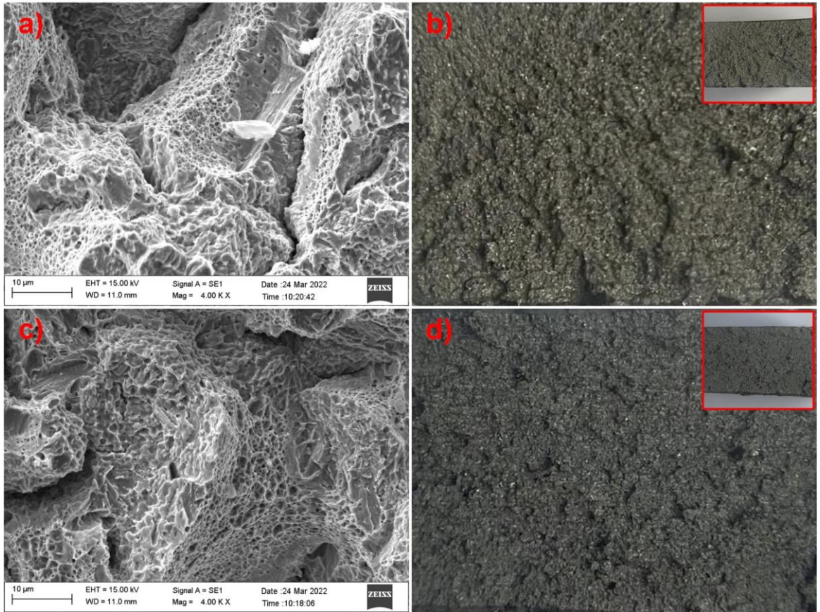
Şekil 5.154. Kopma yüzeylerinin SEM görüntüleri; a) S650 0,430 , c) S650 0,830 ile makro görüntüleri; b) S650 0,430 , d) S650 0,830
