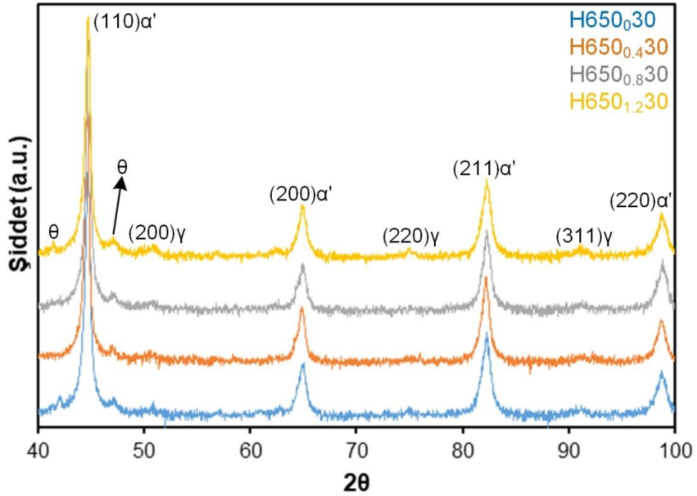
Şekil 5.110. H650 0.30 , H650 0.430 , H650 0.830 ve H650 1.230 numunelerine ait XRD analizi grafiği
