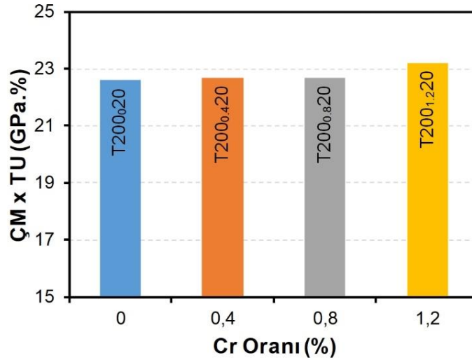
Şekil 5.165. T200 0 20, T200 0,4 20, T200 0,8 20 ve T200 1,2 20 numunelerine ait ÇM x TU değerleri
