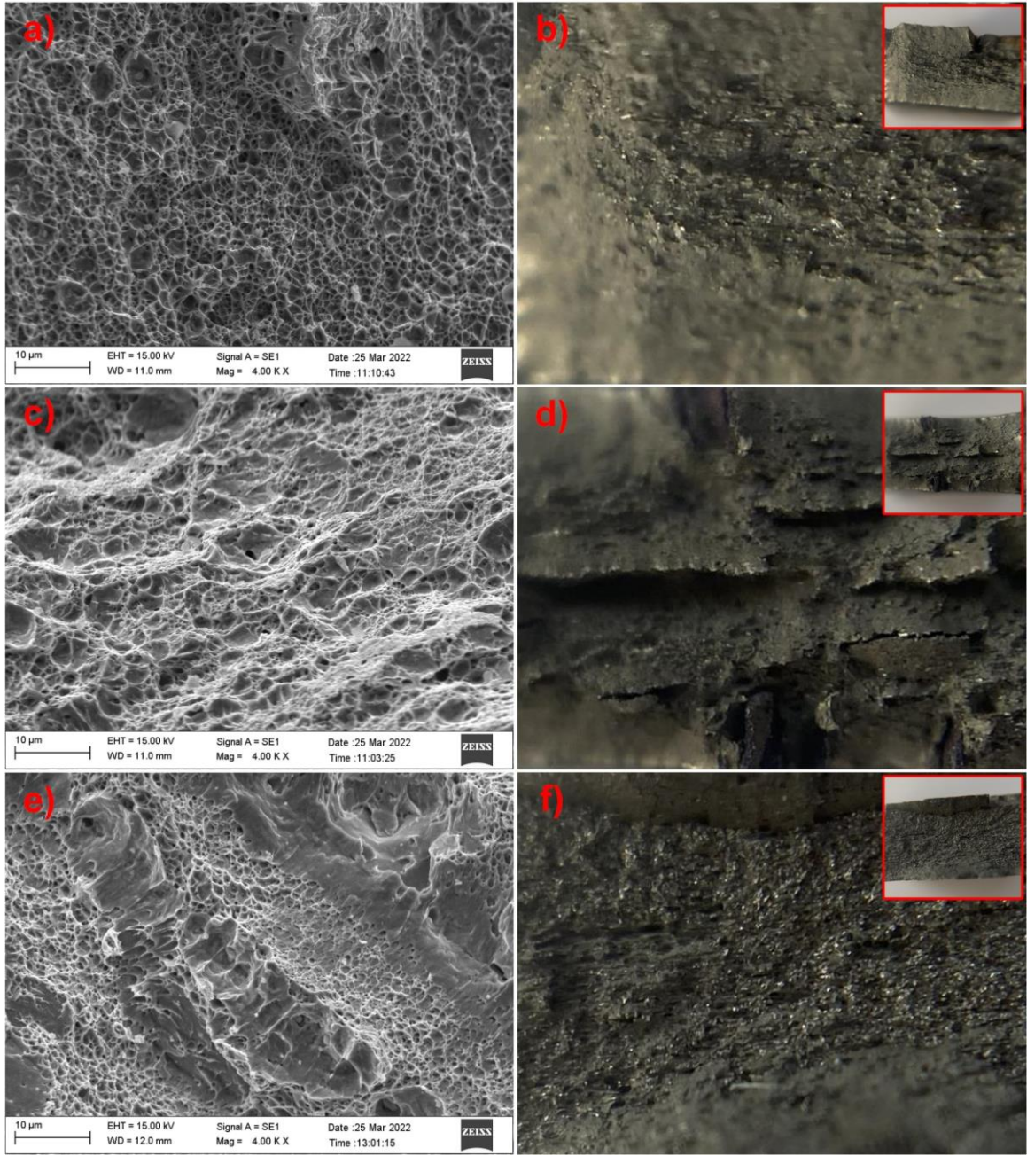
Şekil 5.156. Kopma yüzeylerinin SEM görüntüleri; a) T200 0 20, c) T250 0 20, e) T300 0 20 ile makro görüntüleri; b) T200 0 20, d) T250 0 20, f) T300 0 20
