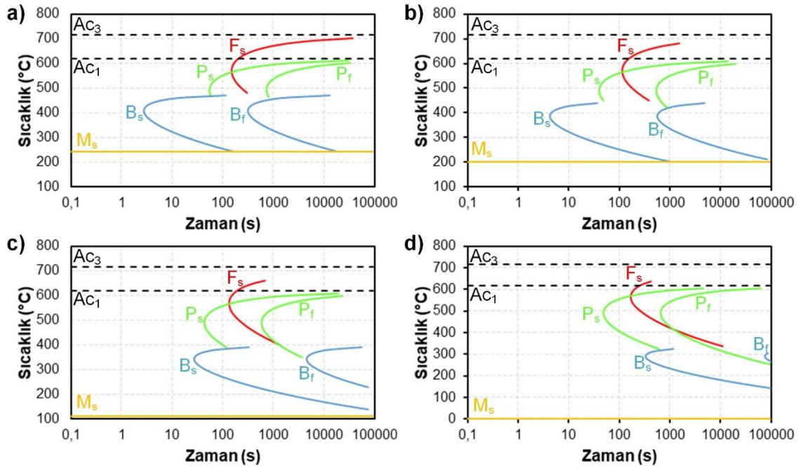
Şekil 5.6. Fe-0.16C-5.5Mn çeliğine ait TTT eğrileri; a) 800 °C, b) 700 °C, c) 675 °C, d) 650 °C
