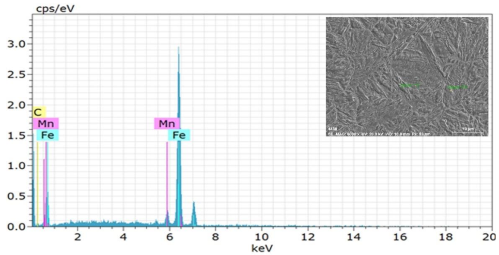
Şekil 5.114. T250 020 numunesine ait EDS analizi grafiği
