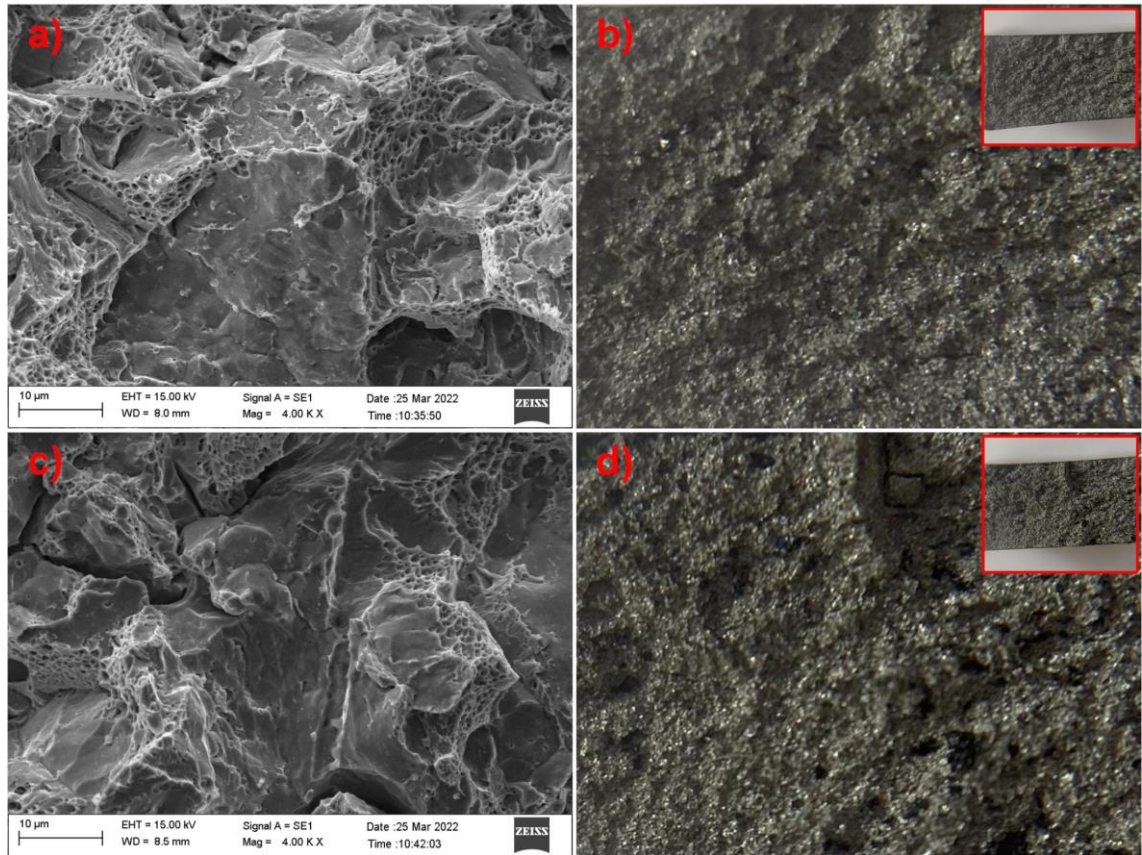
Şekil 5.148. Kopma yüzeylerinin SEM görüntüleri; a) S800 0 60, c) S800 1,2 60 ile makro görüntüleri; b) S800 0 60, d) S800 1,2 60
