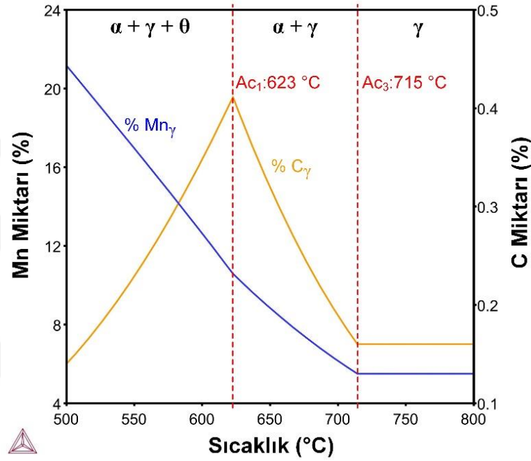
Şekil 5.15. Östenit fazındaki C ve Mn konsantrasyonlarının değişimi
