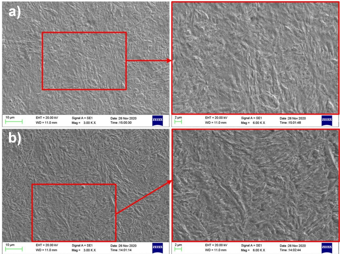
Şekil 5.73. T250 1.220 ve T300 1.220 numunelerinin SEM görüntüleri; a) T250 1.220 , b) T300 1.220
