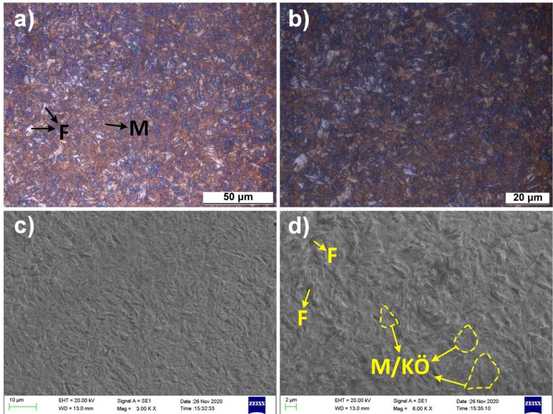
Şekil 5.62. Temperlenmemiş S800 60 numunesine ait OM ve SEM görüntüleri
