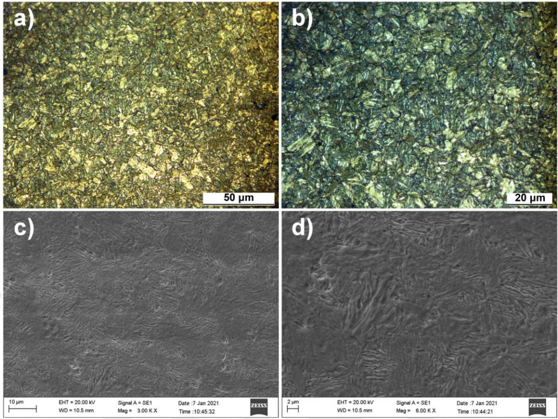
Şekil 5.60. %0.8 Cr ilaveli S650 0.8 30 numunesine ait OM ve SEM görüntüleri
