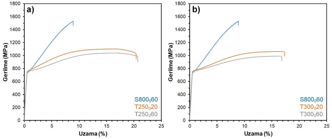
Şekil 5.161. Farklı sürelerde temperlenen T250 20 ve T250 60 numuneleri ile T300 20 ve T300 60 numunelerinin gerilme-uzama grafikleri; a) 250 °C, b) 300 °C
