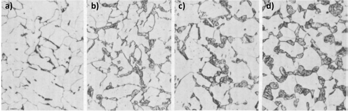
Şekil 2.21. Tavlama süresinin bir fonksiyonu olarak östenit fazı büyümesi; a) 0 dakika, b) 2 dakika, c) 1 saat, d) 24 saat [110]
