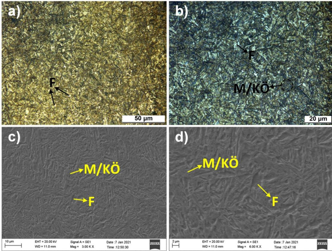
Şekil 5.21. N_{0.4} numunesine ait OM ve SEM görüntüleri
