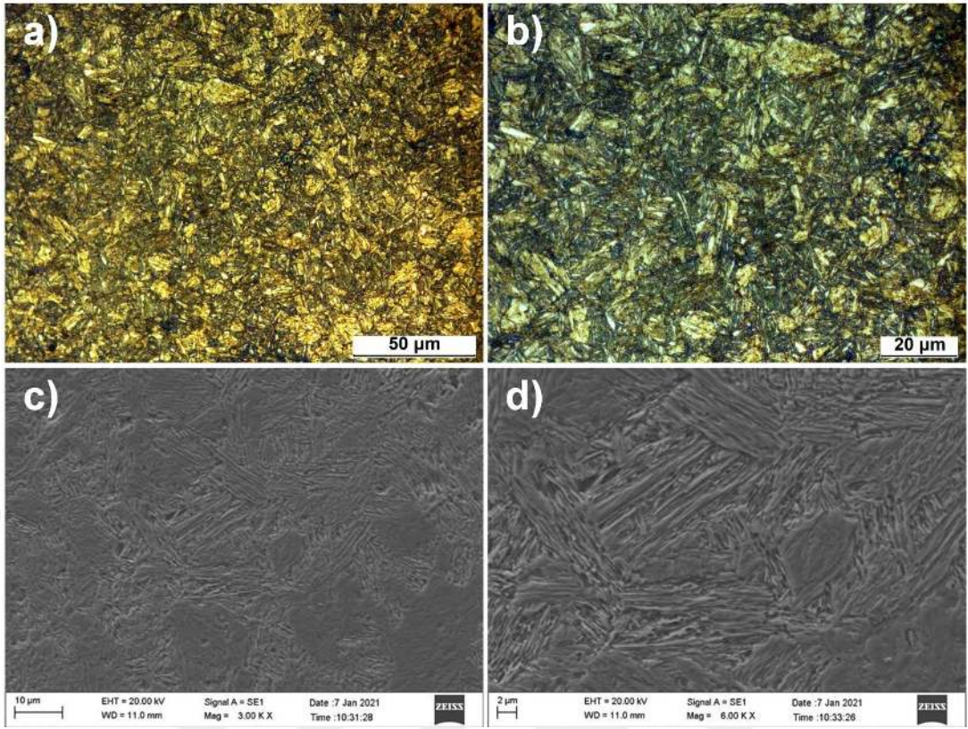
Şekil 5.37. S650 1,230 numunesine ait OM ve SEM görüntüleri
