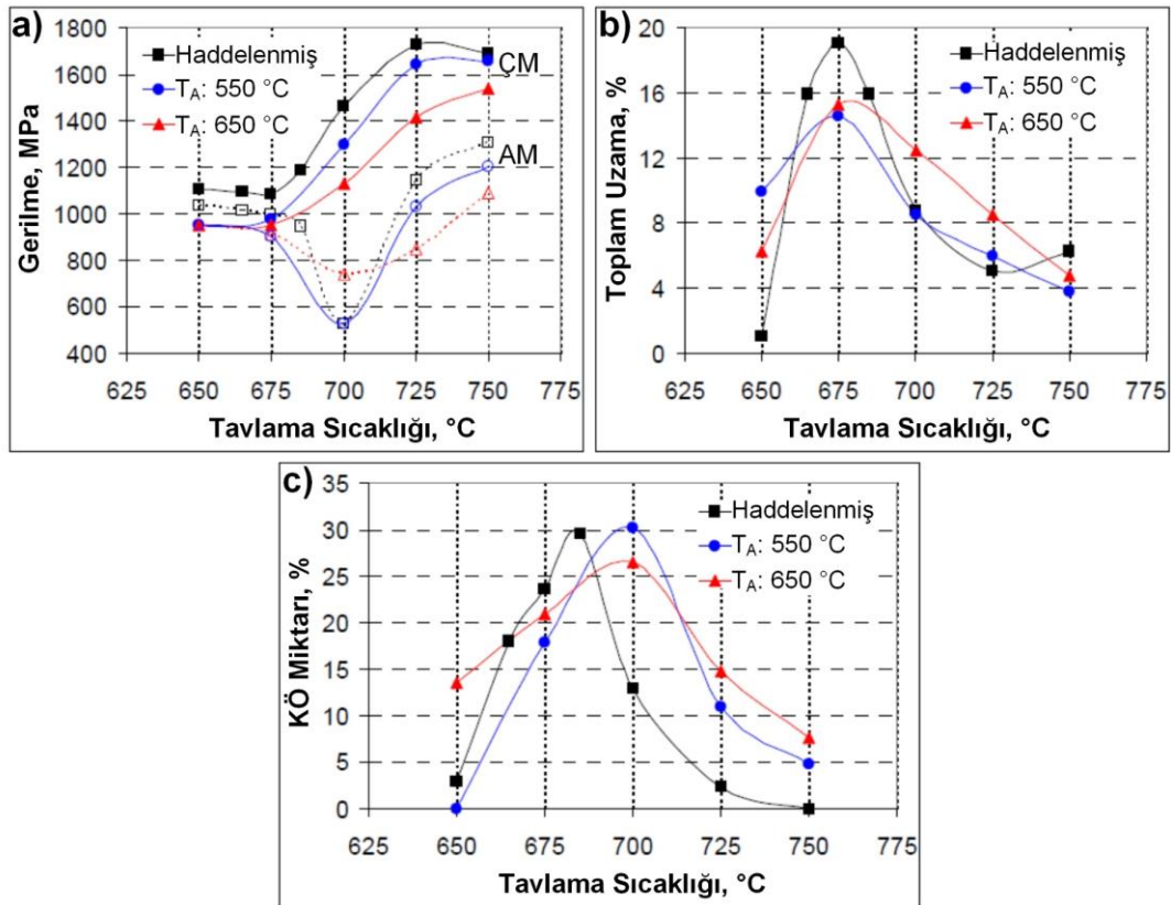
Şekil 3.10. %4 Mn’li bir çelikte birincil mikroyapının ve tavlama sıcaklığının çekme özellikleri ile kalıntı östenit miktarına etkisi [156]
