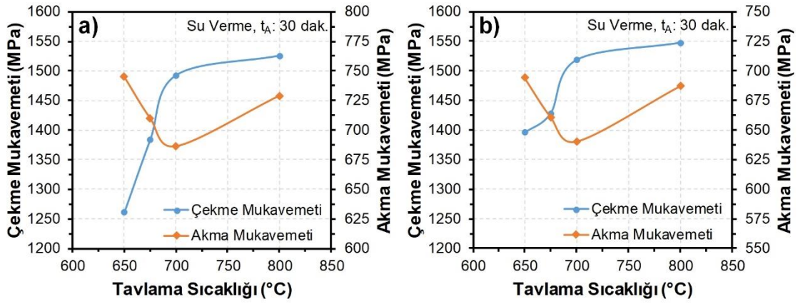
Şekil 5.137. Tavlama sıcaklığına bağlı olarak Cr ilavesiz ve %1.2 Cr ilaveli numunelerin akma ve çekme mukavemetlerinde meydana gelen değişimler; a) %0 Cr, b) %1.2 Cr
