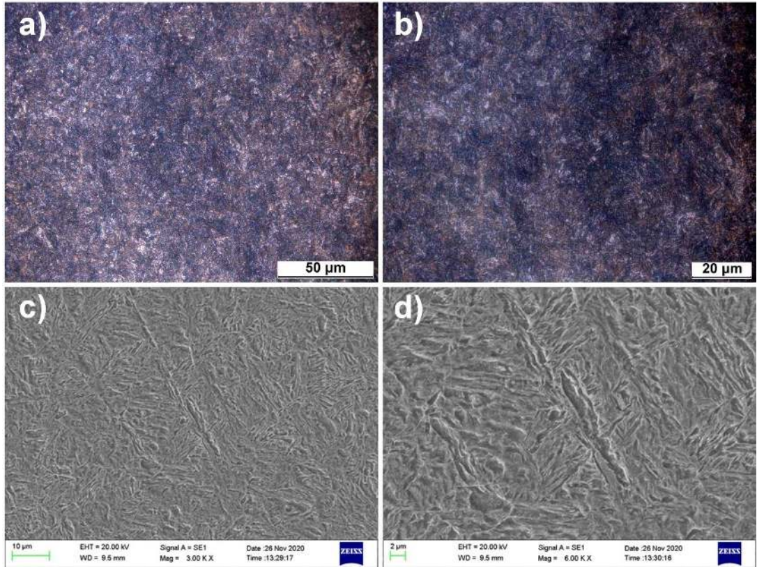
Şekil 5.72. %1.2 Cr ilaveli T200 1.2 20 numunesine ait OM ve SEM görüntüleri
