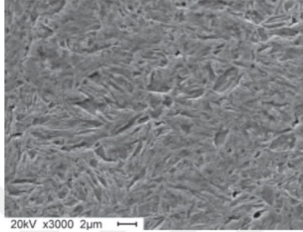
Şekil 2.6. Martenzitik bir mikroyapının (M1200) SEM görüntüsü [52]
