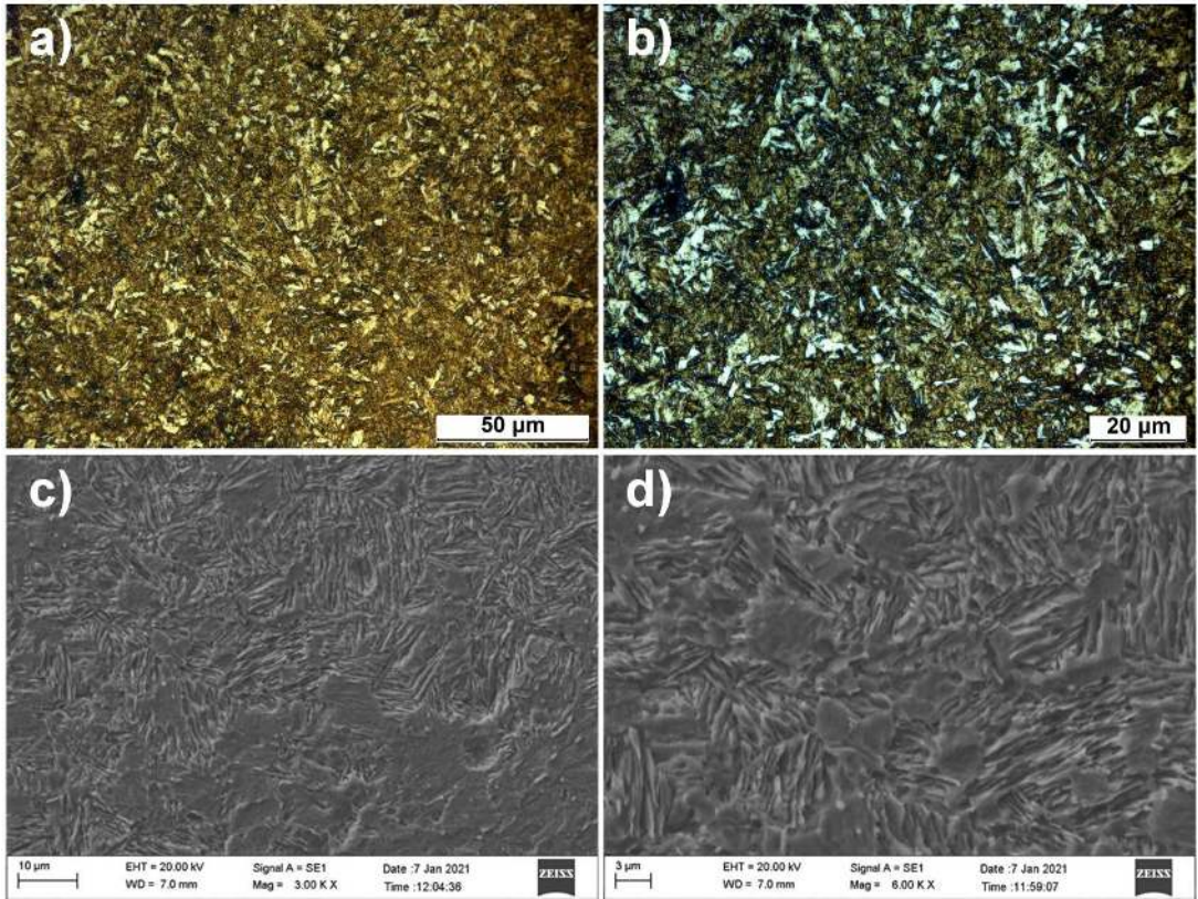
Şekil 5.38. S675 1,230 numunesine ait OM ve SEM görüntüleri
