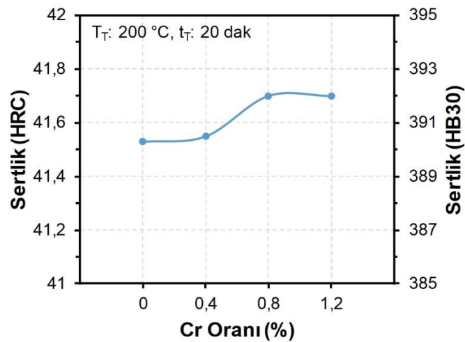
Şekil 5.131. Farklı oranlarda Cr içeren temperlenmiş numunelere ait sertlik grafiği
