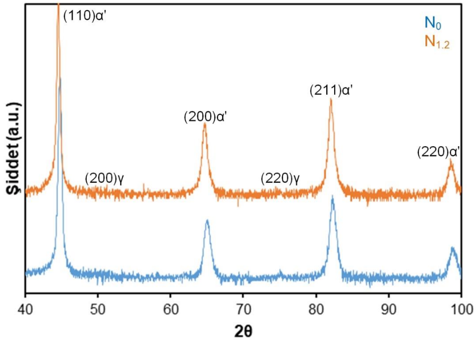
Şekil 5.77. N 0 ve N 1.2 numunelerine ait XRD analizi grafiği
