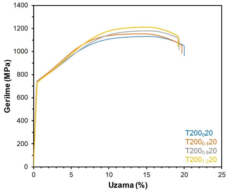
Şekil 5.163. T200 0 20, T200 0,4 20, T200 0,8 20 ve T200 1,2 20 numunelerinin gerilme-uzama grafikleri
