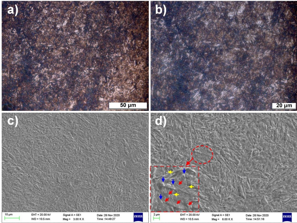
Şekil 5.65. T300 20 numunesine ait OM ve SEM görüntüleri
