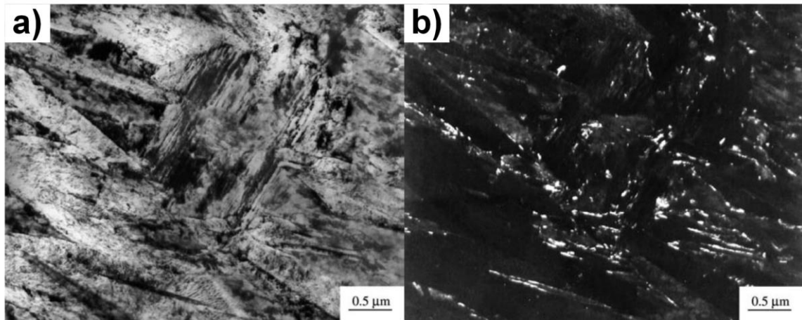
Şekil 2.13. Q&P çeliğine ait TEM görüntüleri; a) Aydınlik alan ( \alpha' ), b) Karanlık alan ( \gamma ) [78]
