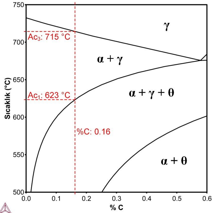
Şekil 5.2. Fe-0.16C-5.5Mn çeliği için A_{c1} ve A_{c3} sıcaklıkları
