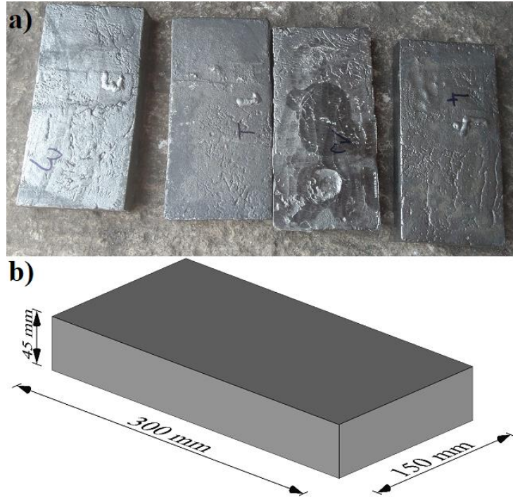
Şekil 4.2. Döküm sonrası çelik plakalar (a) ve plaka ölçüleri (b)
