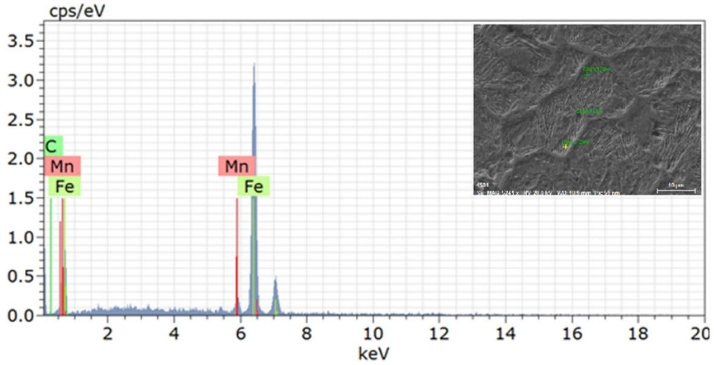
Şekil 5.90. H650 1,2 30 numunesine ait EDS analizi grafiği
