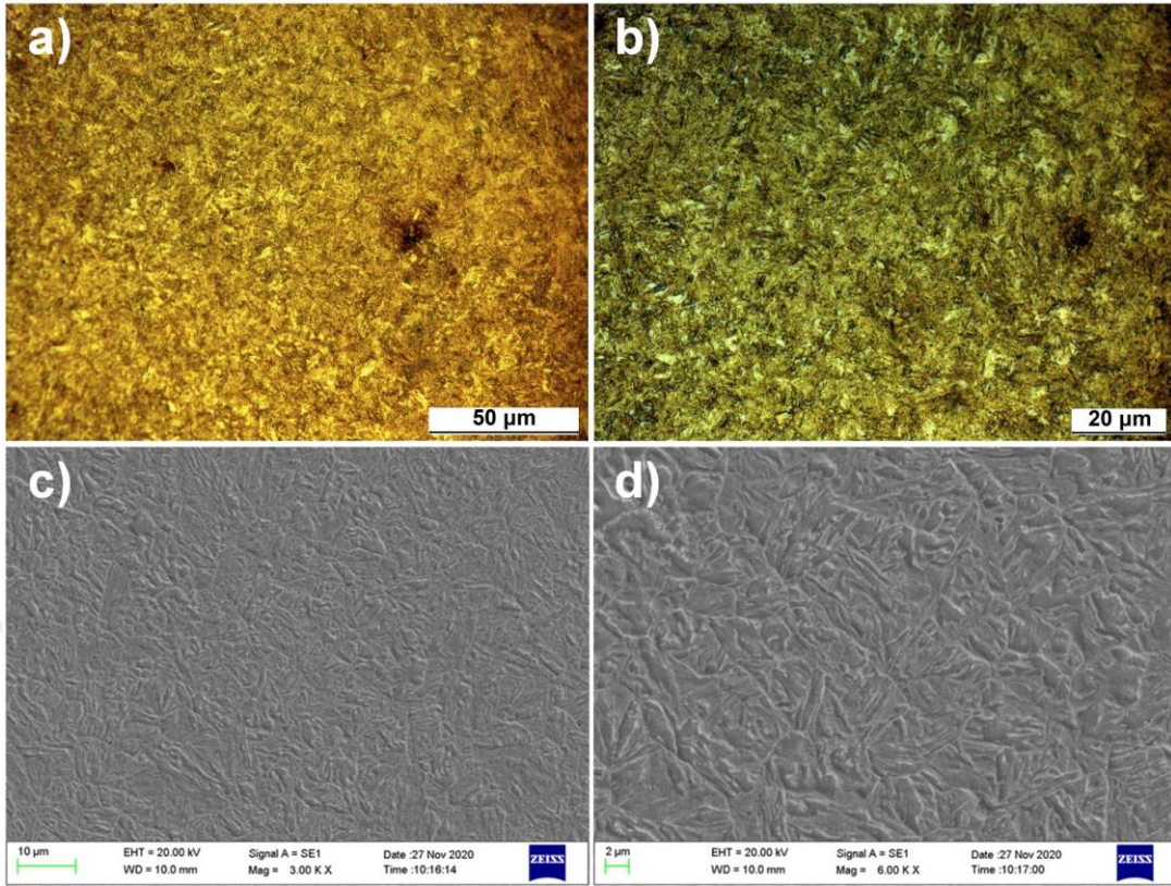
Şekil 5.31. H700 1,230 numunesine ait OM ve SEM görüntüleri
