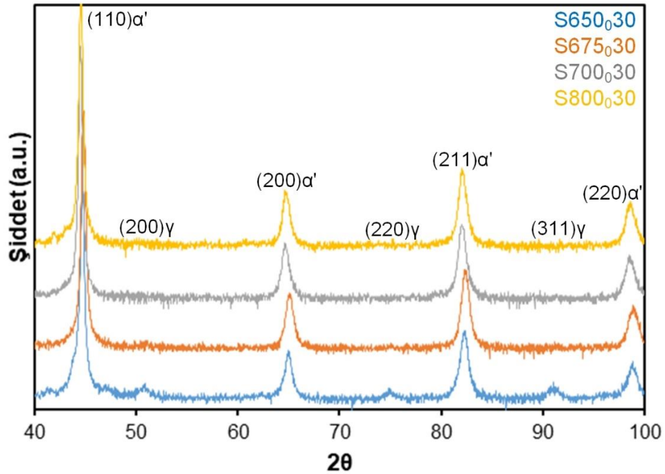
Şekil 5.84. S650 0 30, S675 0 30, S700 0 30 ve S800 0 30 numunelerine ait XRD analizi grafiği
