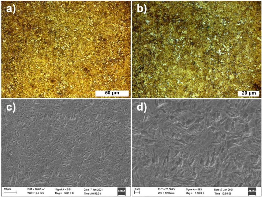
Şekil 5.39. S700 1,230 numunesine ait OM ve SEM görüntüleri
