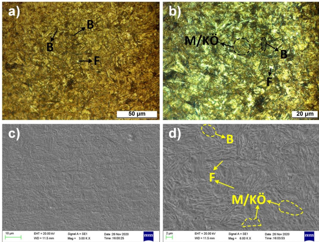
Şekil 5.24. H650 30 numunesine ait OM ve SEM görüntüleri
