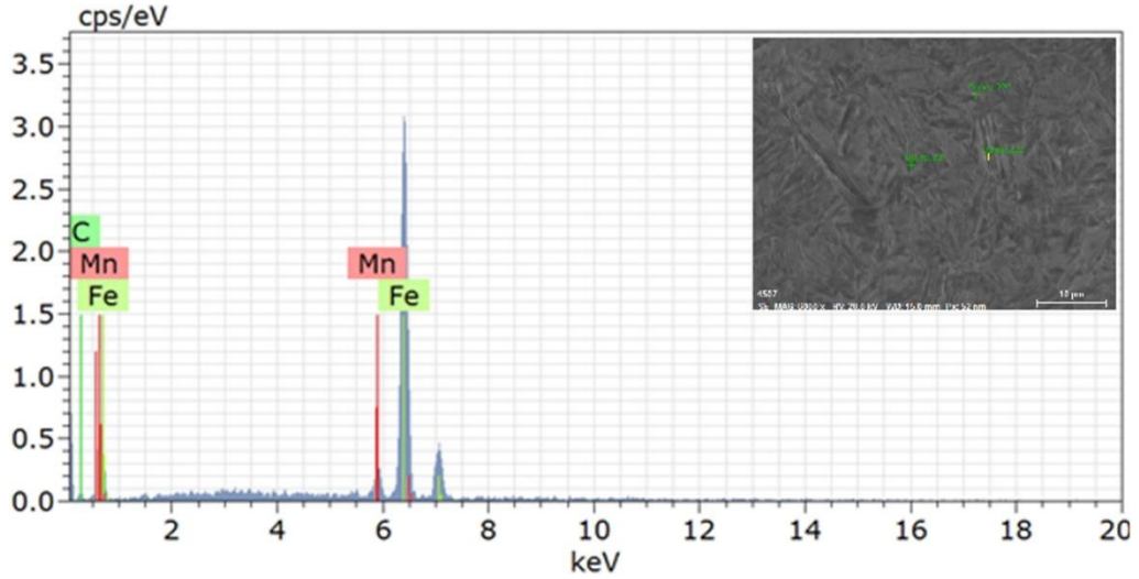
Şekil 5.99. S800 1,2 60 numunesine ait EDS analizi grafiği
