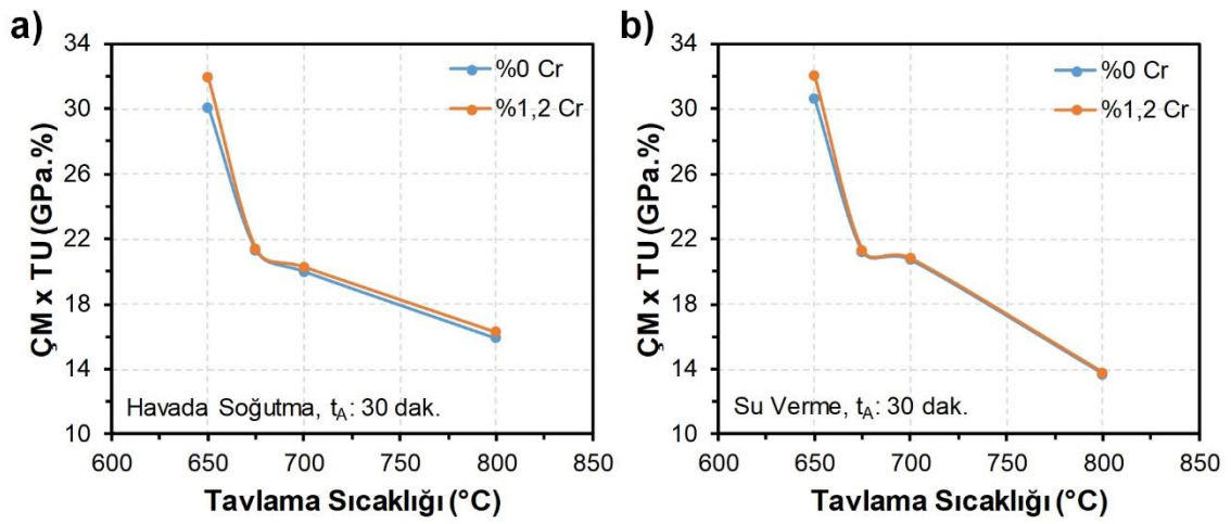
Şekil 5.167. Kritik tavlama parametrelerinin 0.16C-5.5Mn çeliğinin \text{ÇM} - \text{TU} kombinasyonu üzerindeki etkisi; a) Havada soğutma, b) Su verme
