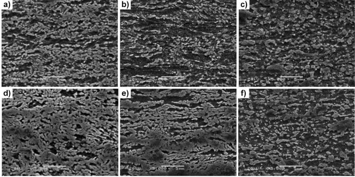
Şekil 3.11. Farklı başlangıç mikroyapılarına sahip %4 Mn’li çeliğe ait SEM görüntüleri; a) sıcak haddeleme + 675 °C, b) 550 °C + 675 °C, c) 650 °C + 675 °C, d) sıcak haddeleme + 700 °C, e) 550 °C + 700 °C, f) 650 °C + 700 °C [156]
