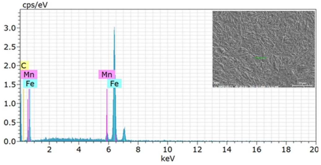
Şekil 5.115. T300 0 20 numunesine ait EDS analizi grafiği
