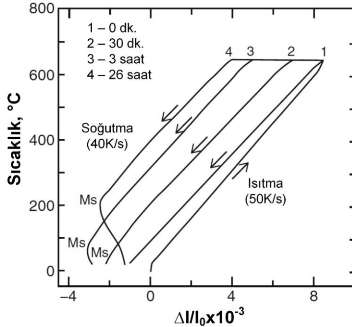
Şekil 3.15. 0.12C-5.1Mn çeliğinin farklı bekleme süreleri için 650 °C'ye ısıtılması ve soğutulması sonrasındaki genleşme eğrileri [160]
