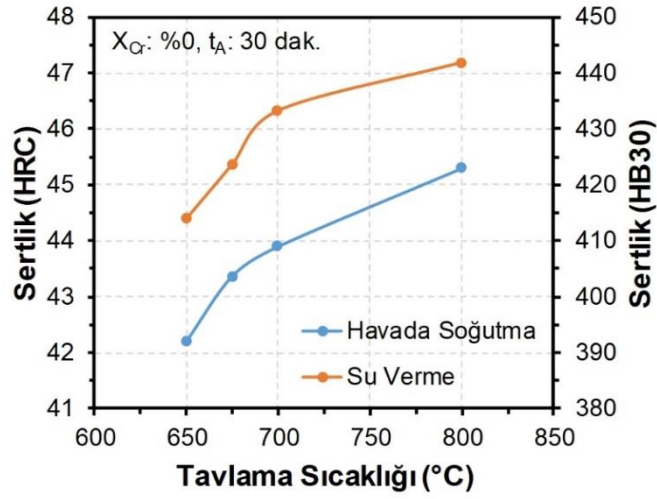
Şekil 5.125. Farklı sıcaklıklarda tavlanan numunelerin sertlik grafiği
