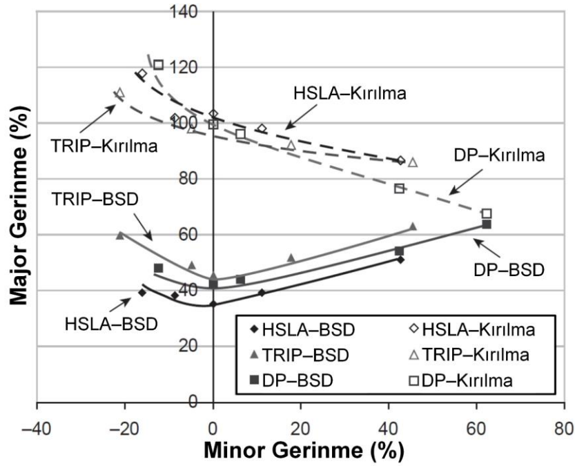
Şekil 2.16. Çift fazlı (DP), dönüşüm kaynaklı plastisite gösteren (TRIP) ve yüksek mukavemetli, düşük alaşımlı (HSLA) çelikler için biçimlendirme sınır diyagramı (BSD) [88]
