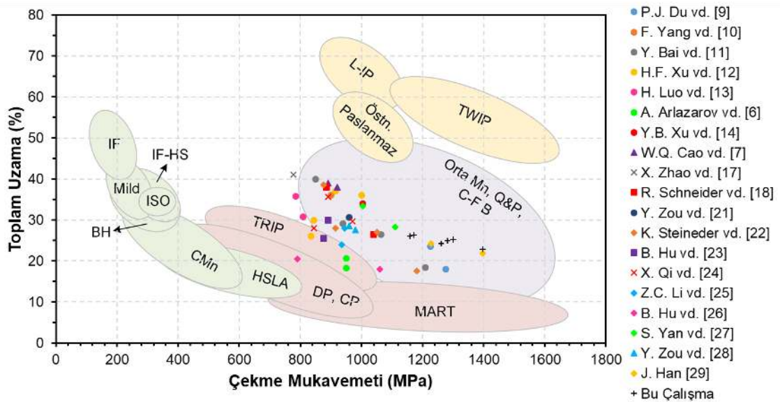
Şekil 5.170. Farklı yazarlar tarafından rapor edilen orta manganlı çelik saclarına ait çekme mukavemeti ve toplam uzama değerleri
