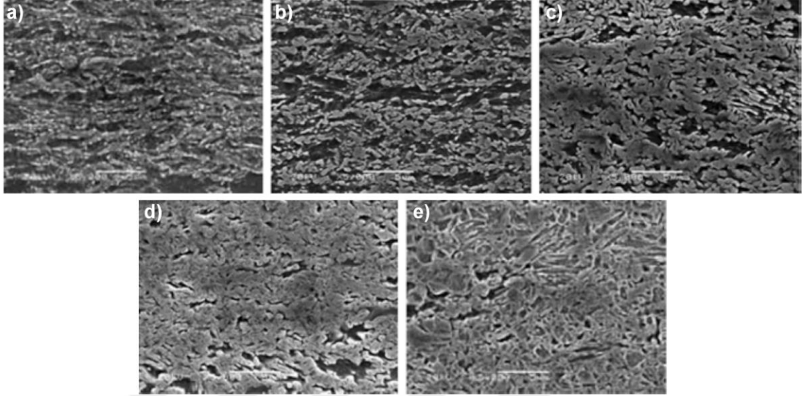
Şekil 3.2. Farklı sıcaklıklarda tavlanan 0.15-4Mn çeliğine ait numunelerin mikroyapısını gösteren SEM mikrografları; Tavlama sıcaklığı, (a) 650, (b) 675, (c) 700, (d) 725 ve (e) 750 °C [5]
