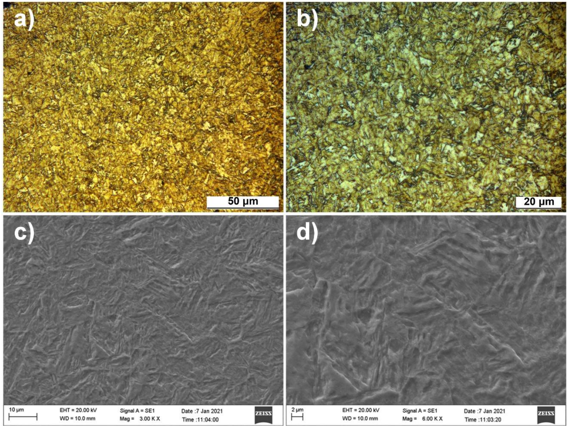
Şekil 5.36. S800 0 30 numunesine ait OM ve SEM görüntüleri
