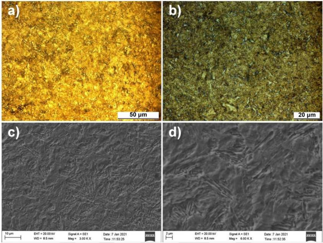
Şekil 5.34. S675 0 30 numunesine ait OM ve SEM görüntüleri
