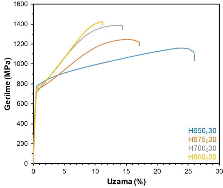
Şekil 5.139. H650 0 30, H675 0 30, H700 0 30 ve H800 0 30 numunelerinin gerilme-uzama grafikleri
