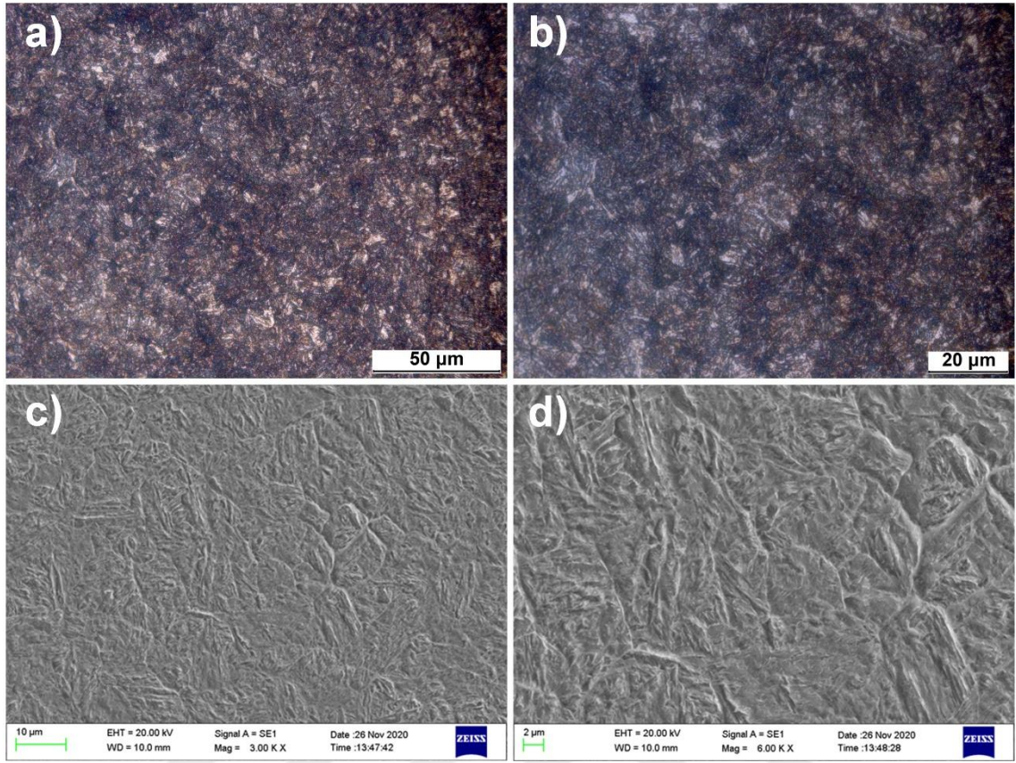
Şekil 5.67. T200 60 numunesine ait OM ve SEM görüntüleri
