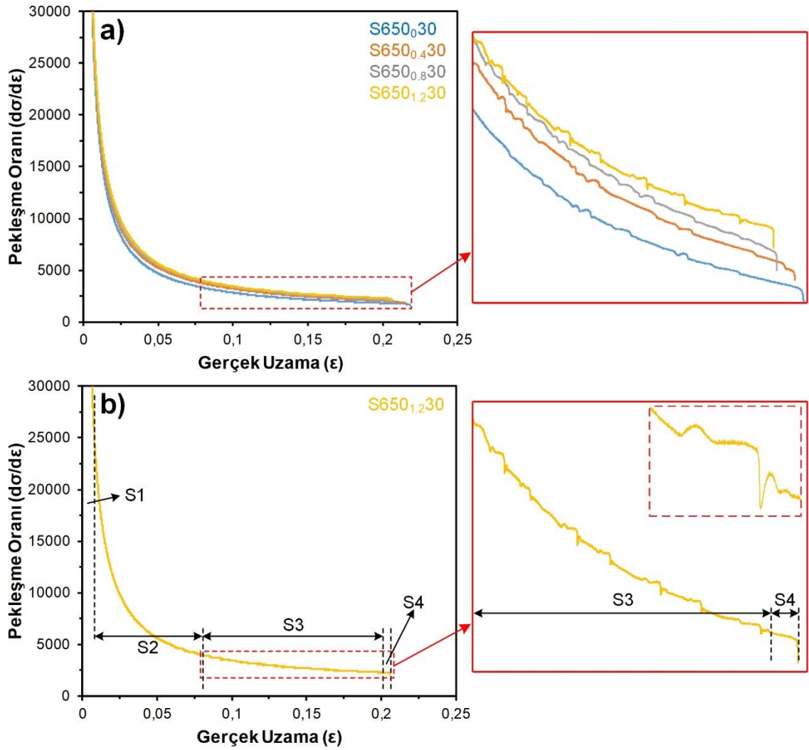
Şekil 5.150. S650 0 .30, S650 0.4 .30, S650 0.8 .30 ve S650 1.2 .30 numunelerinin pekleşme oranı grafikleri (a) ve pekleşme evreleri (b)
