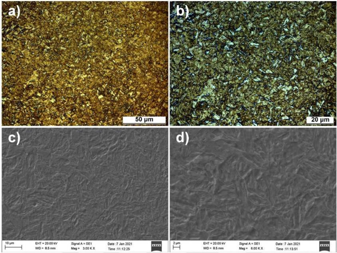
Şekil 5.50. S800 1,230 ( t_A : 30 dk.) numunesine ait OM ve SEM görüntüleri
