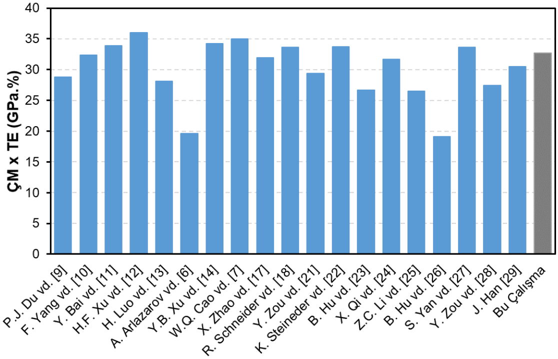
Şekil 5.171. Farklı yazarlar tarafından rapor edilen orta manganlı çelik saclara ait çekme mukavemeti – toplam uzama kombinasyonları
