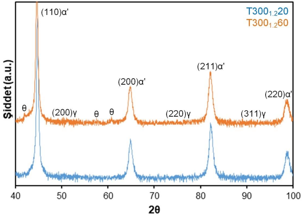
Şekil 5.123. T300 1,2 20 ve T300 1,2 60 numunelerine ait XRD analizi grafiği
