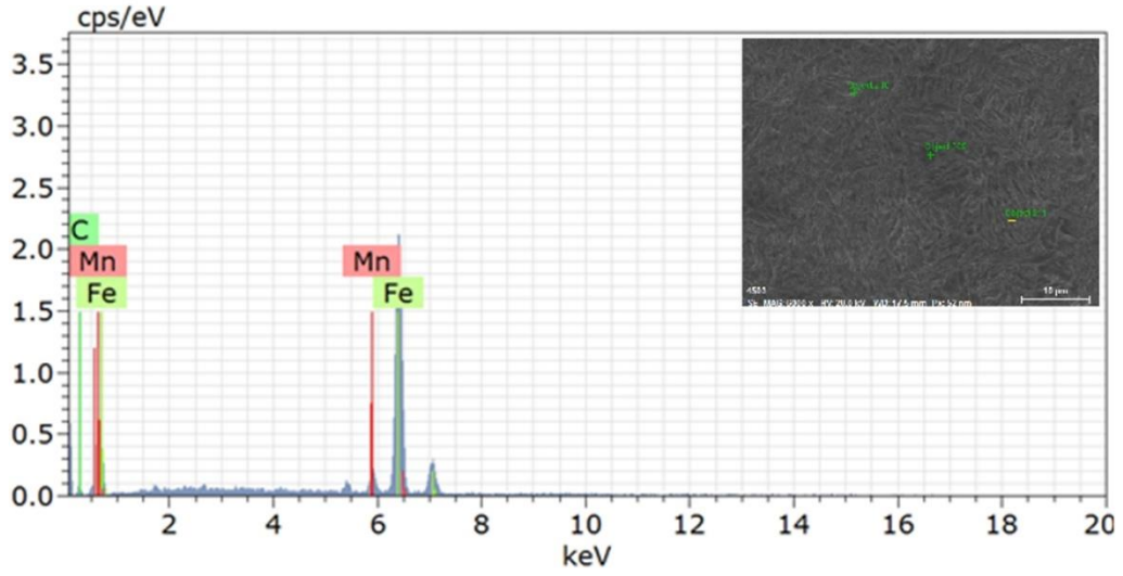
Şekil 5.106. S650 0,430 numunesine ait EDS analizi grafiği
