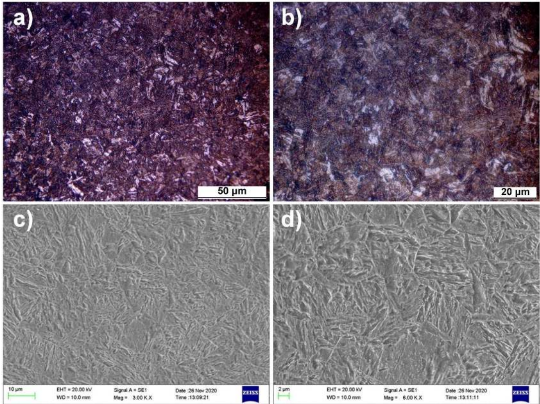
Şekil 5.70. %0.4 Cr ilaveli T200 0 .420 numunesine ait OM ve SEM görüntüleri
