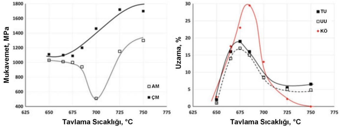
Şekil 3.1. Tavlama sıcaklığının gerilme-uzama davranışı ve kalıntı östenitin hacim fraksiyonu üzerindeki etkisi; a) akma/çekme mukavemeti, b) üniform/toplam uzama ve kalıntı östenit hacmi [145]
