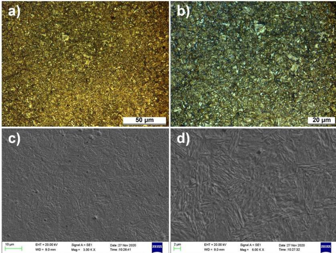
Şekil 5.32. H800 1,230 numunesine ait OM ve SEM görüntüleri
