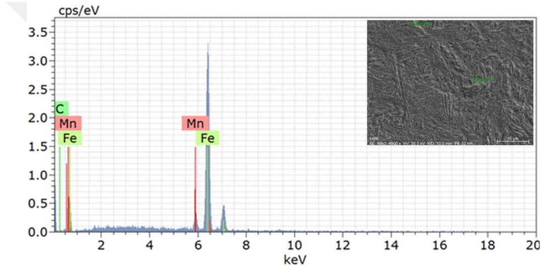
Şekil 5.96. H650 0 60 numunesine ait EDS analizi grafiği
