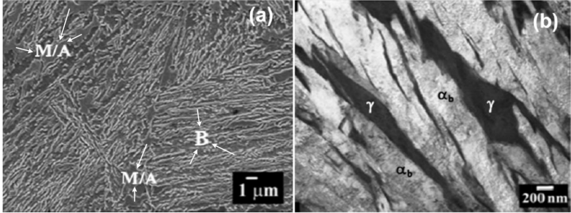
Şekil 2.15. Karbür içermeyen beynitik çeliğe ait (a) SEM ve (b) TEM görüntüsü (M/A: martenzit/kalıntı östenit, B: Beynit; \alpha_b : beynitik ferrit ve \gamma : Kalıntı östenit) [86]
