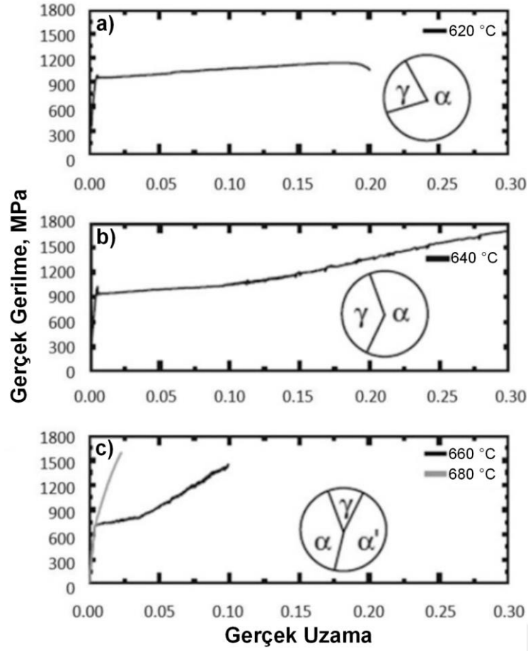
Şekil 3.6. Farklı sıcaklıklarda tavllanmış 0.3C-6Mn çeliği numunelerinin gerçek gerilme-gerçek uzama eğrileri; a) 620 °C, b) 640 °C, c) 660 ve 680 °C (Pasta grafiği, kritik tavlamadan sonra numunelerdeki faz içeriğini göstermektedir) [5]
