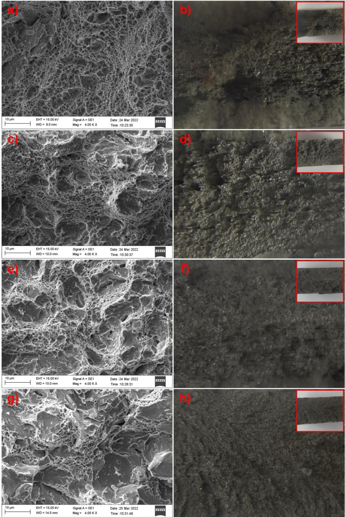
Şekil 5.141. Kopma yüzeylerinin SEM görüntüleri; a) H650 30 , c) H675 30 , e) H700 30 , g) H800 30 ile makro görüntüleri; b) H650 30 , d) H675 30 , f) H700 30 , h) H800 30
