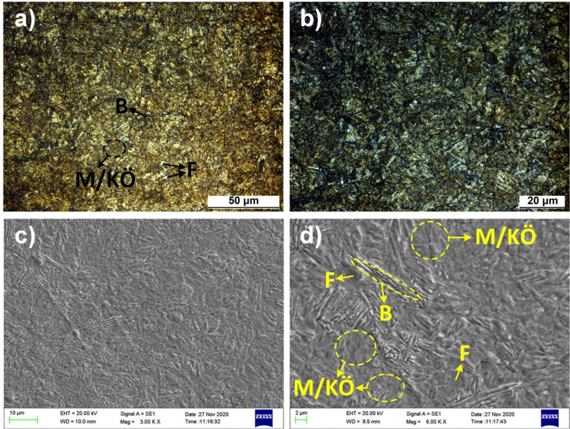
Şekil 5.46. H650 1.2 60 numunesine ait OM ve SEM görüntüleri
