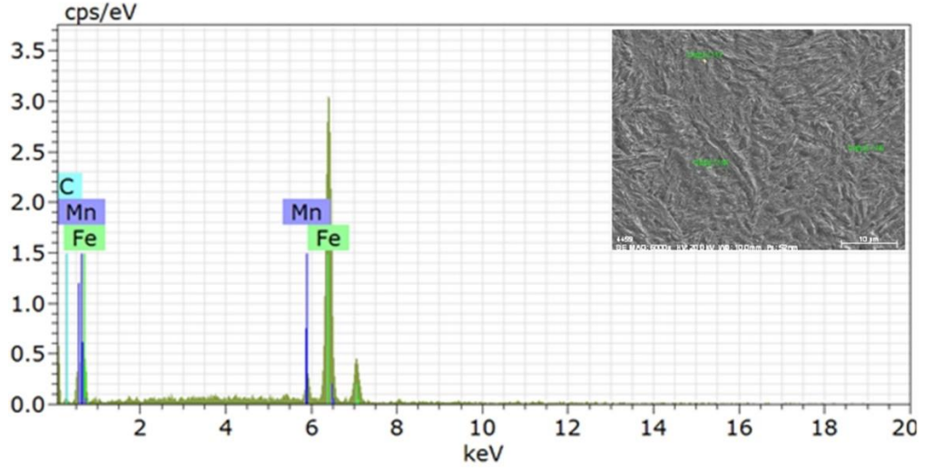
Şekil 5.118. T300 1,220 numunesine ait EDS analizi grafiği
