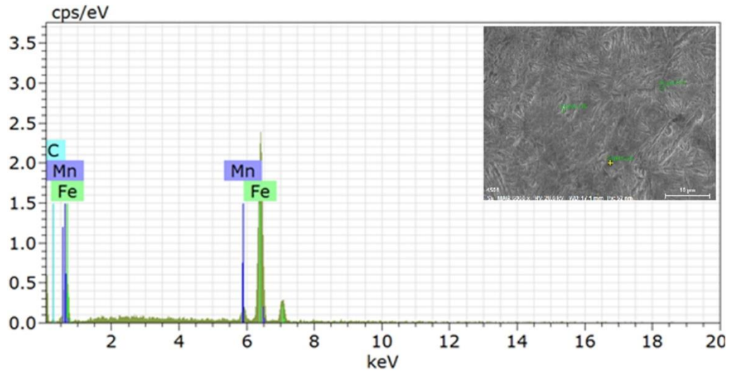
Şekil 5.116. T200 1,2 20 numunesine ait EDS analizi grafiği
