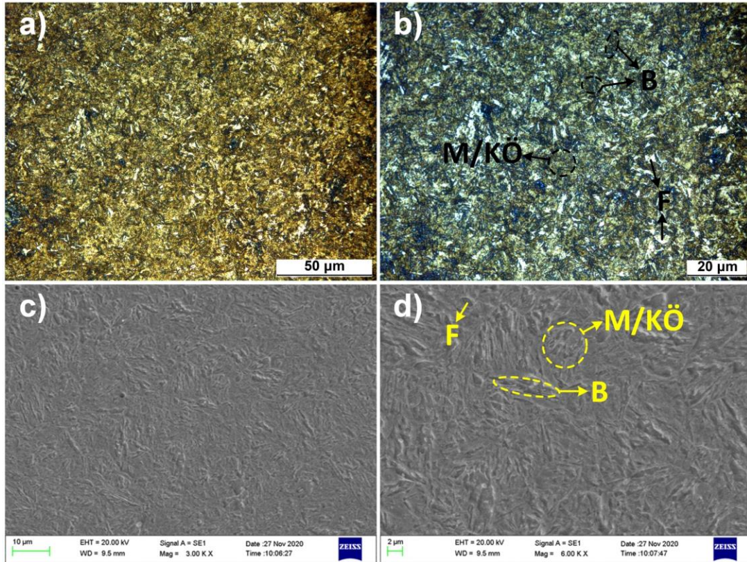
Şekil 5.30. H675 1,2 30 numunesine ait OM ve SEM görüntüleri
