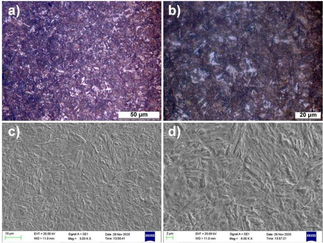
Şekil 5.69. Cr ilavesiz T200 0 20 numunesine ait OM ve SEM görüntüleri
