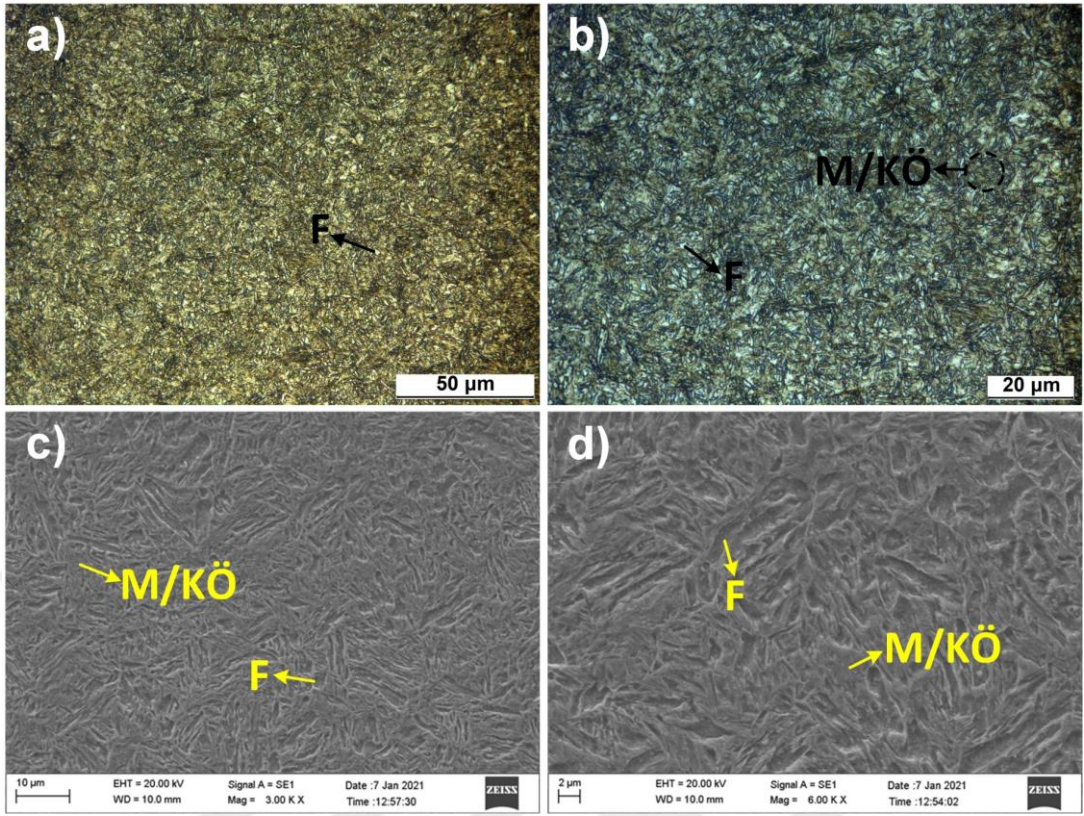
Şekil 5.22. N_{0.8} numunesine ait OM ve SEM görüntüleri
