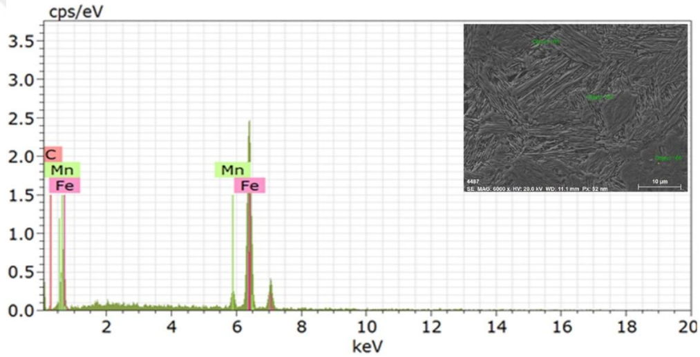
Şekil 5.78. S650 1,230 numunesine ait EDS analizi grafiği
