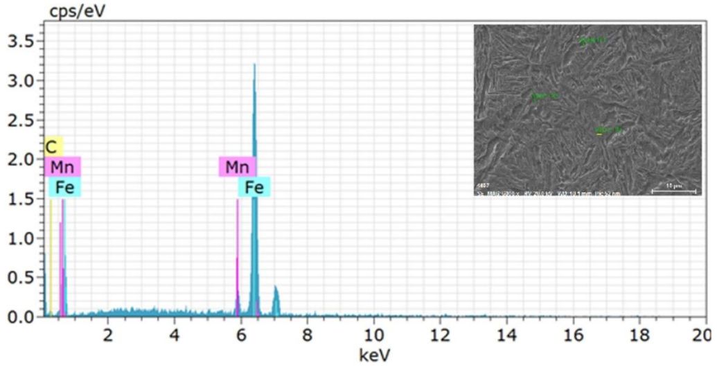
Şekil 5.76. N 1.2 numunesine ait EDS analizi grafiği
