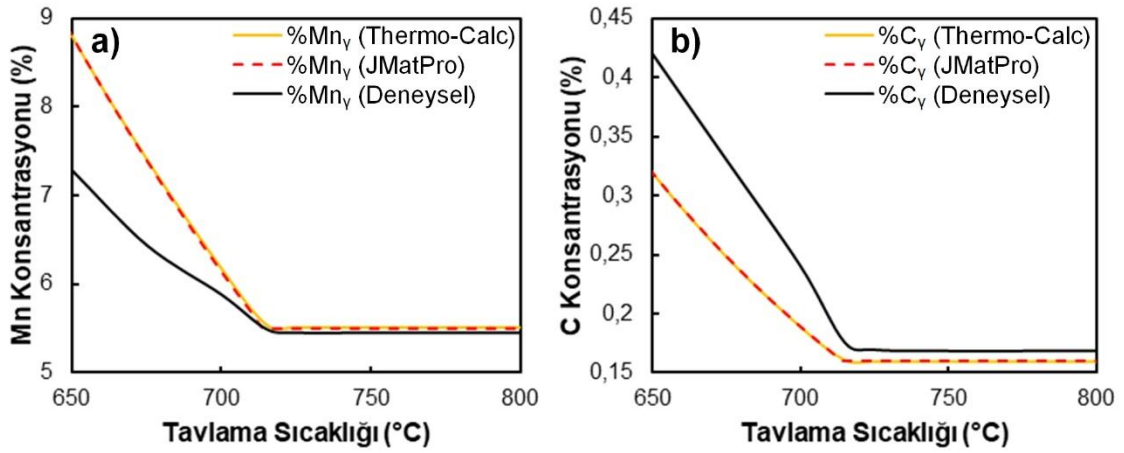
Şekil 5.83. Teorik ve deneysel verilere göre tavlama sıcaklığındaki değişimin kalıntı östenit bileşimi üzerindeki etkisi; a) Mn konsantrasyonu, b) C konsantrasyonu
