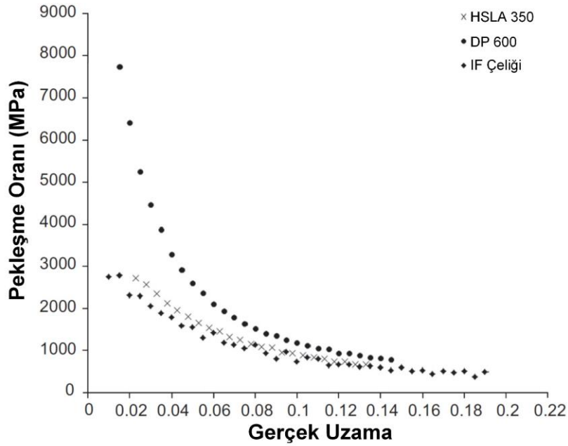
Şekil 2.4. DP, IF ve HSLA 350 çeliklerinin pekleşme oranları [47]
