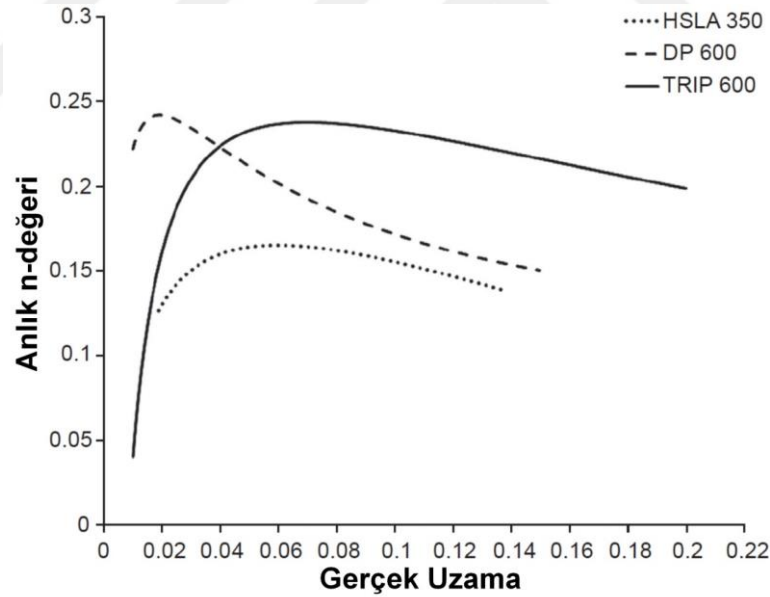
Şekil 2.8. HSLA, TRIP ve DP çelikleri için gerçek uzama değerine karşılık gelen anlık pekleşme üssünün (n değeri) karşılaştırması [47]
