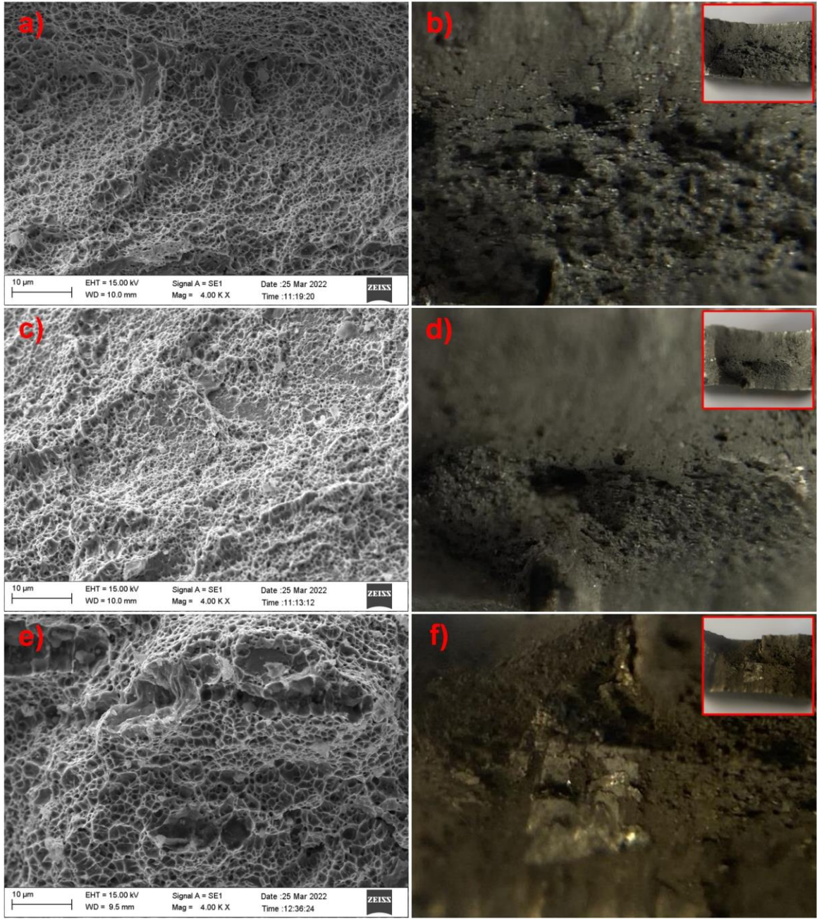
Şekil 5.166. Kopma yüzeylerinin SEM görüntüleri; a) T200 0,420 , c) T200 0,820 , e) T200 1,220 ile makro görüntüleri; b) T200 0,420 , d) T200 0,820 , f) T200 1,220
