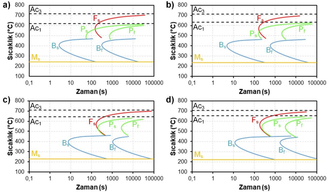
Şekil 5.8. Farklı oranlarda Cr içeren Fe-0.16C-5.5Mn çeliğine ait TTT diyagramları; a) %0 Cr, b) %0,4 Cr, c) %0,8 Cr, d) %1,2 Cr
