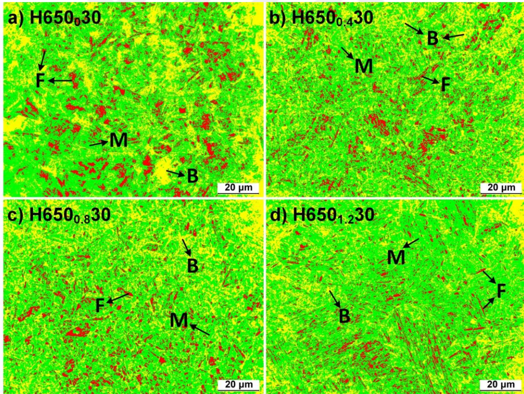
Şekil 5.57. Farklı oranlarda Cr içeren numunelere ait renklendirilmiş OM görüntüleri
