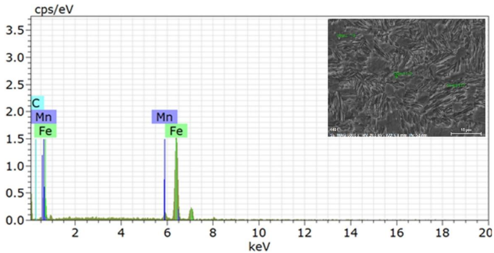
Şekil 5.79. S675 1,230 numunesine ait EDS analizi grafiği
