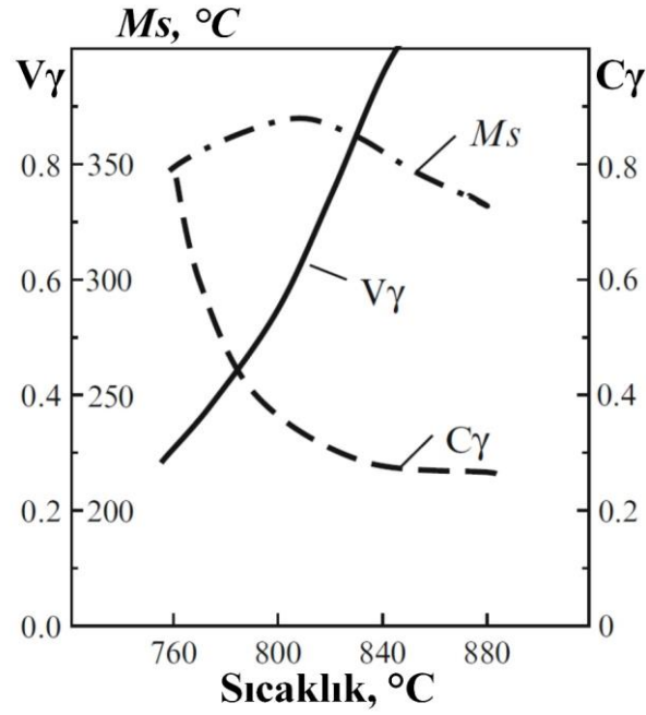
Şekil 2.30. İki fazlı bölgedeki tavlama sıcaklığının, 30 °C/s soğutma hızında 0.06C-Mn-Cr-B çeliği için östenit fraksiyonu, karbon içeriği ve M_s sıcaklığı üzerindeki etkisi [94]
