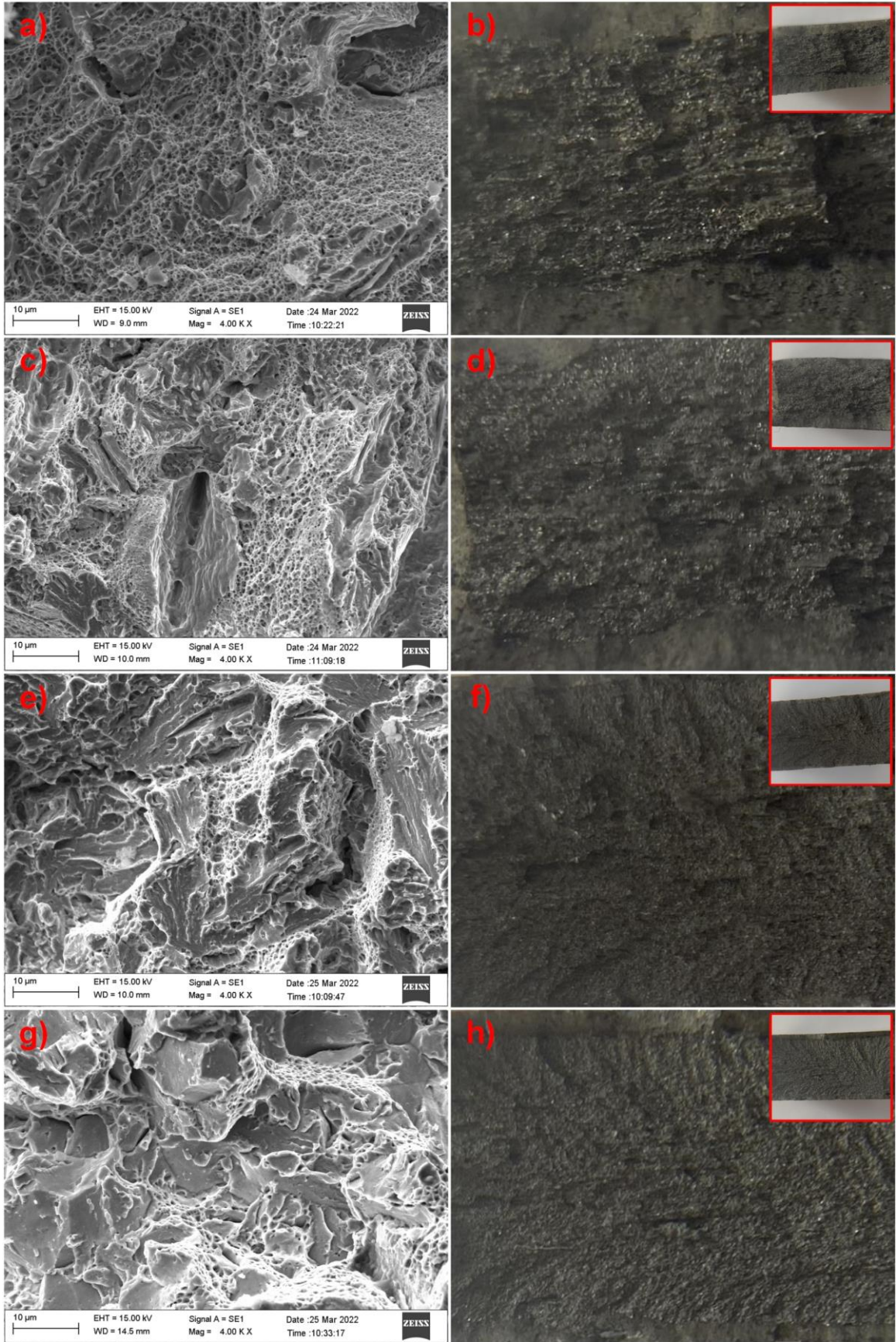
Şekil 5.142. Kopma yüzeylerinin SEM görüntüleri; a) H650 1,230 , c) H675 1,230 , e) H700 1,230 , g) H800 1,230 ile makro görüntüleri; b) H650 1,230 , d) H675 1,230 , f) H700 1,230 , h) H800 1,230
