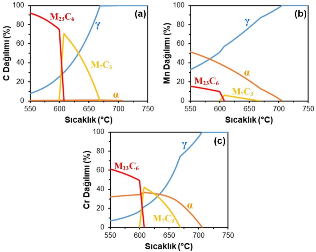
Şekil 5.18. %1,2 Cr ilaveli Fe-0.16C-5.5Mn çeliğinde görülen fazlara ait C, Mn ve Cr dağılımları
