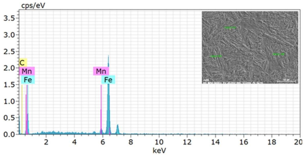
Şekil 5.119. T300 1,260 numunesine ait EDS analizi grafiği
