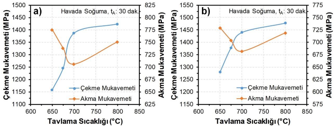
Şekil 5.143. Hava ortamında soğutulan Cr ilavesiz ve %1.2 Cr ilaveli numunelerin akma ve çekme mukavemetleri; a) %0 Cr, b) %1.2 Cr
