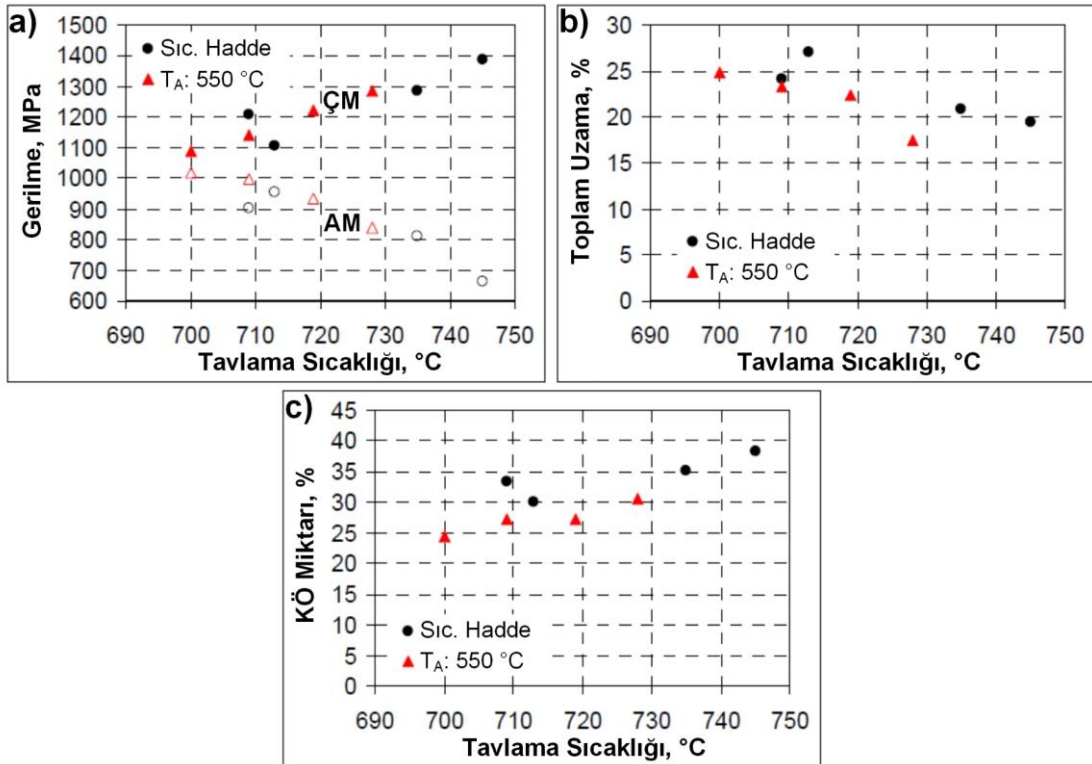
Şekil 3.12. %6.7 Mn’li çeliğin başlangıçtaki mikroyapısının, farklı sıcaklıklardaki kritik tavlama sonrasında çekme özellikleri ve kalıntı östenit miktarı üzerine etkisi [156]
