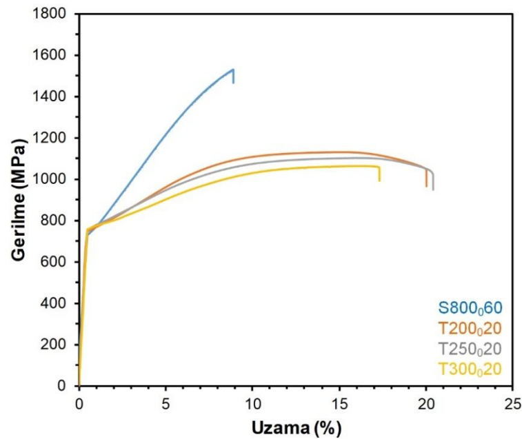
Şekil 5.155. S800 0.60 , T200 0.20 , T250 0.20 ve T300 0.20 numunelerinin gerilme-uzama grafikleri
