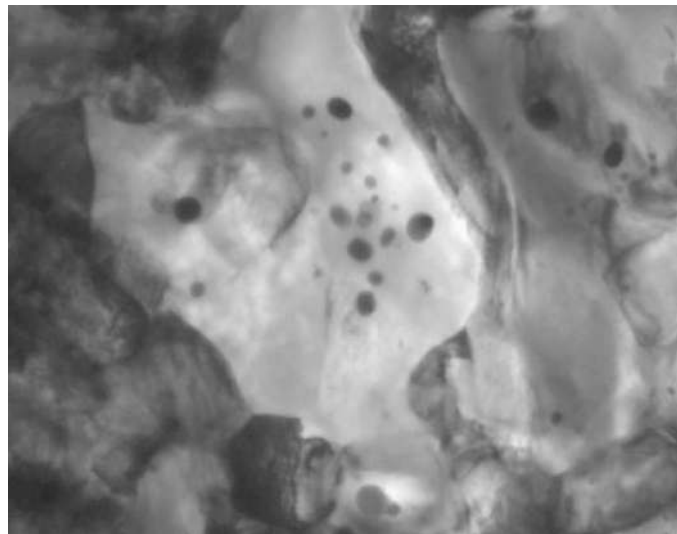
Şekil 2.22. Düşük kritik tavlama sıcaklığında tavllanmış bir çelikte karbür oluşumu [94]
