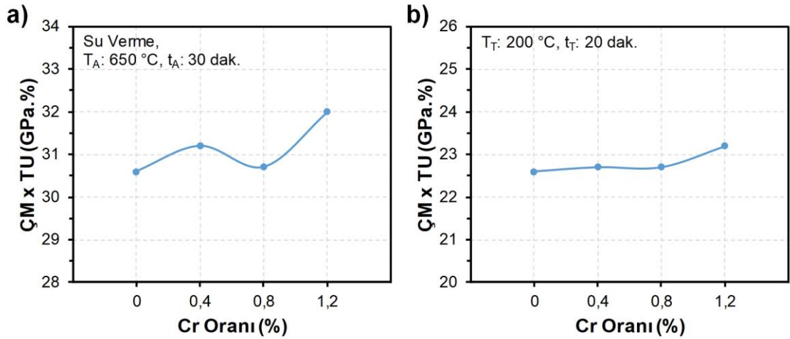
Şekil 5.169. Farklı ısıtım proseslerinde Cr oranının 0.16C-5.5Mn çeliğinin ÇM – TU kombinasyonu üzerindeki etkisi; a) Kritik tavlama işlemi, b) Temperleme ısıtım işlemi
