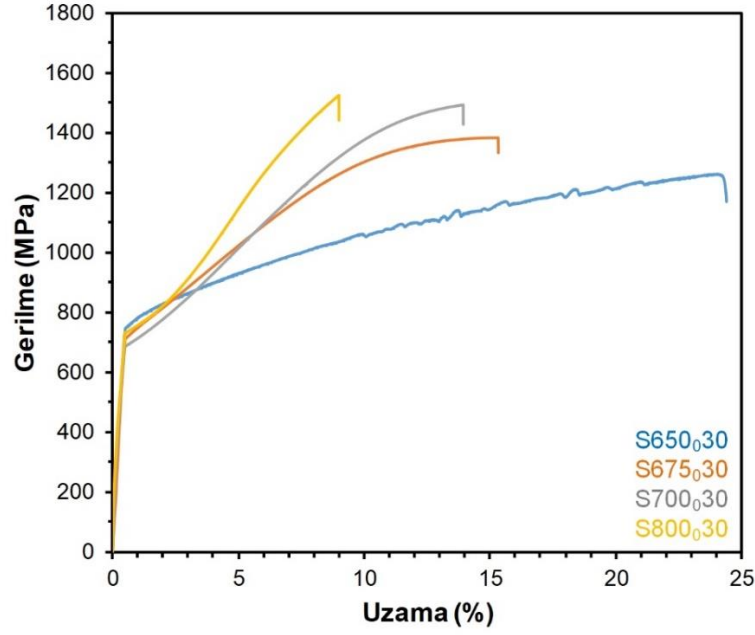
Şekil 5.133. S650 0 30, S675 0 30, S700 0 30 ve S800 0 30 numunelerinin gerilme-uzama grafikleri
