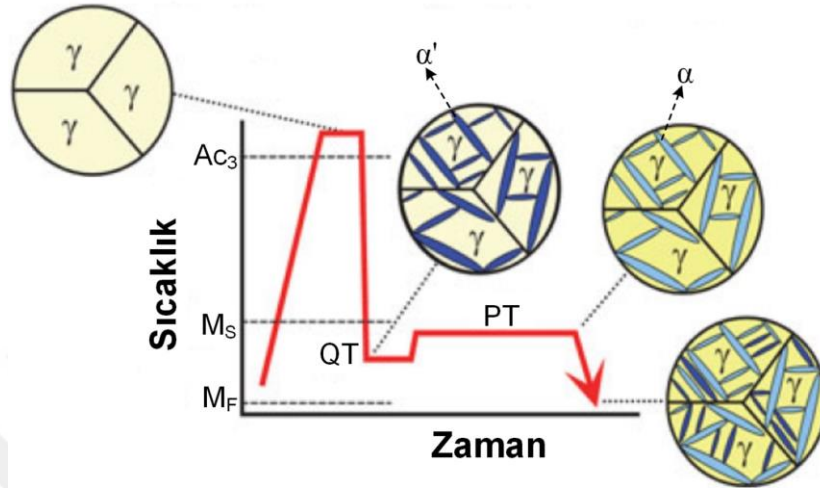
Şekil 2.14. Q&P çelikleri için ısıtma işlemi döngüsü ve gerçekleşen faz dönüşümlerinin şematik gösterimi. (QT: Su verme sıcaklığı, PT: Ayrıştırma sıcaklığı) [79]
