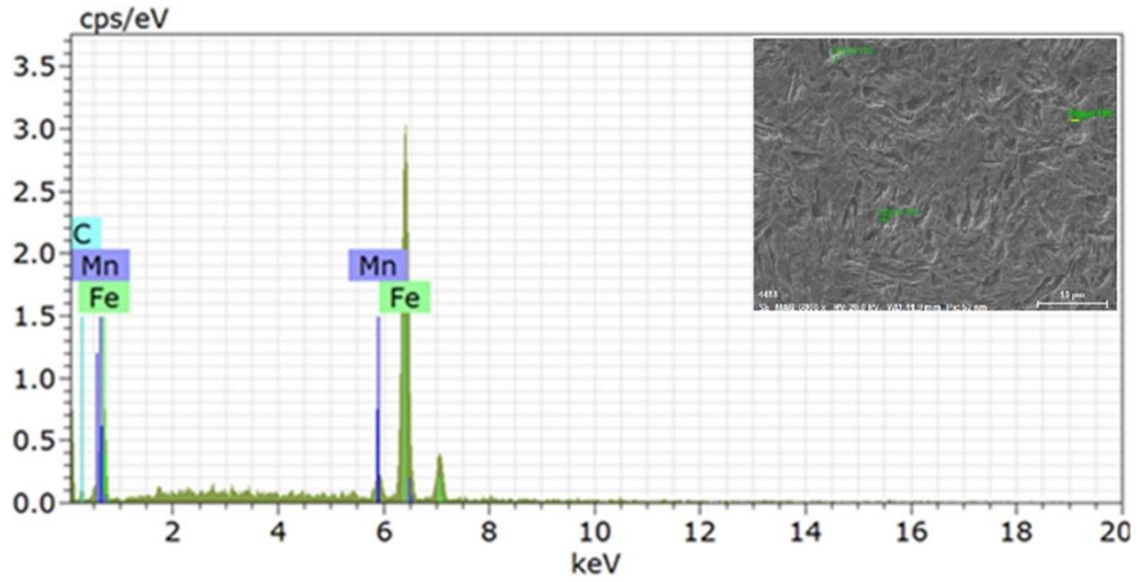
Şekil 5.80. S700 1,230 numunesine ait EDS analizi grafiği
