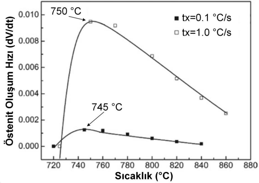
Şekil 2.20. Sıcaklığın bir fonksiyonu olarak östenit fazı oluşum hızı (tx: ısıtma hızı) [107]
