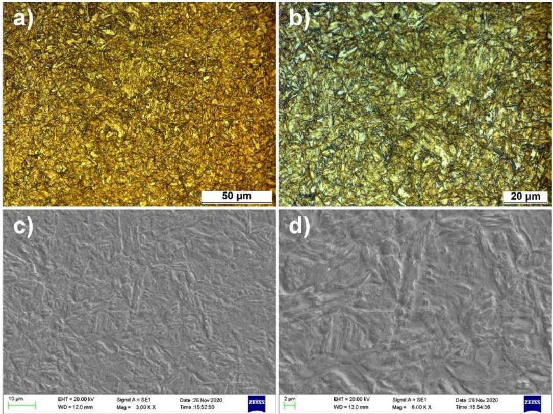
Şekil 5.51. S800 1,260 ( t_A : 60 dk.) numunesine ait OM ve SEM görüntüleri
