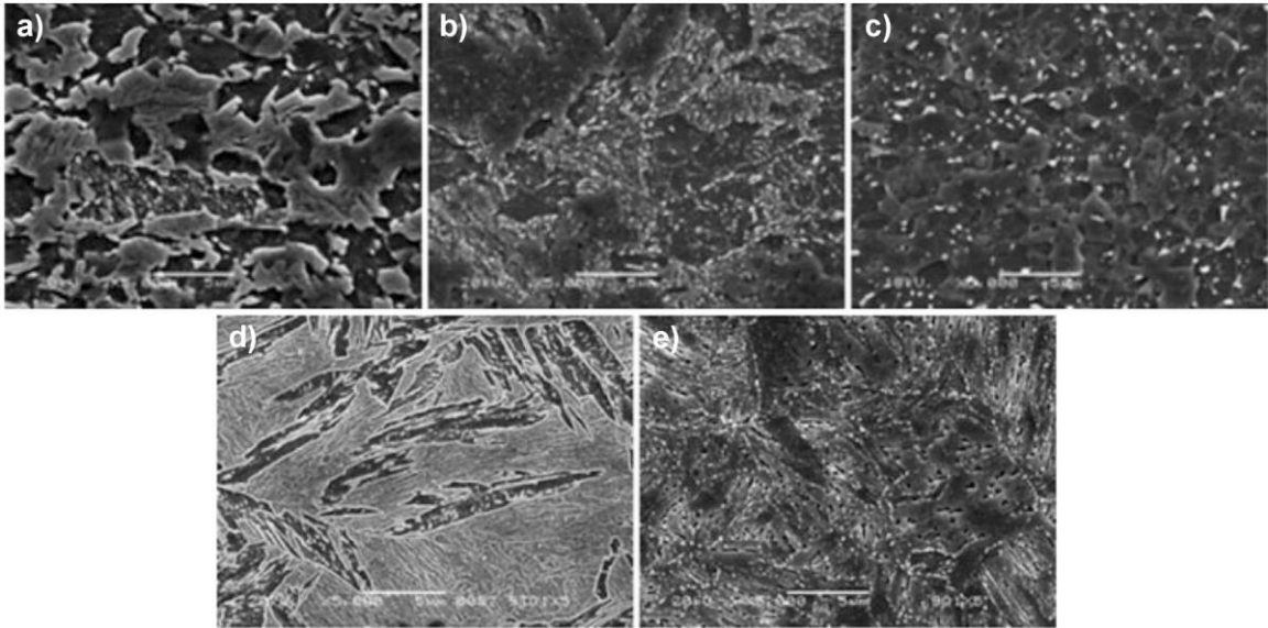
Şekil 3.8. %4 ve %6.7 Mn’li sıcak haddelenmiş ve yığın halinde tavllanmış çeliklerin mikroyapısı; a) %4 Mn - Sıcak haddelenmiş, b) %4 Mn - 550°C’de tavlama, c) %4 Mn - 650°C’de tavlama, (d) %6.7 Mn - Sıcak haddelenmiş, e) %6.7 Mn - 550°C’de tavlama [5]
