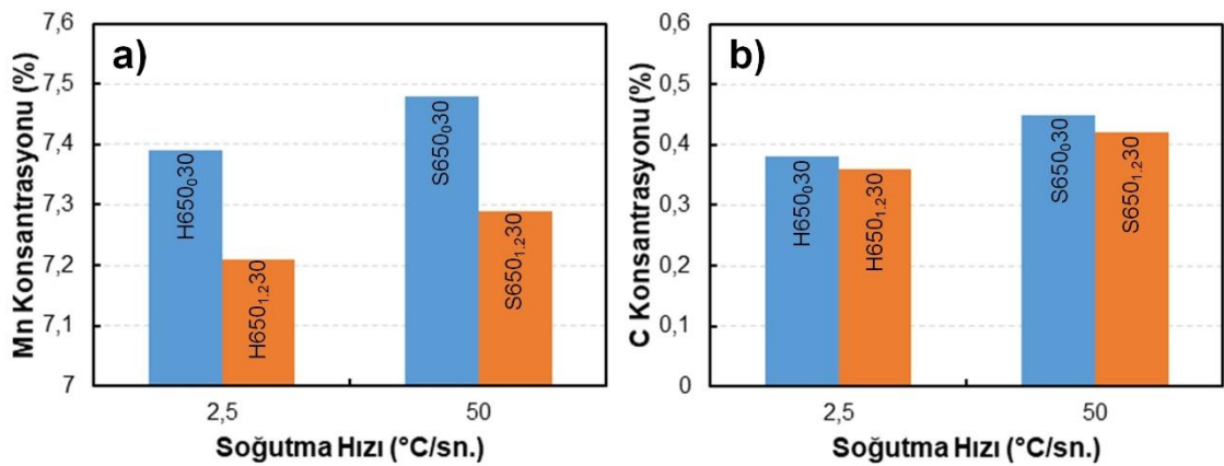
Şekil 5.91. Soğutma hızındaki değişimin kalıntı östenit bileşimi üzerindeki etkisi; a) % Mn, b) % C
