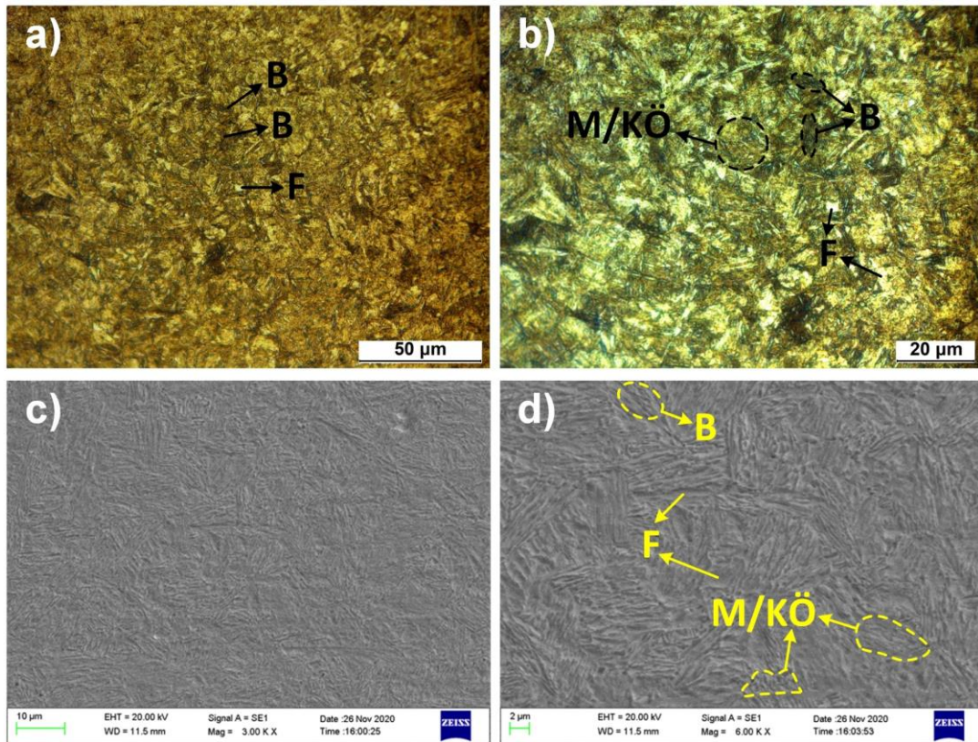
Şekil 5.52. Cr ilavesiz H650 0,30 numunesine ait OM ve SEM görüntüleri
