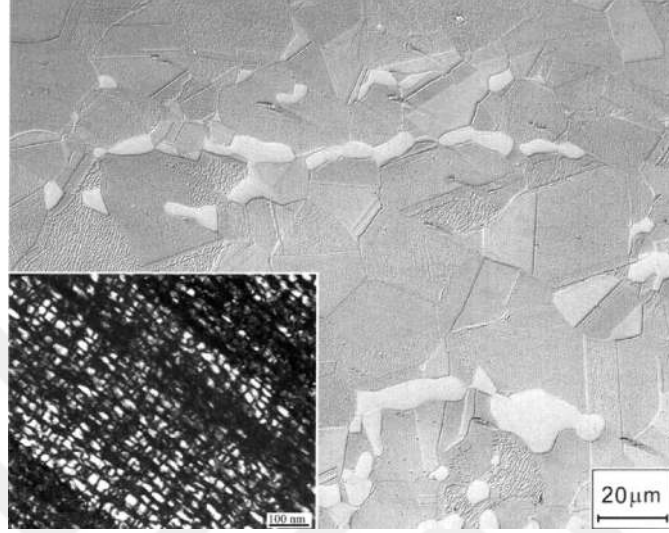
Şekil 2.9. Tipik bir L-IP çeliğine ait optik mikrogram; östenit matrisi, ikizleri ortaya çıkarır ve \alpha -ferrit, parlak faz olarak görünür. TEM (karanlık alan) görüntüsü ise, nano boyutlu \kappa -karbür çökeltilerini temsil etmektedir [59]
