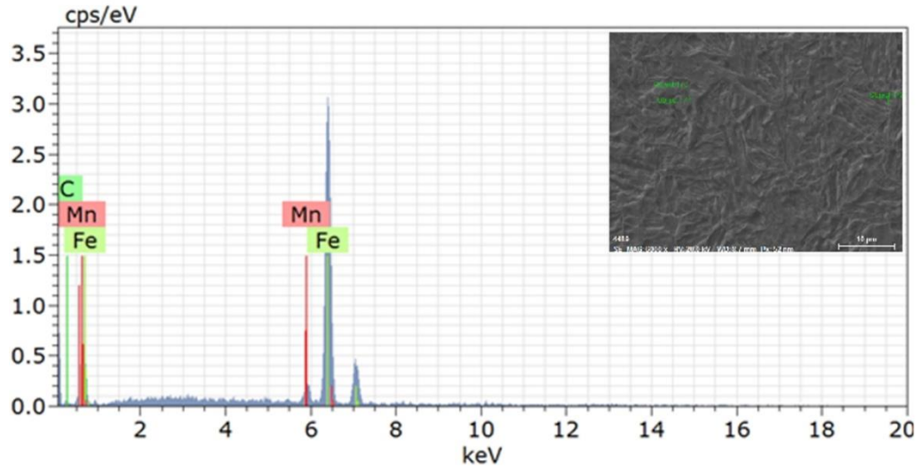
Şekil 5.81. S800 1,230 numunesine ait EDS analizi grafiği
