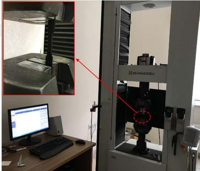
Şekil 4.17. Çekme testi cihazı
