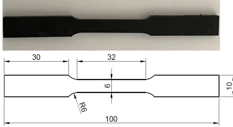
Şekil 4.18. ASTM E8 Çekme numunesi ve standart ölçüleri
