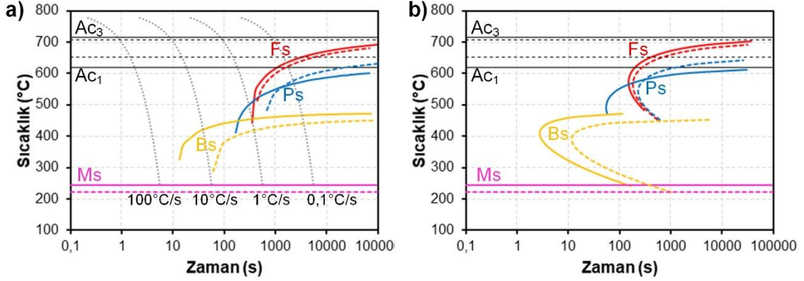
Şekil 5.9. Cr oranı %0 (Düz çizgiler) ve %1,2 (Kesikli çizgiler) olan Fe-0.16C-5.5Mn çelikleri için dönüşüm eğrileri; a) CCT eğrileri, b) TTT eğrileri
