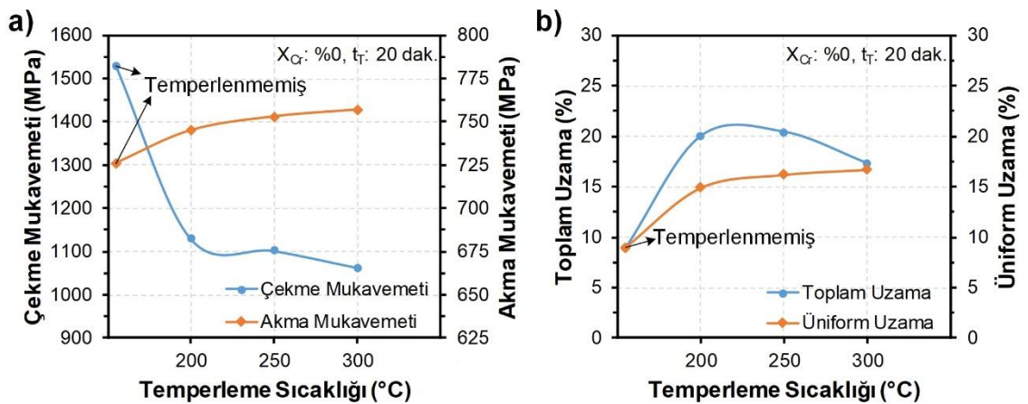
Şekil 5.157. Temperleme sıcaklığının 0.16C-5.5Mn çeliğinin mekanik özellikleri üzerindeki etkisi, a) Çekme ve akma mukavemeti; b) Üniform ve toplam uzama miktarı
