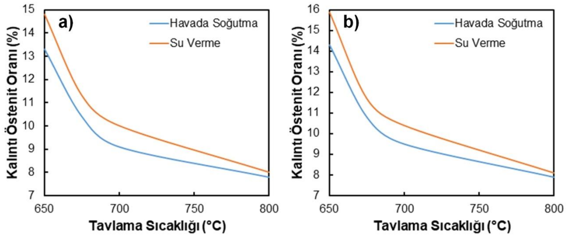
Şekil 5.95. Hava ve su ortamlarında soğutulmuş numunelerdeki kalıntı östenit fazı oranlarının değişimi; a) 0.16C-5.5Mn, b) 0.16C-5.5Mn-1.2Cr
