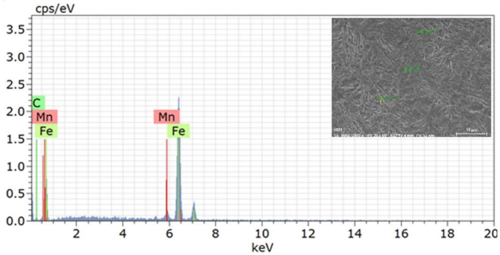
Şekil 5.113. T200 020 numunesine ait EDS analizi grafiği
