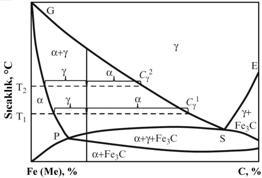
Şekil 2.17. Kritik bölge için tasarlanan ikili Fe (Me) – C diyagramı [94]
