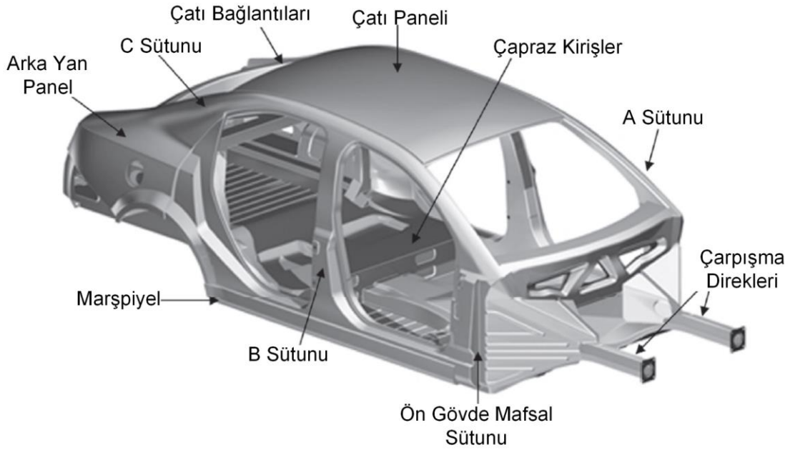
Şekil 2.34. Bazı önemli gövde yapı elemanları [133]
