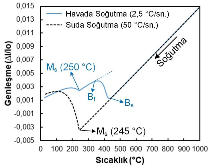
Şekil 5.94. Farklı soğuma hızlarına ait genleşme eğrileri
