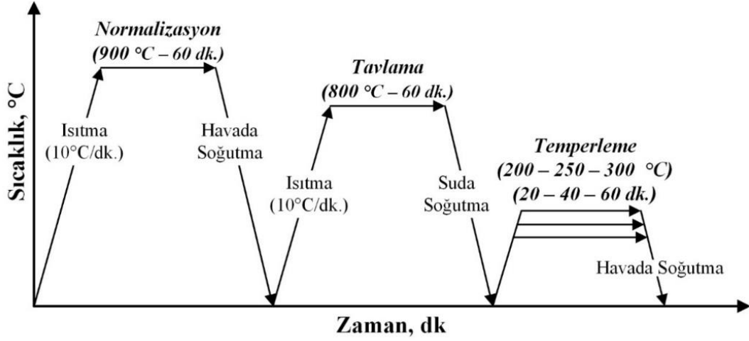
Şekil 4.9. Temperleme işlemine ait termal döngülerin şematik gösterimi
