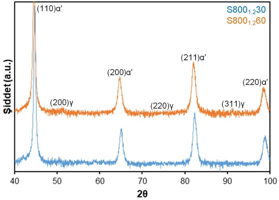
Şekil 5.104. S800 1,2 30 ve S800 1,2 60 numunelerine ait XRD analizi grafiği
