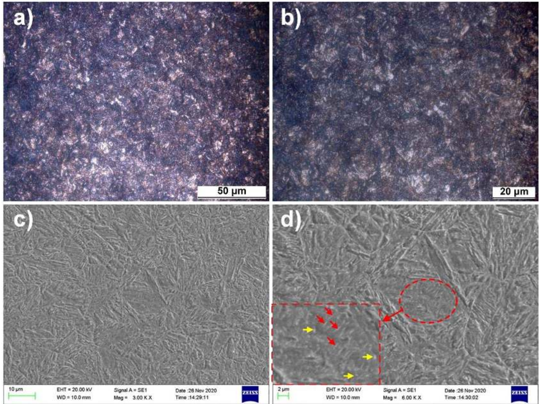
Şekil 5.64. T250 0 20 numunesine ait OM ve SEM görüntüleri
