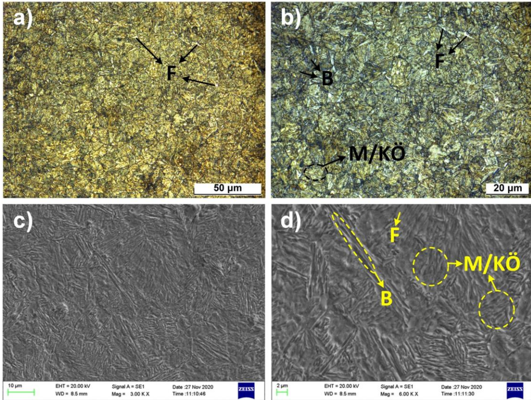
Şekil 5.45. H650 0,8 60 numunesine ait OM ve SEM görüntüleri
