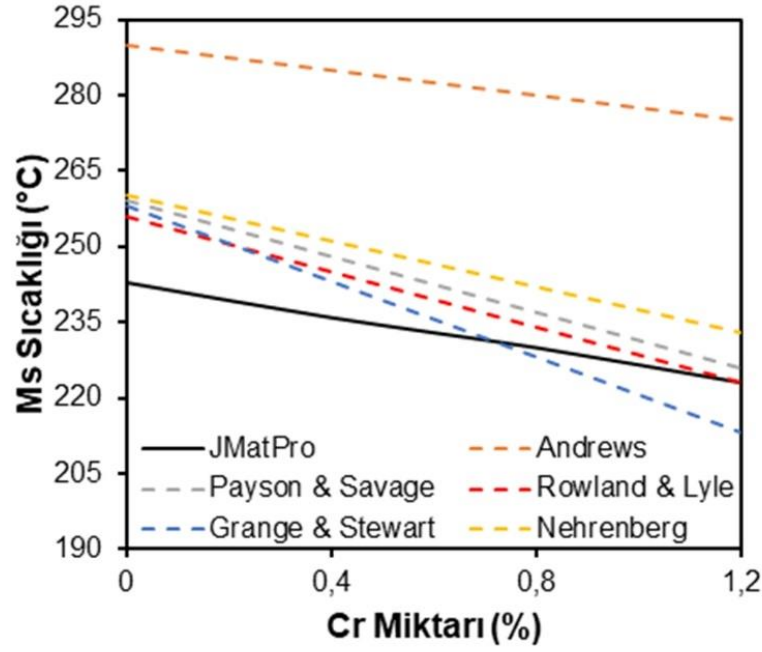
Şekil 5.19. Cr oranındaki artışın M_s sıcaklığı üzerindeki etkisi
