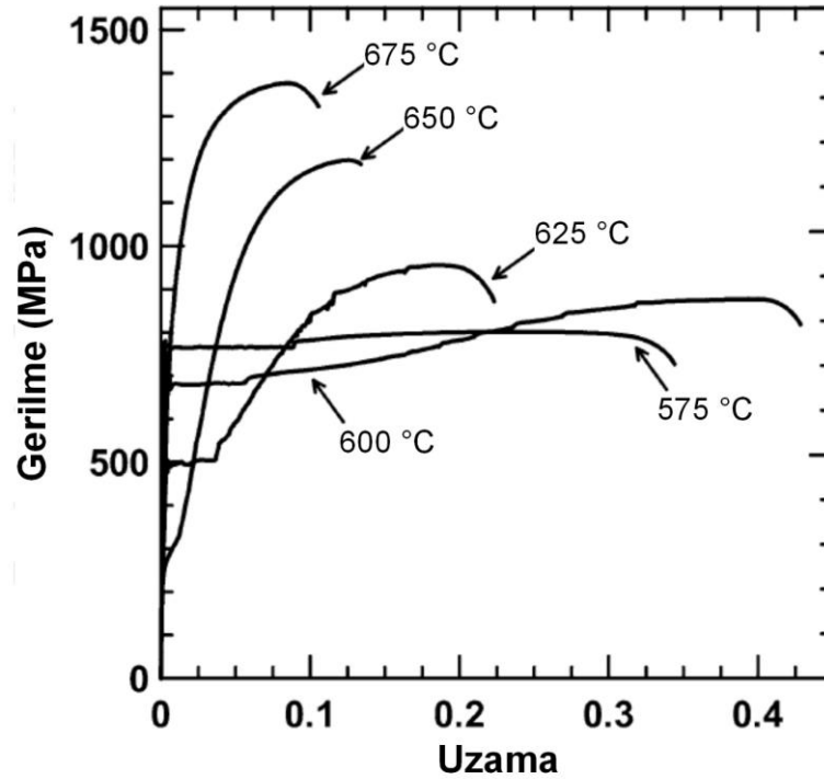
Şekil 3.7. Farklı sıcaklıklarda 1 hafta süresince tavllanmış 0.1C-7.1Mn çeliği numuneleri için gerilme-uzama eğrileri [75]
