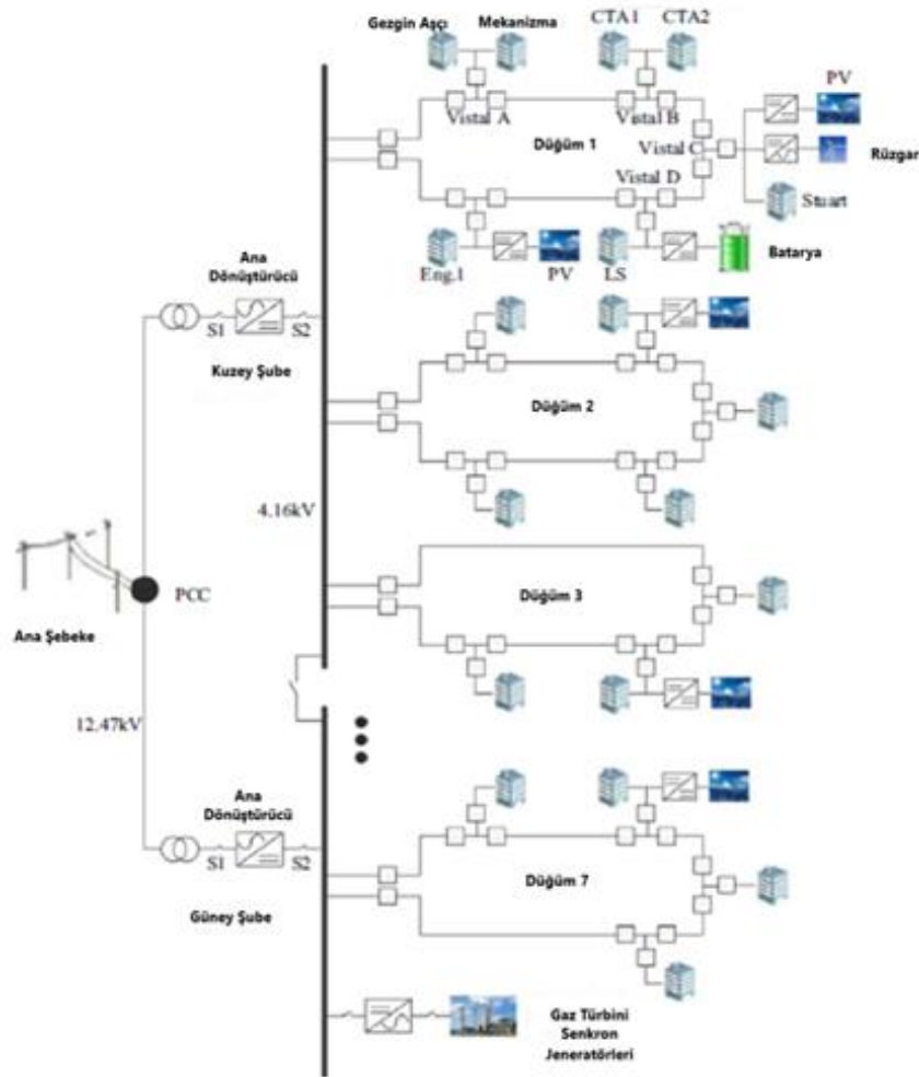
Şekil 2.13. DA-ÇMŞ Mimarisi [50]
