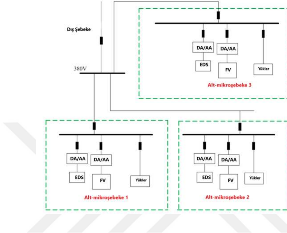
Şekil 2.21. SZ Ecopark ÇMŞ Topolojileri [45]
