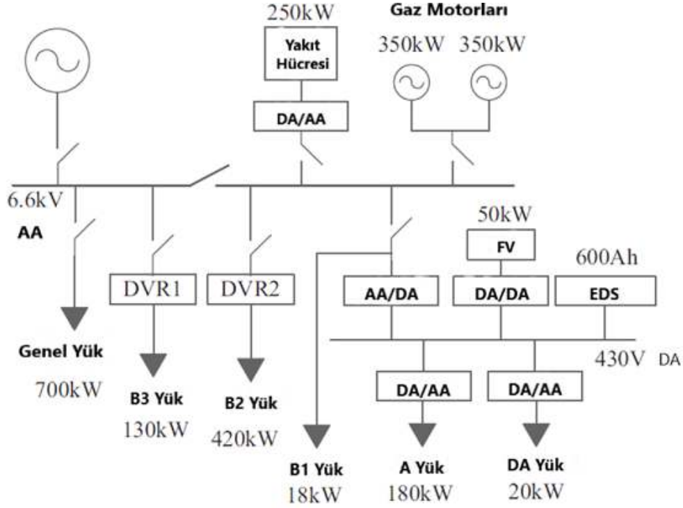
Şekil 2.17. Sendai ÇMŞ topolojisi [45]
