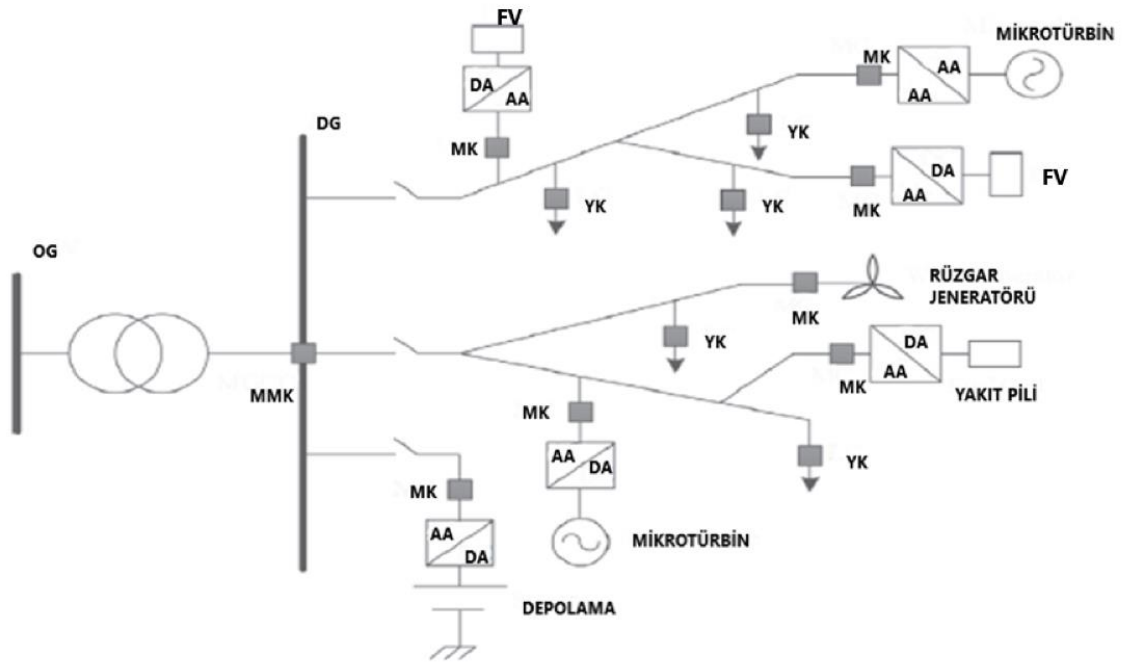
Şekil 2.12. AA-ÇMŞ Mimarisi [49]
