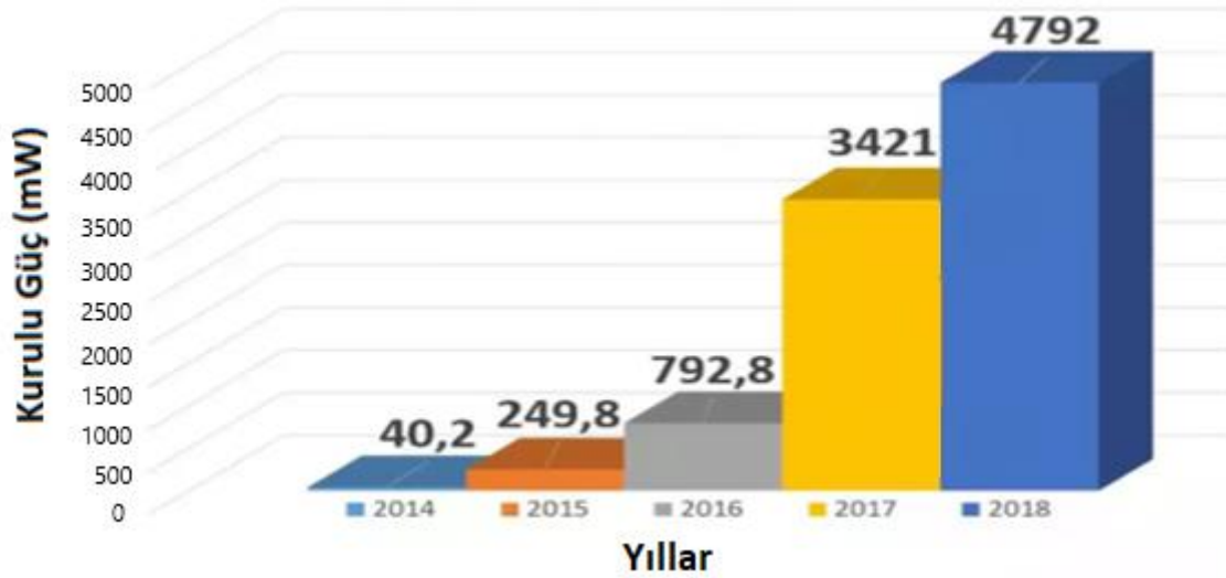
Şekil 2.3 Türkiye'deki Güneş Enerjisi Kurulu Gücünün Yıllara Göre Değişimi Grafiği [26]
