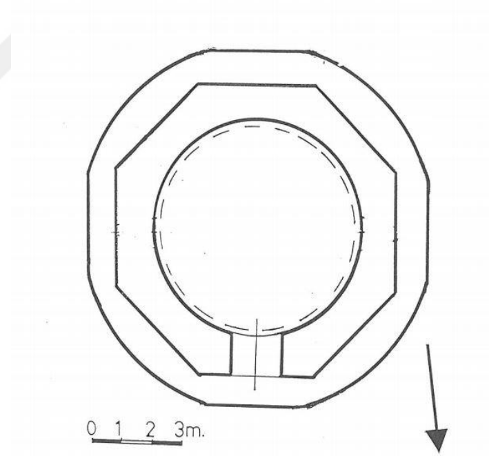
Çizim 5. Kul Yusuf Kümbet Planı (H. Buyruk'tan).
