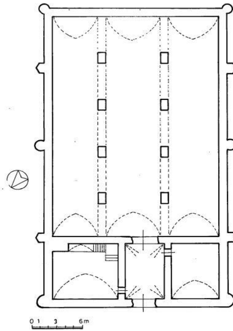
Çizim 7. Aşkale Hacı Bekir Hamı (R.H. Ünal'dan).
