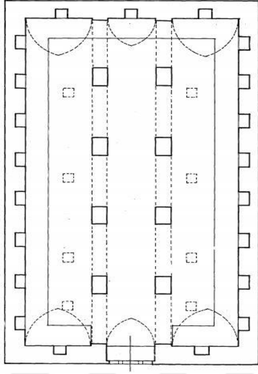
Çizim 8. Aşkale Karasu Hanı (H. Gündoğdu'dan).
