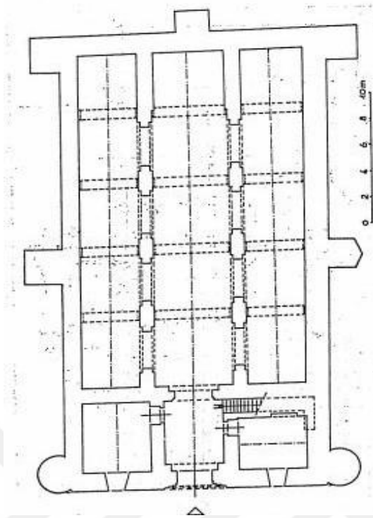
Çizim 6. Bitlis Hüsrev Paşa Hamı (R. H. Ünal'dan).
