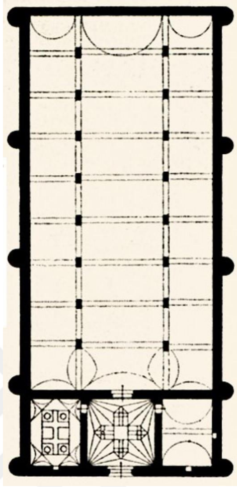
Çizim 1. Kervansaray genel planı (O.Aslanapa'dan)
