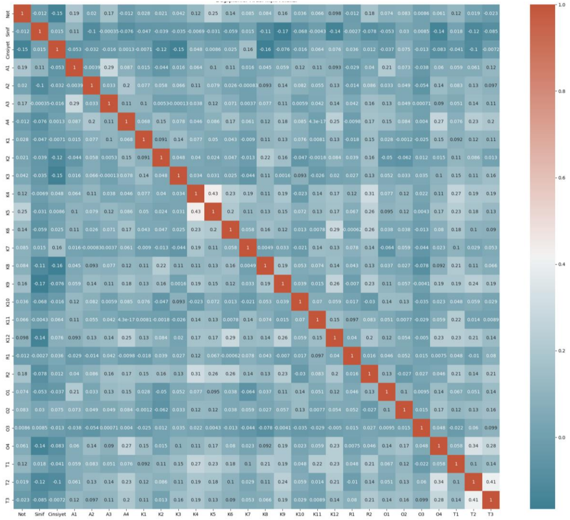
Şekil 4.6 Tüm değişkenlerin korelasyonu
