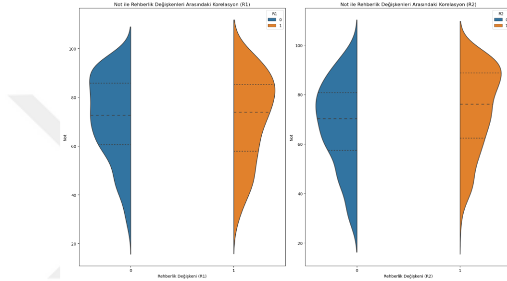
Şekil 4.14 Rehberlik ile Not arasındaki korelasyon
