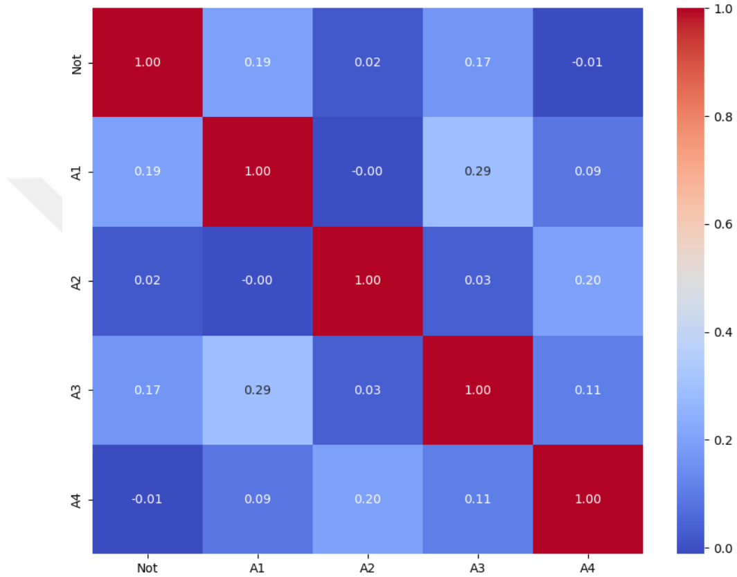
Şekil 4.1. Aile durumları ile Not Arasındaki korelasyon matrisi
