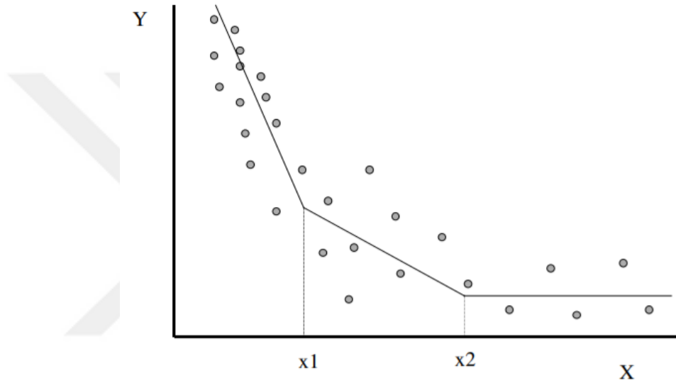
Şekil 2.1: y = f(x) fonksiyonu için düğüm noktaları (Briand vd., 2004)
