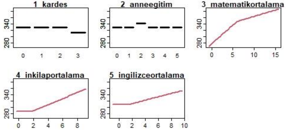
Şekil 3.5. Temel fonksiyonların grafiksel incelenmesi
