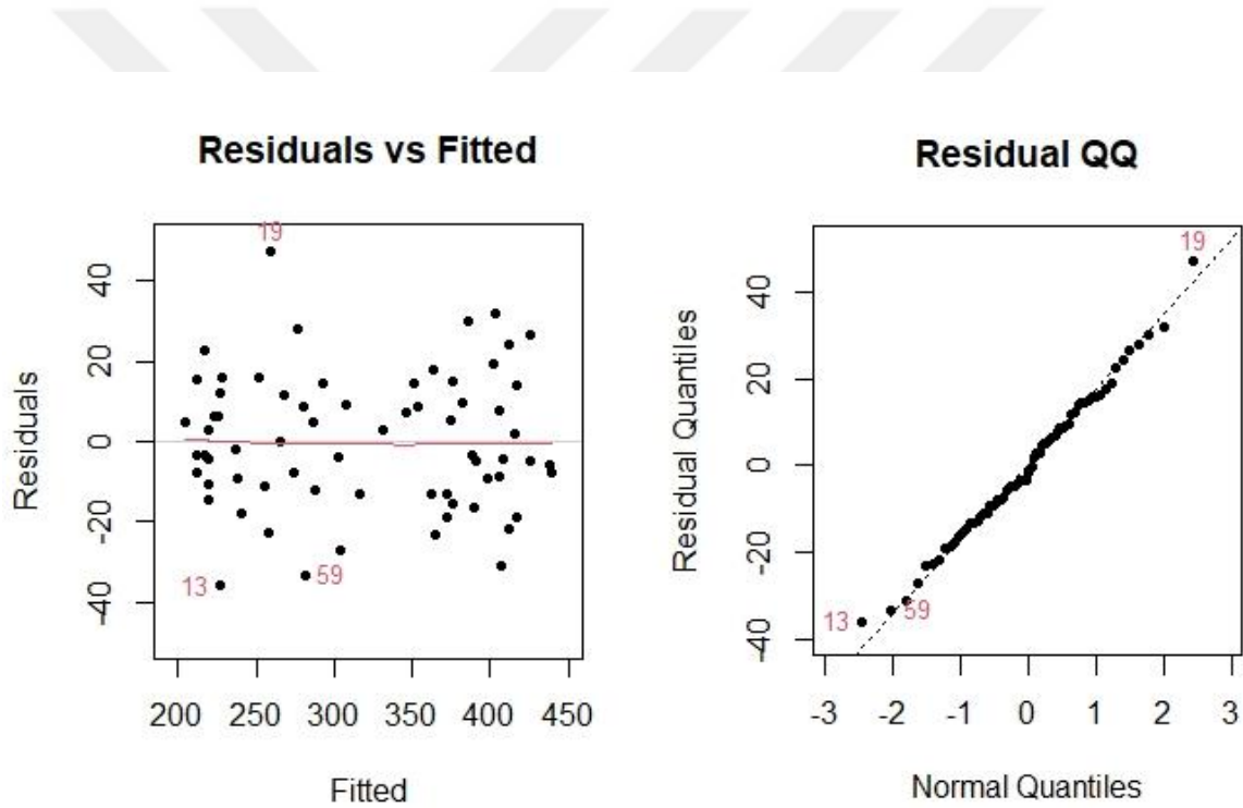
Şekil 3.4: MARS modeli için model uyumunun incelenmesi
