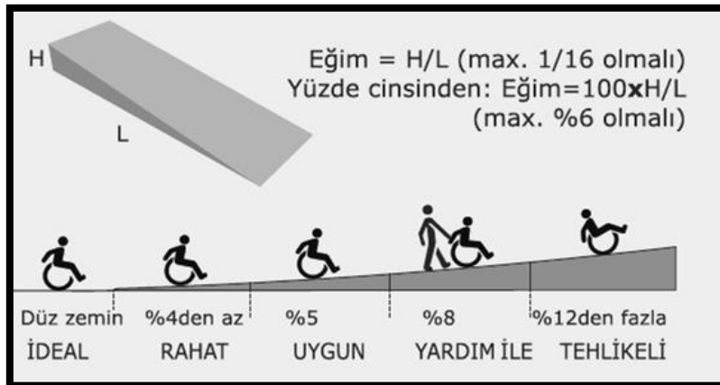
Şekil 131. Rampalarda güvenli eğim yüzde ve aralıkları
