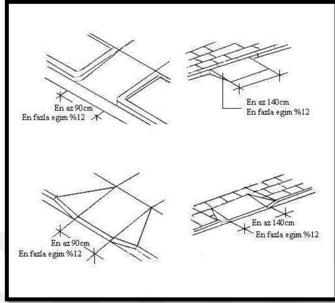
Ek Şekil 41. Kaldırım rampaları 1 (Sürmen, 1995).
