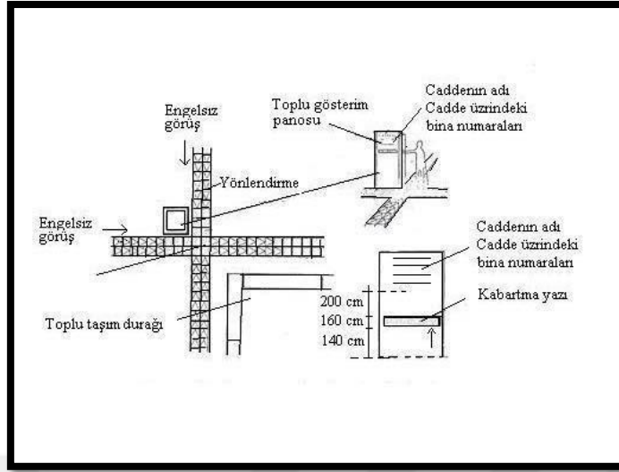
Ek Şekil 40. Yaya yolunda yer kaplamalarıyla yönlendirmeler (TSE,1990).
