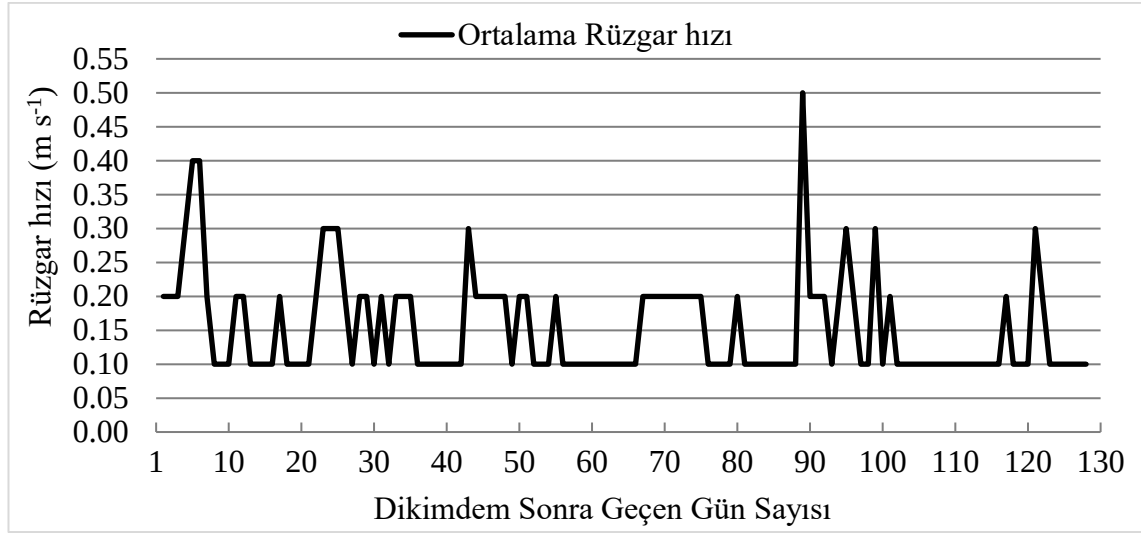
Şekil 4.5. Deneme boyunca sera içinde ölçülen ortalama rüzgâr hızı ( u ) değerleri
