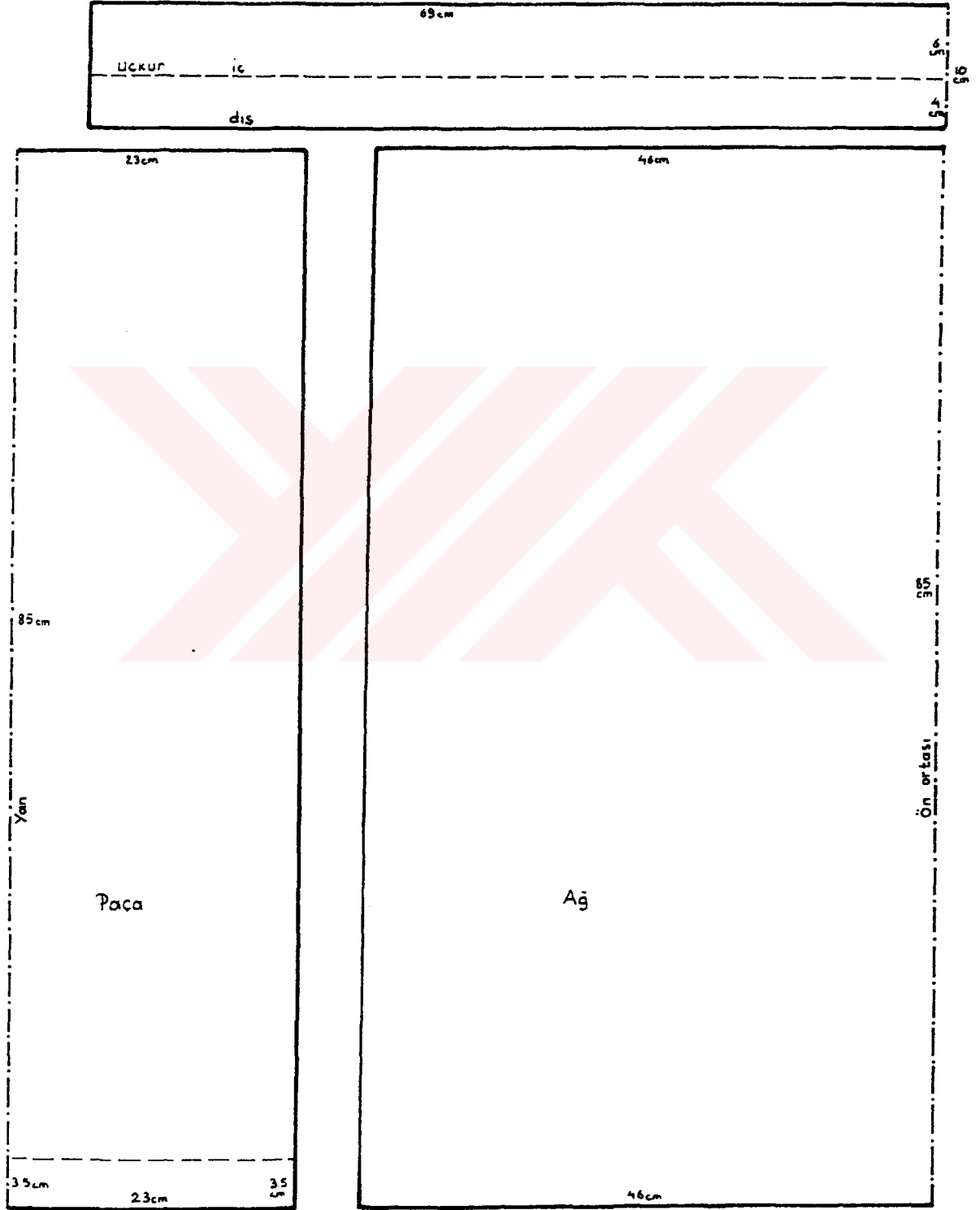
ÇİZİM 53b ÇOCUK ŞALVARI KALIP ÇİZİMİ
