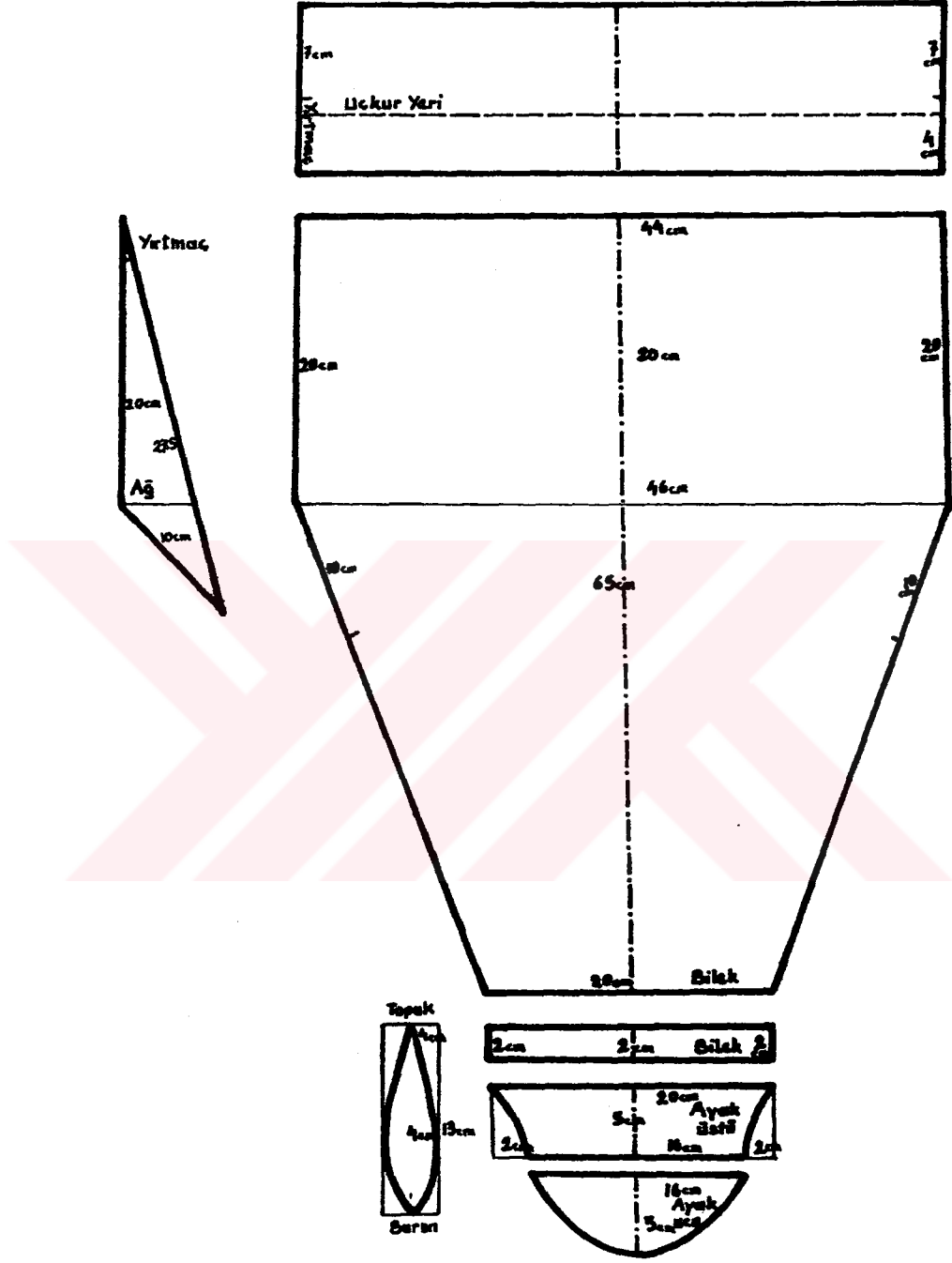
ÇİZİM 1c ÇOCUK ÇAKŞIRI KALIP ÇİZİMİ
