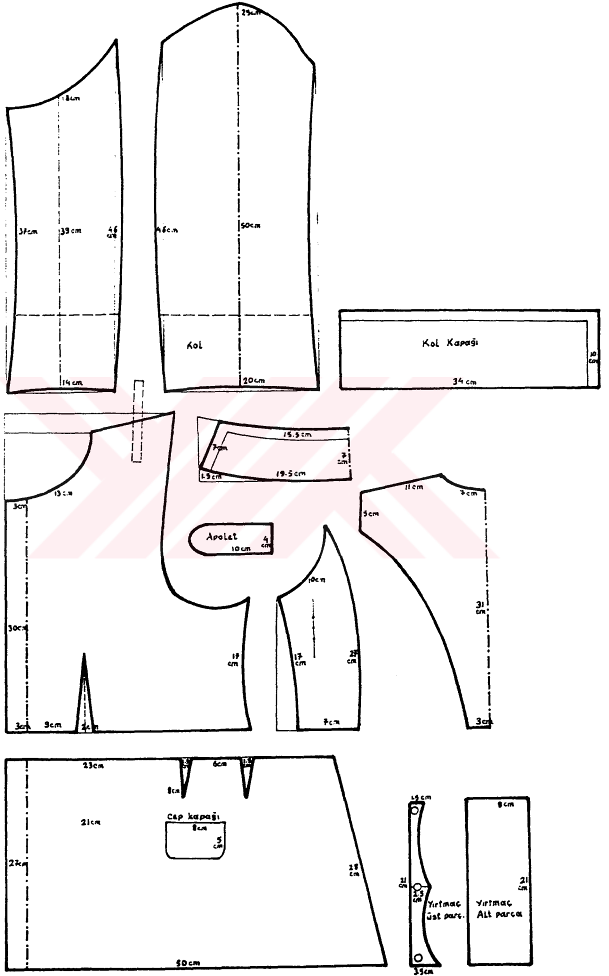
ÇİZİM 44b ÇOCUK CEKETİ KALIP ÇİZİMİ
