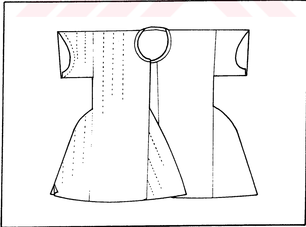
ÇİZİM 39a ÇOCUK KAFTANI TEKNİK ÇİZİMİ
