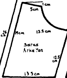
ÇİZİM 47d ÇOCUK CEPKEN TAKIM KALIP ÇİZİMİ
