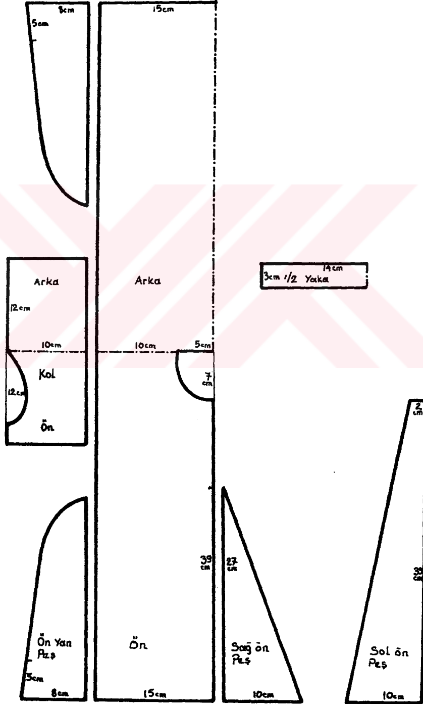
ÇİZİM 36 ÇOCUK ENTARİSİ KALIP ÇİZİMİ
