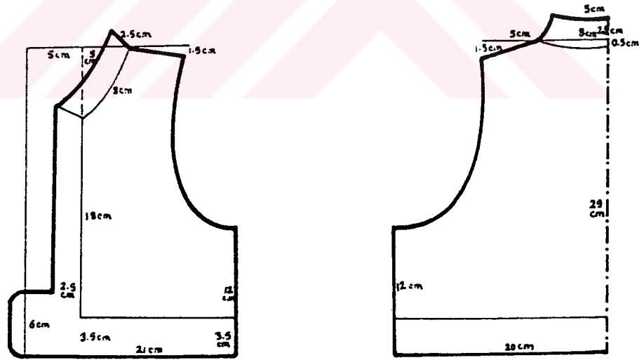
ÇİZİM 65b ÇOCUK YELEĞİ KALIP ÇİZİMİ
