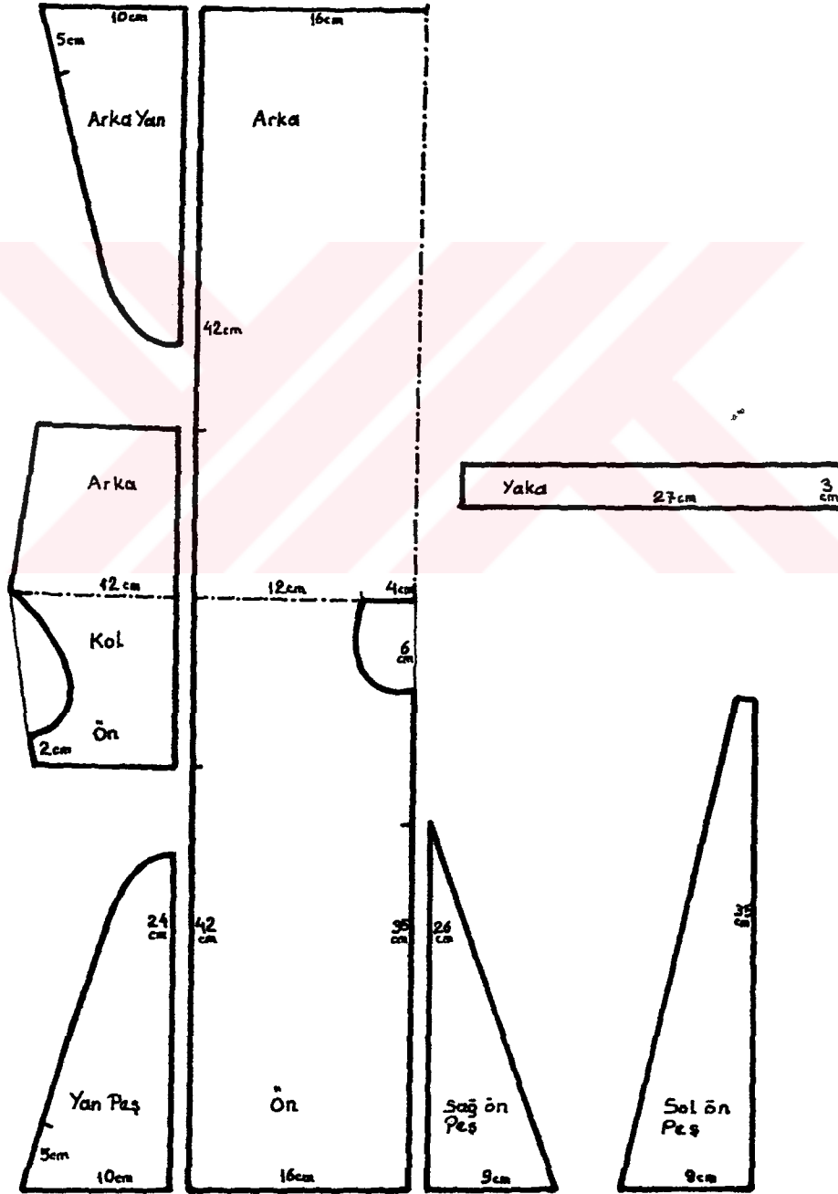
ÇİZİM 96 ÇOCUK KAFTANI KALIP ÇİZİMİ
