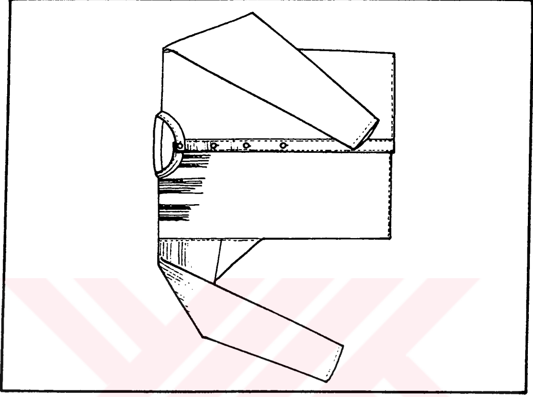
ÇİZİM 45c ÇOCUK GÖMLEĞİ TEKNİK ÇİZİMİ
