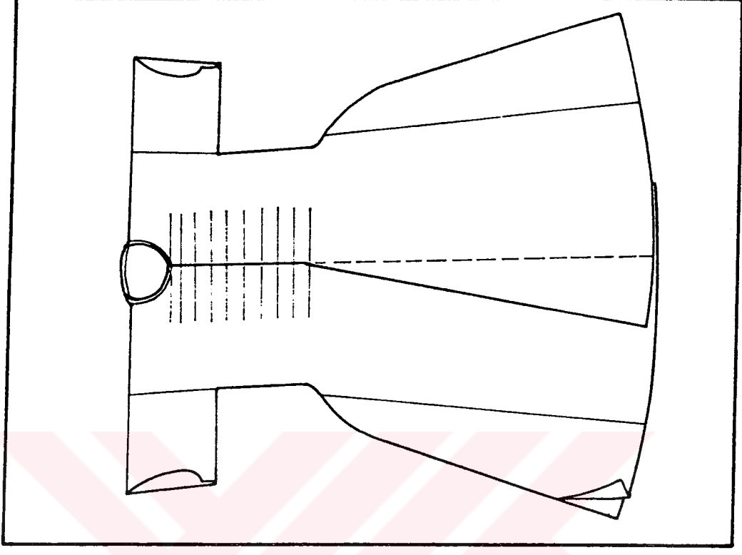
ÇİZİM 28a ÇOCUK KAFTANI TEKNİK ÇİZİMİ
