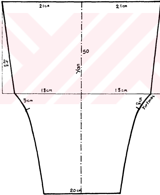
ÇİZİM 15b ÇOCUK ÇAKŞIRI KALIP ÇİZİMİ
