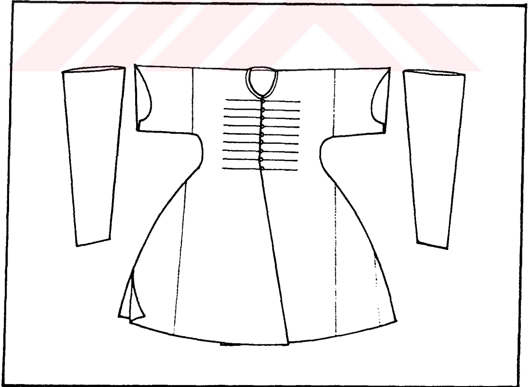
ÇİZİM 11a ÇOCUK KAFTANI TEKNİK ÇİZİMİ
