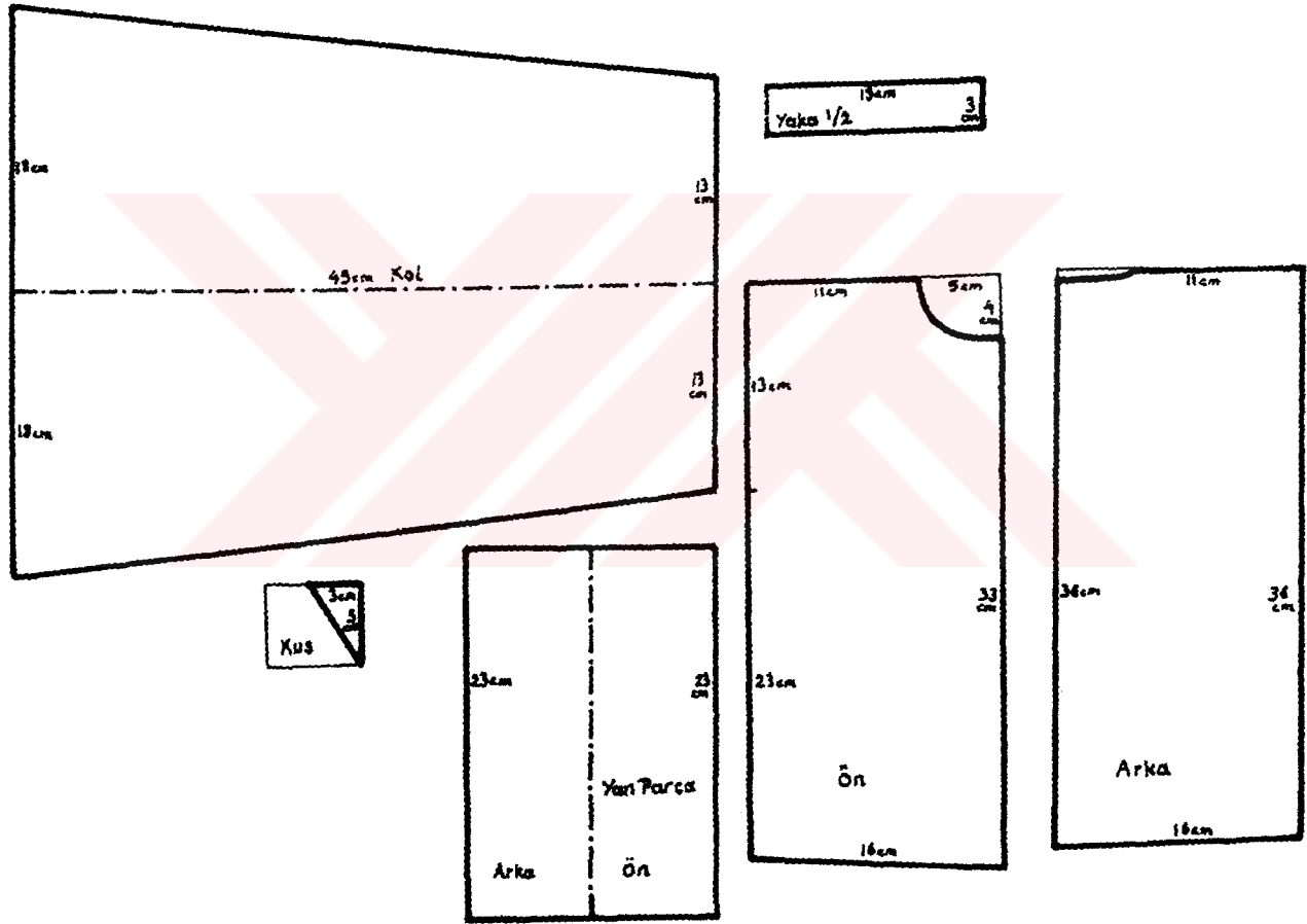
ÇİZİM 50c ÇOCUK CEPKENİ KALIP ÇİZİMİ
