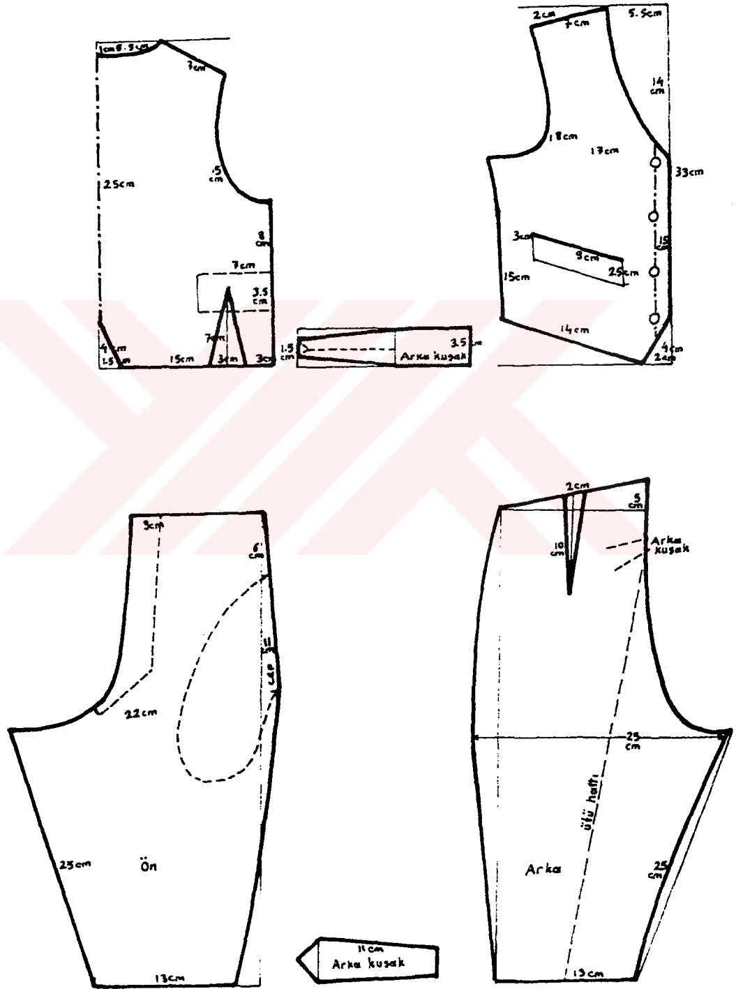
ÇİZİM 59e ÇOCUK YELEĞİ VE PANTOLONU KALIP ÇİZİMİ
