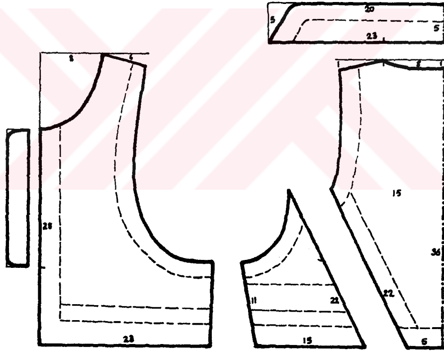
ÇİZİM 69b ÇOCUK YELEĞİ KALIP ÇİZİMİ
