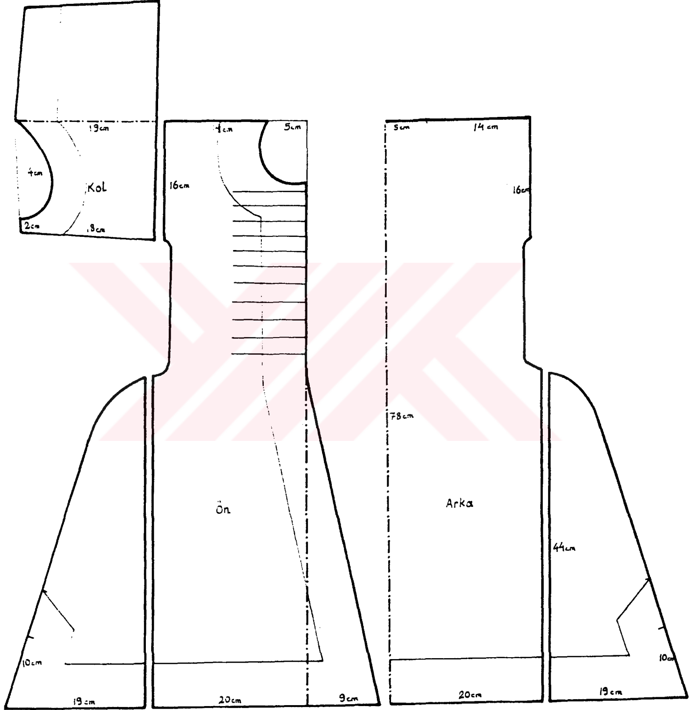
ÇİZİM 28b ÇOCUK KAFTANI KALIP ÇİZİMİ
