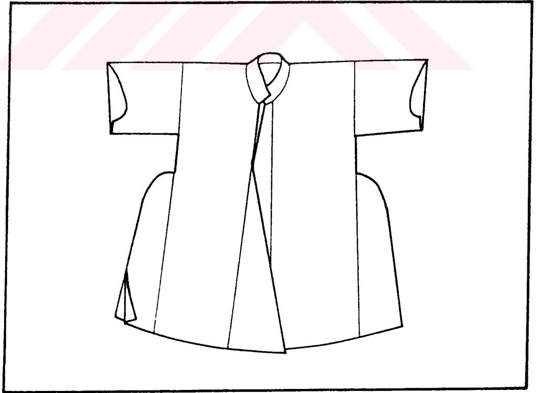
ÇİZİM 4a ÇOCUK ENTARİSİ TEKNİK ÇİZİMİ
