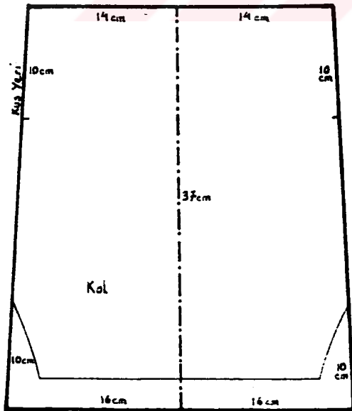
ÇİZİM 51D ÇOCUK CEPKENİ VE YELEĞİ KALIP ÇİZİMİ
