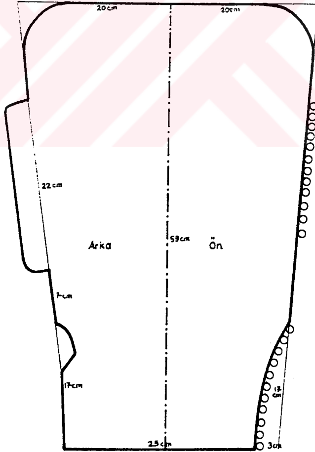
ÇİZİM 49b ÇOCUK CEPKENİ KALIP ÇİZİMİ
