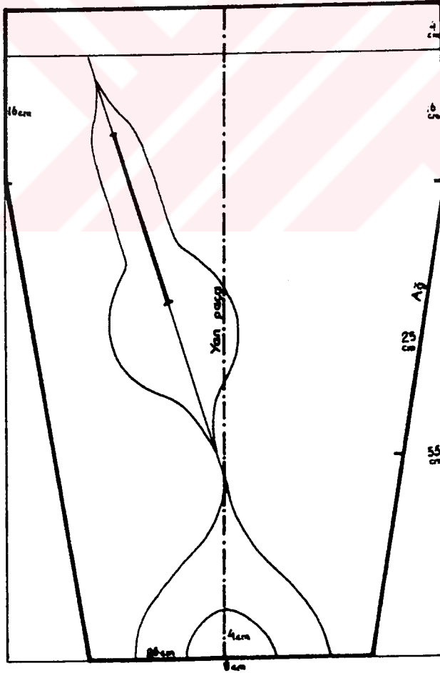
ÇİZİM 57c ÇOCUK YELEĞİ VE ŞALVARI KALIP ÇİZİMİ
