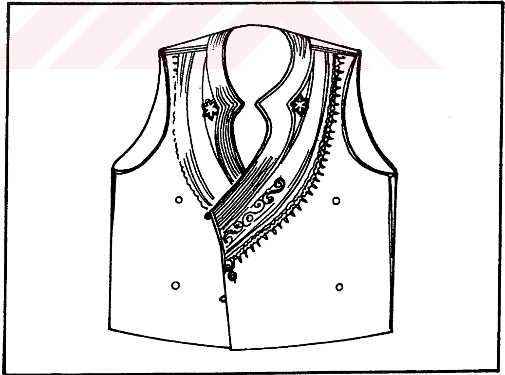
ÇİZİM 57a ÇOCUK YELEĐİ TEKNİK ÇİZİMİ
