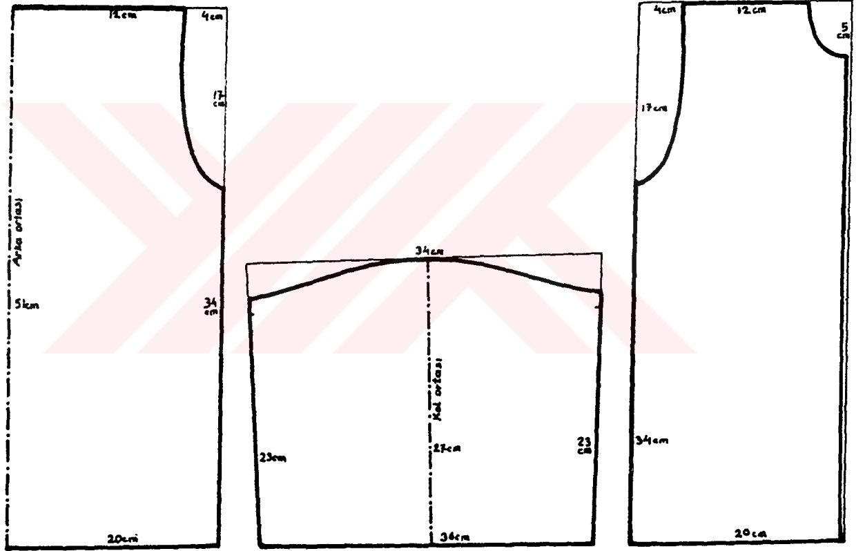
ÇİZİM 50d ÇOCUK GÖMLEĞİ KALIP ÇİZİMİ
