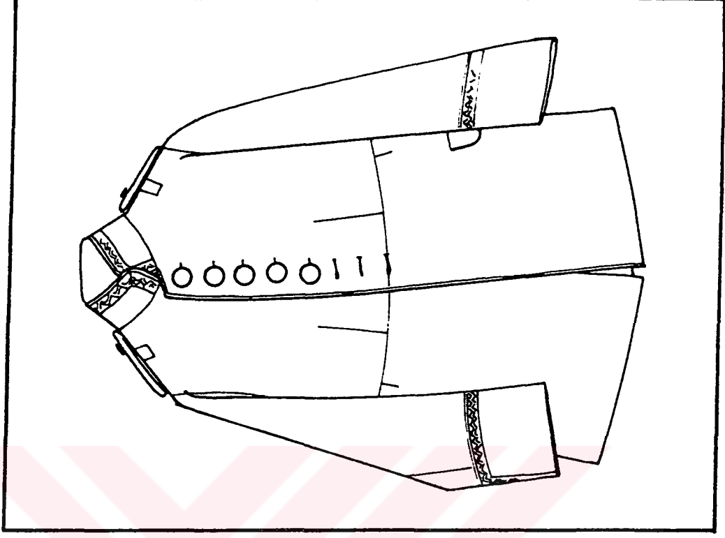
ÇİZİM 44a ÇOCUK CEKETİ TEKNİK ÇİZİMİ
