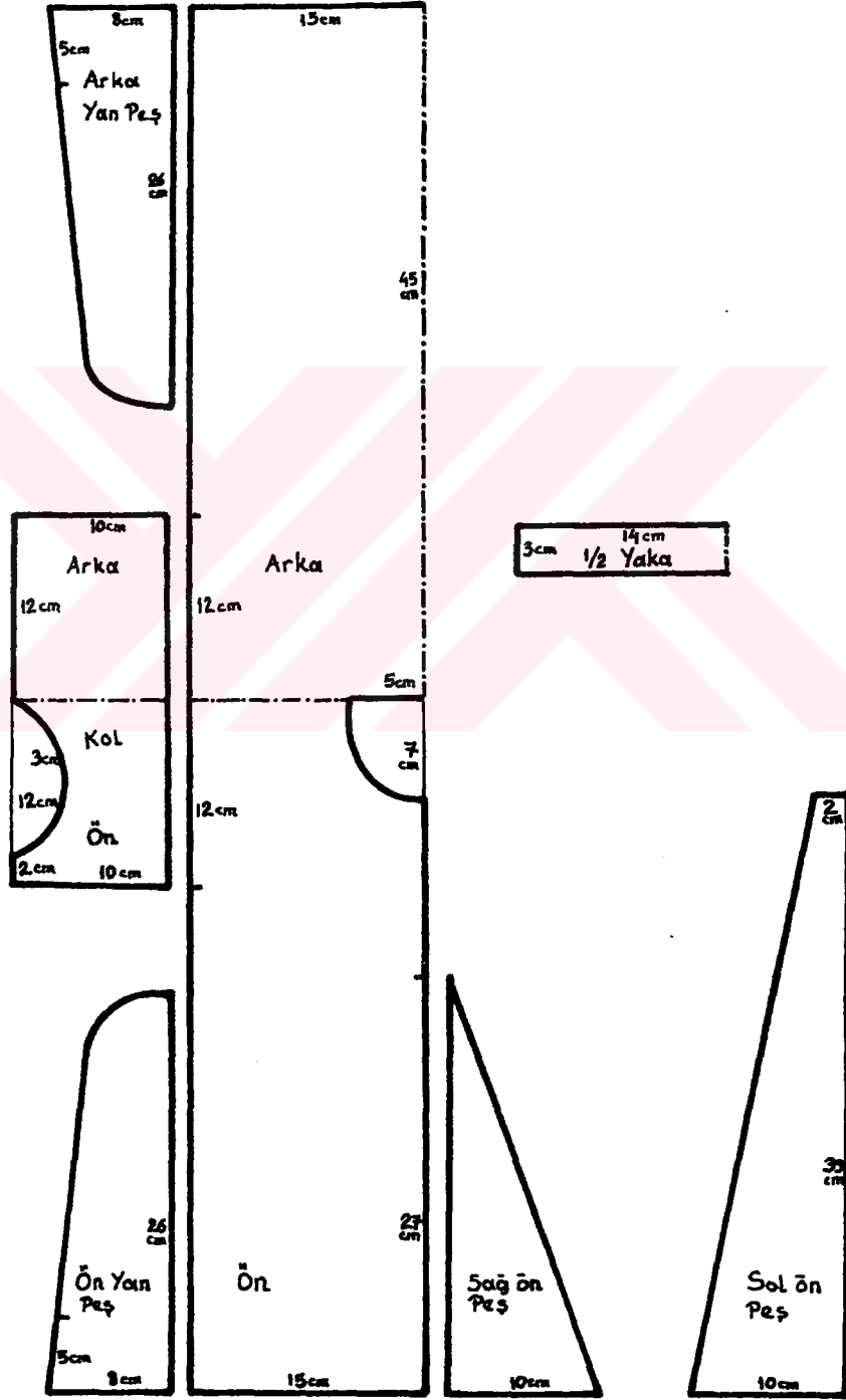
ÇİZİM 40 ÇOCUK ENTARİSİ KALIP ÇİZİMİ
