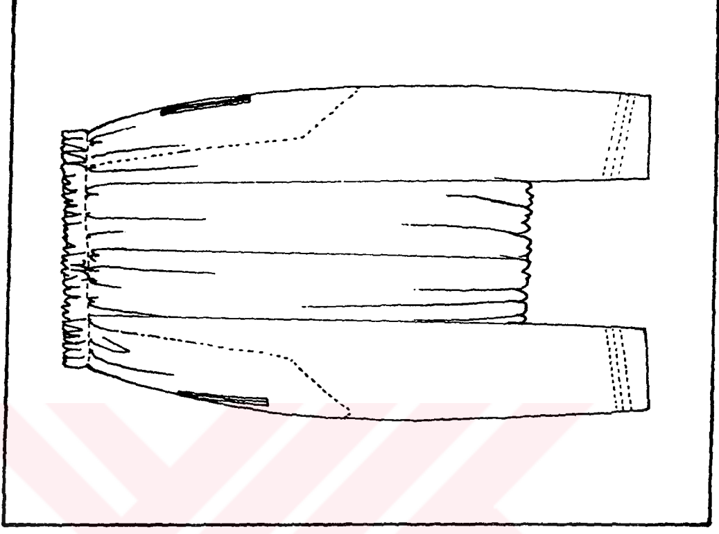
ÇİZİM 50c ÇOCUK ŞALVARI TEKNİK ÇİZİMİ
