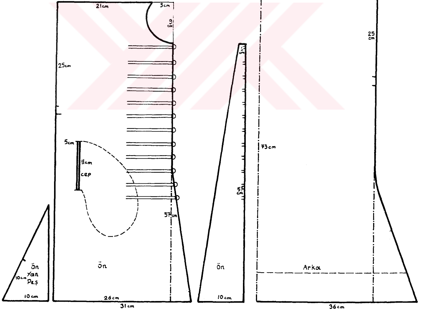
ÇİZİM 10b ÇOCUK KAFTANI KALIP ÇİZİMİ
