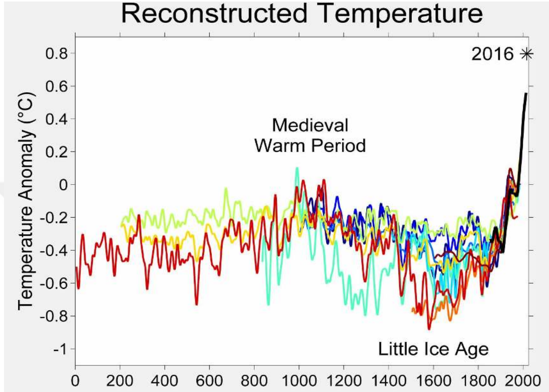
řekil 3.6 Sıcaklık anomalilerin rekontrüksiyonu
