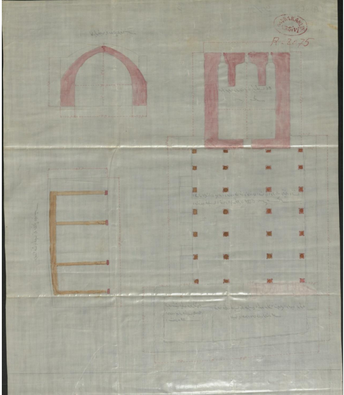
Resim 8. Nurşin köyünde tamiri yapılacak kilise ve kilise bitişiğinde yapılacak olan Katolik Ermeni Milleti'ne ait mektebin krokisi
