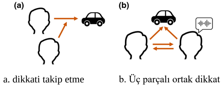
Şekil 2.2 Ortak dikkat ve işlemlenin eşzamanlılığı
