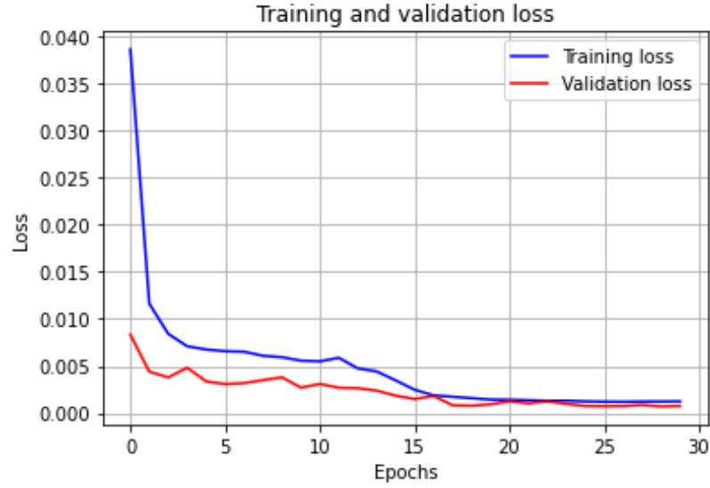
Şekil 4.6. Kayıp fonksiyonuna dayalı eğitim sonuçları
