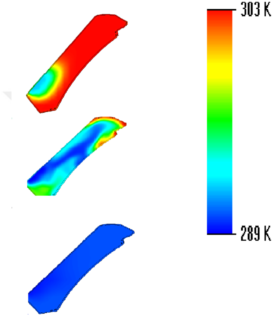
Şekil 4.2. Yakıt tipli otobüslerde hava kanalının yan görünüşü sıcaklık dağılımı
