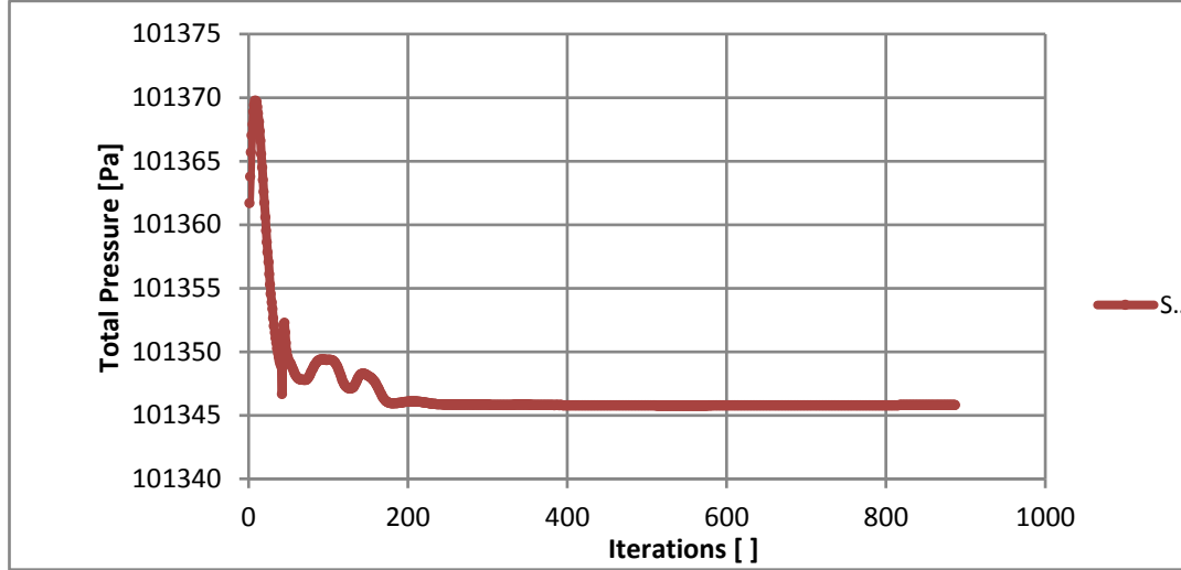
Grafik 4.21. Elektrikli otobüsün hava kanalının otobüs ortasındaki çıkışında oluşan basınç dağılımı
