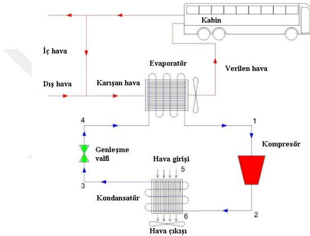
Şekil 2.1. ICBAC sistemin şematik görünümü (Ediz Çardak 2017)
