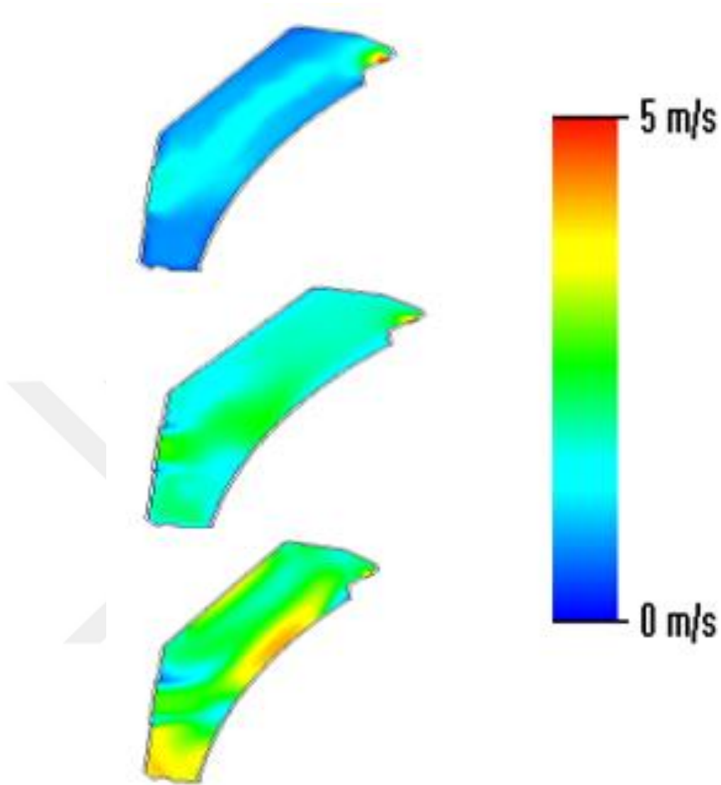
Şekil 4.8. Elektrikli otobüslerde hava kanalının yan görünüşü hız dağılımı
