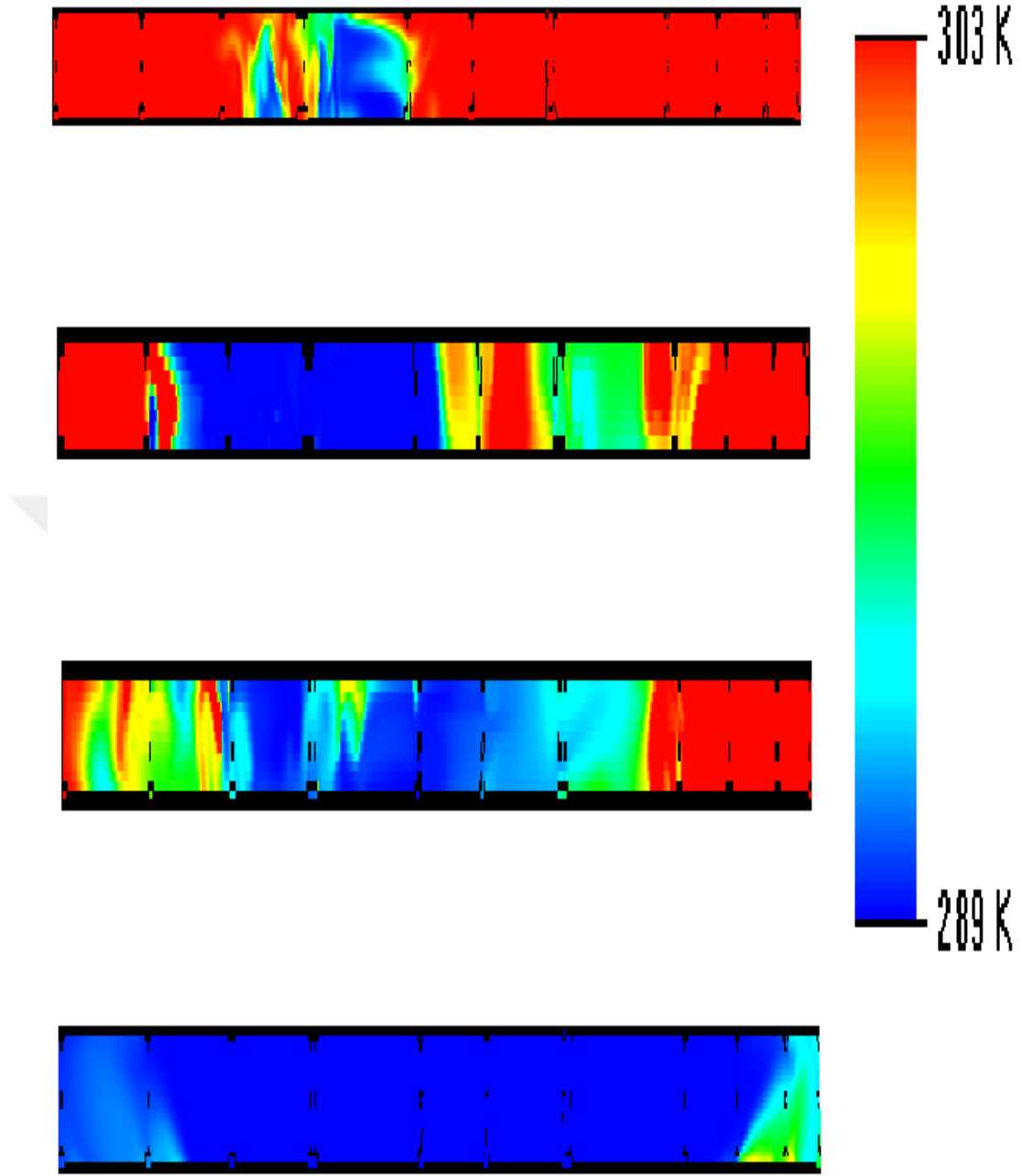
Şekil 4.3. Elektrikli otobüslerde hava kanalı arka görünüş sıcaklık dağılımı
