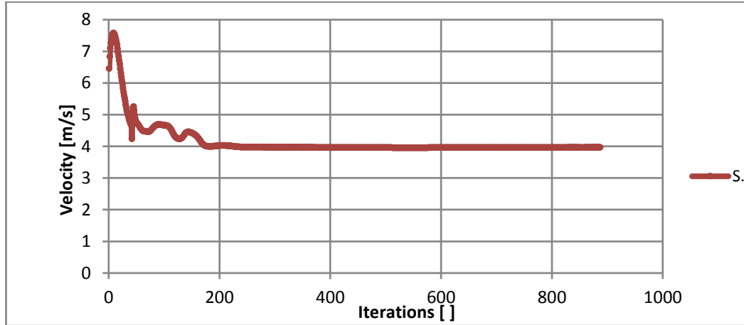
Grafik 4. 13. Elektrikli otobüsün hava kanalının otobüs orta tarafındaki çıkış hızı
