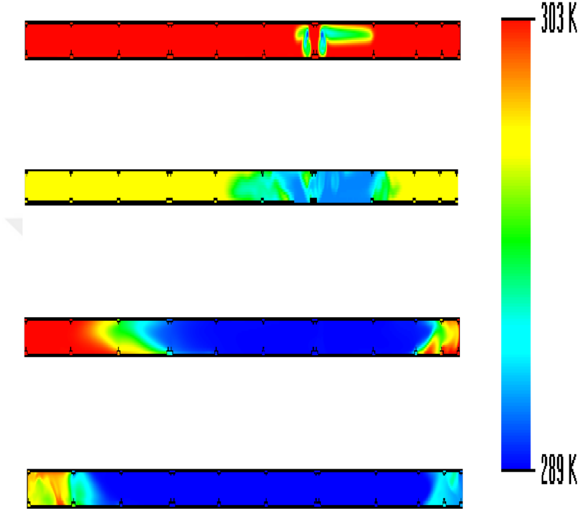
Şekil 4.1. Yakıt tipli otobüslerde hava kanalı arka görünüşü sıcaklık dağılımı
