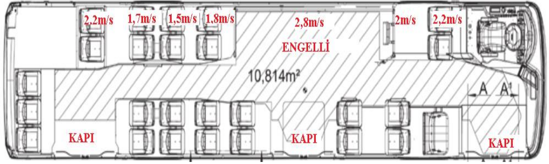
Şekil 5.2. 24 °C sıcaklıkta yolcu bölgesi üzerindeki hava çıkış hızı
