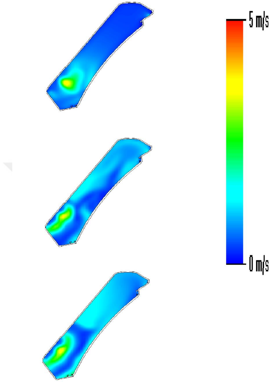
Şekil 4.6. Yakıt Tipli otobüslerde hava kanalının yan görünüşü hız dağılımı
