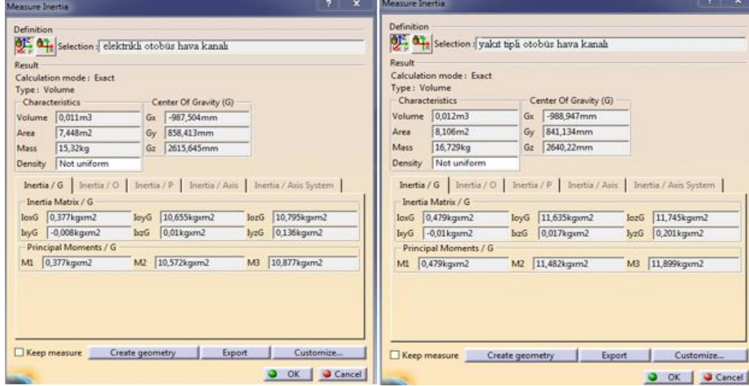
Şekil 4.10. Hava kanallarının kütle karşılaştırılması
