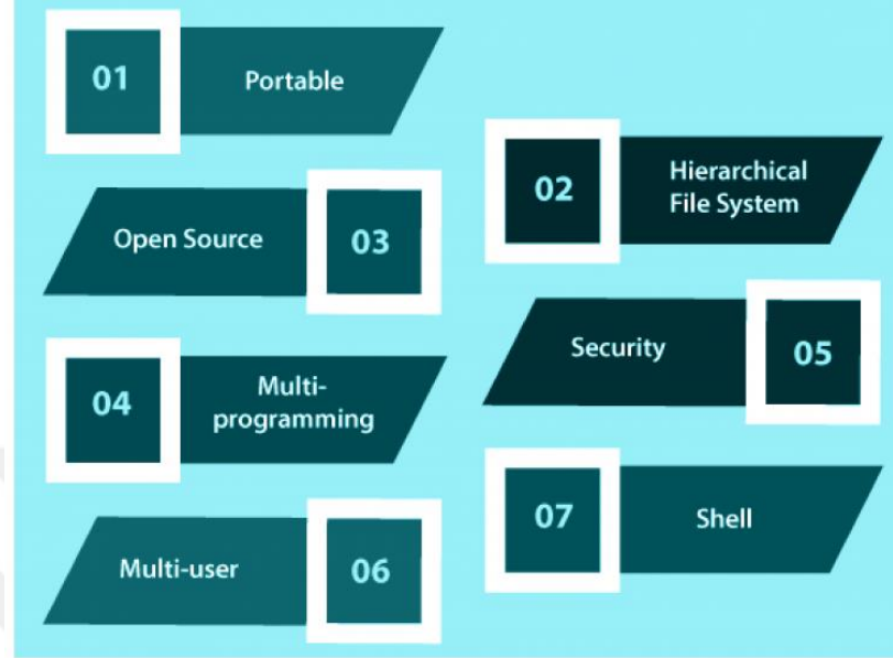
Şekil 3.11. Linux'ün özellikleri [43]
