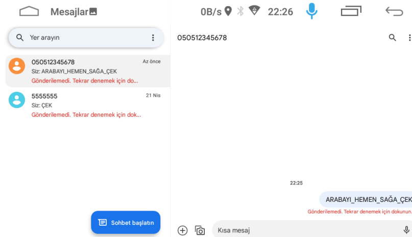
Şekil 4.13. Gelen mesajlar
