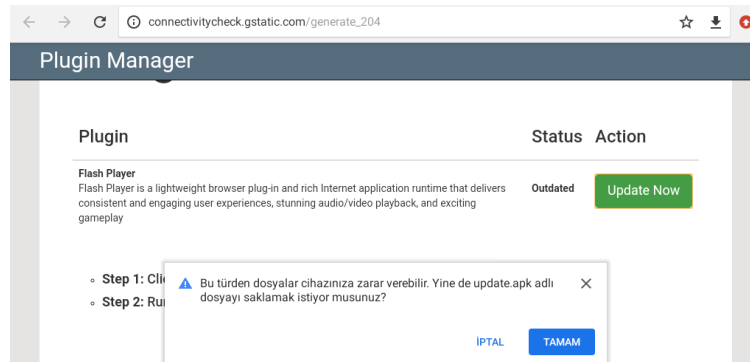
Şekil 4.7. Sistem uyarısı
