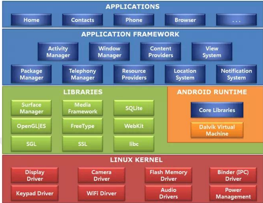
Şekil 3.2. Android katmanları [34]
