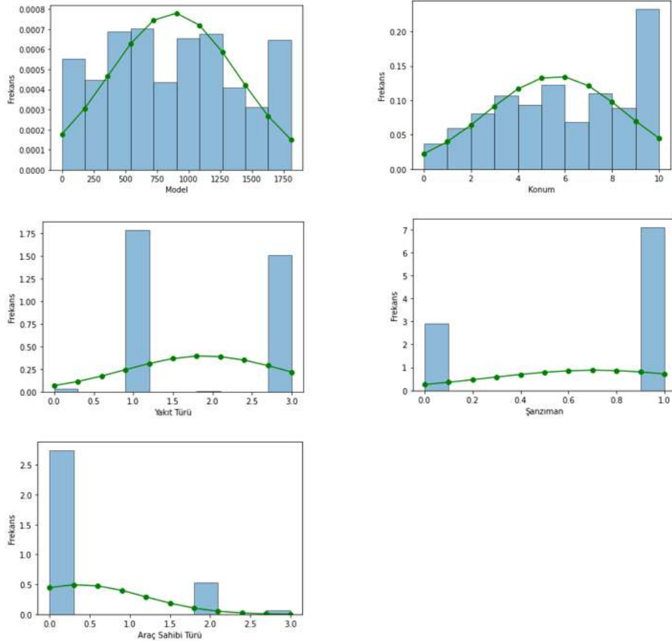
Şekil 3.2 Sayısal olmayan değerler içeren özelliklerin histogram grafikleri
