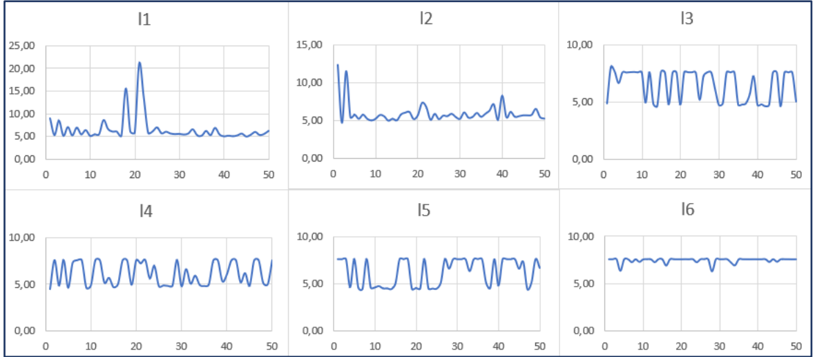
Şekil 3.10 Frekans Kodlama Metodu Uygulanan Veri Setinin YSA Yöntemi Sonucu Nöron Sayısına Göre L1, L2, L3, L4, L5 ve L6 Katmanlarındaki RMSE Değerleri.
