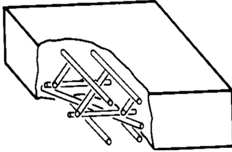
Şekil 1.10 : Rastgele düzlemsel yönlendirilerek takviyelendirilmiş MMK yapısı [11].
