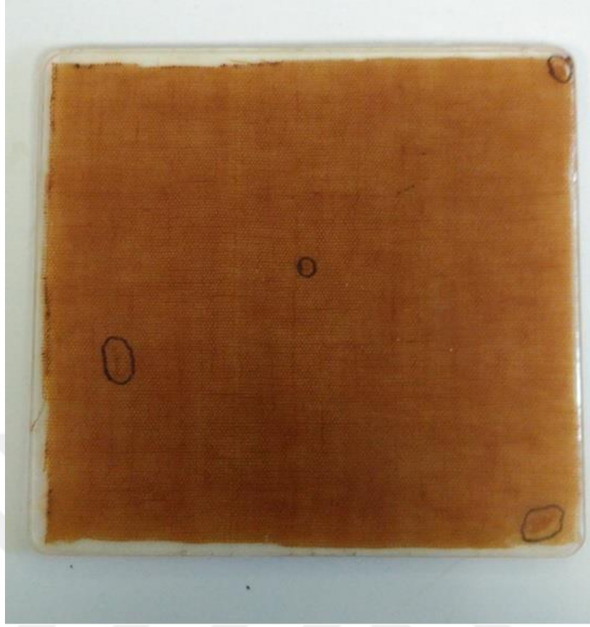
Şekil 3.9 : Keten/PLA kompoziti.
