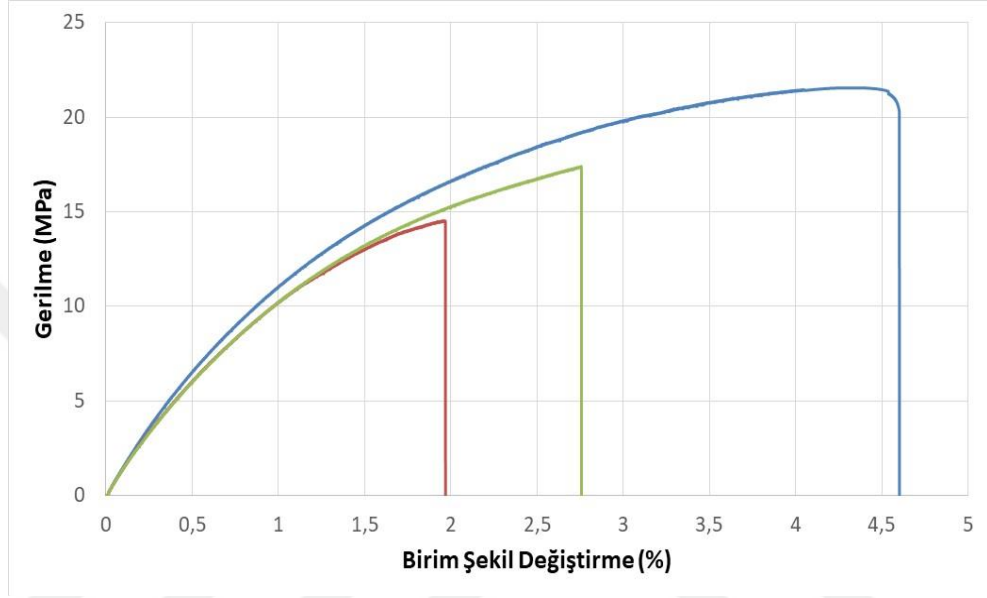
Şekil 5.7 : PP/Jüt kompoziti çekme numuneleri grafiği.
