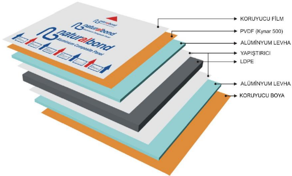
Şekil 1.12 : Tabakalı kompozit [12].
