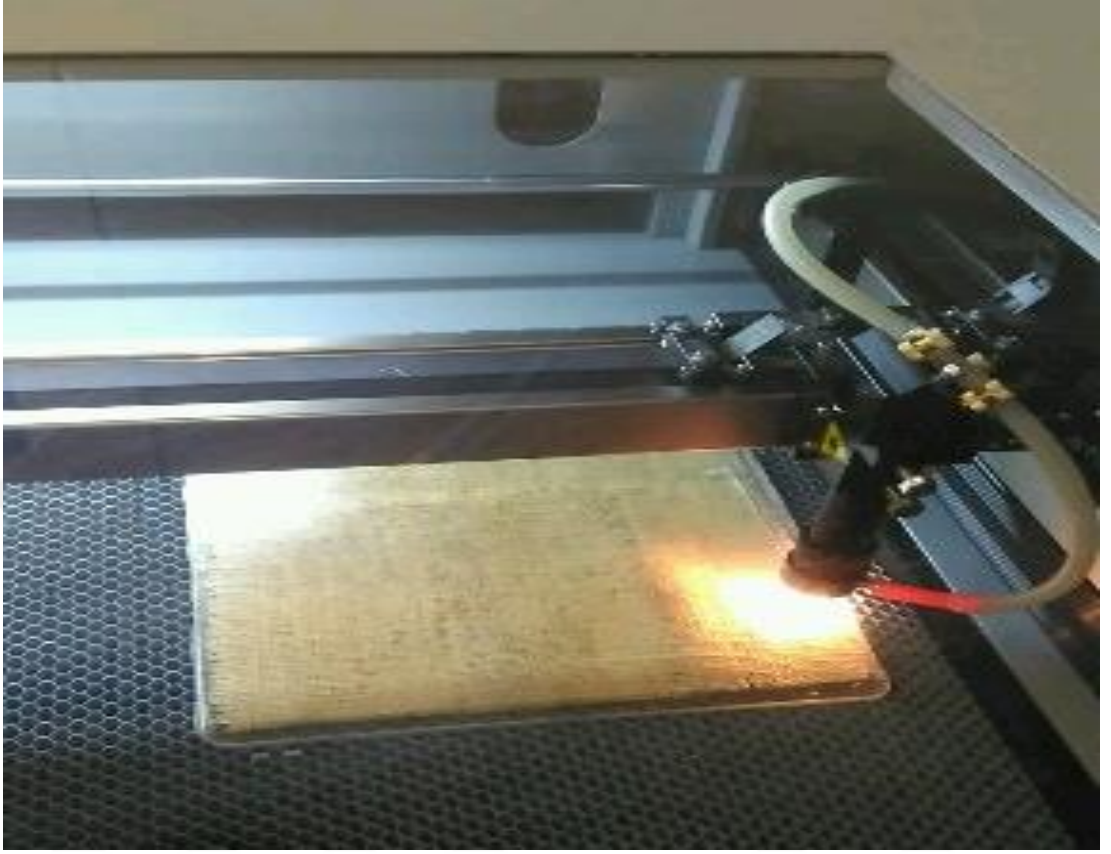
řekil 3.11 : Kare numunenin lazer kesimle hazırlanması.
