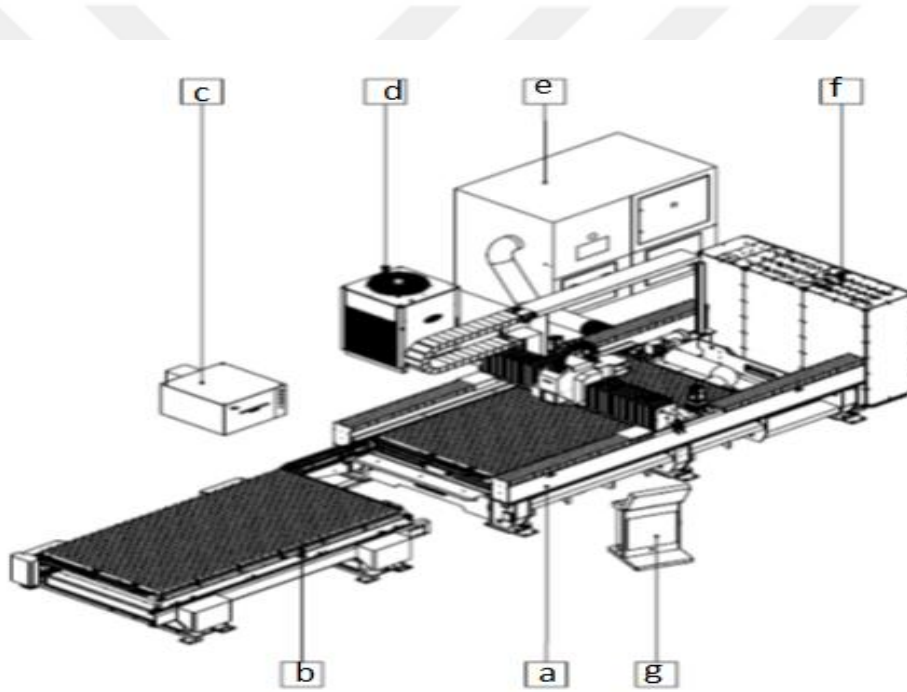
Şekil 2.10 Lazer kesim tezgâhı ana parçaları (Çelenk 2018).
