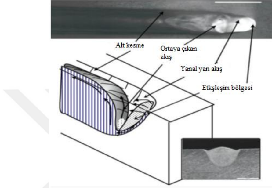
Şekil 2.23 “Ön-tümsek” rejiminin eriyik havuzu akışının taslağı, sonuçta azalmaya neden olur.
