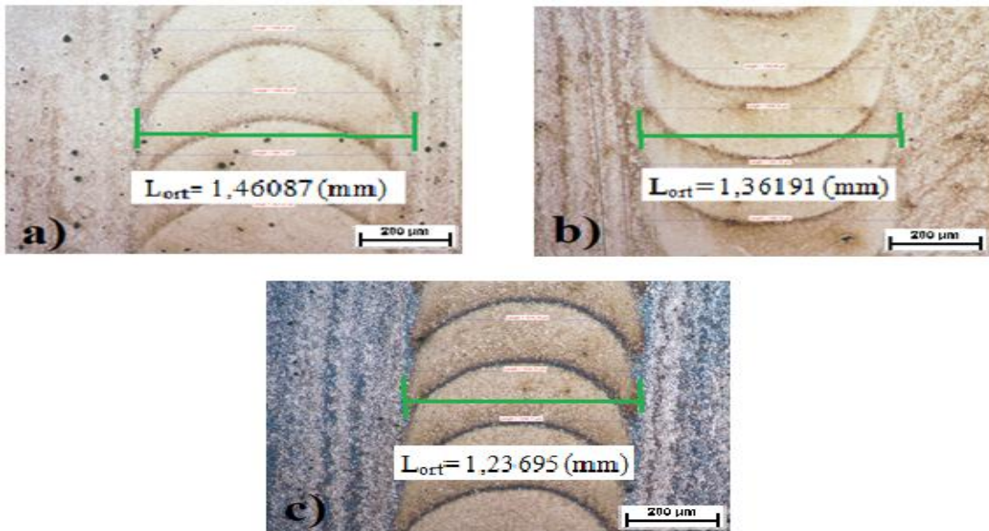
Şekil 4.4 DP 600 çeliği numunelerinde lazer gücü parametresinin kaynak dikişine etkisi; a) Yüksek, b) Orta, c) Düşük.
