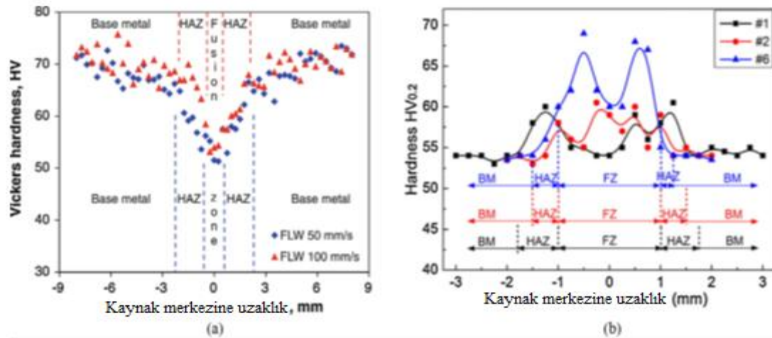
Şekil 2.18 Mikro sertlik profili (a) Fiber lazerle kaynaklı AZ31B-H24 alın derzleri P = 2 \text{ kW} , V = 3, 6 \text{ m / dak} (Chowdhury ve ark. (2012), © Springer 2012). (b) Fiber lazer kaynaklı ekstrüde edilmiş AZ31 alın derzleri # 1: P = 2,0 \text{ kW} , V = 1,4 \text{ m / dak} , # 2 P = 2,5 \text{ kW} , V = 2,4 \text{ m / dak} , # 6 P = 6,0 \text{ kW} , V = 7,8 \text{ m / dak} (Hong and Shin 2016).
