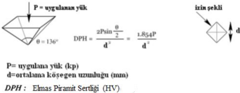
Şekil 3.1 Vickers sertlik testi geometrik hesabının formülize edilmesi.
