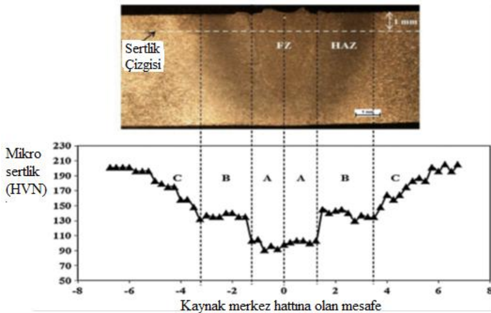
Şekil 2.16 AA7075-T561'in mikro sertlik profilleri ( P = 3,5 \text{ kW} , V = 0,6 \text{ m / dak} ) (Hong and Shin 2016).
