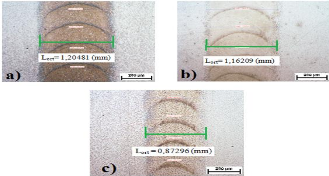
Şekil 4.2 St 6222 çeliği numunelerinde lazer gücü parametresinin kaynak dikişine etkisi; a) Yüksek, b) Orta, c) Düşük.
