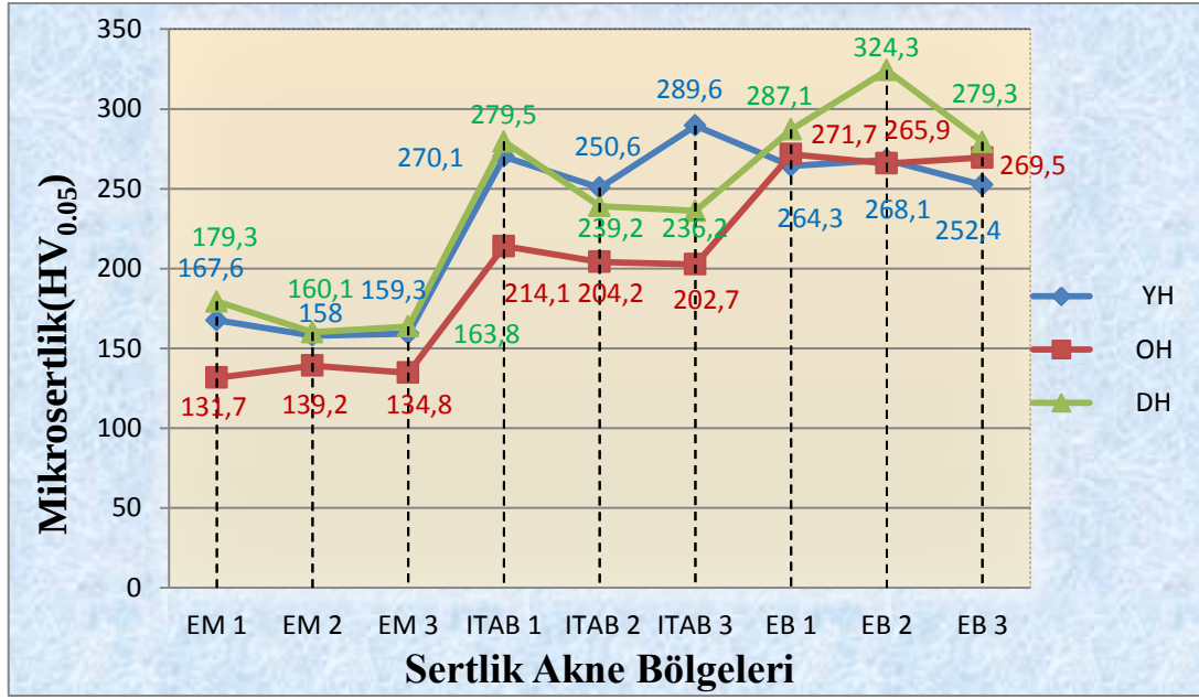
Şekil 4. 10 Hız parametresinin mikrosertliğe etkisi; St 6222 çeliği numuneleri.
