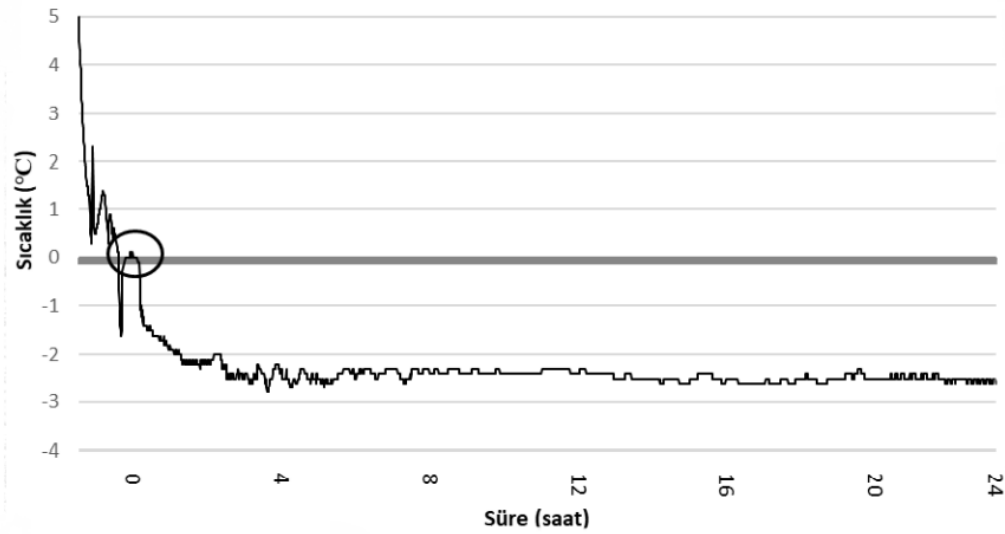
Şekil 3.5: Donma sırasında datalogger verilerinin kayıtlarına ait bir örnek. İşaretli bölge ekzotermik noktasının gerçekleştiğini göstermekte ve yaklaşık 90. dakikaya denk gelir.
