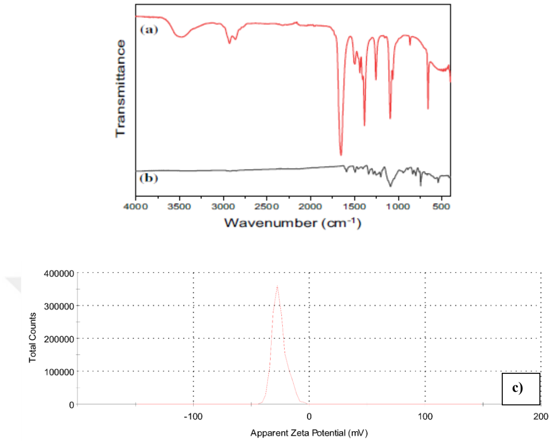
Şekil 4.4. (a) Hazırlanan \beta borofenin (b) CuPc-borofen FTIR görüntüsü (c) hazırlanan \beta borofenin Zeta potansiyel profili.
