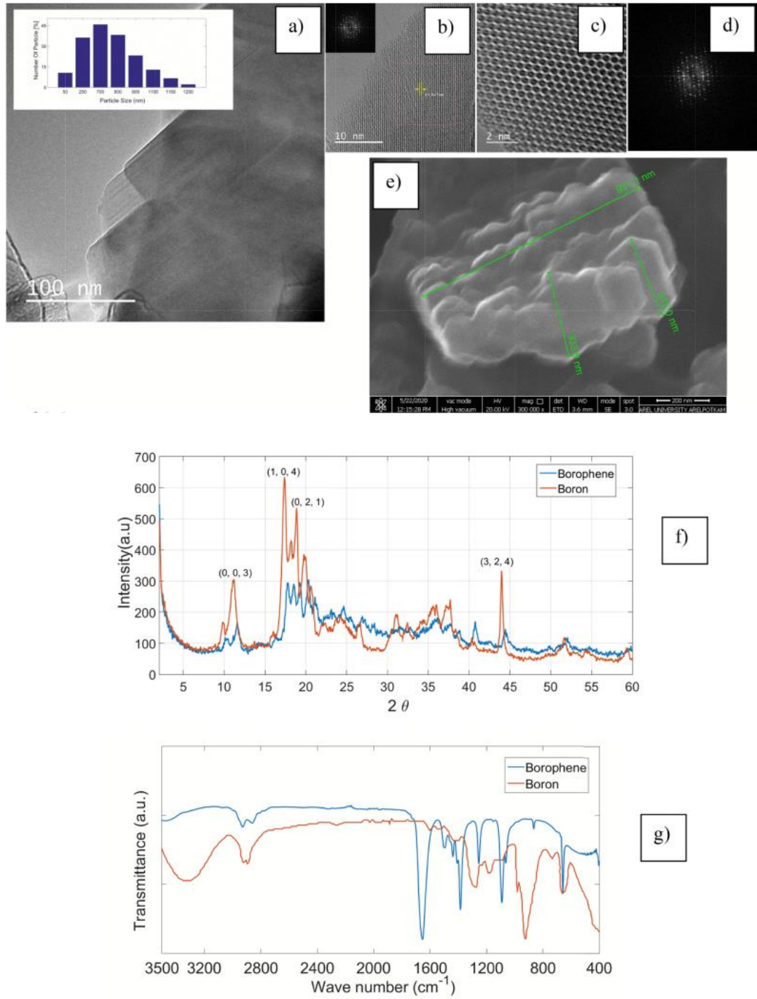
Şekil 5.1. (a-d) HRTEM histogram sonucu ile borofen nano tabakaların TEM görüntüleri, (e) Borofen nano tabakaların SEM görüntüsü, (f) bor ve borofen nano tabakaların XRD desenleri ve (g) bor ve borofen nano tabakaların FTIR spektrumları.
