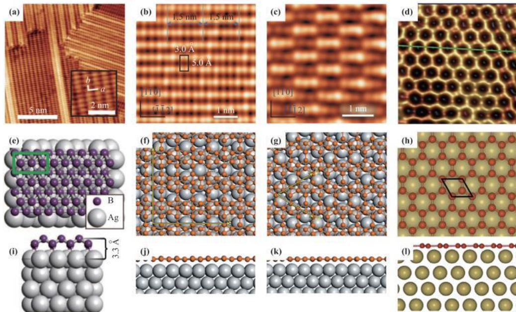
Şekil 2.4. STM (Tarama tünel mikroskopu) topografya görüntüleri (a–d), yukarıdan bakış (e–h) ve yandan bakış (i–l) Ag/Al(III) alttabanda 2-Pmmn, \beta 12, \alpha 3 ve grafen benzeri fazlarını için [114].
