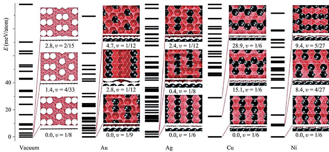
Şekil 2.5. Au, Ag, Cu ve Ni altabaları ile desteklenen borofenlerin enerji spektrumları [114].
