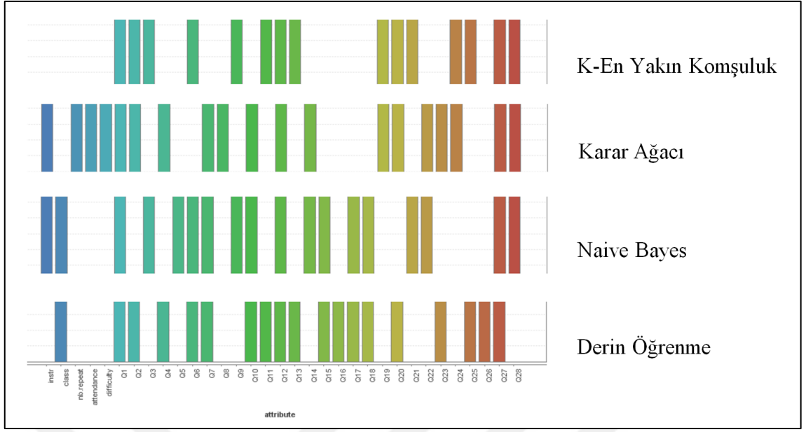
Şekil 6.1 Dört Farklı Makine Öğrenmesi yöntemi için GA tarafından seçilen öznitelikler
