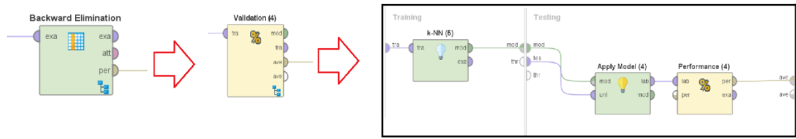
Şekil 5.7 GYE Modülü ve alt prosesleri
