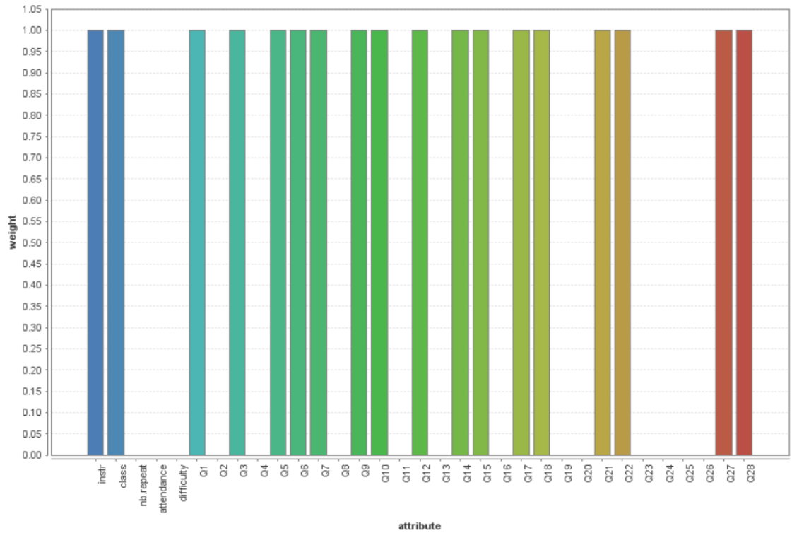
Şekil 5.15 Naive Bayes Algoritması Kullanımı Öncesinde Seçilen Öznitelikler
