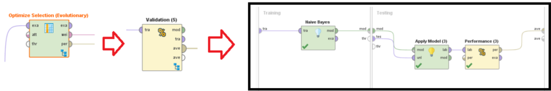
Şekil 5.14 Naive Bayes Algoritması ile Tahmin Yapılması
