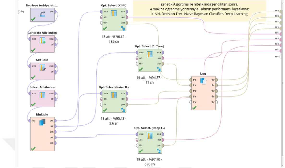
Şekil 5.9 Çeşitli Makine Öğrenmesi yöntemleri ile tahmin yapılması
