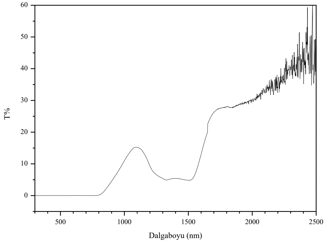
Şekil 7.4. FTO/ p-Co 3 O 4 / n-In 2 O 3 yapıya ait geçirgenlik spektrumu
