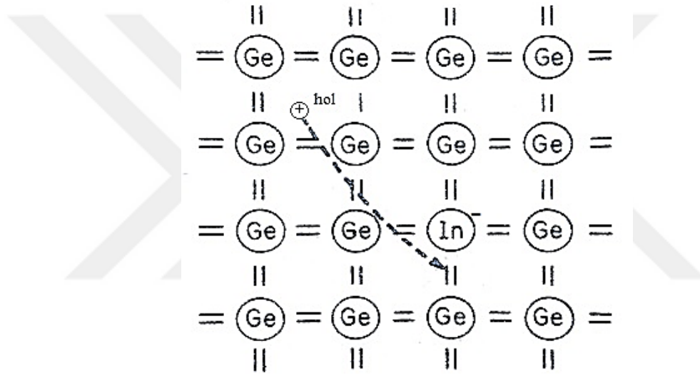
Şekil 2.6. Ge kristaline In atomu katkılanması (McKelvey, 1966).
