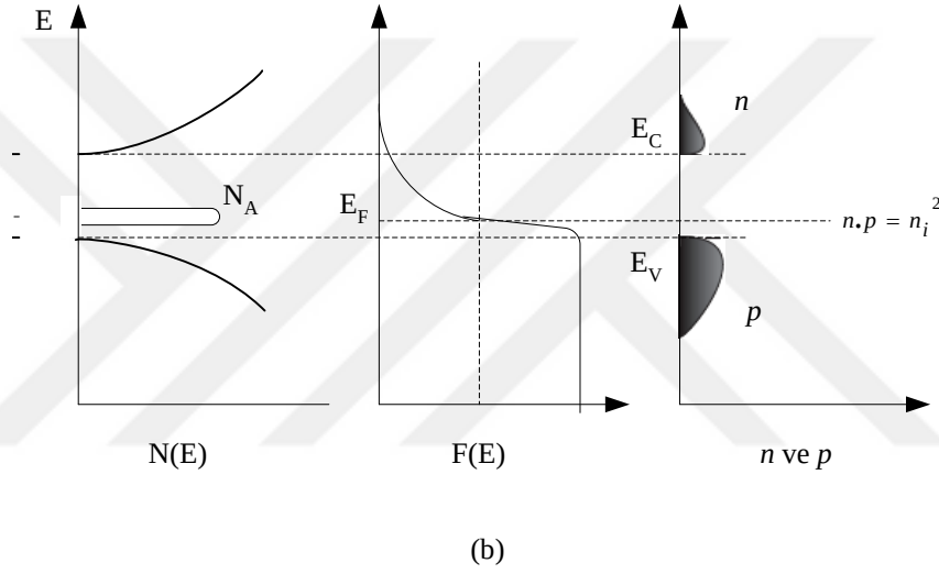
Şekil 2.10. Isıl dengede (a) n-tipi ve (b) p-tipi yarıiletkenler için sırasıyla durum yoğunluğu, Fermi-Dirac dağılımı ve serbest taşıyıcı yoğunluğu (Sze ve Kwok, 2007)
