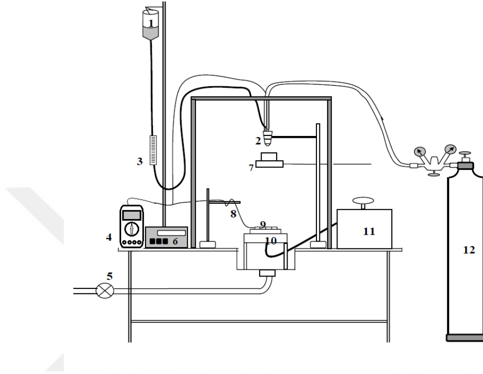
Şekil 5.21. Ultrasonik püskürtme deney seti (Turan, 2007)
