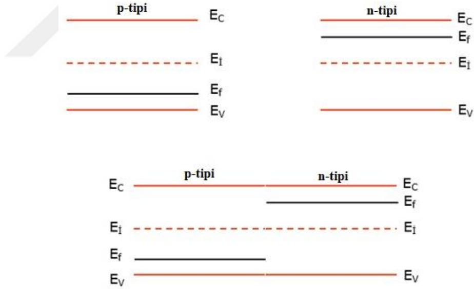
Şekil 6.1. p-tipi bir yarıiletkenin n-tipi bir yarıiletken ile bir araya getirilmesinin şematik gösterimi
