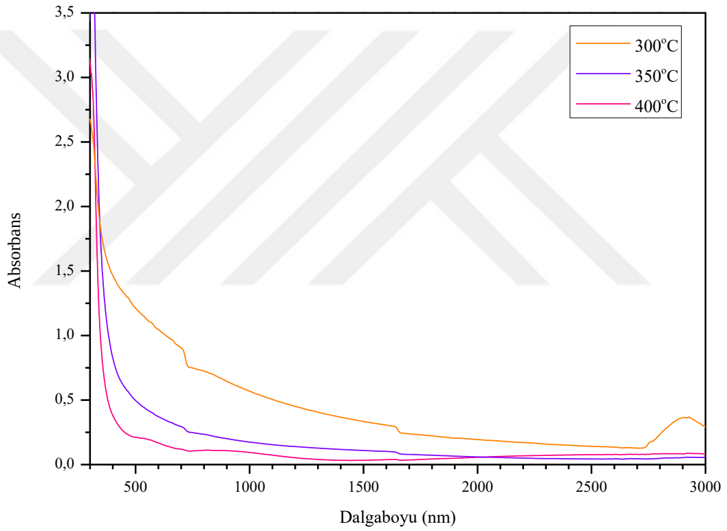
Şekil 5.35. Ultrasonik püskürtme yöntemiyle cam taban üzerine elde edilen \text{In}_2\text{O}_3 filmlerinin absorbans spektrumları
