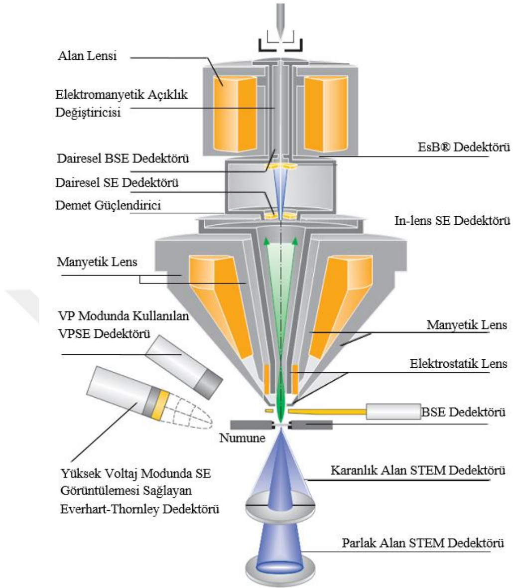
Şekil 3.4. Zeiss Ultra Plus FESEM cihazının iç yapısı (Carl Zeiss Microscopy, 2004)
