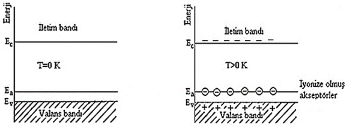
Şekil 2.7. p-tipi bir yarıiletkenin (a) mutlak sıcaklıkta (0 K) ve (b) T > 0 K'de enerji bant diyagramı (Neamen, 1997)
