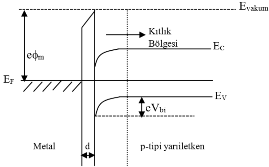
Şekil 4.4. \phi_m < \phi_s durumunda metal-yarıiletken kontak oluştuktan sonra bant yapısı (Bar-Lev, 1984)
