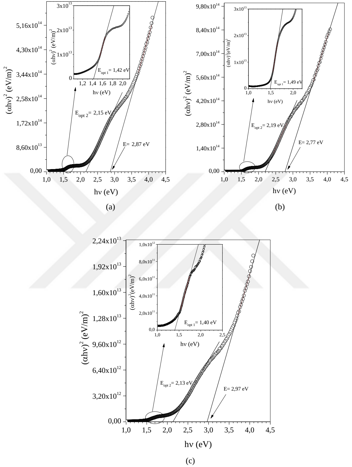
Şekil 5.11. KBD yöntemiyle 65^\circ\text{C} banyo sıcaklığında (a) 4 (b) 6 ve (c) 8 saat depolama sürelerinde elde edilen tavlanmış \text{Co}_3\text{O}_4 filmlerinin optik bant aralıkları
