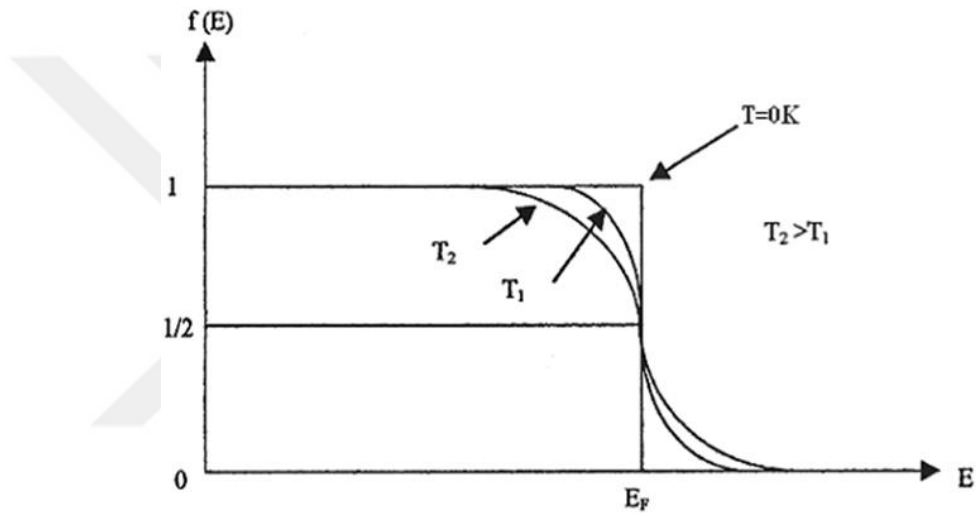
Şekil 2.3. Fermi-Dirac dağılımının iki farklı sıcaklık için şematik gösterimi (Neamen, 1997)
