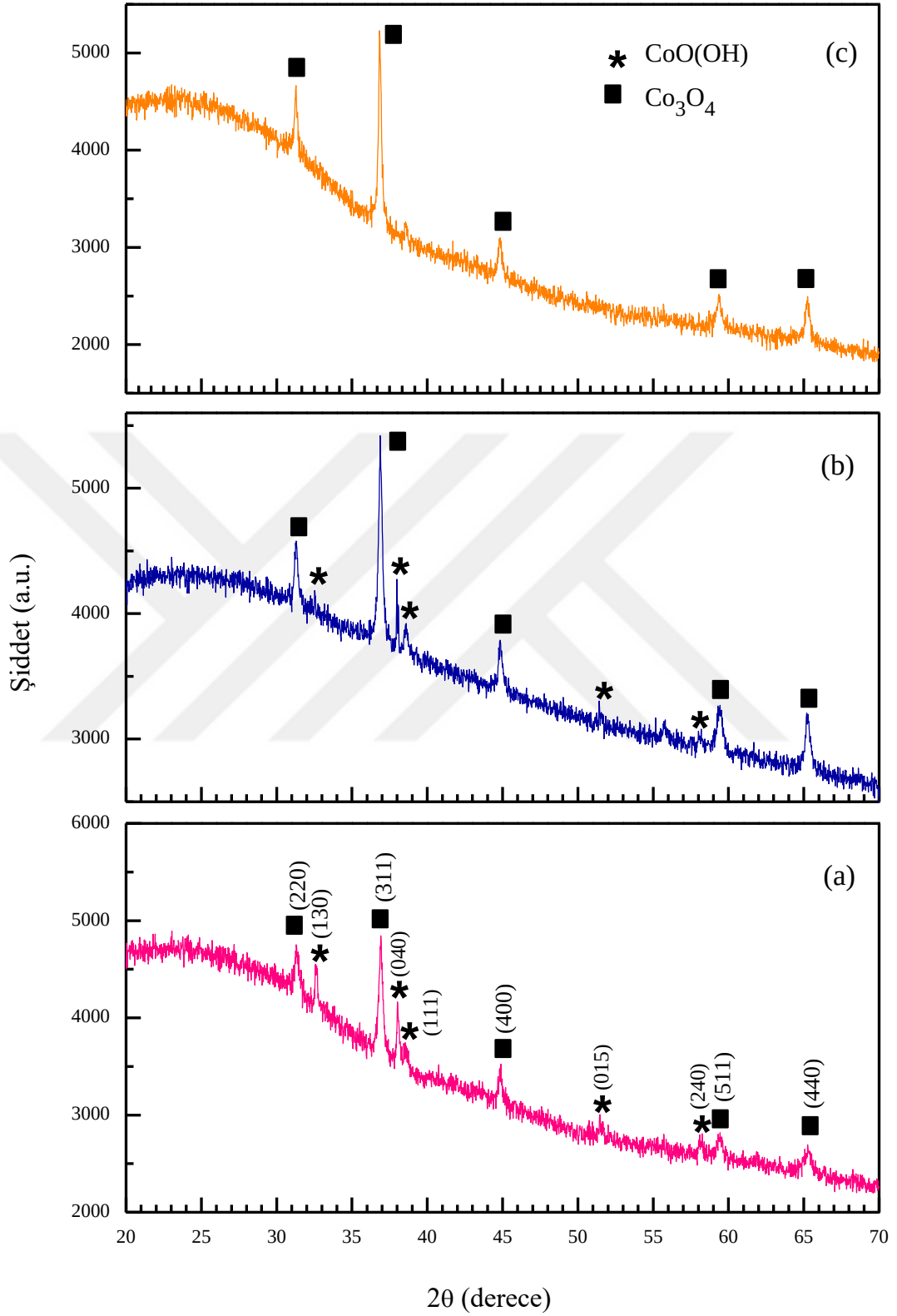
Şekil 5.4. KBD yöntemiyle 95^\circ\text{C} banyo sıcaklığında (a) 4, (b) 6 ve (c) 8 saat depolama sürelerinde üretilen tavlınmamış numunelere ait XRD desenleri
