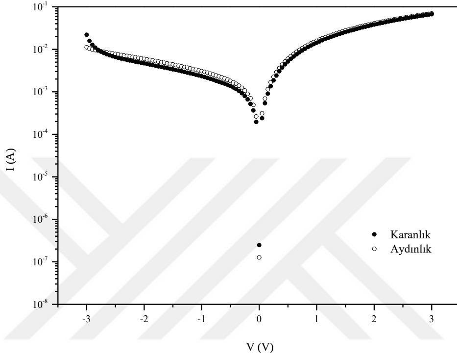
Şekil 7.10. FTO/ p\text{-Co}_3\text{O}_4 / n\text{-In}_2\text{O}_3 heteroeklem yapının karanlıkta ve aydınlıkta yarı logaritmik I - V grafiği
