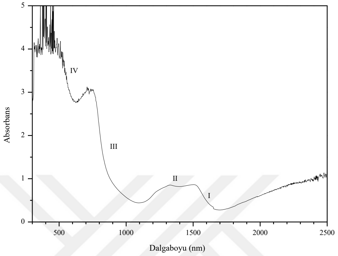
Şekil 7.3. FTO/ p-Co 3 O 4 / n-In 2 O 3 yapıya ait absorban spektrumu
