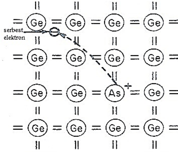
Şekil 2.8. Ge kristaline As atomu katkılanması (McKelvey, 1966).
