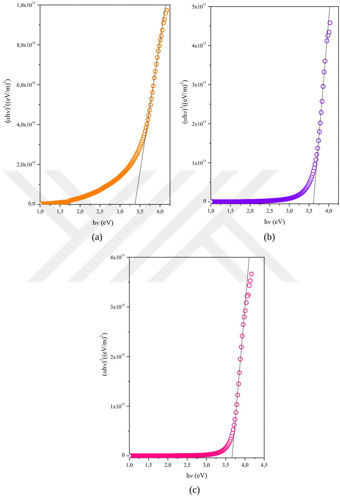
Şekil 5.37. Ultrasonik püskürtme yöntemiyle (a) 300°C, (b) 350°C ve (c) 400°C taban sıcaklıklarında elde edilen \text{In}_2\text{O}_3 filmlerinin (\alpha h\nu)^2 - h\nu grafikleri
