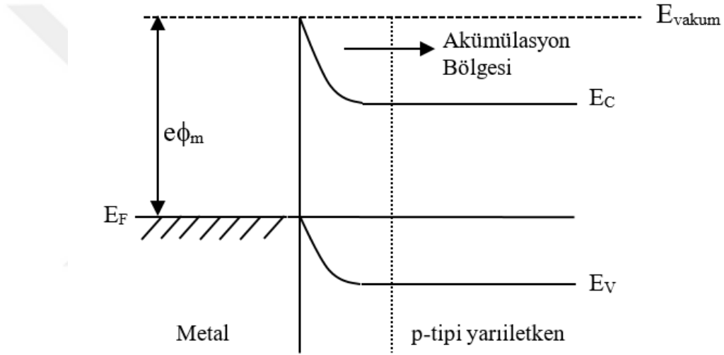
Şekil 4.2. \phi_m > \phi_s durumunda metal- yarıiletken kontak oluştuktan sonra bant yapısı (Bar-Lev, 1984)
