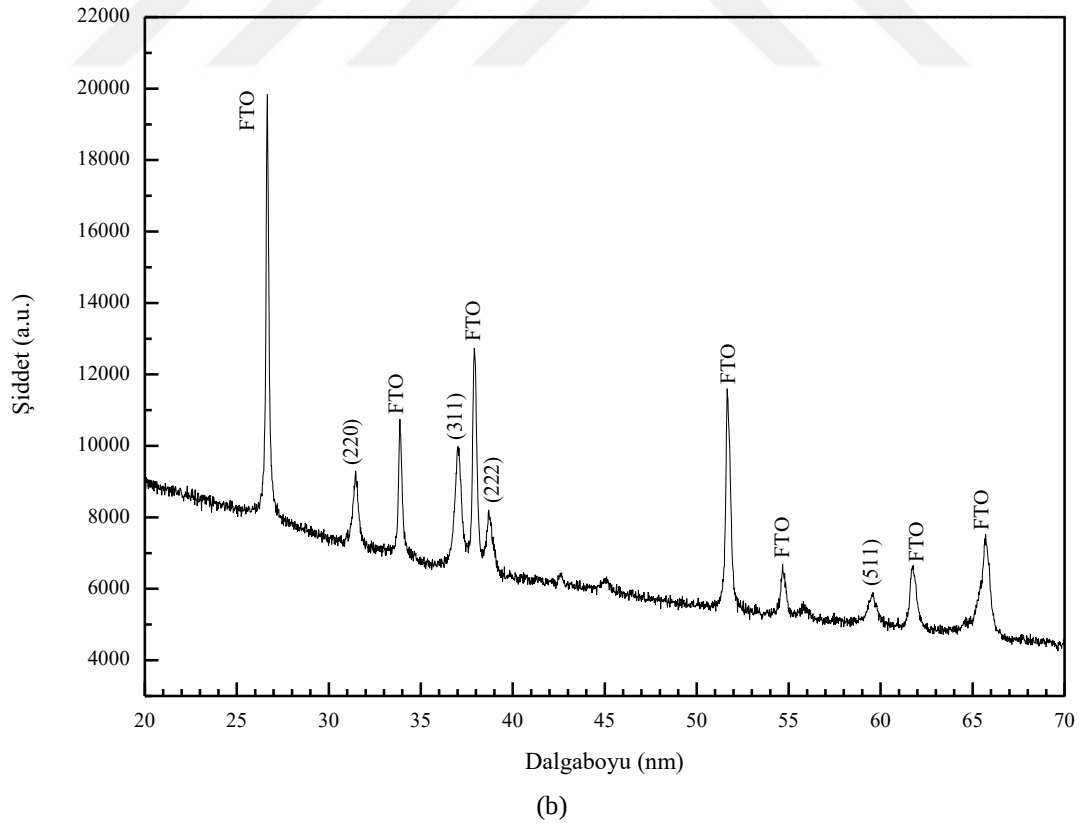
Şekil 5.24. (a) FTO tabana ve (b) FTO/ p-Co 3 O 4 yapıya ait x-ışını kırınım deseni
