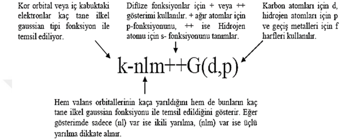
Şekil 3.1. Temel setlerin adlandırılması.
