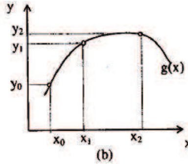
Şekil 2.3. Üç noktadan geçen uydurulmuş eğri
