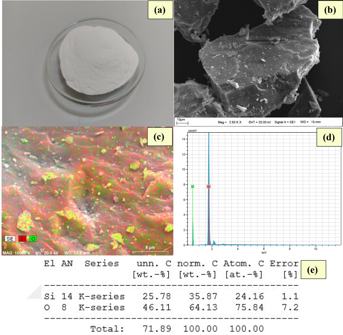
Şekil 3.8. Tez çalışmasında kullanılan kuvars örnekleri (a), bu örneklerle ait SEM görüntüleri ((b), (c)), örneklerin EDX analiz sonuçları ((d), (e))
