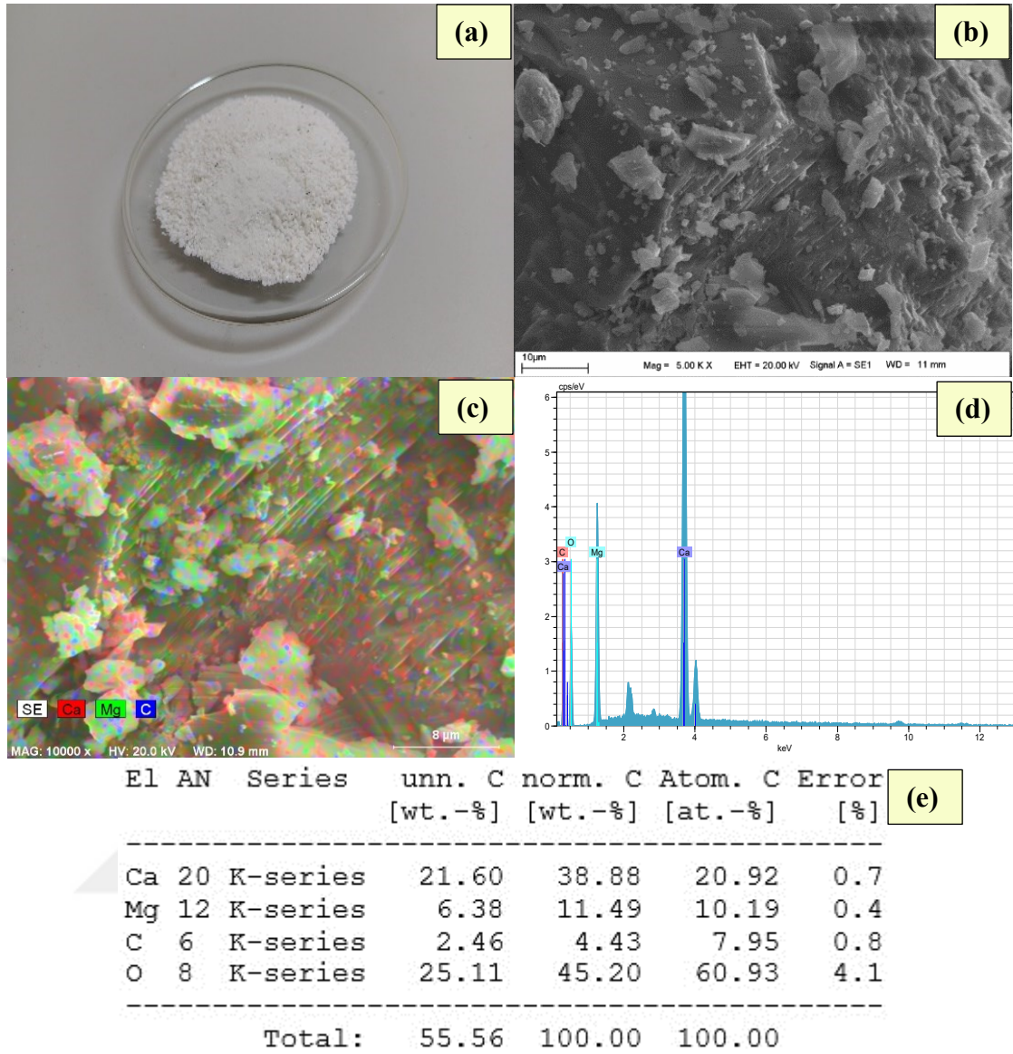
Şekil 3.20. Tez çalışmasında kullanılan dolomit örnekleri (a), bu örneklerle ait SEM görüntüleri ((b), (c)), örneklerin EDX analiz sonuçları ((d), (e))
