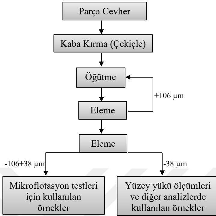
Şekil 3.22. Numune hazırlama akım şeması
