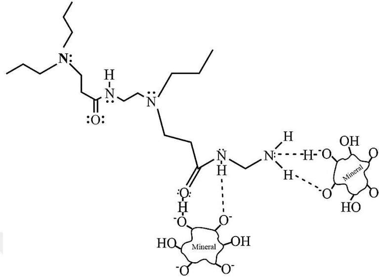
Şekil 2.13. Sentezlenen dendrimerler ve hedef minerallerle planlanan etkileşimi
