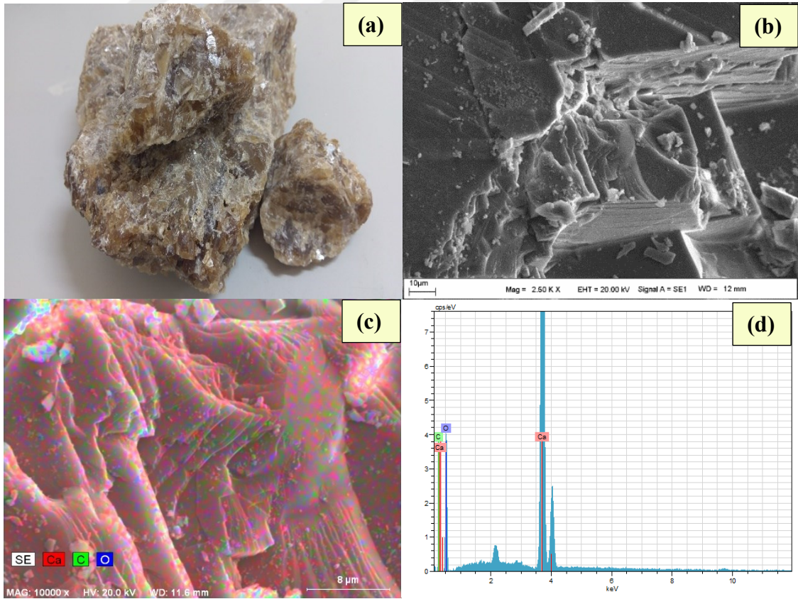
Şekil 3.14. Tez çalışmasında kullanılan kalsit örnekleri (a), bu örnekler için SEM görüntüleri ((b), (c)), örneklerin EDX analiz sonuçları (d)
