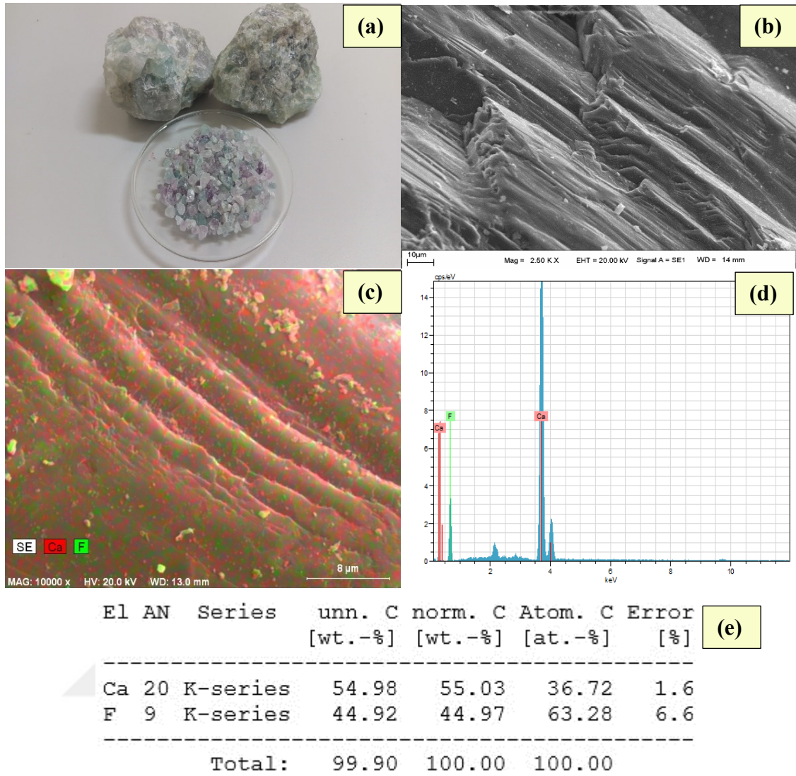
Şekil 3.12. Tez çalışmasında kullanılan florit örnekleri (a), bu örneklerle ait SEM görüntüleri ((b), (c)), örneklerin EDX analiz sonuçları ((d), (e))
