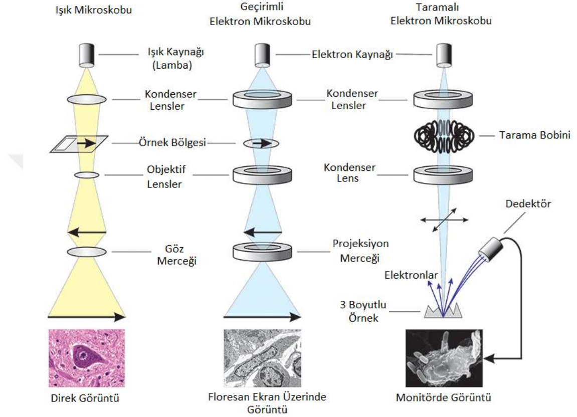
Şekil 2.19. Işık (LM), geçirimli (TEM) ve taramalı (SEM) elektron mikroskobunun karşılaştırmalı şematik gösterimi (İnkson, 2016)
