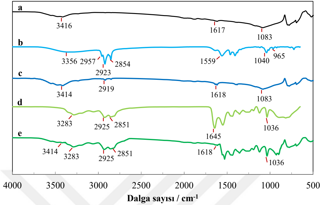
Şekil 4.10. Kuvarsın toplayıcısız (a), Aero3000C (c) ve PAMAM (e) varlığında FTIR spektrumu (Saf Aero3000C (b), Sentezlenen PAMAM (d), pH=8)
