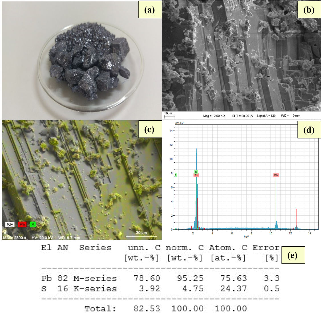
Şekil 3.16. Tez çalışmasında kullanılan galen örnekleri (a), bu örneklerle ait SEM görüntüleri ((b), (c)), örneklerin EDX analiz sonuçları ((d), (e))
