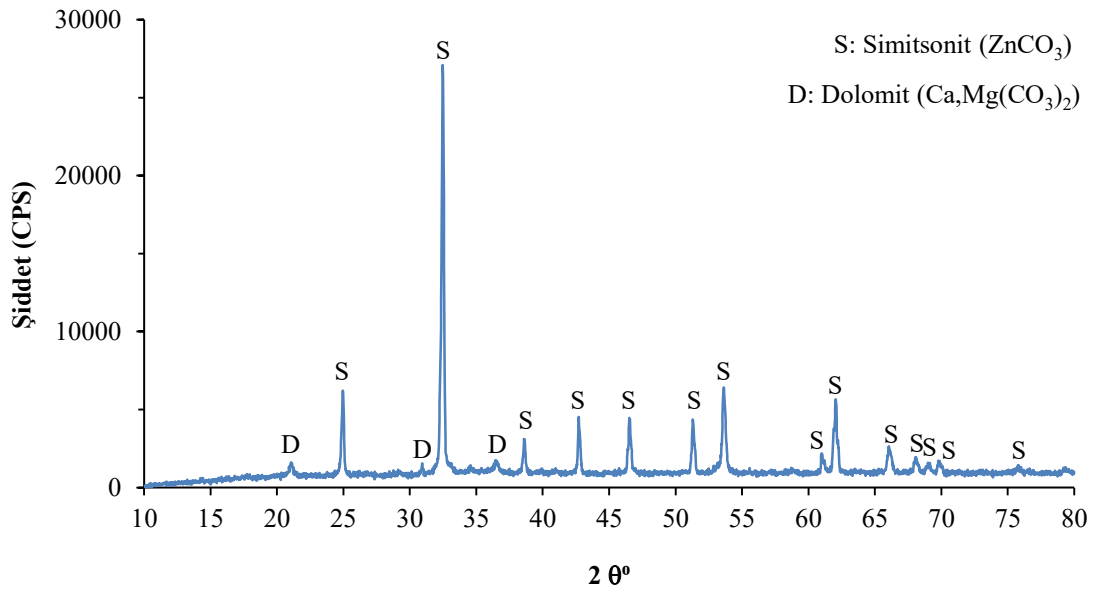
Şekil 3.17. Saf simitsonit mineraline ait XRD deseni
