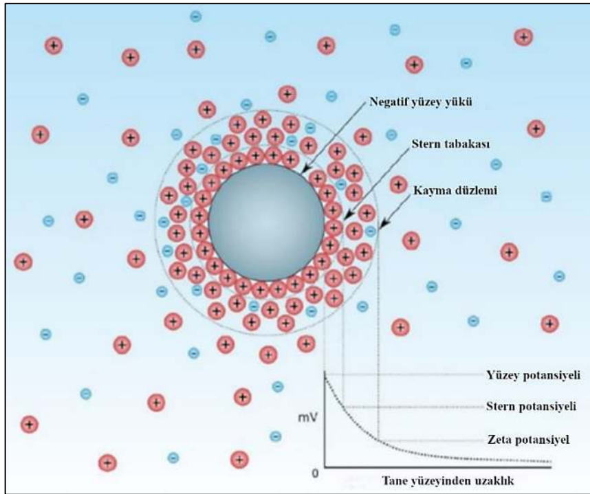
Şekil 2.18. Stern'e göre elektriksel çift tabaka modeli (Pate ve Safier, 2016)
