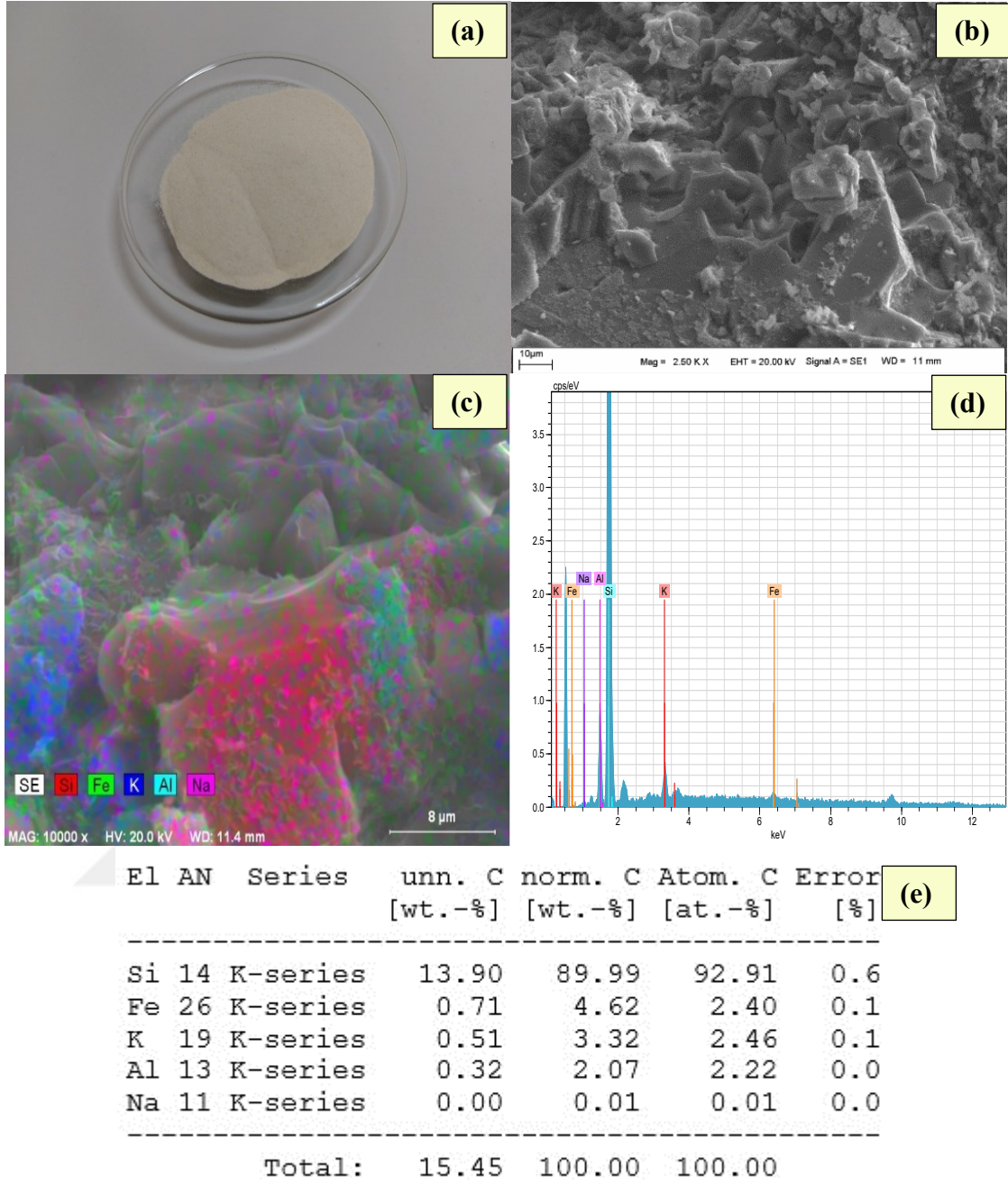
Şekil 3.6. Tez çalışmasında kullanılan feldspat örnekleri (a), bu örneklerle ait SEM görüntüleri ((b), (c)), örneklerin EDX analiz sonuçları ((d), (e))
