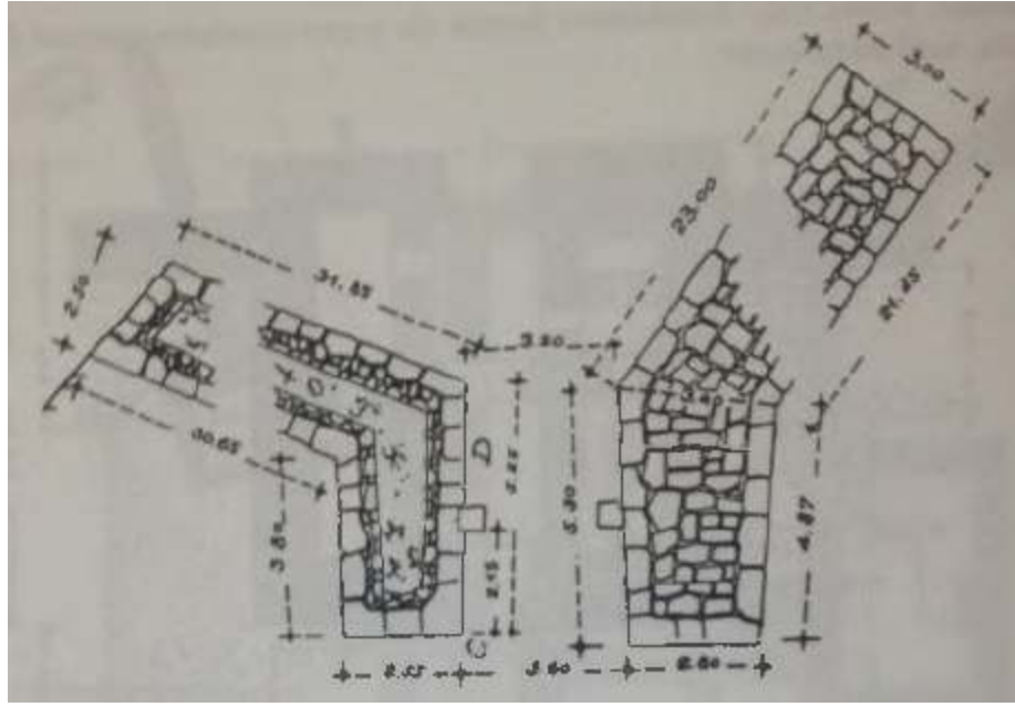
Resim 15: Gortis B Kapısı
