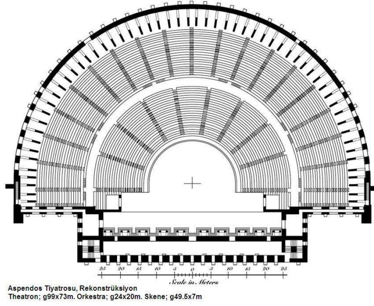
Resim 41: Aspendos Tiyatro Planı
