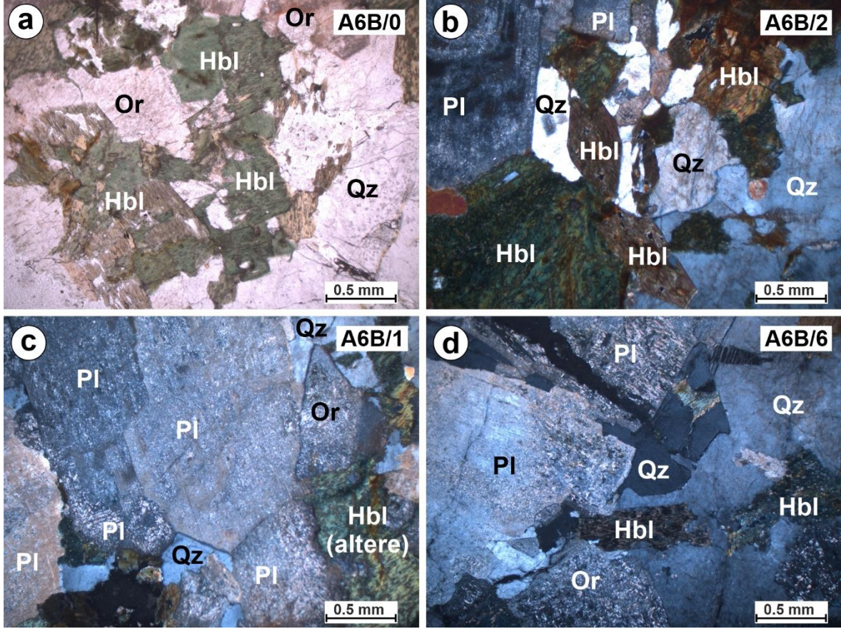
Şekil 3.7. Granodiyoritlerin mikroskobik görünüşleri. a) Yeşilimsi renkli hornblend minerallerinin tek nikoldeki görünümü. b) Yarı özşekilli ve özşekilli hornblend mineralleri ile kuvars ve plajiyoklas minerallerinin görünümü. c-d) İri kristalli plajiyoklas ve ortoklas mineralleri ile nispeten küçük kristalli gelişmiş kuvars mineralleri ve altere hornblend. Qz: Kuvars, Or: Ortoklas, Pl: Plajiyoklas, Hbl: Hornblend (a görüntüsü tek nikol, diğer görüntüler ise çapraz nikolde alınmıştır)
