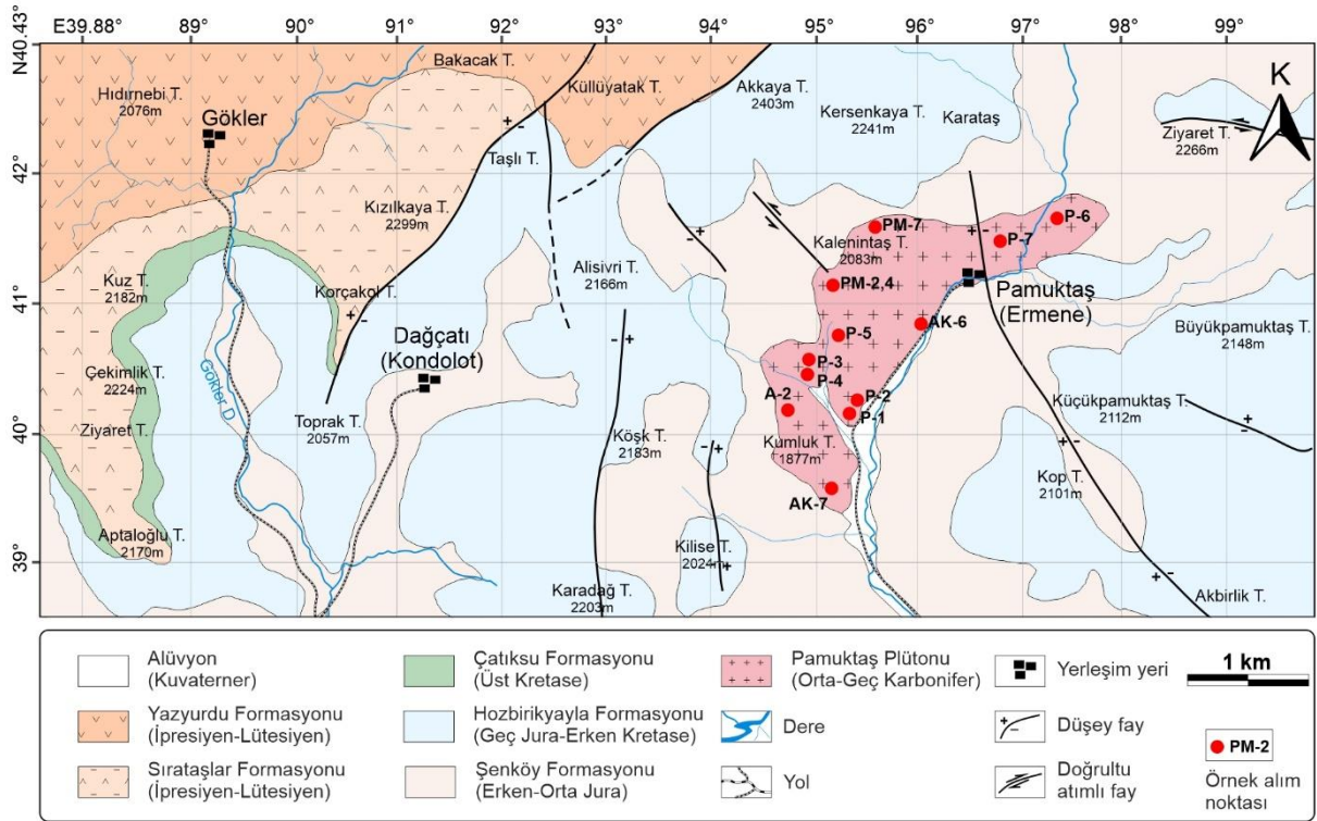
Şekil 3.1. Pamuktaş (Bayburt, KD Türkiye) ve civarının jeoloji haritası
