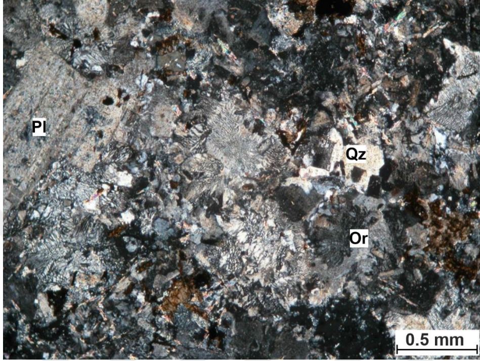
Şekil 3.8. Kuvarslı mikrodiorit örneğinin mikroskopik görünümü (Pl: Plajiyoklas, Qz: Kuvars, Or: Ortoklas, görüntü çapraz nikelde alınmıştır)
