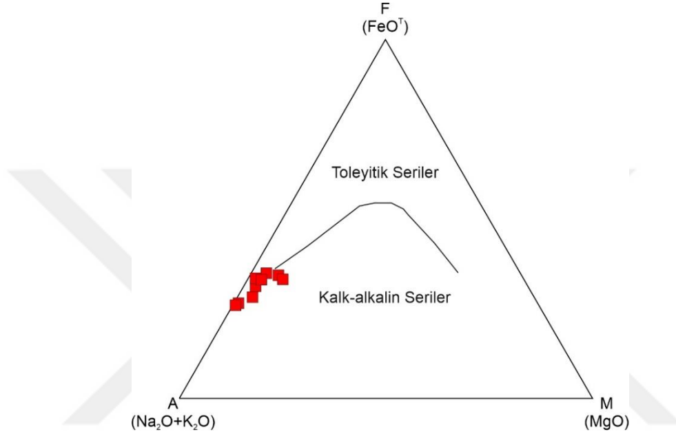
Şekil 3.10. Granitlerin AFM ( Na_2O+K_2O , Fe_2O_3^T , MgO) diyagramı. Toleyitik-kalk-alkalin ayırım eğrisi Irvine ve Baragar (1971)'e göre
