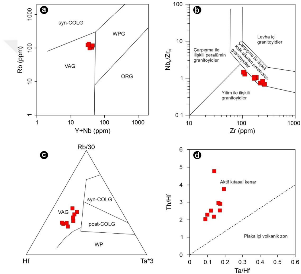
Şekil 4.10. a) Rb (ppm)-Y+Nb (ppm) (Pearce vd., 1984), b) Zr (ppm) - Nb N /Zr N (Thiéblemont ve Téguy, 1994), c) Rb/30-Hf-Ta*3 (Harris vd., 1986) ve d) Th/Hf-Ta/Hf (Schandl ve Gorton, 2002) diyagramları. syn-COLG: çarpışma ile eş yaşlı granitler, post-COLG: çarpışma sonrası granitleri, VAG: volkanik yay granitleri, WPG: levha-içi granitleri, ORG: okyanus sırtı granitleri. Nb/Zr oranları Hofmann (1988)'in ilksel manto değerine (Nb: 0.6175, Zr: 9.714) göre normalize edilmiştir
