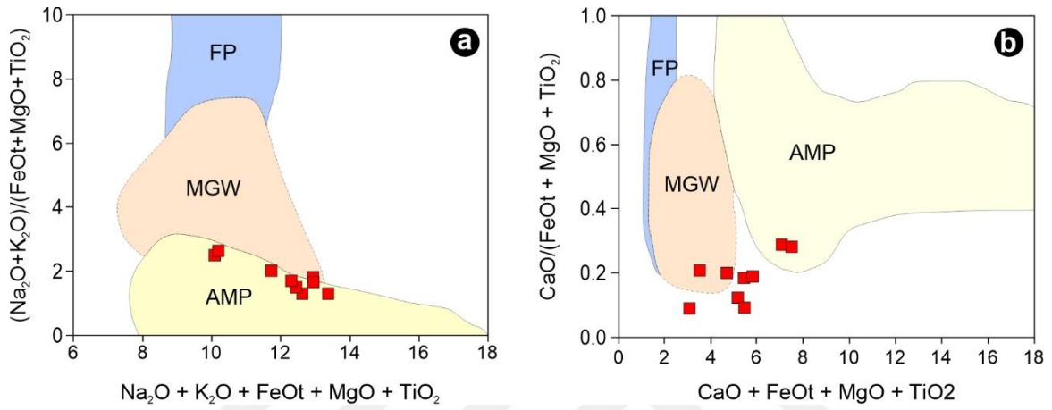
Şekil 4.7. Pamultaş plütönu örneklerinin bazı ana oksit oranlarına göre kökensel ayırım diyagramları. MGW: metagrovak, FP: felsik pelit, AMP: amfibolit. Veri kaynak alanları Patiño Douce (1999)'dan alınmıştır
