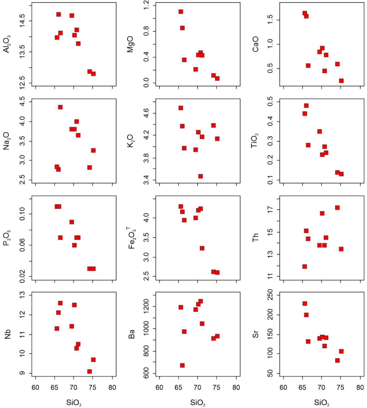
Şekil 3.12. Pamuktaş plütonu kayaçlarının SiO 2 (%)’e karşı ana oksit (%) ve iz element (ppm) değişim diyagramları
