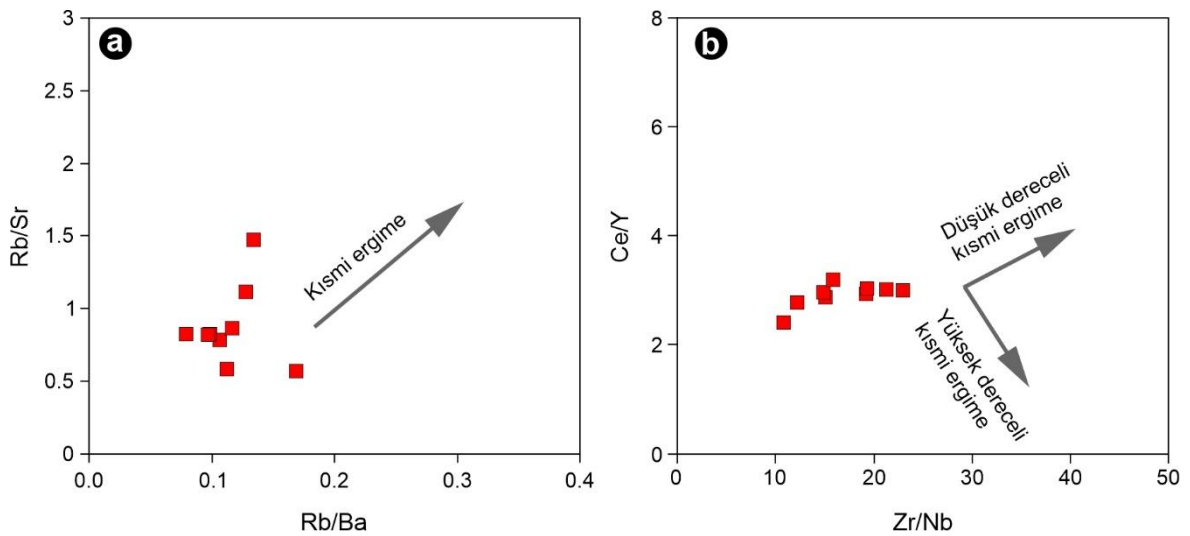
Şekil 4.1. Pamuktaş plütönü kayalarının a) Rb/Sr-Rb/Ba ve b) Ce/Y-Zr/Nb diyagramları
