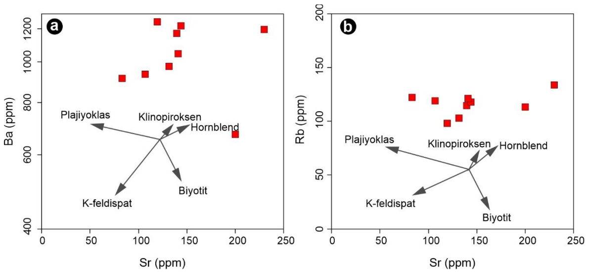
Şekil 4.2. Örneklerin mineral fraksiyonlaşma yönünü gösteren diyagramlar. a) Ba (ppm)'a karşı Sr (ppm) ve b) Rb (ppm)'a karşı Sr (ppm) diyagramları
