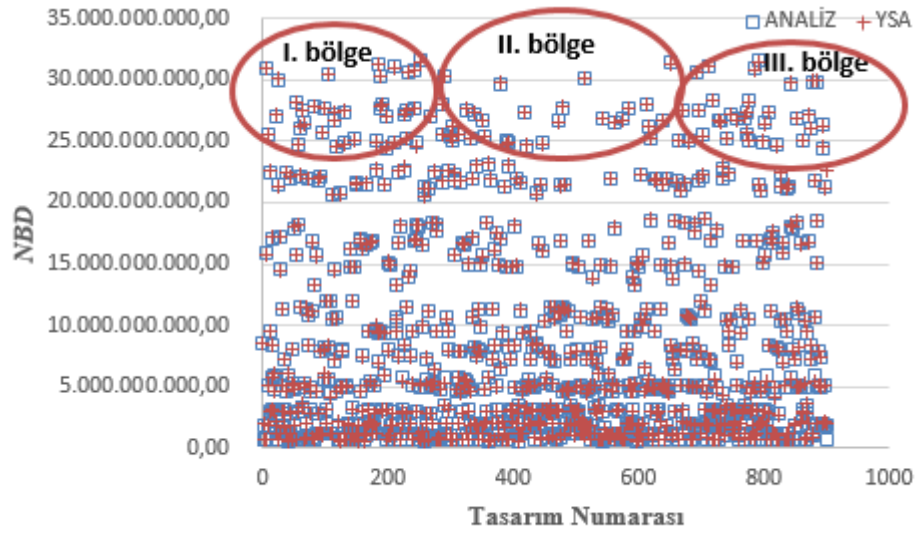
Şekil 6.26. R-1234ze kullanılan sistemin optimizasyonu için belirlenen bölgeler.
