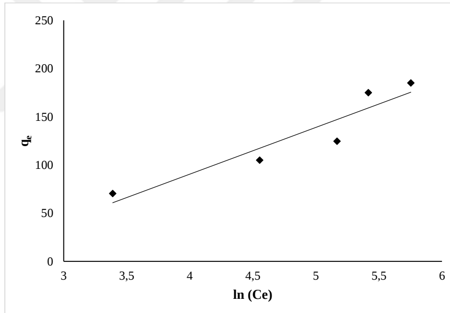
Şekil 5.7. Temkin izotermi
