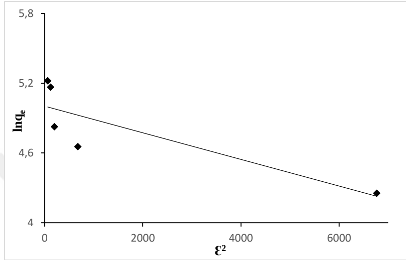
Şekil 5.8. Dubinin-Radushkevich izotermi
