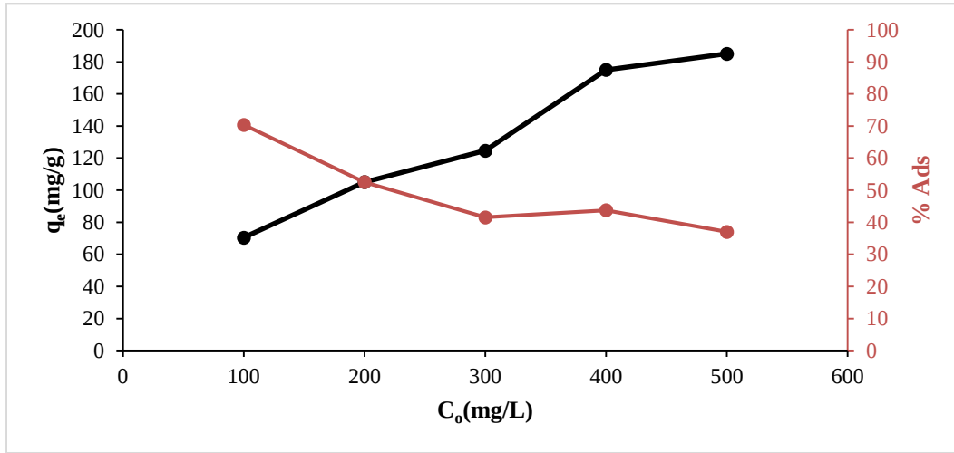
Şekil 5.4. Başlangıç konsantrasyonunun PSM giderimi üzerindeki etkisi
