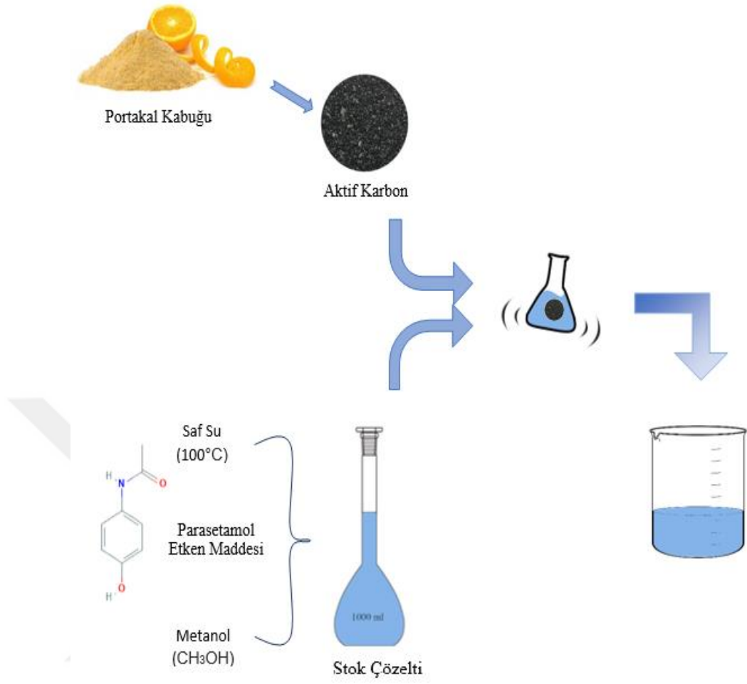
Şekil 4.1. Proses akım şeması
