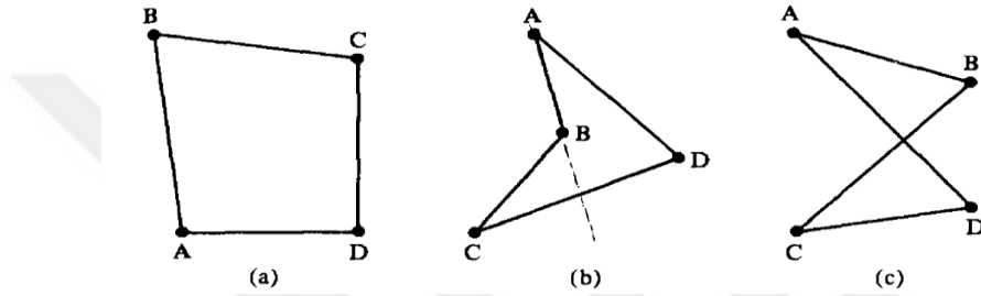
Şekil 3.19 Dörtgen ve dörtgen olmayan şekiller
