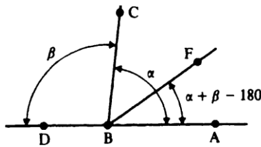
Şekil 4.11 m(\angle ABF) = \alpha + \beta - 180 olması durumunu gösteren \overrightarrow{BF} ışını
