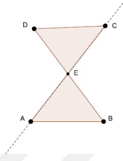
Şekil 3.22 Hiçbir köşesi karşı açısının içinde olmayan dörtgen
