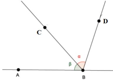
Şekil 4.9 \overrightarrow{BD} nin aynı tarafında olan A ve C noktalarının oluşturduğu açılar
