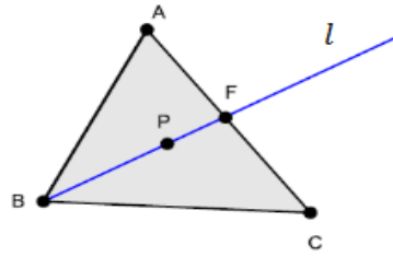
Şekil 3.15 l \cap \text{int}(\Delta ABC) \neq \emptyset olması durumu
