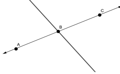
Şekil 3.6 l doğrusunun zıt tarafında bulunan int(\overrightarrow{BA}) ve int(\overrightarrow{BC})
