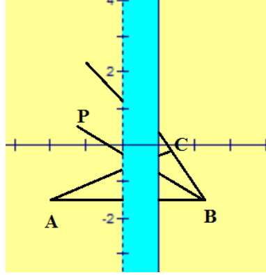
Şekil 3.14 Missing Strip düzleminde \overline{AC} yi kesmeyen \overrightarrow{BP} ışını
