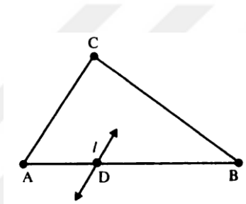
Şekil 3.1 Metrik geometride PP yi sağlayan \Delta ABC üçgeni
