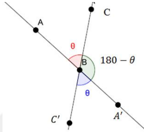
Şekil 4.17 Açıölçer geometride ters açılar
