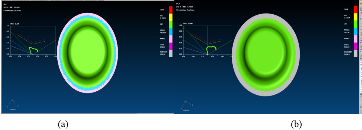
Şekil 4.12. 12,7 mm zımba radüsü kullanımı sonucunda şekillendirme sınır diyagramlarının karşılaştırılması
