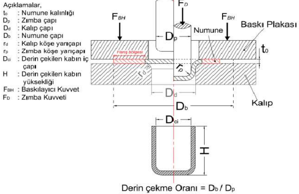
Şekil 2.1. Derin çekme terimleri ve açıklamalar
