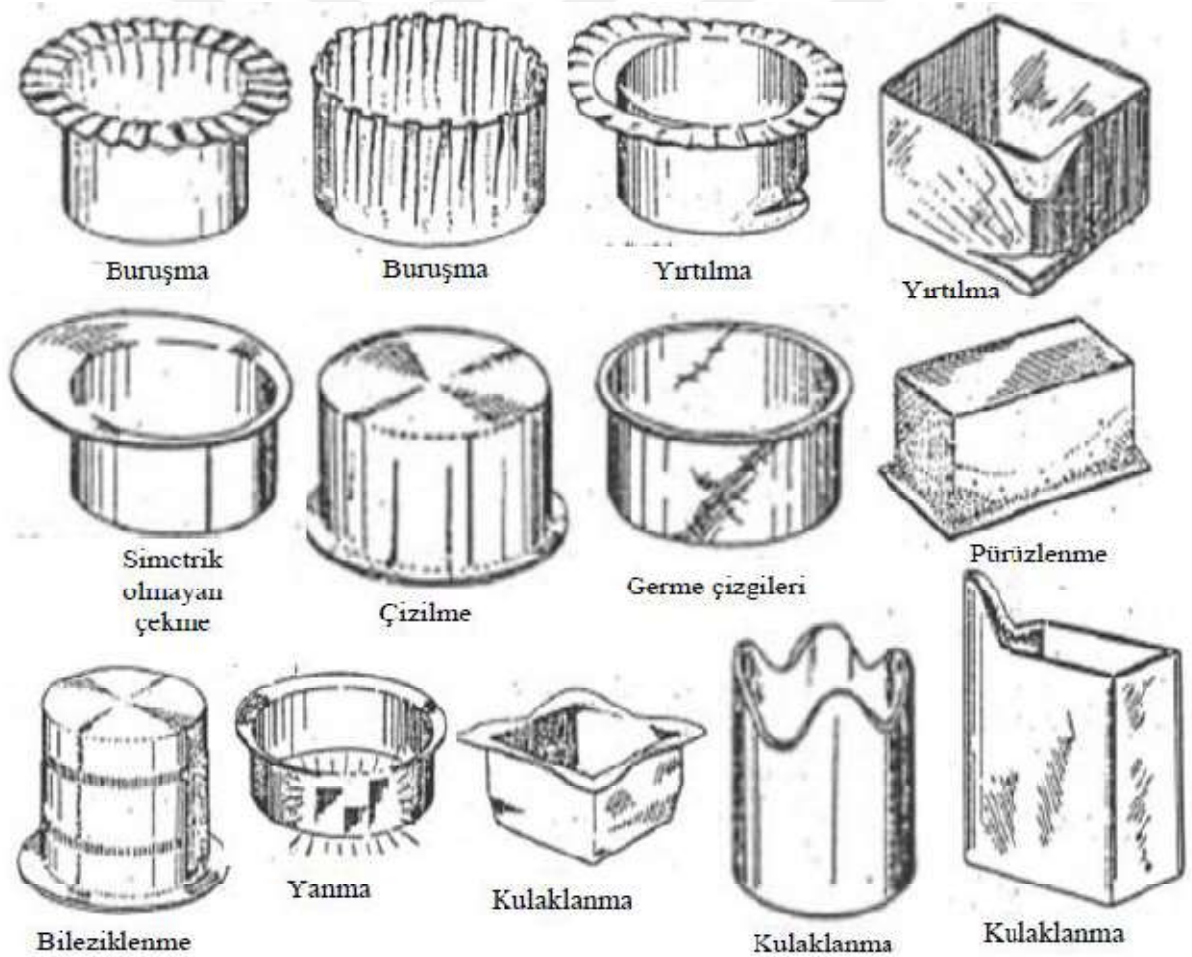
Şekil 2.10. Derin çekme işleminde görülen çekme kusurlar
