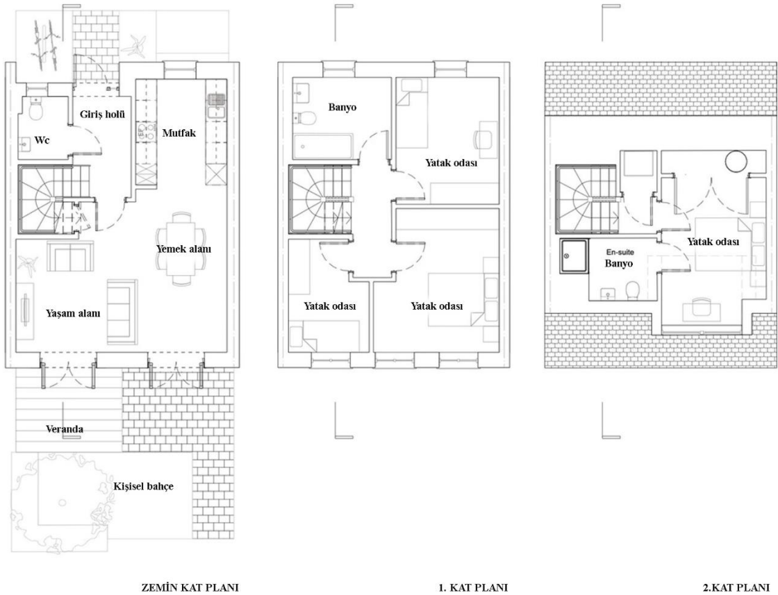
Şekil 4.3. Marmalade Lane Paylaşımlı Konut projesi, konut ünitesi tip planı (Url-2)
