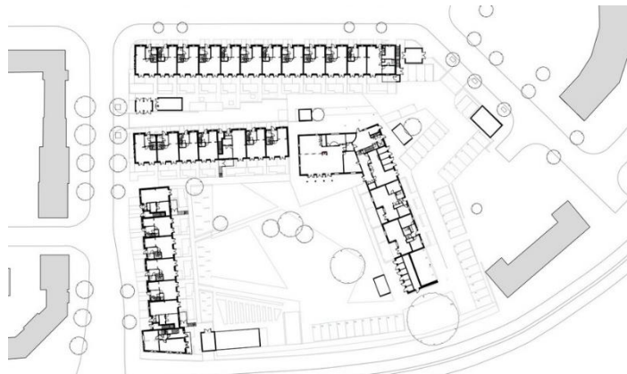
Şekil 4.7. Marmalade Lane Paylaşımlı Konut projesi, yerleşim planı (Url-5)
