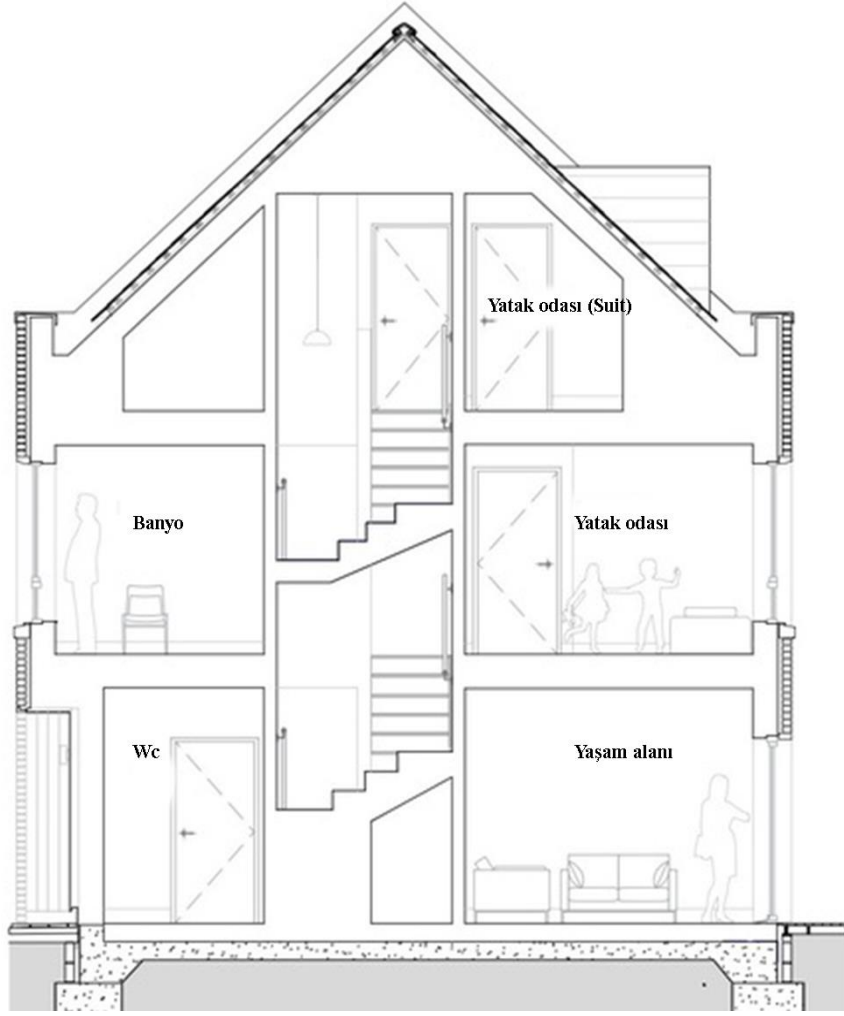
Şekil 4.4. Marmalade Lane Paylaşımlı Konut projesi, tip konut ünitesi kesiti (Url-3)
