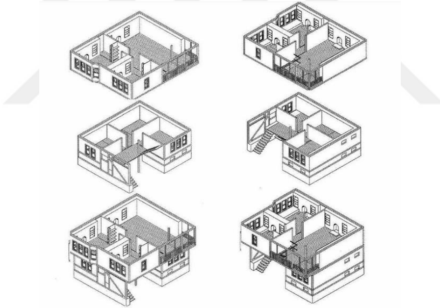
Şekil 3.19. Türk Evi'nde dikey süreklilik, aynı yapı için iki farklı noktadan alınan patlatılmış perspektif (Yürekli & Yürekli, 2005, p.28; Kömürcüoğlu, 1966'dan aktarıldığı üzere)
