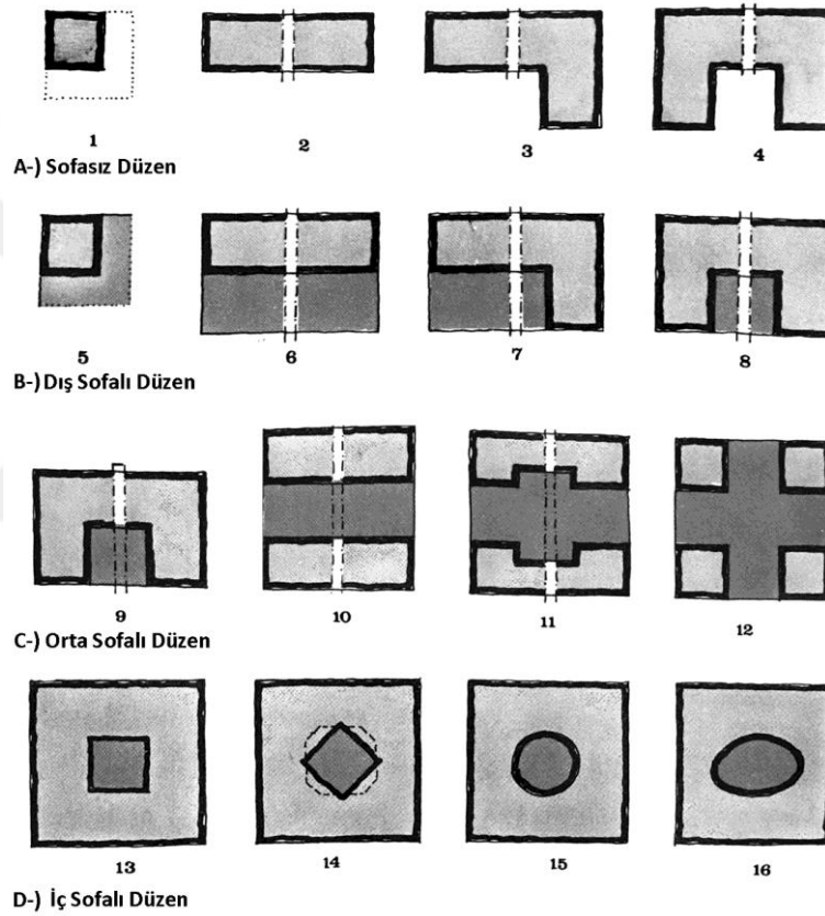
Şekil 3.20. Türk Evi'ndeki sofa düzeninde, standartlaşma ve çeşitlilik (Küçükerman, 1991, p.102-103)
