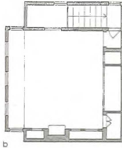
Şekil 3.21. Tek odalı Türk Evi plan örneği (Kuban, 1995, p.106)
