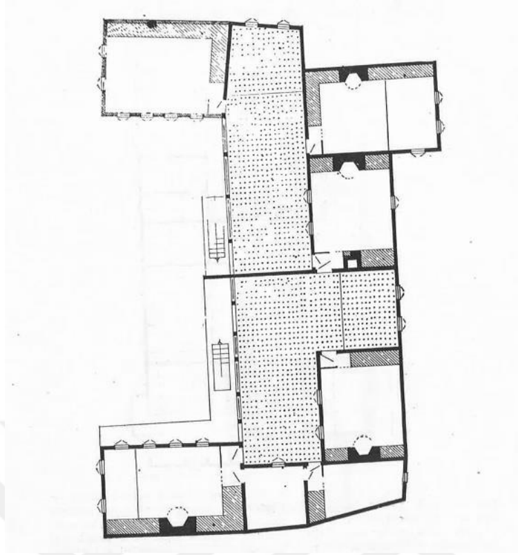
Şekil 3.18. İki bölümlü dış sofalı Türk Evi plan örneği, Köprülüler konağı-Vezirköprü (Eldem, 1954, p.153)
