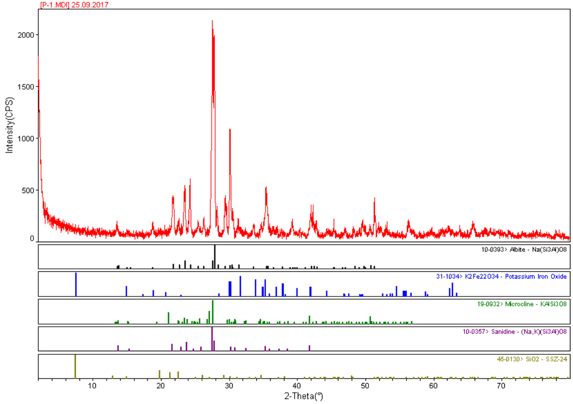
Şekil 4. 22. Pazarcık (Kahramanmaraş) magmatitiği XRD grafiği
