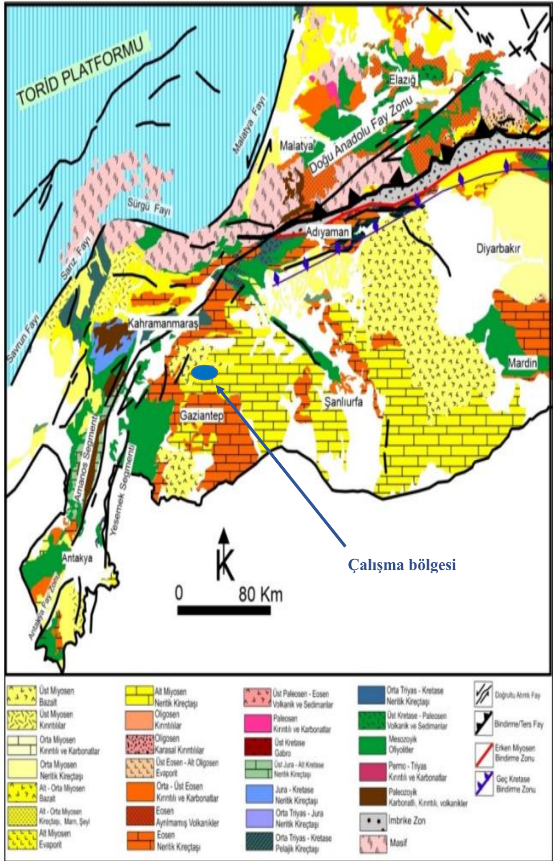
Şekil 2. 1. Pazarcık (Kahramanmaraş) bölgesinin genel jeoloji haritası [2].
