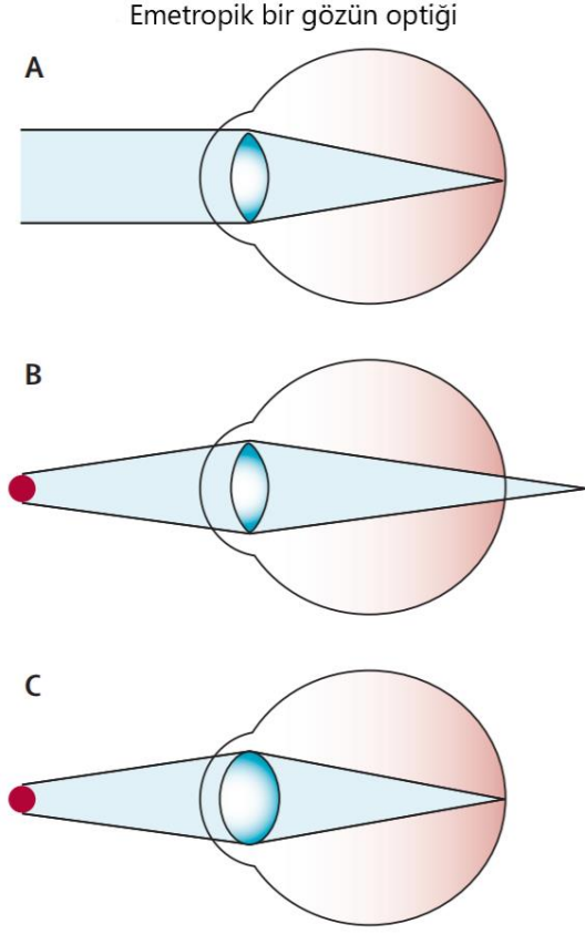
Şekil 2.11. Emetropik gözlerde gözün şematik optiği (121)
