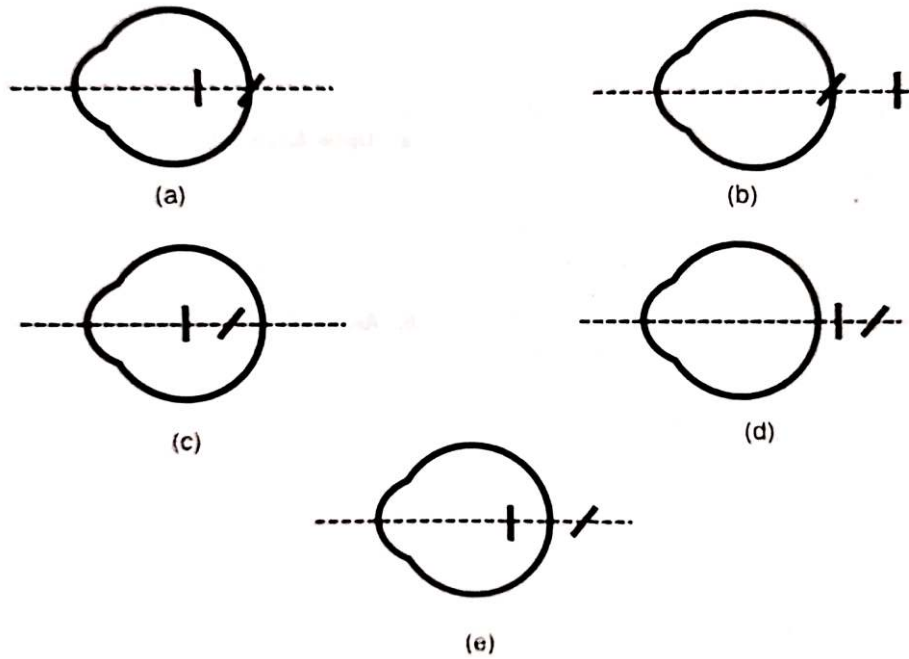
Şekil 2.15. Astigmatizma tiplerinde fokal çizgilerinin retinaya göre konumları (1)
