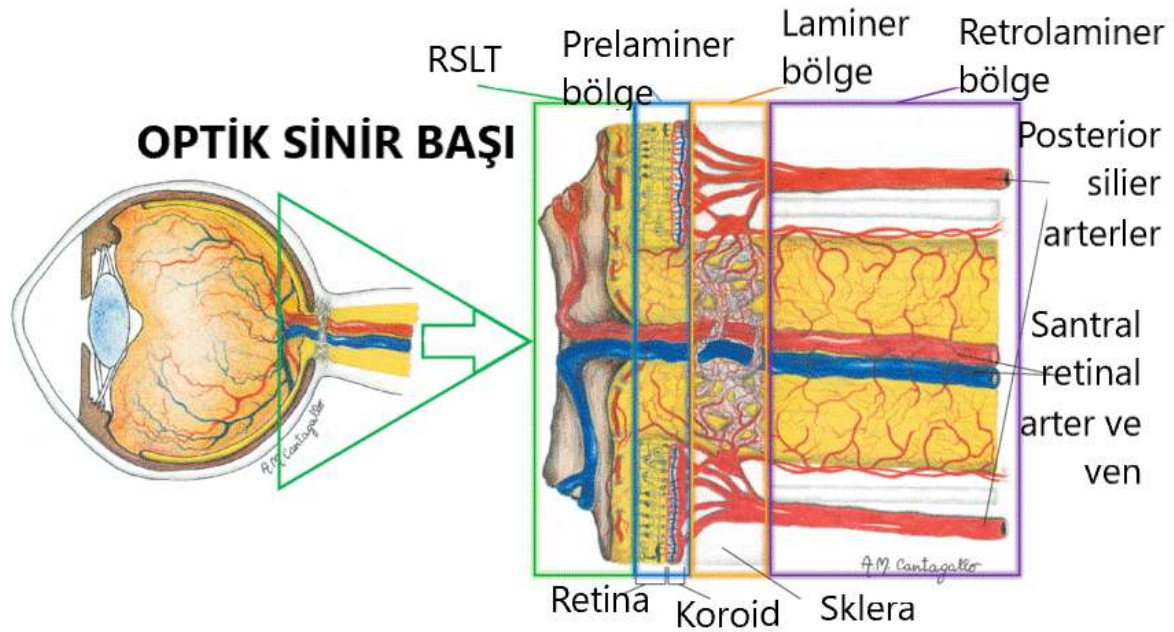
Şekil 2.7. Optik sinir başının topografisi ve vasküler yapısı (91)
