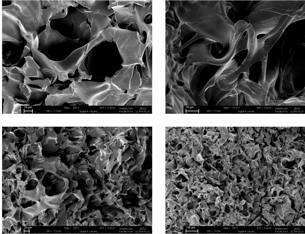
Şekil 4.1. Poli(HEMA-co-MAAP) kriyojelin SEM görüntüsü
