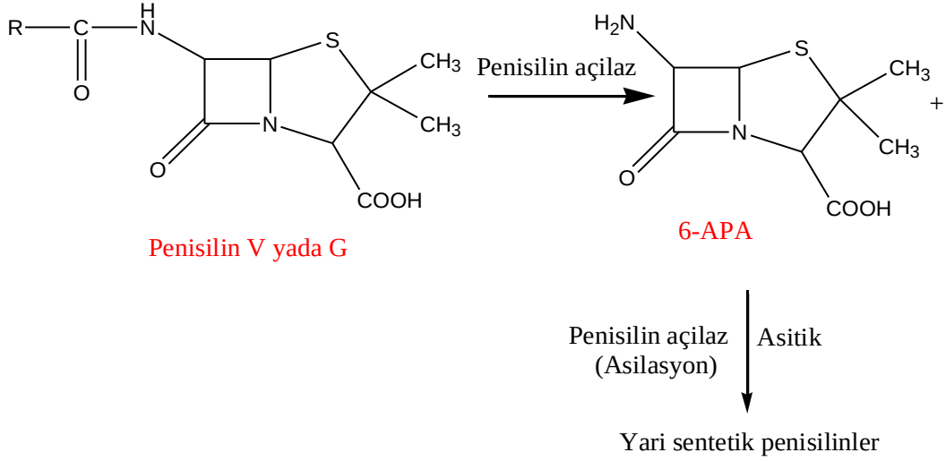
Şekil 2.15. Penisilinin, 6-APA ve yarı sentetik penisilinlere enzimatik modifikasyonu (Parmar ve ark. 2000)
