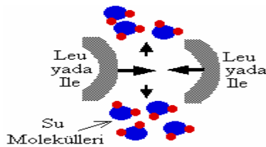
Şekil 2.5. Hidrofobik etkileşimler
