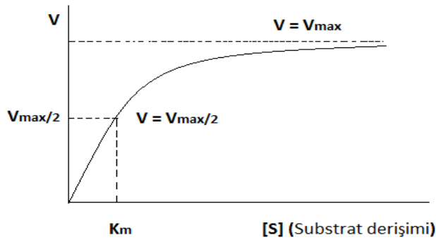
Şekil 2.9. Enzimatik reaksiyonun hızı üzerine substrat derişiminin etkisi
