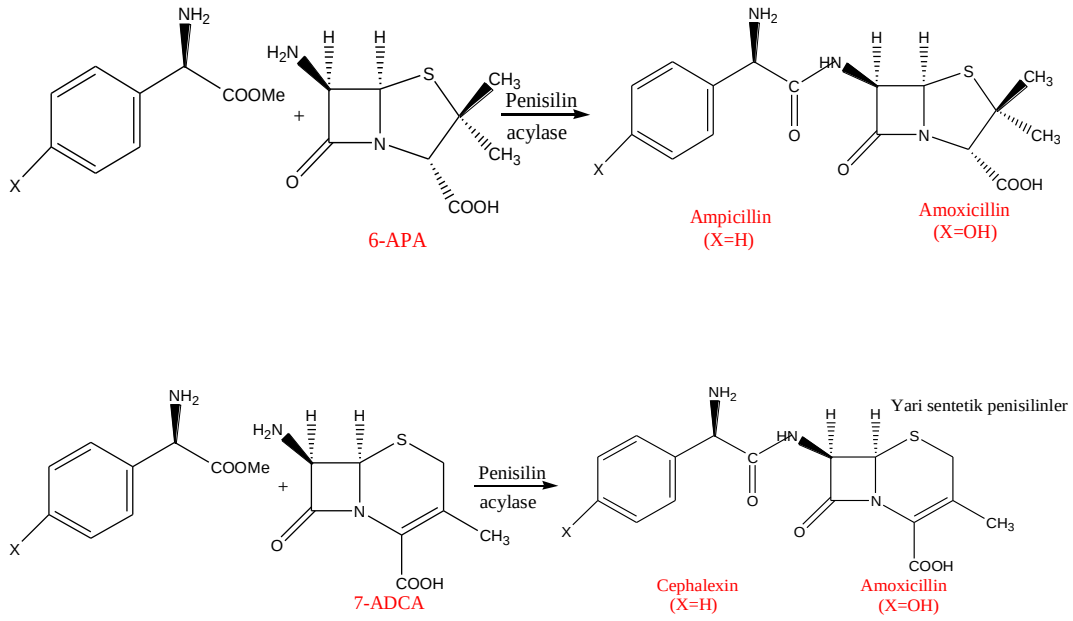
Şekil 2.16. Bazı önemli \beta -laktam antibiyotiklerin penisilin açılazla katalize edilen sentezi (Arroyo ve ark. 2003)
