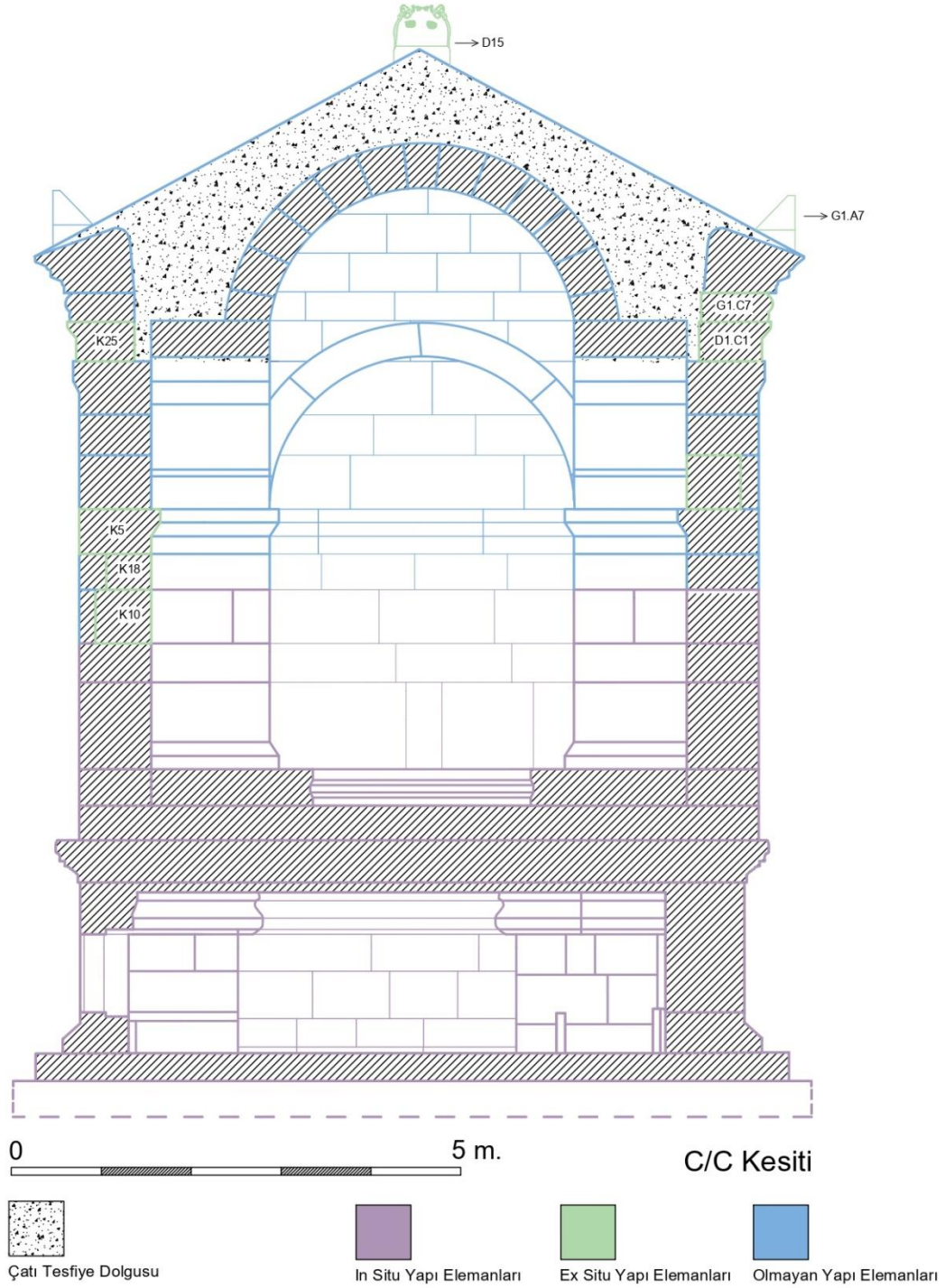
Çizim 21: Doğu Görünüşlü Kuzey-Güney Kesiti
