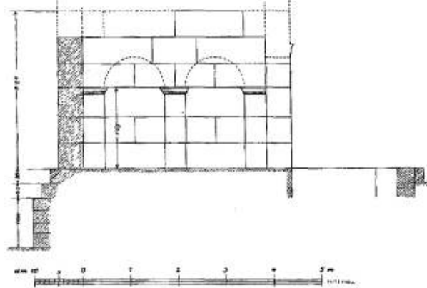
Çizim 58: Semneia/Senneia 1 Numaralı Mezar (Swoboda- Keil- Knoll, 1935: Fig.26)
