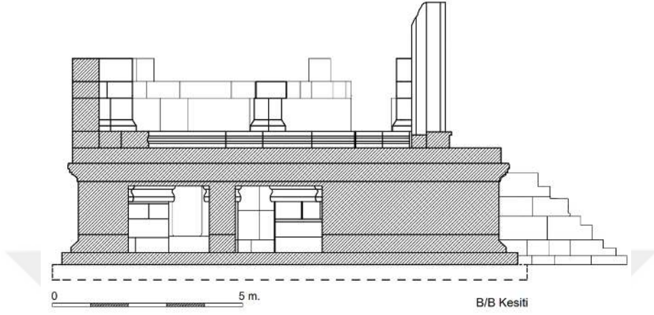
Çizim 7: M58 Mezarı Kuzey Görünüşlü Doğu-Batı Kesiti
