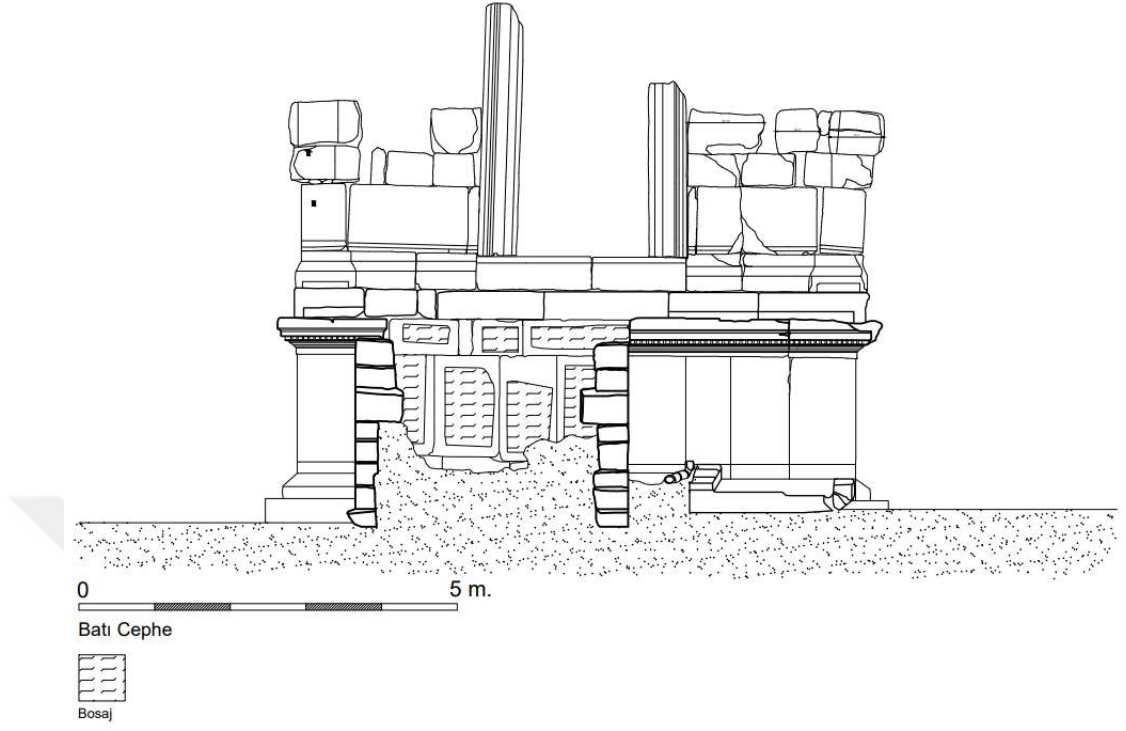
Çizim 2: M58 Mezarı Batı Cephe Rölövesi
