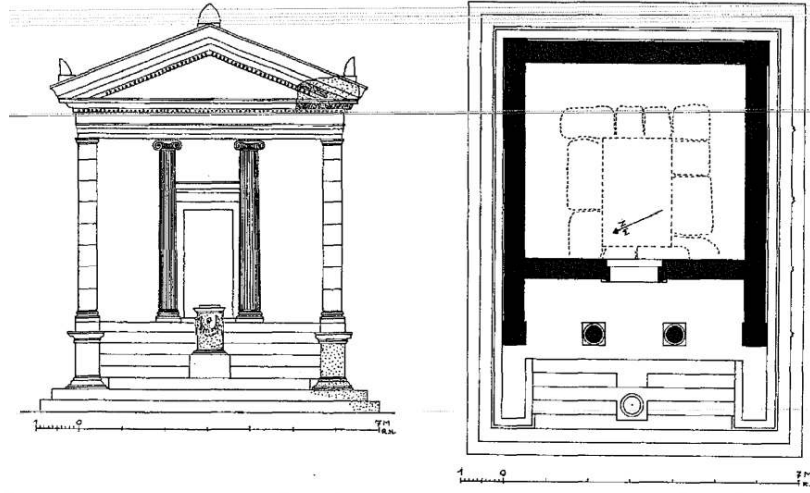
Çizim 37: Aizonai'den İnamural Tapınak Tipli Mezar
