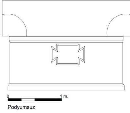
Çizim 24: L1 Lahdi, Güney Yüz
