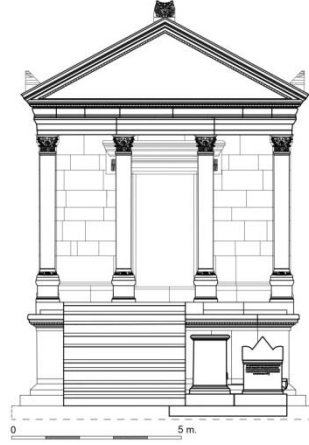
Çizim 15: Batı Cephe Rekonstrüksiyonu
