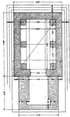
Çizim 58: Semneia/Senneia 1 Numaralı Mezar (Swoboda- Keil- Knoll, 1935: Fig.26)
