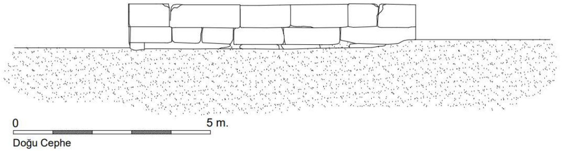
Çizim 5: M58 Mezarı Doğu Cephe Rölövesi
