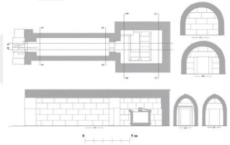
Çizim 30: Hekatomnos Mezarı Plan ve Kesitler (Diler, 2021: 93, Fig.78, Çizim: G.Putgül)
