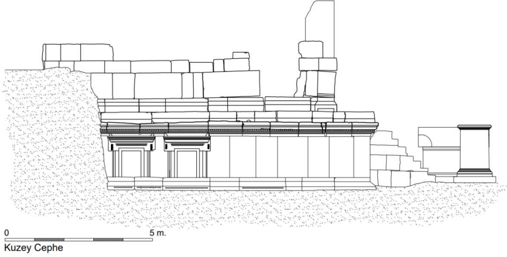
Çizim 3: M58 Mezarı Kuzey Cephe Rölövesi
