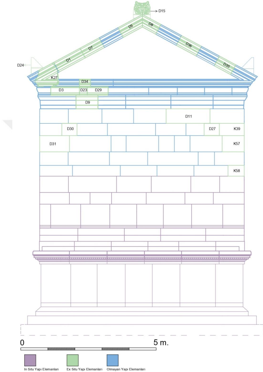
Çizim 14: Doğu Cephe Rekonstrüksiyonu
