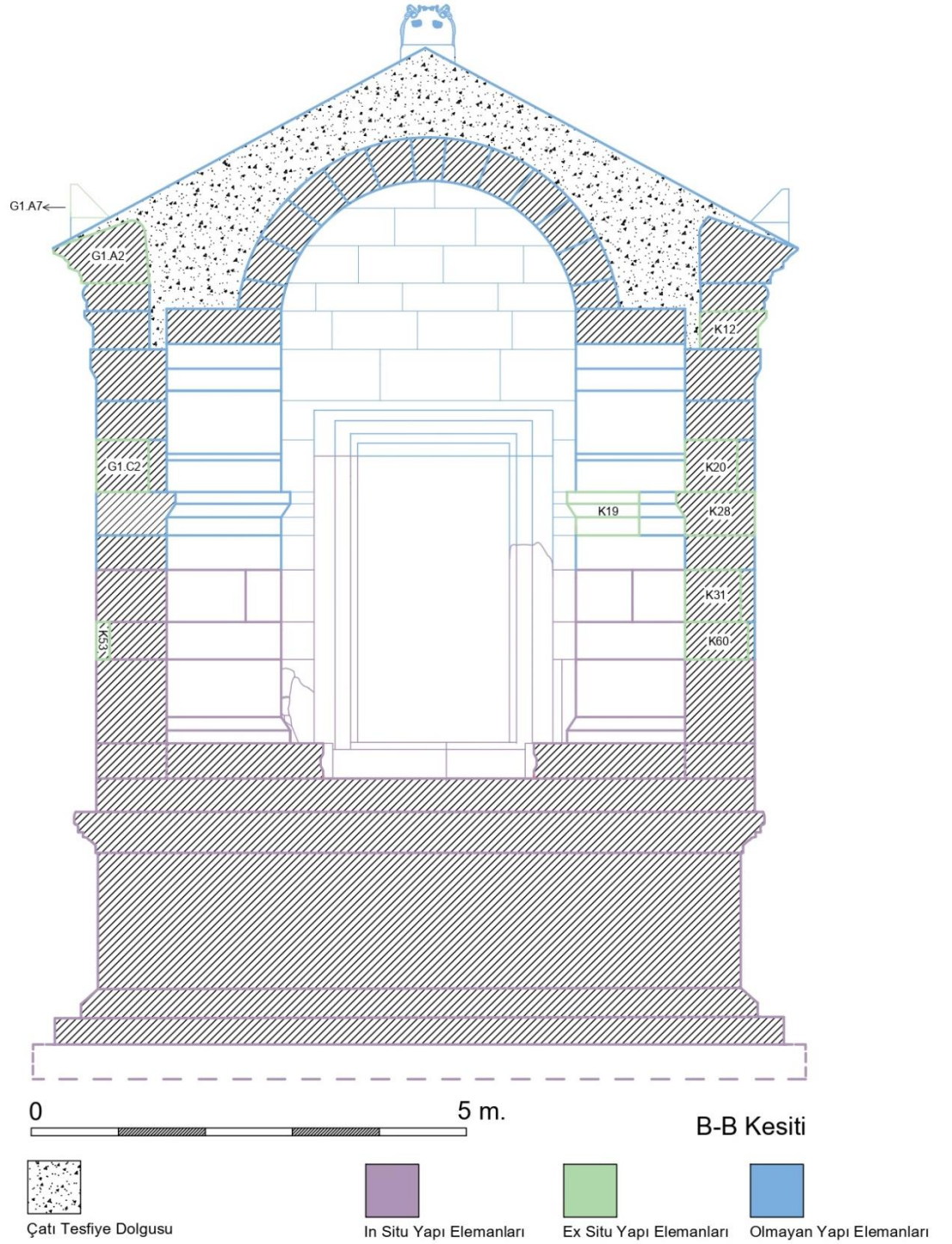
Çizim 20: Batı Görünüşlü Kuzey-Güney Kesiti
