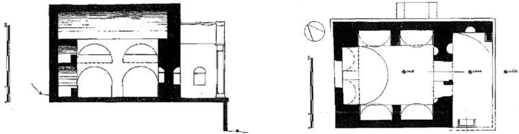
Çizim 50: İotape, 3 Numaralı Tapınak Tipli Mezar (Rosenbaum vd., 1967: Fig.38-39)
