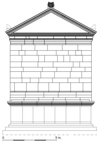
Çizim 18: Doğu Cephe Rekonstrüksiyonu
