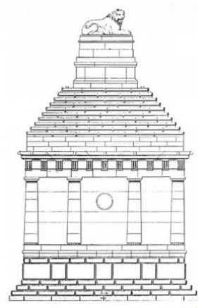
Çizim 31: Aslanlı Mezar (Rumscheid 1994: lev. 60, 1)
