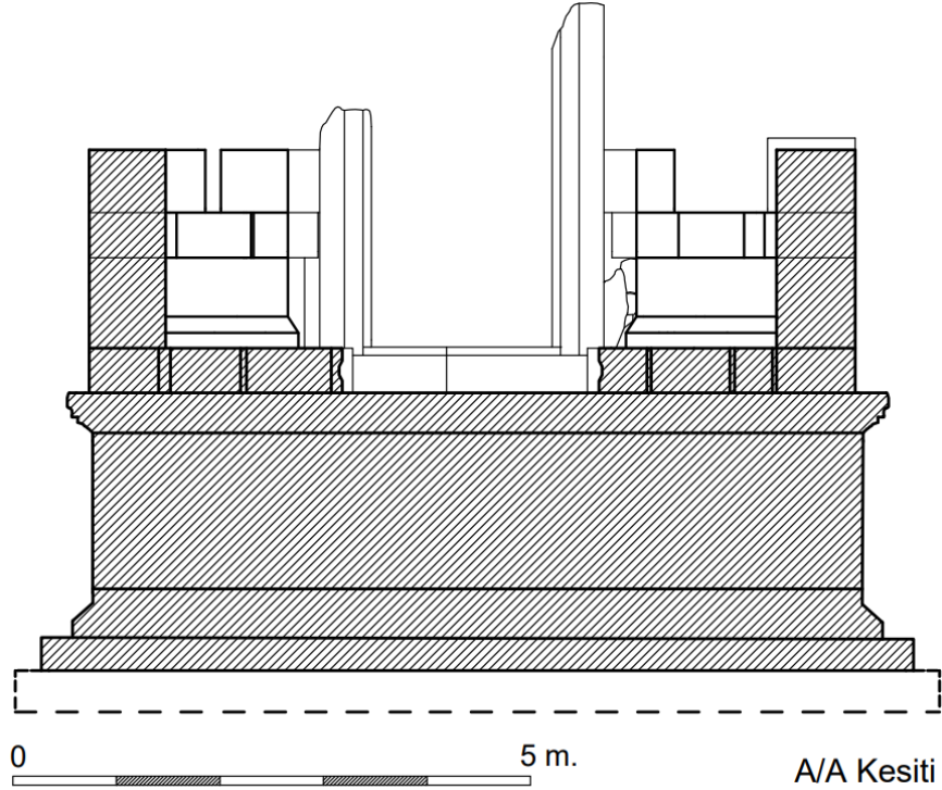
Çizim 6: M58 Mezarı Batı Görünüşlü Kuzey-Güney Kesiti
