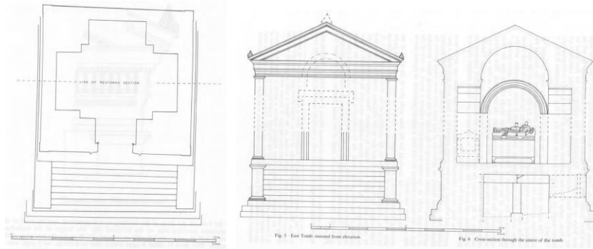
Çizim 43: Balboursa Doğu Mezar (Hallet- Coulton, 1993: 47, Fig.5-6)
