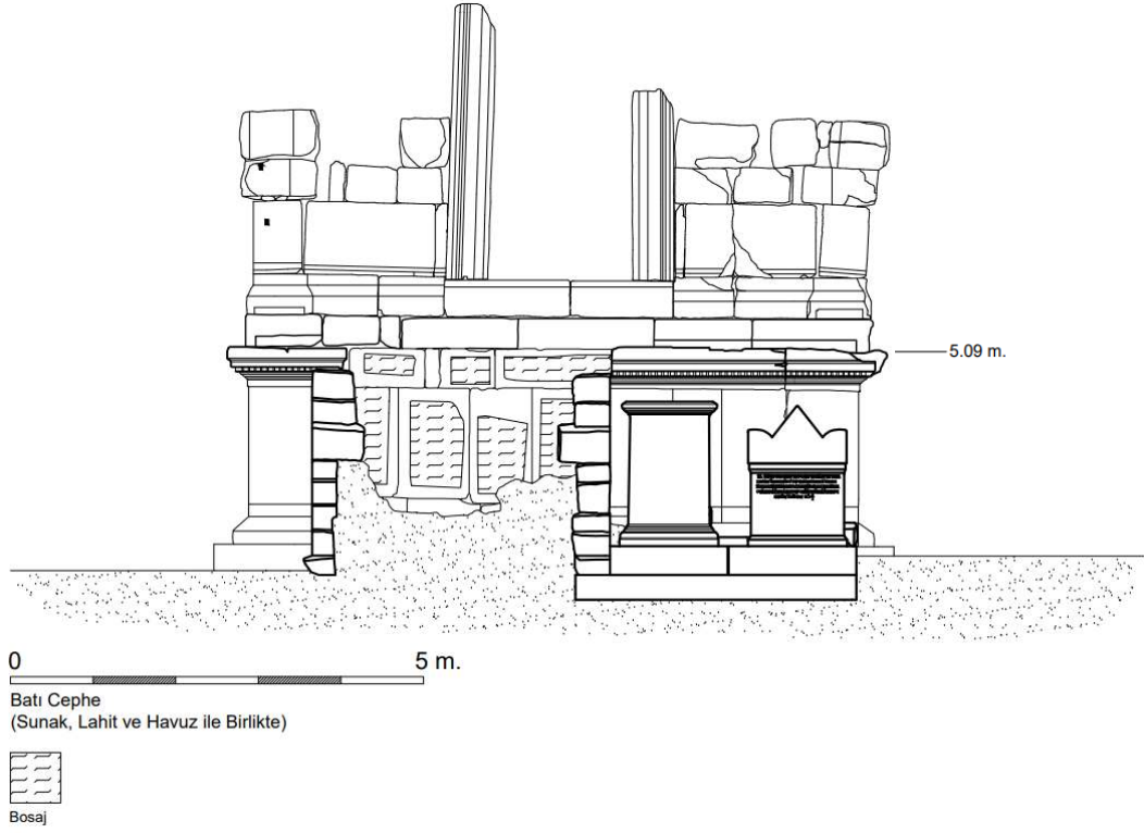
Çizim 1: M58 Mezarı Batı Cephe Rölövesi
