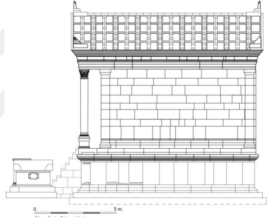
Çizim 17: Güney Cephe Rekonstrüksiyonu
