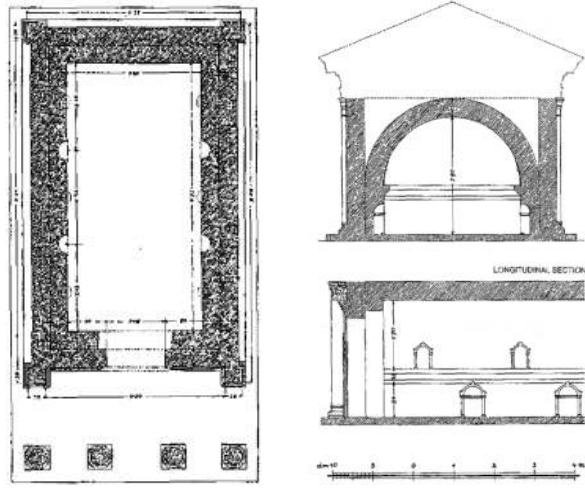
Çizim 51: Isauria'dan Tapınak Tipli Mezar (Swoboda vd. 1935: Fig.71)
