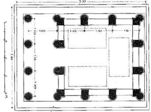
Çizim 61: Termessos, Tiberia Klaudia Agrippina Tarafından Yaptırılan Mezar (Heberdey-Wilberg, 1900: Fig.52,55.)
