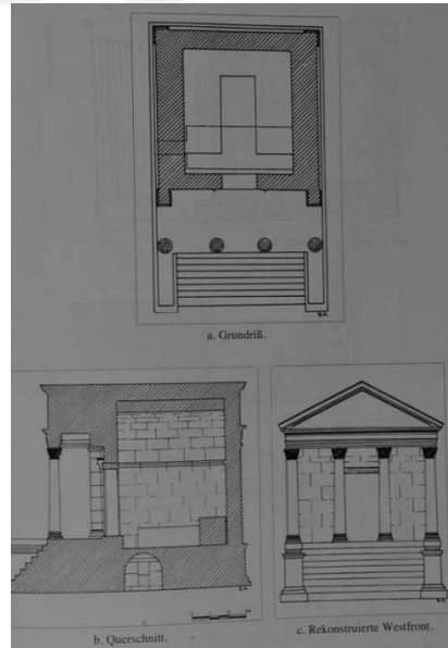
Çizim 53: Patara Akdam Mezarı (Işık, 1995: 179, Abb.3a-c)
