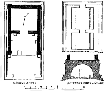
Çizim 44: Cambazlı Büyük Mezar (Keil- Wilhelm, 1931: 35, Fig.54)
