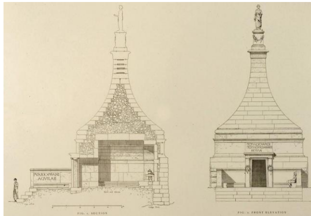
Çizim 34: Publius Varius Aquila'nın Mezarı (Clarke- Bacon- Koldewey, 1902: 231, Fig. 1, 2)
