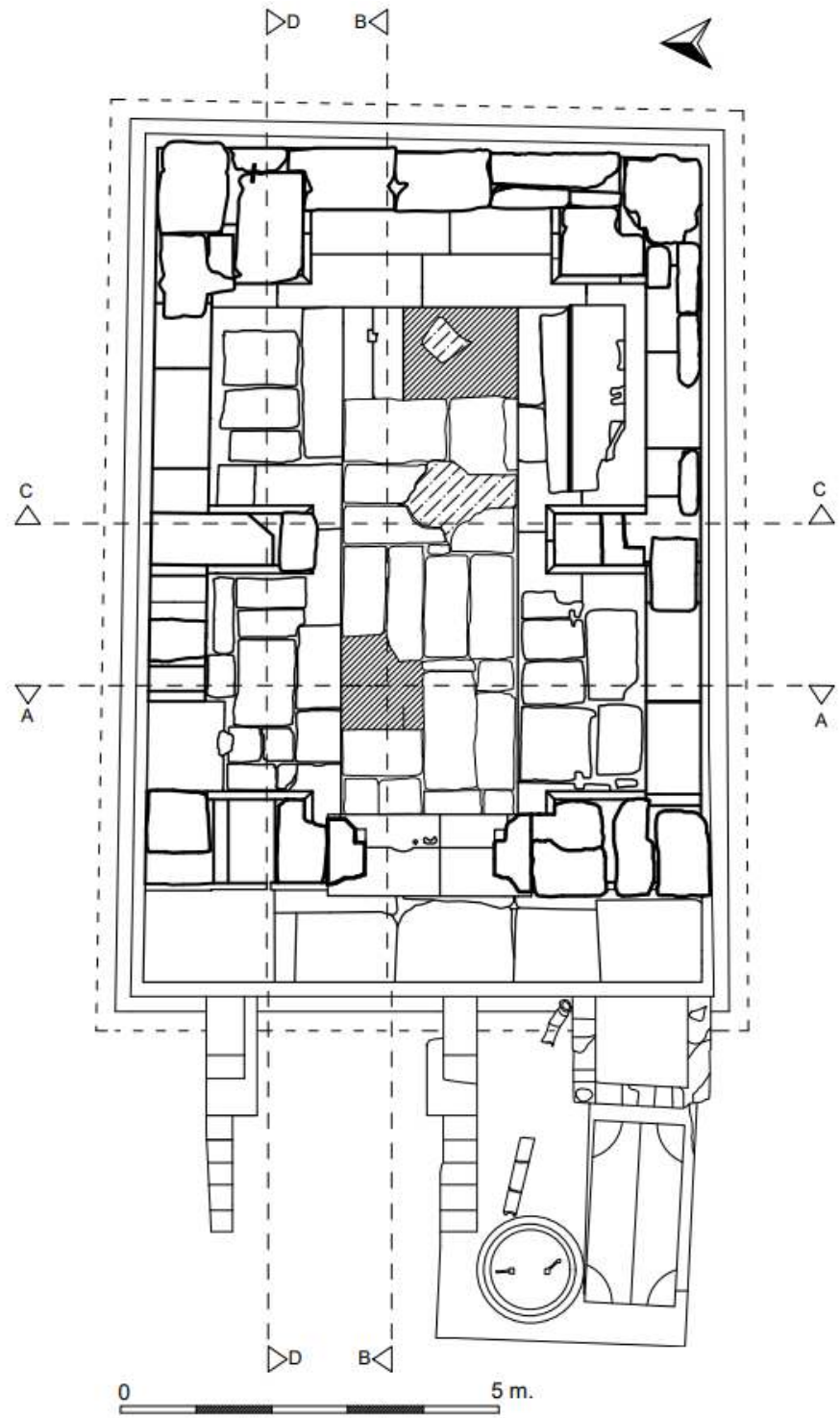
Plan 8: M58 Planı
