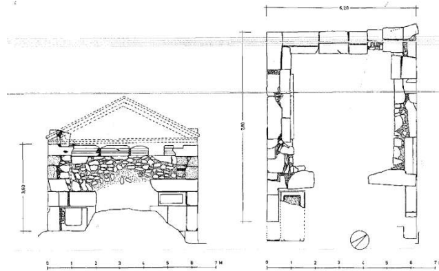
Çizim 39: Ariassos E7 Mezarı (Cormack, 2004: 181, Fig.38-39)
