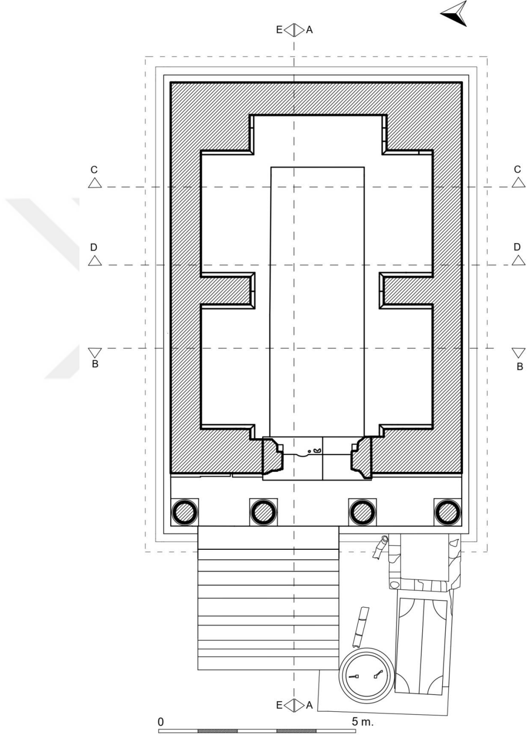
Plan 10: M58 Rekonstrüksiyon Planı
