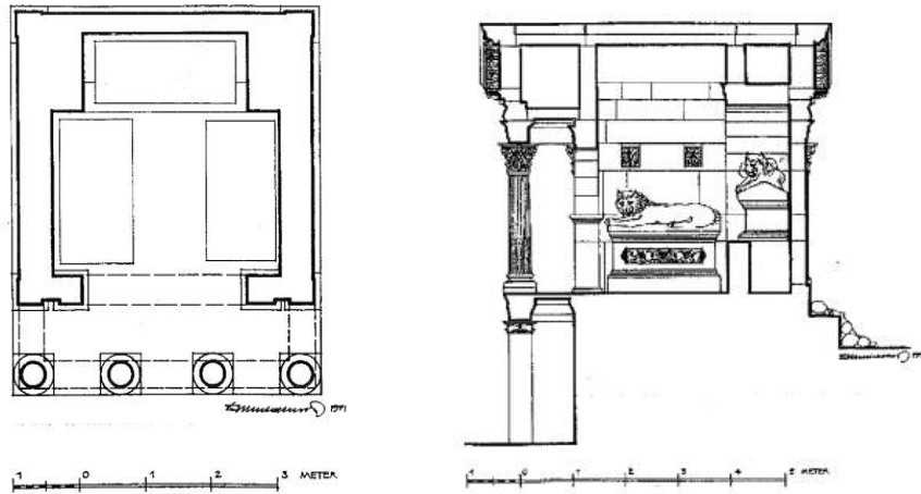
Çizim 47: Demircili/Dösene 2 Numaralı Tapınak Tipli Mezar
