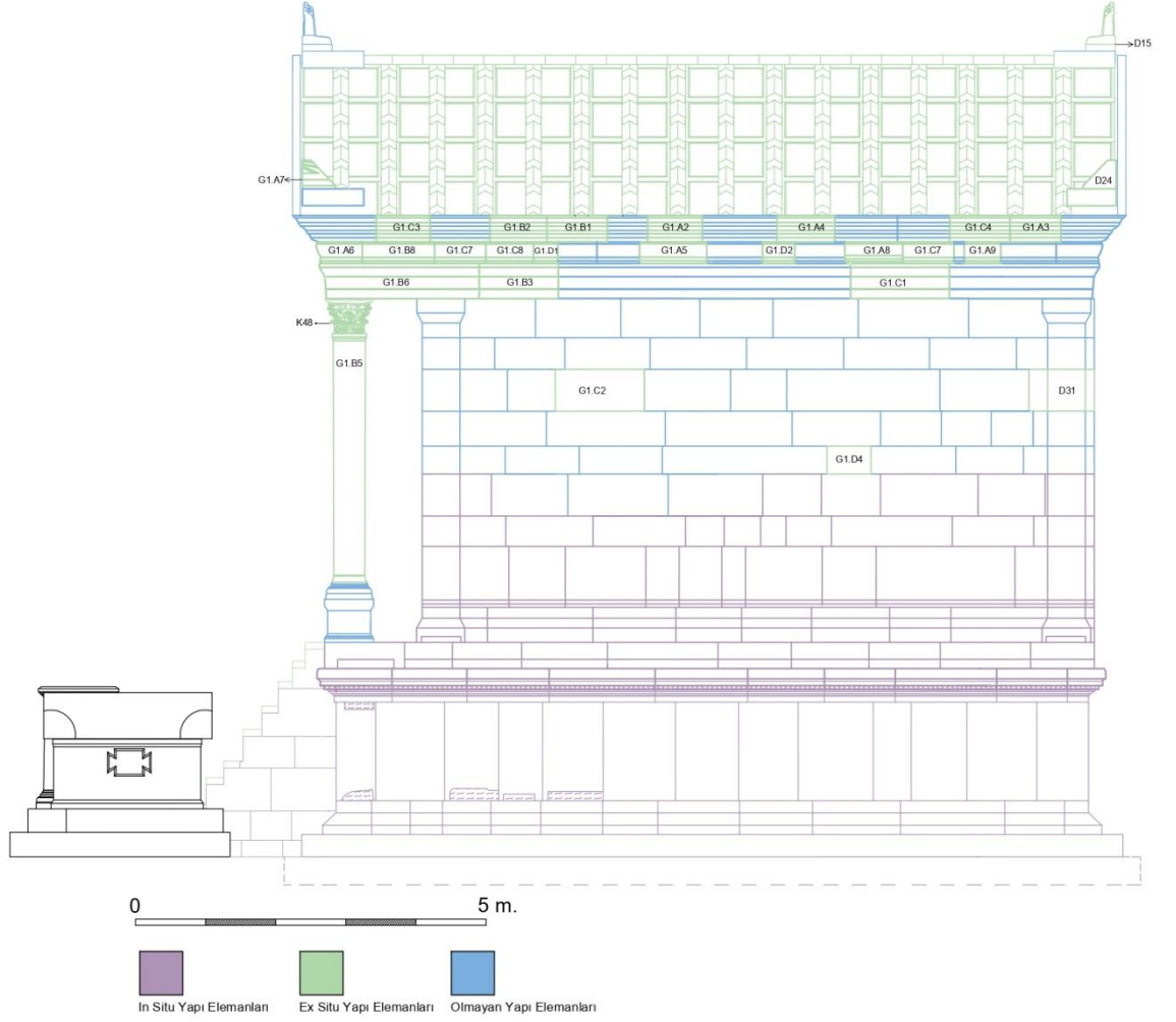
Çizim 13: Güney Cephe Rekonstrüksiyonu
