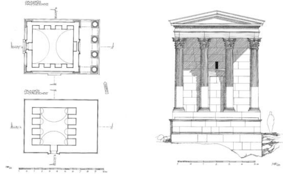
Çizim 49: Elauissa Sebaste T11 Mezarı
