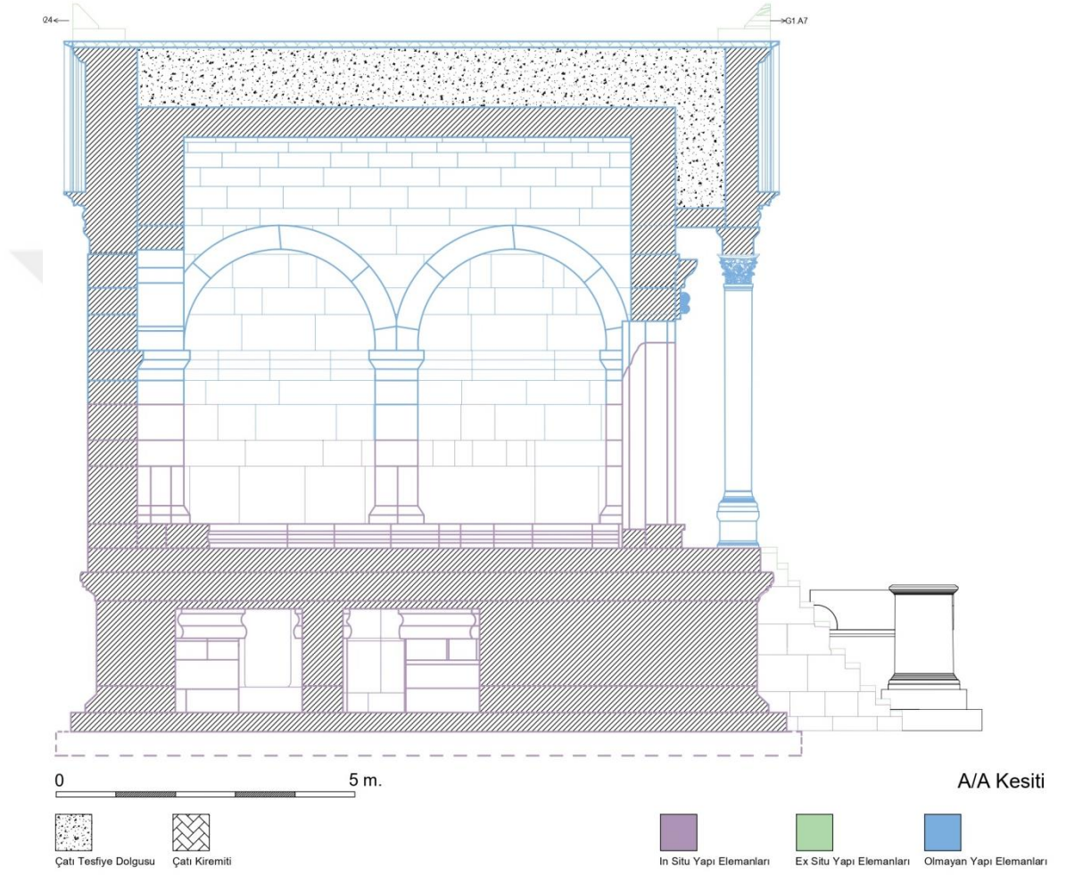
Çizim 19: Güney Görünüşlü Doğu-Batı Kesiti
