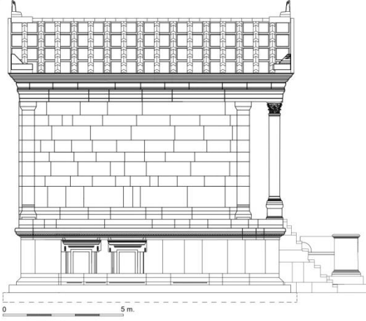
Çizim 16: Kuzey Cephe Rekonstrüksiyonu
