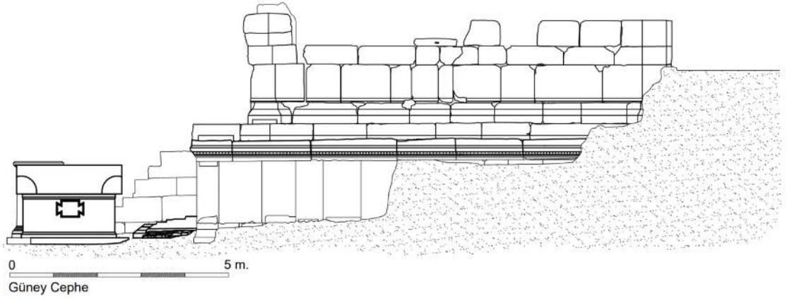
Çizim 4: M58 Mezarı Güney Cephe Rölövesi
