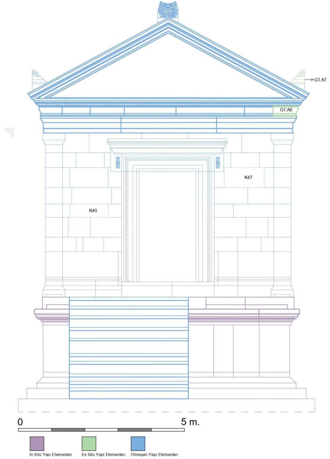
Çizim 11: Batı Cephe Rekonstrüksiyonu (Sütunsuz Görünüm)
