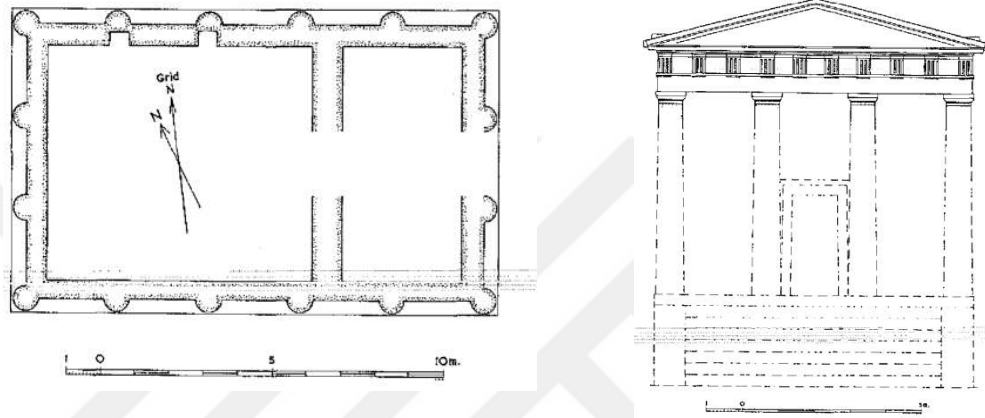
Çizim 52: Oinoanda MK2 Mezarı (Coulton, 1982:48,54, Fig.3,7)
