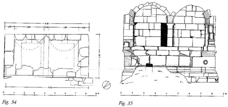
Çizim 41: Ariassos ST6 Mezarı (Cormack, 2004: 179, Fig.34-35)
