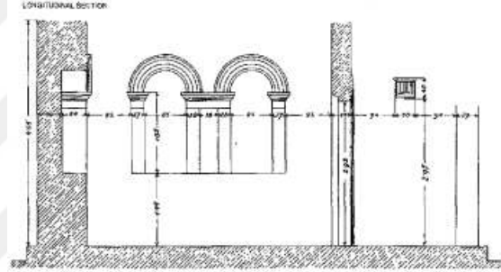
Çizim 59: Semneia/Senneia 2 Numaralı Mezar (Swoboda- Keil- Knoll, 1935: Fig.29)
