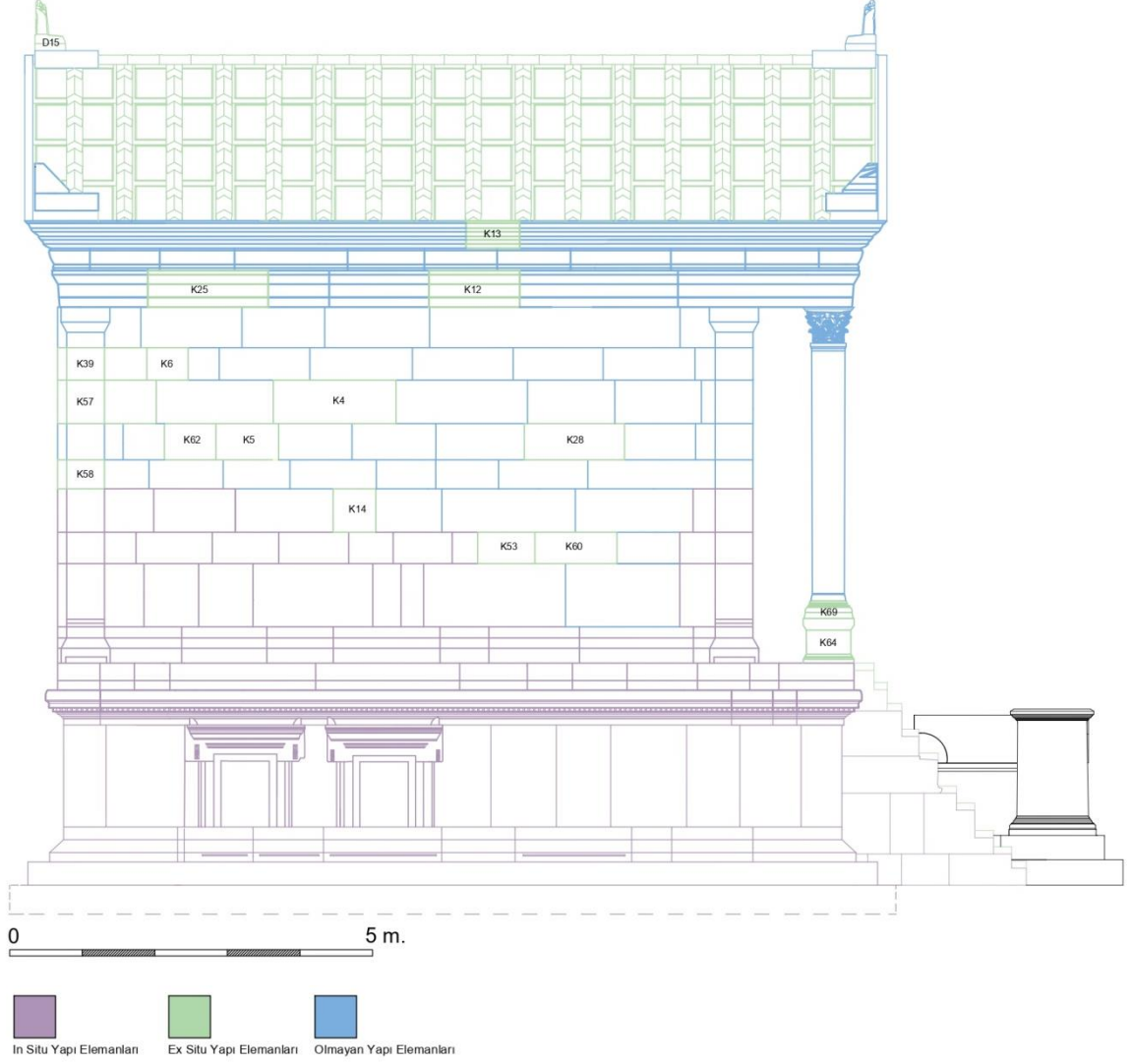
Çizim 12: Kuzey Cephe Rekonstrüksiyonu
