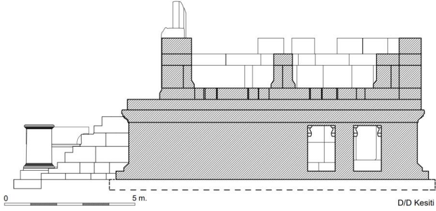
Çizim 8: Güney Görünüşlü Doğu-Batı Kesiti
