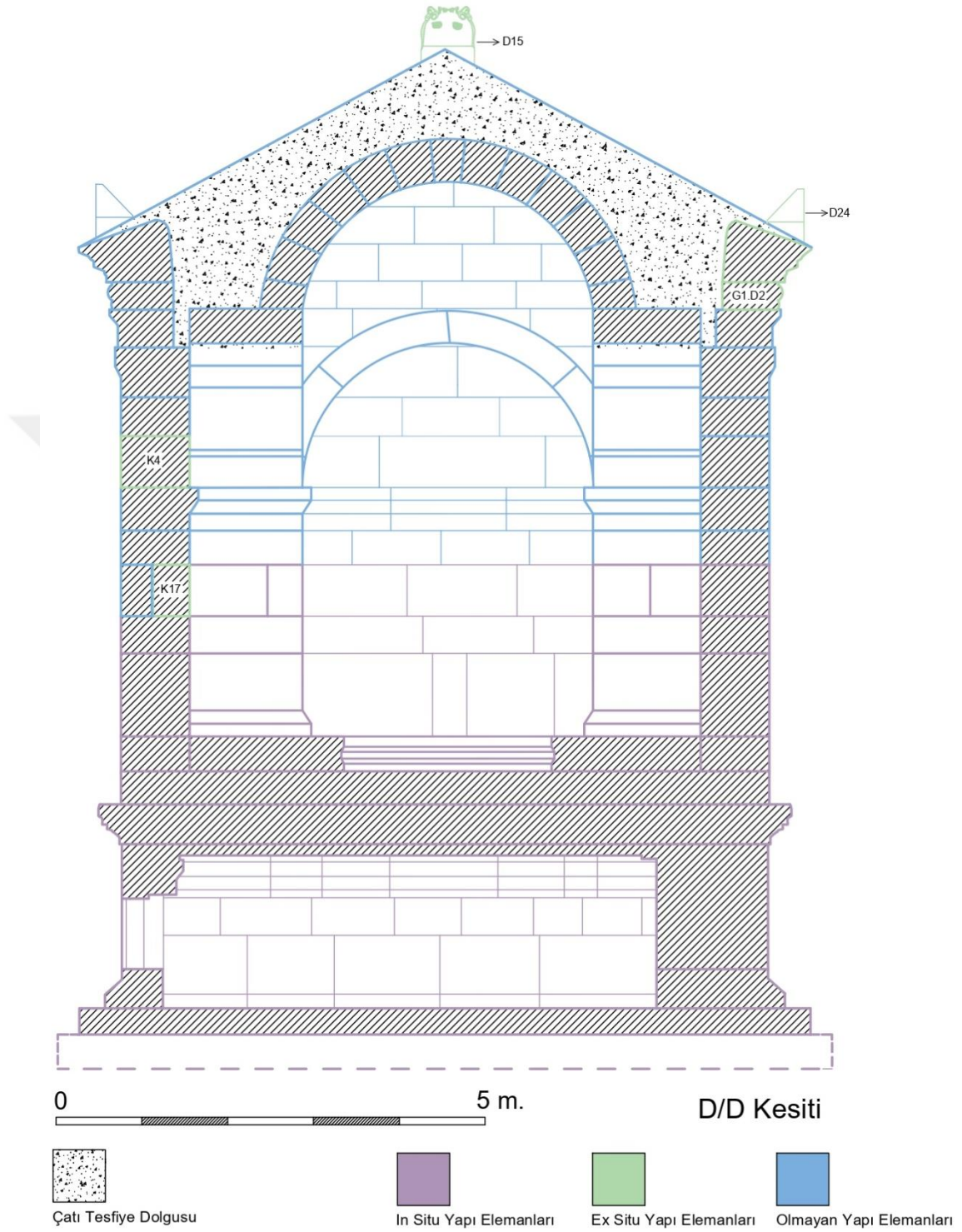
Çizim 22: Doğu Görünüşlü Kuzey-Güney Kesiti
