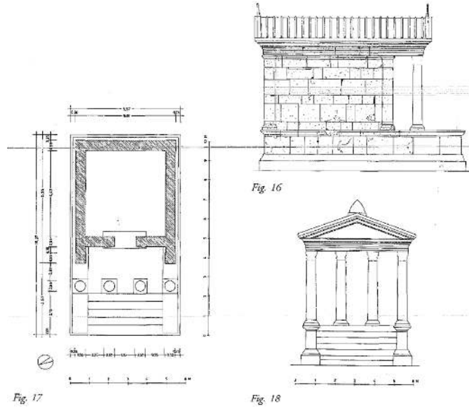
Çizim: 36: Adada, Kuzey Mezarı
