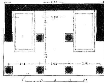
Çizim 63: Termessos, Aurelia Padamuriane Nanelis'in Mezarı (Heberdey- Wilberg, 1900: Fig.71-72)
