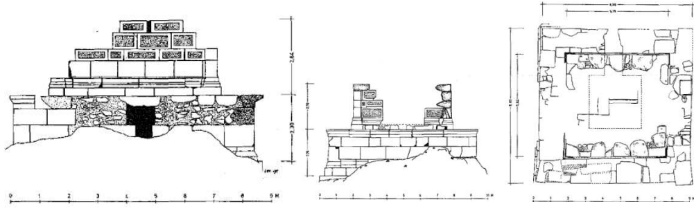
Çizim 38: Ariassos N8 Mezarı (Cormack, 2004: 177, Fig. 27-29)
