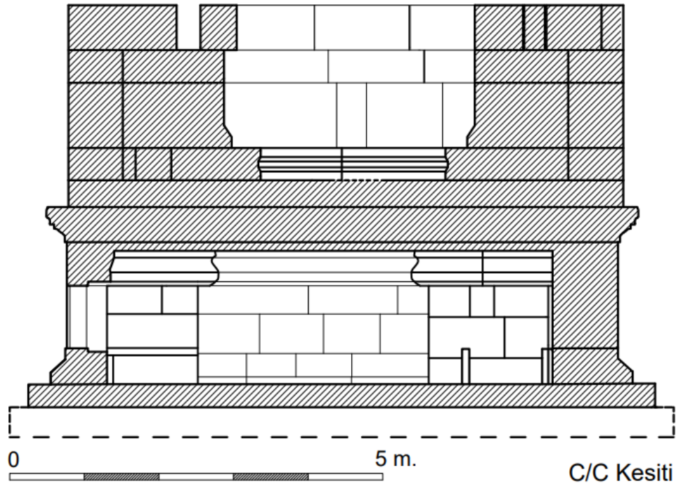
Çizim 9: M58 Mezarı, Doğu Görünüşlü Kuzey-Güney Kesiti, C-C
