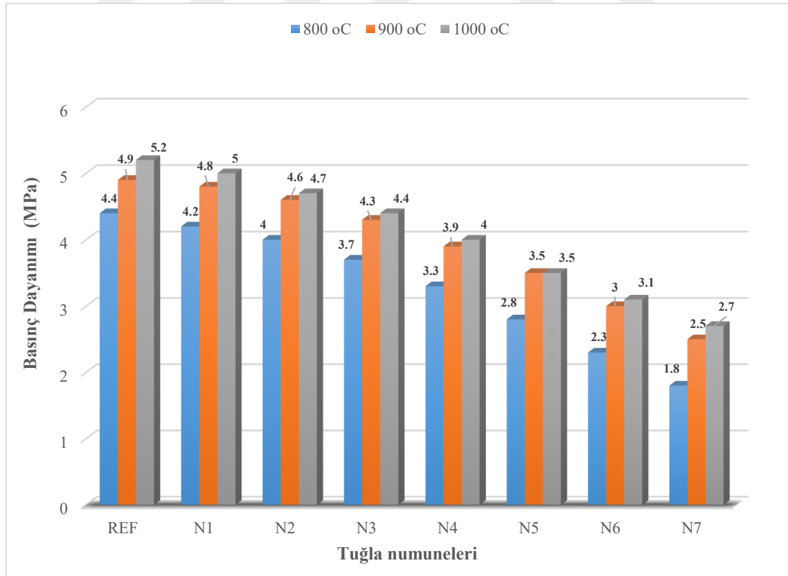
Şekil 4.6. Basınç dayanımı grafiği
