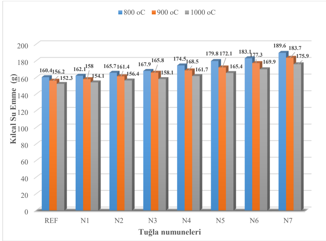
Şekil 4.4. Kılcal su emme grafiği
