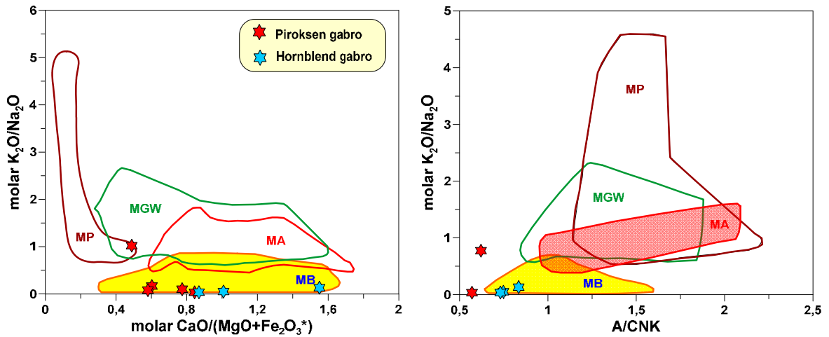
Şekil 36. Kovanlık Plütunu kayaçlarının molar K_2O/Na_2O karşı molar CaO/(MgO+Fe_2O_3^*) (a) ve A/CNK (b) kökensel ayırım diyagramları. MB, metabazalt; MA, metaandezit; MGW, metagrovak; MP, metapelit. Alanlar; Vielzeuf ve Holloway (1988), Patiño Douce ve Johnston (1991), Rapp vd. (1991), Gardien vd. (1995), Rapp (1995), Rapp ve Watson (1995), Patiño Douce ve Beard (1996), Stevens vd. (1997), Skjerlie ve Johnston (1996), Patiño Douce (1997), Patiño Douce ve McCarthy (1998), Patiño Douce (1999)'ye göre.
