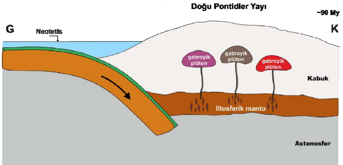
Şekil 37. Pontidlerde yay ile ilişkili Üst Kretase mafik plütonların gelişimine ait şematik jeodinamik model
