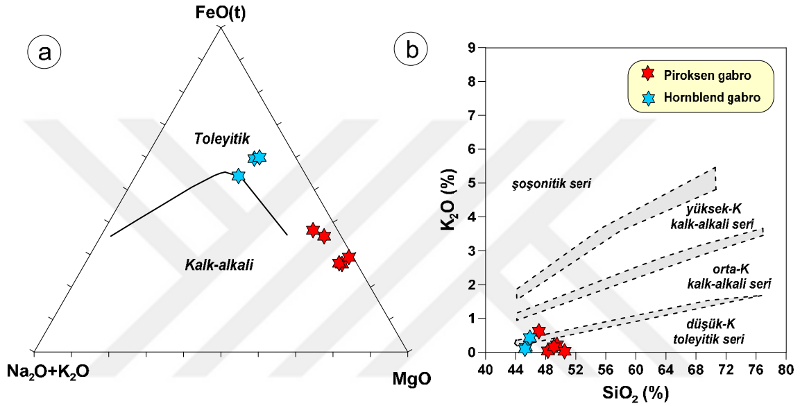
Şekil 25. Kovanlık Plütönu'nu oluşturan kayaçların, (a) AFM diyagramı (toleyitik-kalkalkali eğrisi, Irvine ve Baragar, 1971'e göredir), (b) \text{SiO}_2 (%) karşı \text{K}_2\text{O} (%) diyagramı (Le Maitre vd., 2002).
