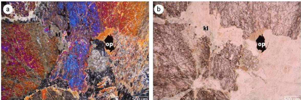
Şekil 16. Kovanlık Plütönu gabroyik kayaçlarındaki piroksen minerallerinde gözlenen kloritleşme (Örn.: KV-1; a, Ç.N. ve b, T.N.; kl, klorit; op, opak mineral).
