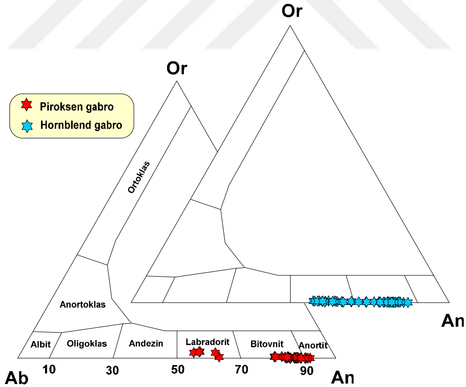
Şekil 17. Kovanlık Plütunu'na ait piroksen gabro ve hornblend gabrolardaki feldispatların An-Ab-Or üçgen diyagramı (Deer vd., 1992)
