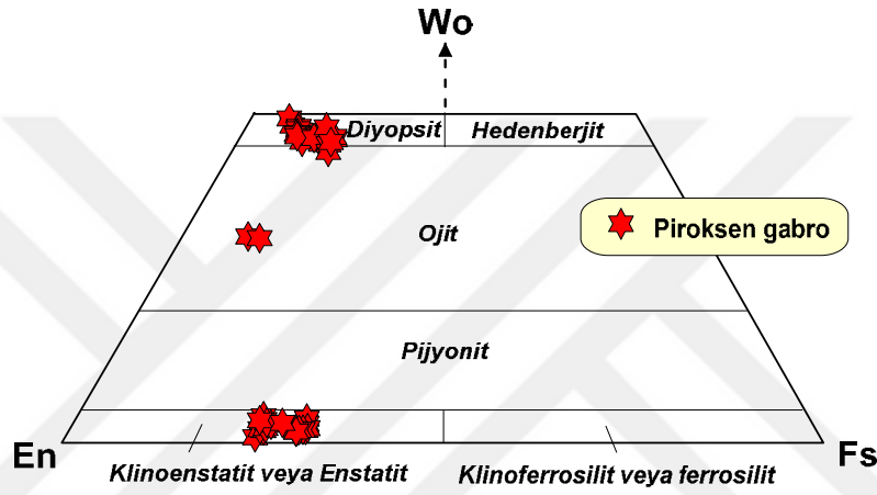
Şekil 18. Kovanlık Plütonu'na ait piroksen gabrolardaki piroksenlerin Wo-En-Fs üçgen diyagramı (Morimoto vd., 1988)
