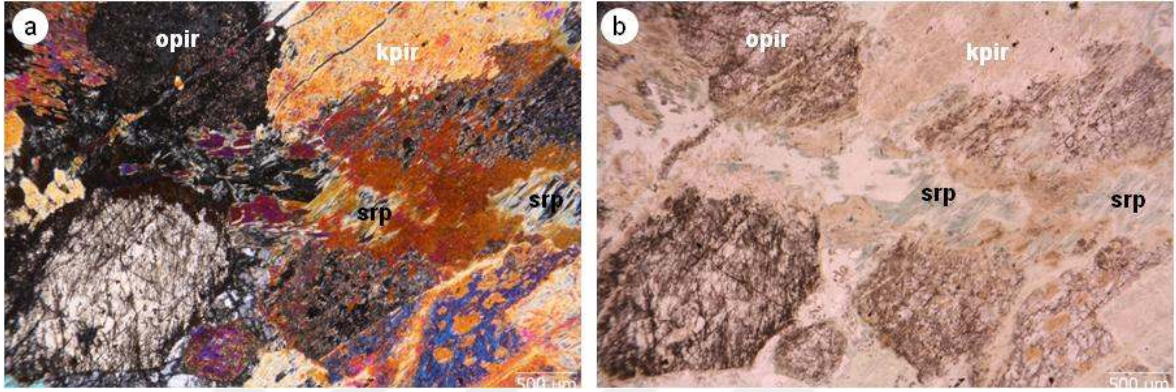
Şekil 15. Kovanlık Plütönu piroksen gabrolarının içerdiği klinopiroksen ve ortopiroksen minerallerinde gözlenen serpanlinleşme (Örn: KV-1; a, Ç.N. ve b, T.N.; srp, serpanlin; opir, ortopiroksen; kpir, klinopiroksen).
