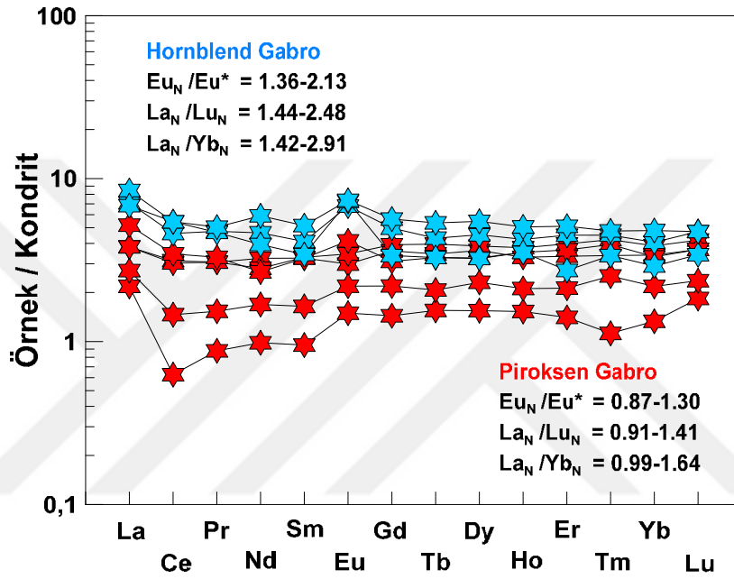
Şekil 29. Kovanlık Plütunu'nu oluşturan kayaçların kondrite normalize edilmiş nadir toprak element dağılımları (Normalize değerler, Taylor ve McLennan (1985)'dan alınmıştır).
