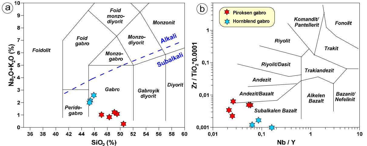
Şekil 24. Kovanlık Plütönu'nu oluşturan kayaların (a) Na_2O+K_2O (%) karşı SiO_2 (%) (TAS, Middlemost, 1994), (b) Zr/TiO_2 \cdot 0.0001 karşı Nb/Y (Winchester ve Floyd, 1977'den revize edilmiş Pearce, 1996) sınıflama diyagramları (Alkali-subalkali ayırım çizgisi, Miyashiro (1978)'e göredir).
