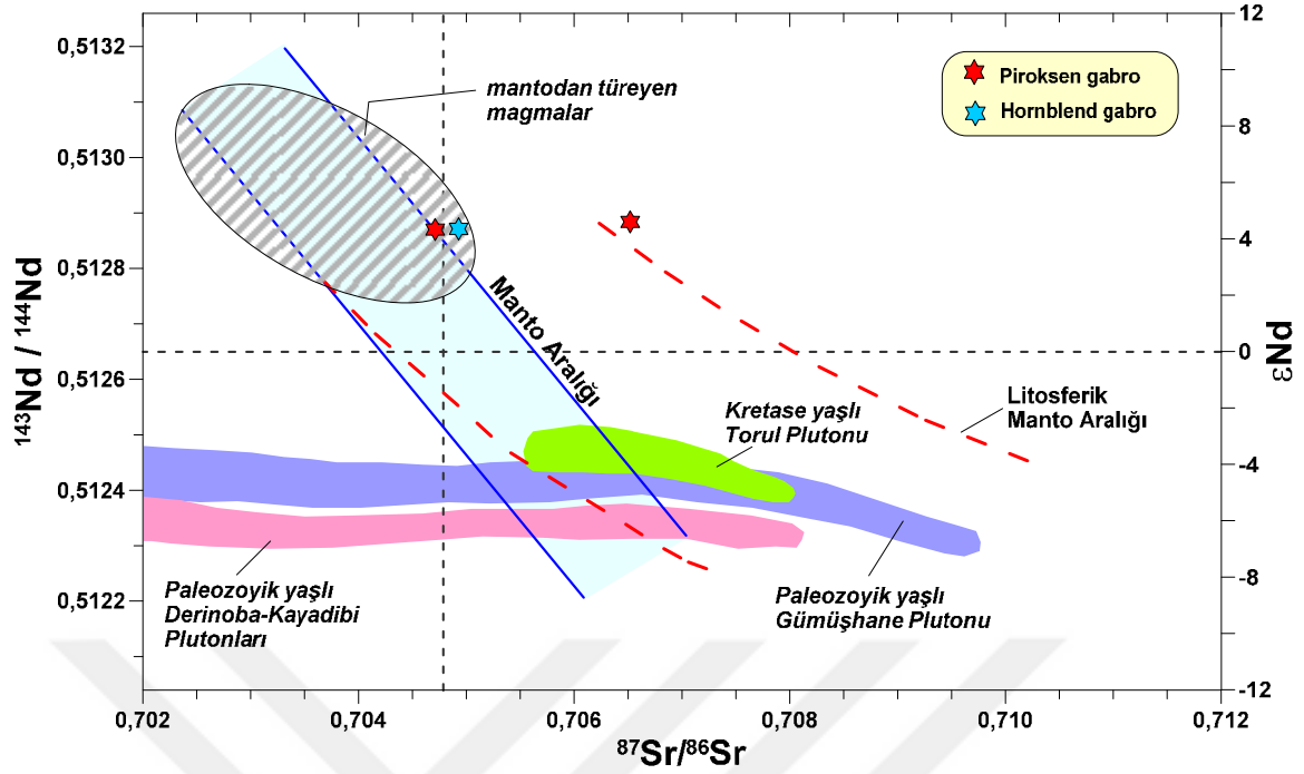
Şekil 31. Kovanlık Plütönu kayaçlarının ^{87}\text{Sr}/^{86}\text{Sr} karşı ^{143}\text{Nd}/^{144}\text{Nd} diyagramı ve Doğu Pontidler'deki diğer Kretase ve Paleozoyik yaşı plütönlr ile karşılaştırılması. Mantodan türeyen magmaların alanı, Manto aralığı, Hart (1984, 1988) ve Hawkesworth vd. (1984)'ne, litosferik manto aralığı ise Davies ve Von Blanckenburg (1995)'a göre'dir. Doğu Pontidler'deki bileşimsel alanlar; Torul Plütönu Kaygusuz vd. (2008, 2010)'den, Derinoba-Kayadibi Plütönlr Kaygusuz vd. (2012)'den ve Gümüşhane Plütönu Topuz vd. (2010)'den alınmıştır.
