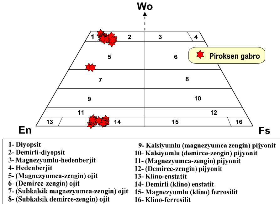
Şekil 19. Kovanlık Plütonu'na ait piroksen gabrolardaki piroksenlerin Wo-En-Fs üçgen diyagramı (Rock, 1990).
