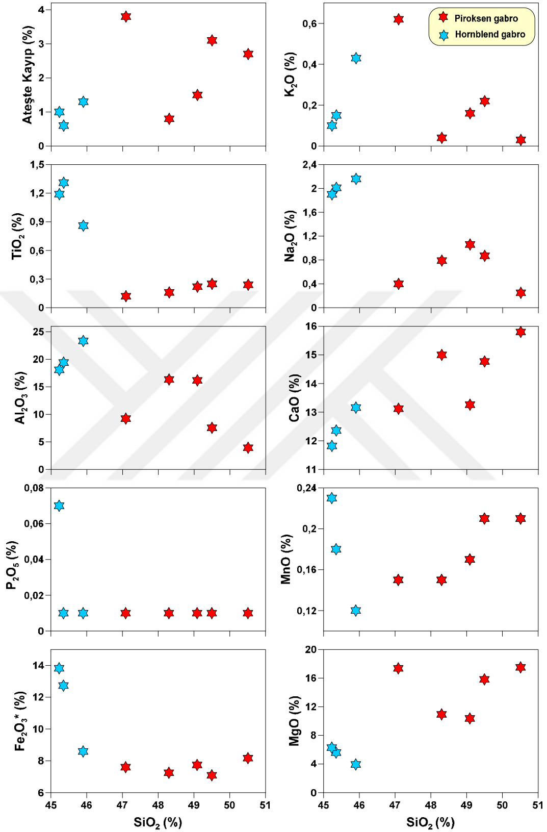
Şekil 26. Kovanlık Plütunu'nu oluşturan kayaçların \text{SiO}_2 (%)'ye karşı ana oksit (%) değişim diyagramları.
