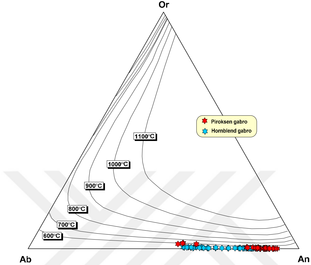
Şekil 22. Kovanlık Plütünü'nu oluşturan kayalara ait feldispatların Ab-An-Or üçgen diyagramı. İzoterm eğrileri, Fuhrman ve Lindsley (1988)'e göre.
