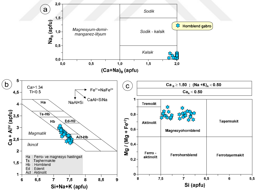
Şekil 20. Kovanlık Plütonu'na ait hornblend gabrolardaki hornblendlerin; (a) (Ca+Na)_B (apfu) karşı Na_B (apfu) (Leake vd., 1997), (b) (Ca+Al^{IV}) (apfu) karşı (Si+Na+K) (apfu) (Giret vd., 1980) ve (c) Si (apfu) karşı Mg/(Mg+Fe^{+2}) (Leake vd., 1997) sınıflama diyagramları.
