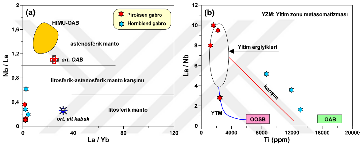
Şekil 34. Kovanlık Plütönu gabroyik kayaçlarının (a) La/Yb karşı Nb/La ve (b) Ti (ppm) karşı La/Nb diyagramları. Veriler; (a) Astenosferik manto, litosferik manto ve litosferik-astenosferik manto karışımı arasındaki sınırlar Smith vd. (1999)'dan, HIMU-OAB alanı Weaver vd. (1987)'den, ort. OAB (ortalama Okyanus Adası Bazaltı) değeri Fitton vd. (1991)'den, ortalama alt kabuk değeri ise Chen ve Arculus (1995)'den alınmıştır. (b)Yitim ergiyikleri alanı Schiano vd. (1995) ve Yogodzinski vd. (1995)'den, OOSB (Okyanus Ortası Sırtı Bazaltı) ve OAB alanları ise Sun ve McDonough (1989) alınmıştır.
