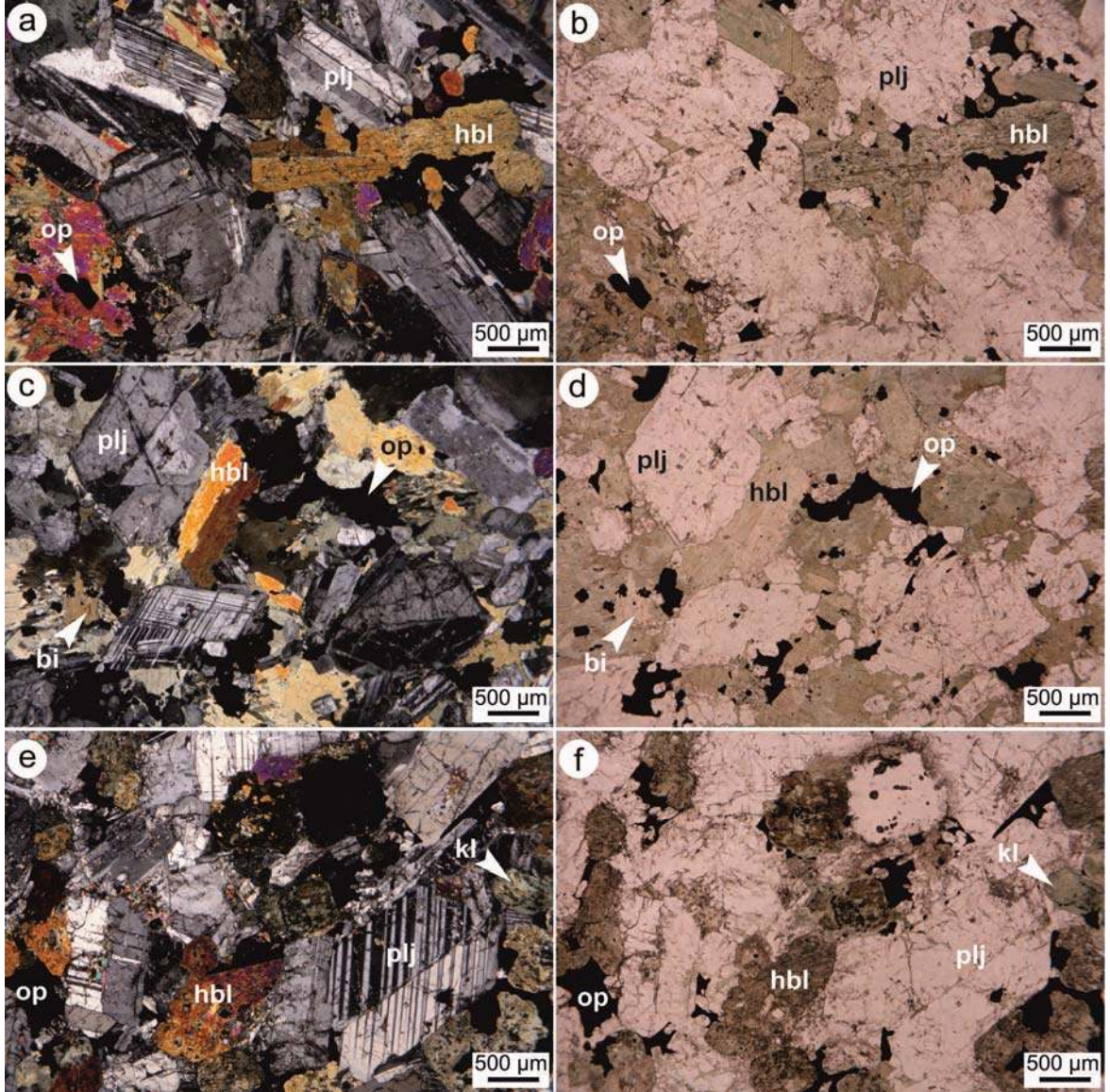
Şekil 13. Kovanlık Plütunu'na ait ince taneli doku gösteren hornblend gabroların mikrofotoğrafları. a-b) Albit ve albit-karlsbad karmaşık ikizi gösteren plajiyoklaslar ve opak mineral kapanımları içeren hornblend (Örnek No: KV-3; Ç.N. ve T.N.); c-d) albit-karlsbad ikizi ve optik zonlanma gösteren plajiyoklas, basit ikiz gösteren hornblend ve özşekilsiz küçük biyotit (Örnek No: KV-3; Ç.N. ve T.N.); e-f) albit-karlsbad karmaşık ikizi gösteren plajiyoklas, özşekilsiz opak mineral ve kısmen kloritleşmiş hornblend kristalleri (Örnek No: KV-4; Ç.N. ve T.N.) (açıklamalar; Ç.N., çapraz nikol; T.N., tek nikol; hbl, hornblend; bi, biyotit; plj, plajiyoklas; op, opak mineral).
