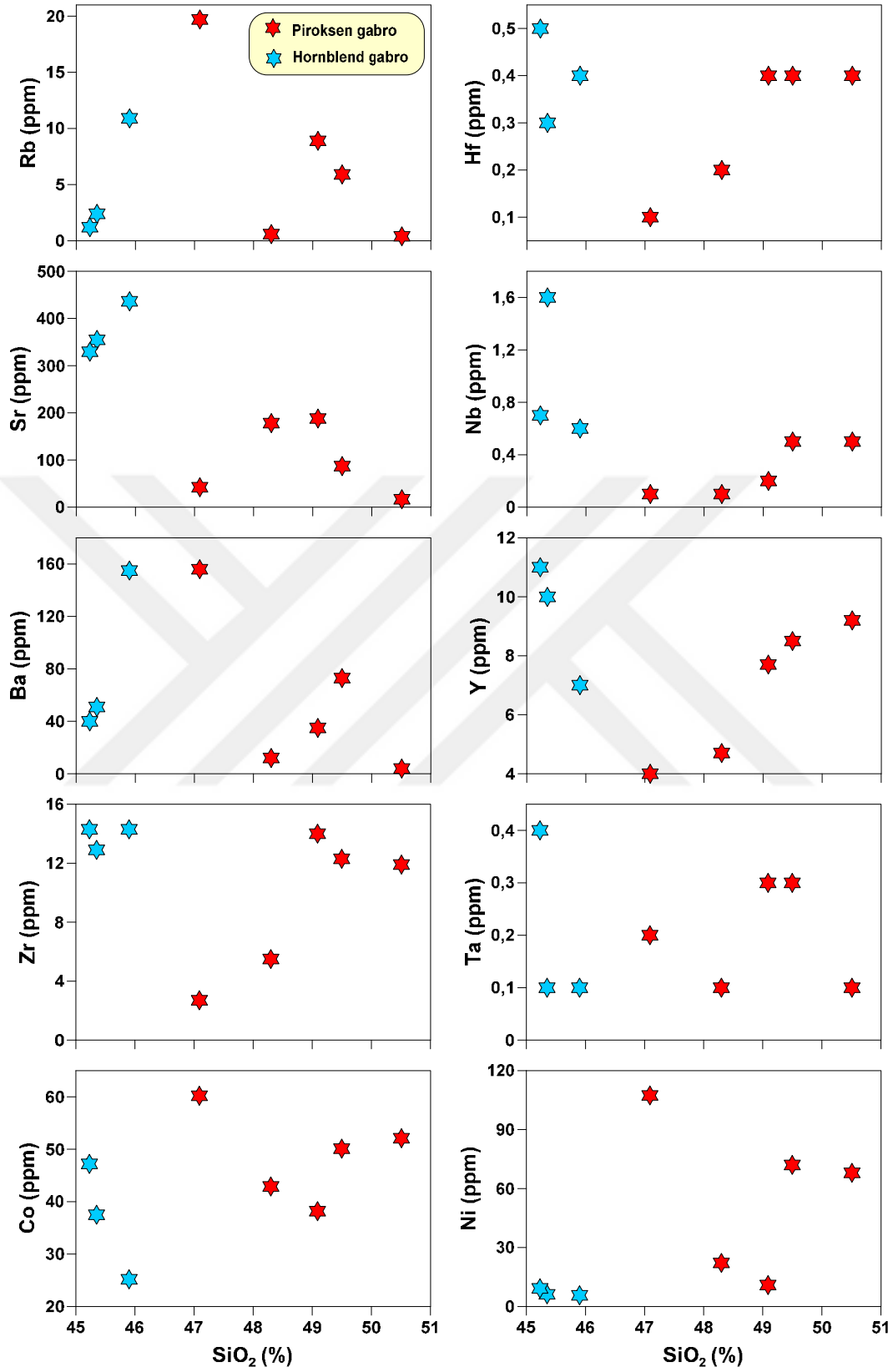
Şekil 27. Kovanlık Plütünü'nu oluşturan kayaların \text{SiO}_2 (%)'ye karşı iz element (ppm) değişim diyagramları.
