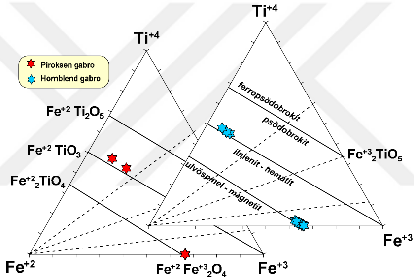
Şekil 21. Kovanlık Plütunu'na ait piroksen gabro ve hornblend gabrolardaki Fe-Ti oksitlerin Ti 4+ -Fe 3+ -Fe 2+ üçgen diyagramı (Bacon ve Hirschmann, 1988)
