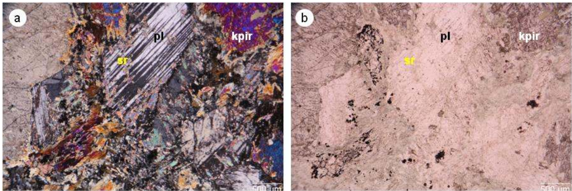
Şekil 14. Kovanlık Plütonu piroksen gabrolarının içerdiği plajiyoklas minerallerinde gözlenen serisitleşme (Örn: KV-1; a, Ç.N. ve b, T.N.; sr, serisit; kpir, klinopiroksen; pl, plajiyoklas).
