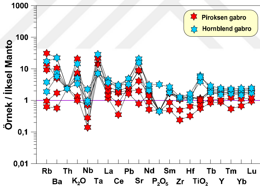
Şekil 28. Kovanlık Plütunu'nu oluşturan kayaçların ilksel manto'ya göre normalize edilmiş iz element dağılımları (Normalize değerleri, Sun ve McDonough, 1989'dan alınmıştır).
