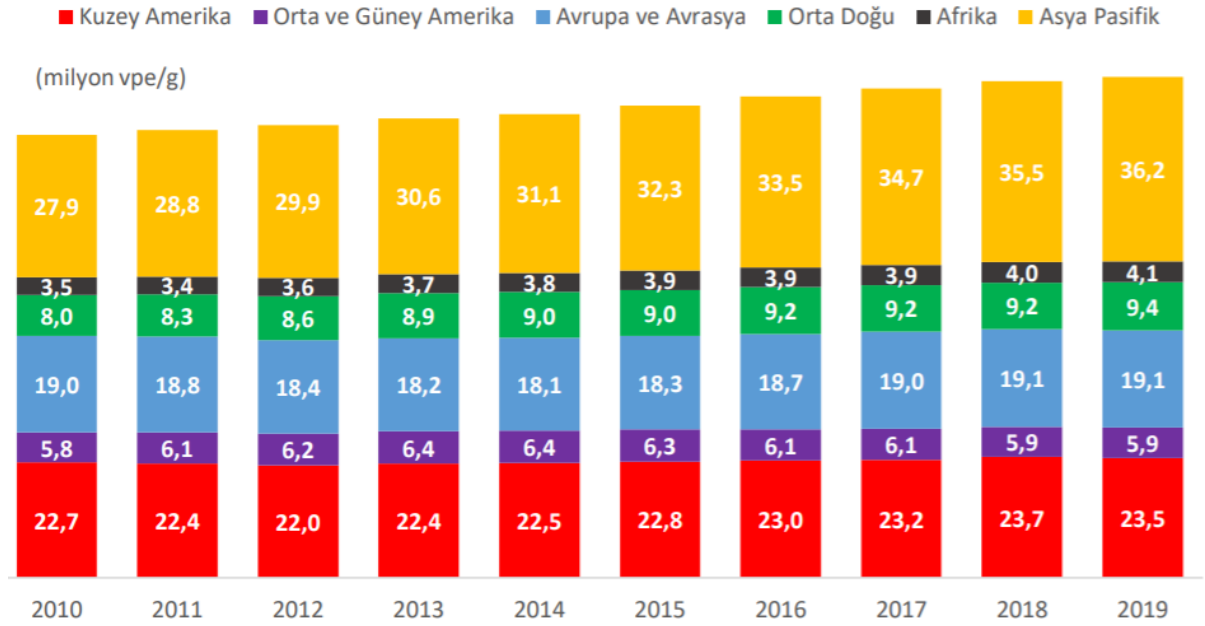
Şekil 2.4: 2010-2019 Bölgelere Göre Dünya Petrol Tüketimi
