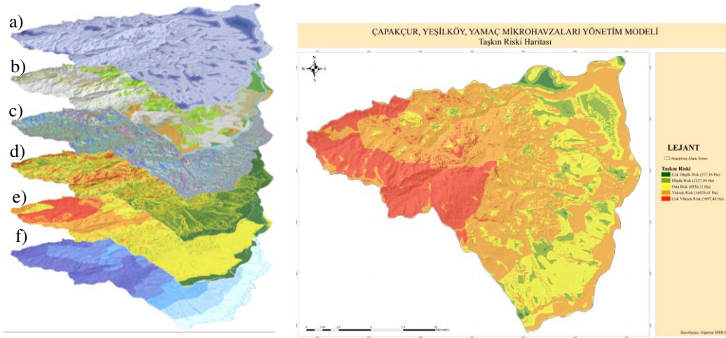
Harita 3.17. Araştırma alanı Taşkın Riski haritası a) Akarsulara yakınlık b) Mevcut arazi kullanımı c) Bakı d) Eğim grupları e) Toprak geçirimsizliği f) Yağış.
