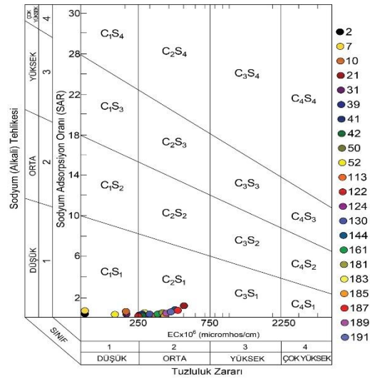
Şekil 2.8. ABD tuzluluk laboratuvarı diyagramı.
