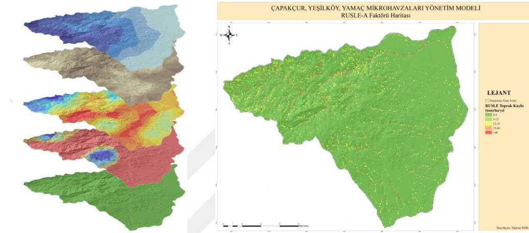
Harita 3.16. Araştırma alanı RUSLE Erozyon Modeli.
