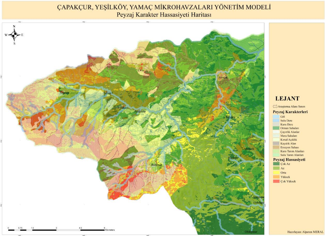
Harita 3.28. Araştırma alanı Peyzaj Karakter Hassasiyeti haritası.
