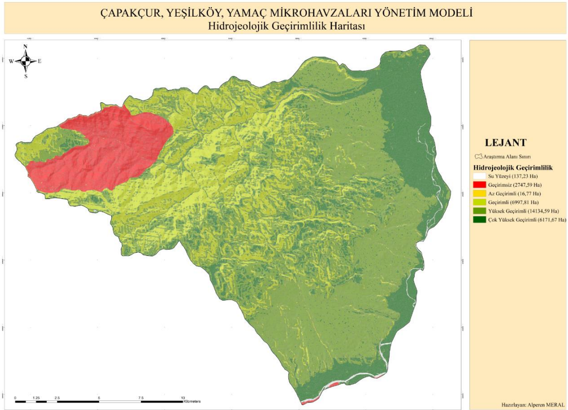
Harita 3.9. Araştırma alanı hidrojeolojik geçirirliilik haritası.
