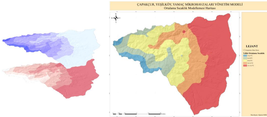
Harita 3.14. Araştırma alanı yıllık ortalama sıcaklık modellemesi a)Yıllık ortalama en düşük sıcaklık b)Yıllık ortalama en yüksek sıcaklık).
