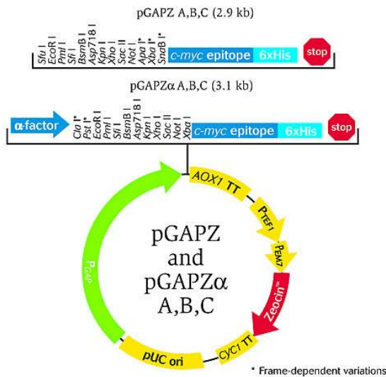
Şekil 3.2. P. pastoris 'te Mig1 proteinini hücre içi üretmekte kullanılan PGAPZB (Invitrogen, CA, ABD) vektörü
