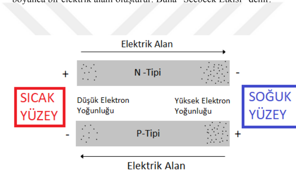
Şekil 2.7. Seebeck Etkisi
