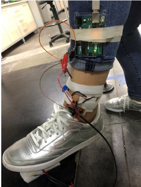
Şekil 4.4. Oturma Pozisyonunda Test Düzeneği Görüntüsü
