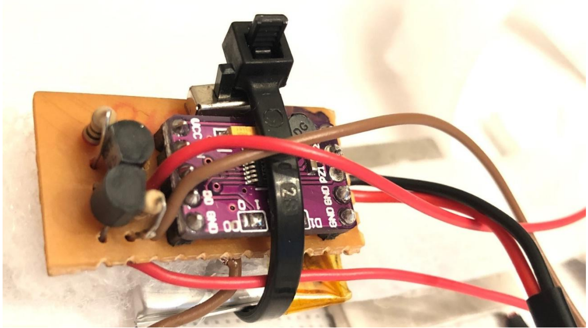
Şekil 3.10. LTC 3588-1 enerji hasat modülü modifikasyonu
