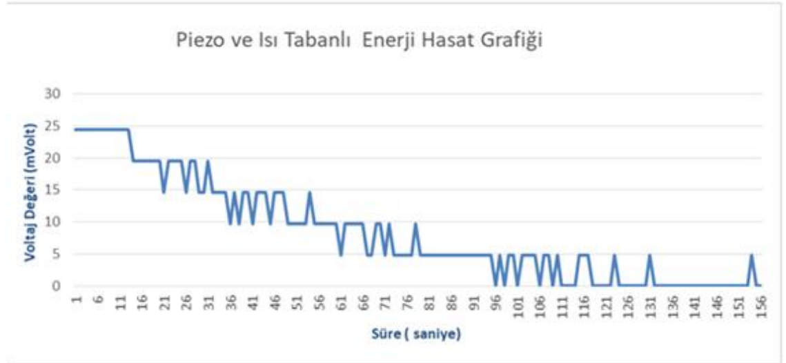
Şekil 4.9. Ayaktaki denek diz kapağı arkasına uygulanmış hibrit enerji hasat grafiği
