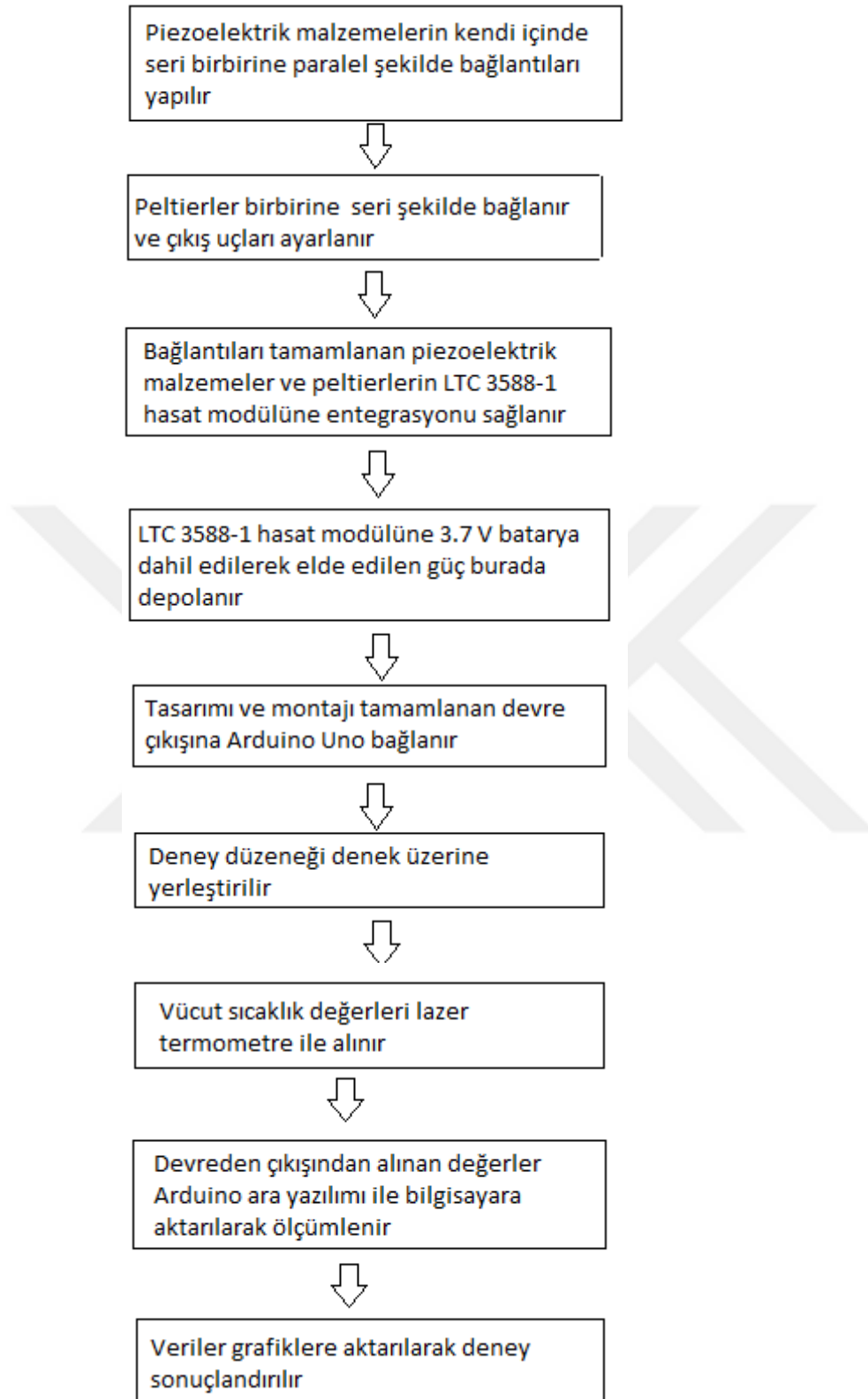
Şekil 3.5. Proses Algoritması
