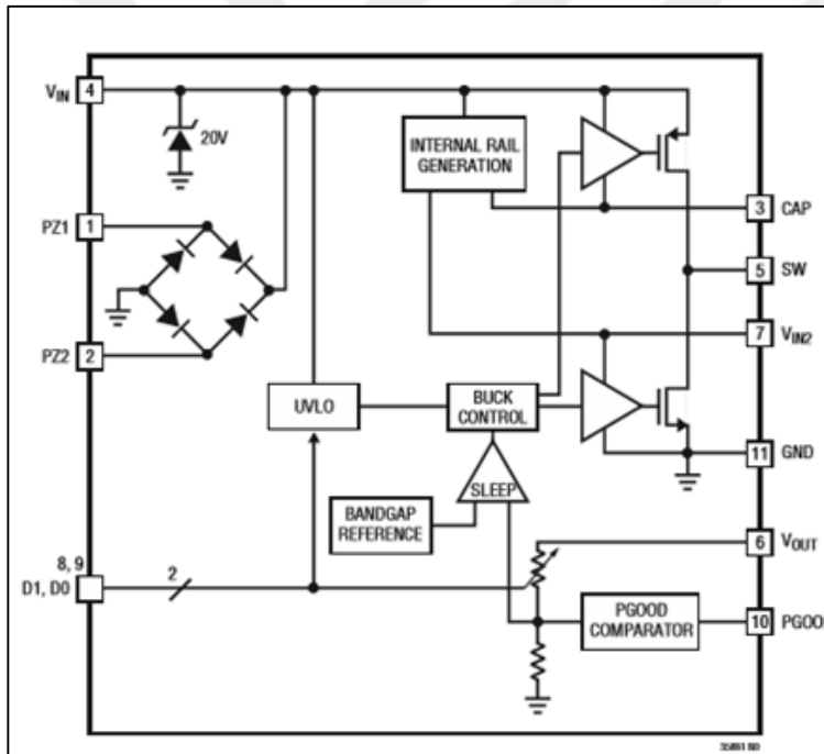
Şekil 3.1. LTC 3588-1 mikroişlemci Blok Diyagramı
