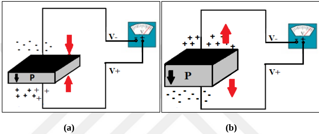
Şekil 2.2. a) Piezoelektrik malzemeye gerilim uygulanmadan önceki görüntüsü
