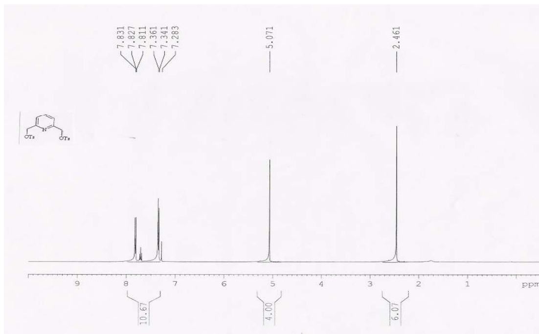
Spektrum 1. 2,6-Bis(hidroksimetil)piridinditosilat (2,6-Piridindimetanoditosilat)'ın 1 H NMR spektrumu.
