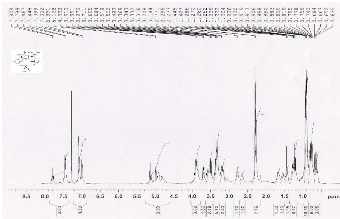
Spektrum 18. Leucinol Aminoalkolü içeren Makrohalkanın ^1\text{H} NMR spektrumu
