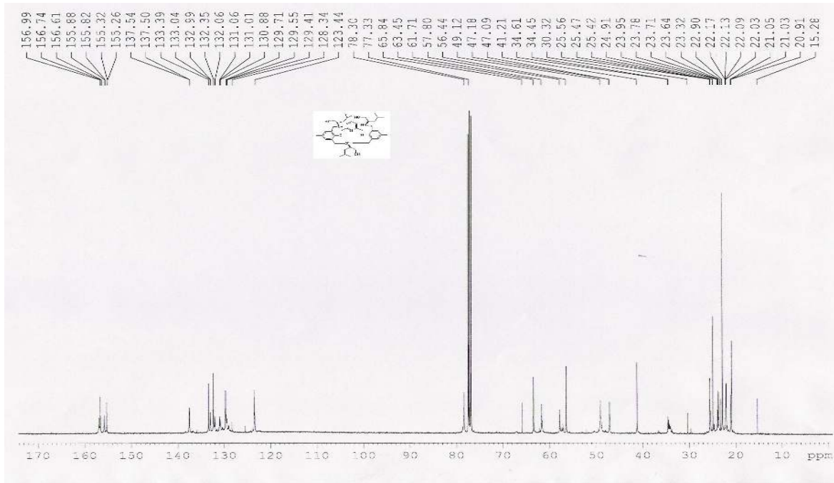
Spektrum 19. Leucinol Aminoalkolü içeren Makrohalkanın ^{13}\text{C} NMR spektrumu
