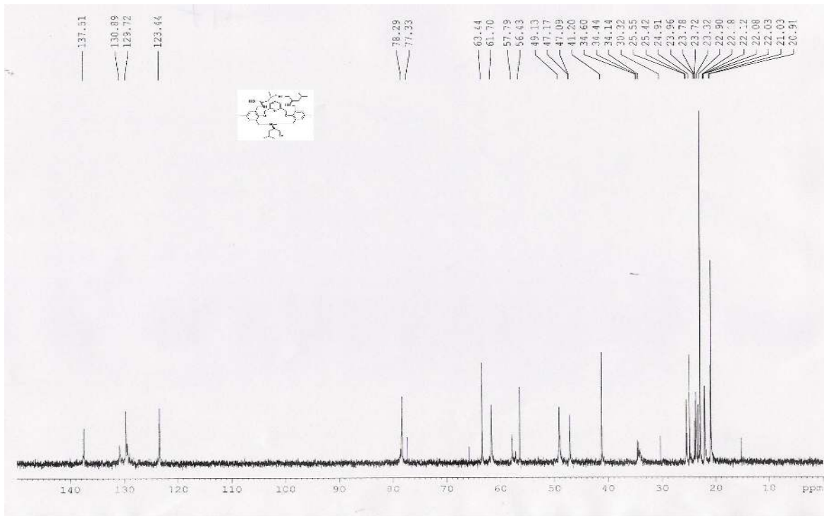
Spektrum 20. Leucinol Aminoalkolü içeren Makrohalkanın DEPT 45 spektrumu
