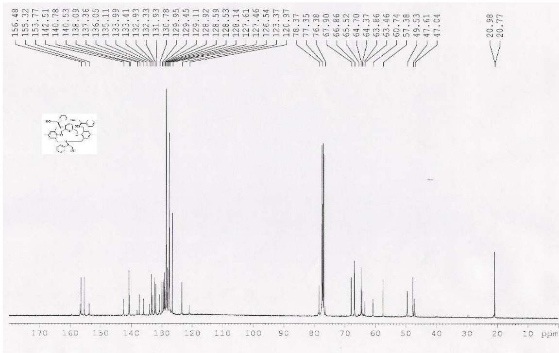
Spektrum 10. Fenilglisinol Aminoalkolü içeren Makrohalkanın 13 C NMR spektrum
