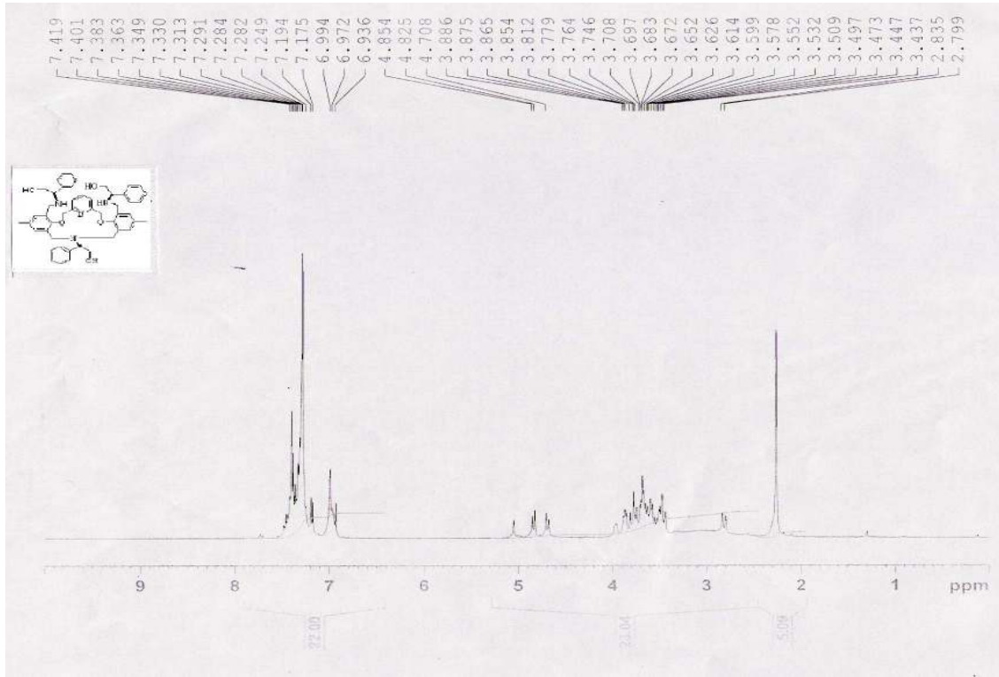
Spektrum 9. Fenilglisinol Aminoalkolü içeren Makrohalkanın 1 H NMR spektrumu
