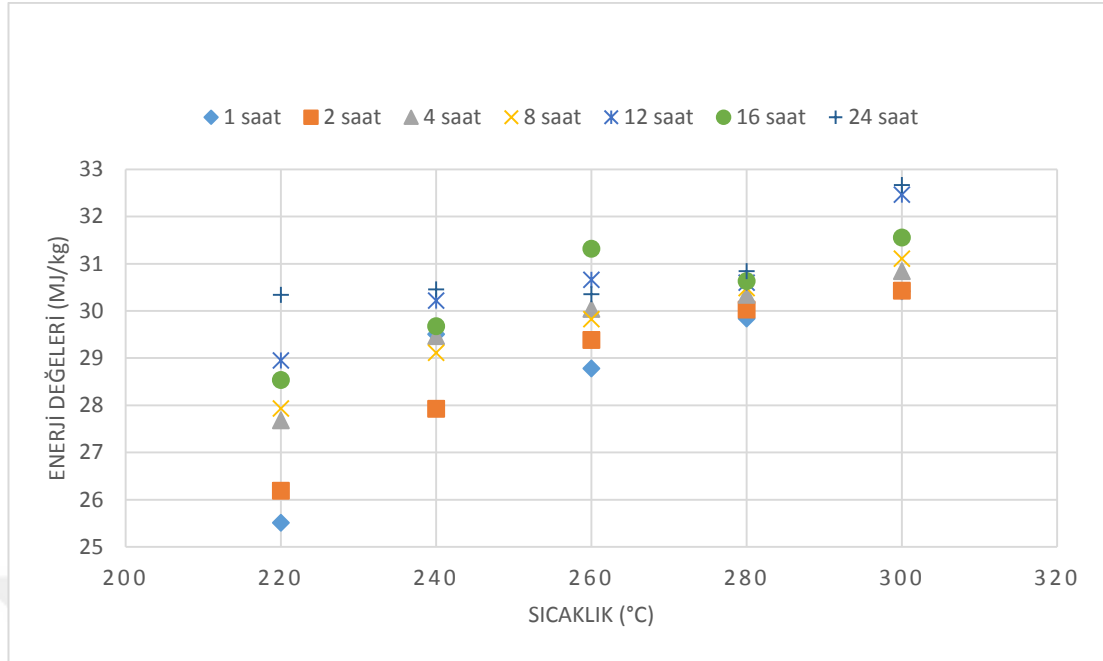
Şekil 9.2 Farklı sıcaklık ve bekletme sürelerinde hidrokömür enerji değerleri
