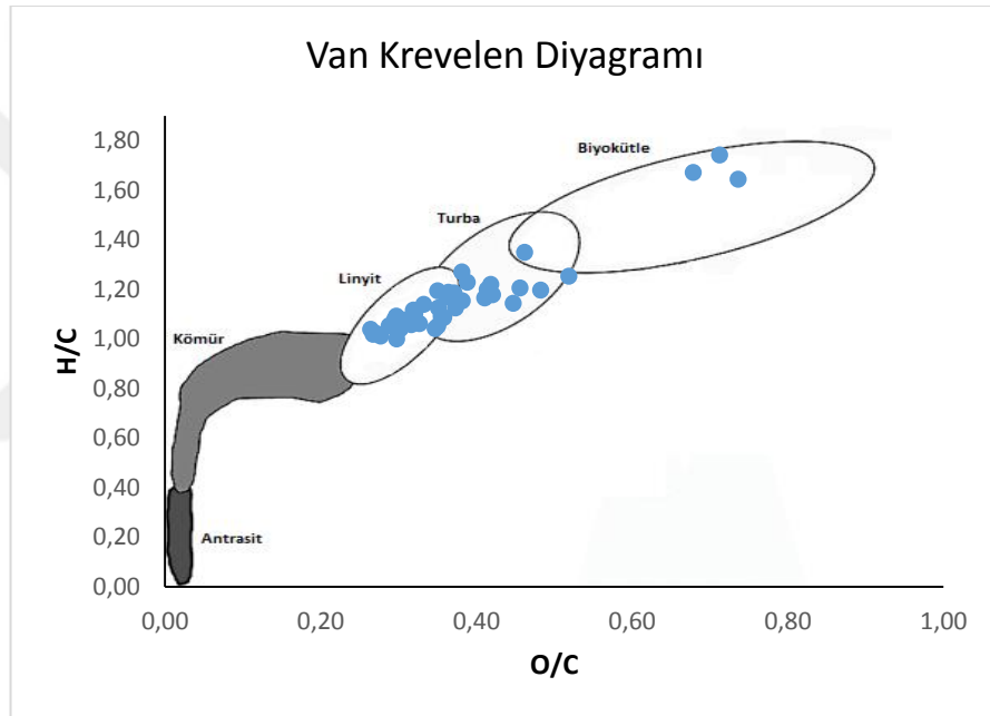
Şekil 9.5. Ham pirina ve çeşitli sıcaklık, bekletme sürelerinde elde edilen hidrokömürlerin Van Krevelen Diyagramı
