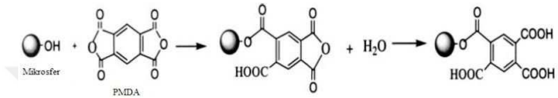
Şekil 2.9. PMDA ile modifiye edilmiş \beta -siklodekstrin mikrokürenin hazırlanması (Li ve ark., 2007)
