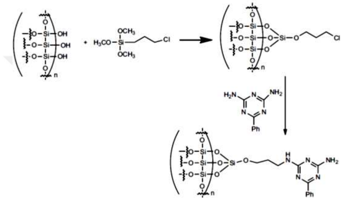
Şekil 2.2. 2,6-diamino-4-fenil-1,3,5-triazin bağlı silika jel (TZ-SG) sentezi (Mendil ve ark., 2016)
