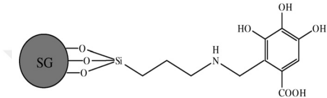
Şekil 2.6. Gallik asit bağlı silika jelin yapısı (Xie ve ark., 2008)
