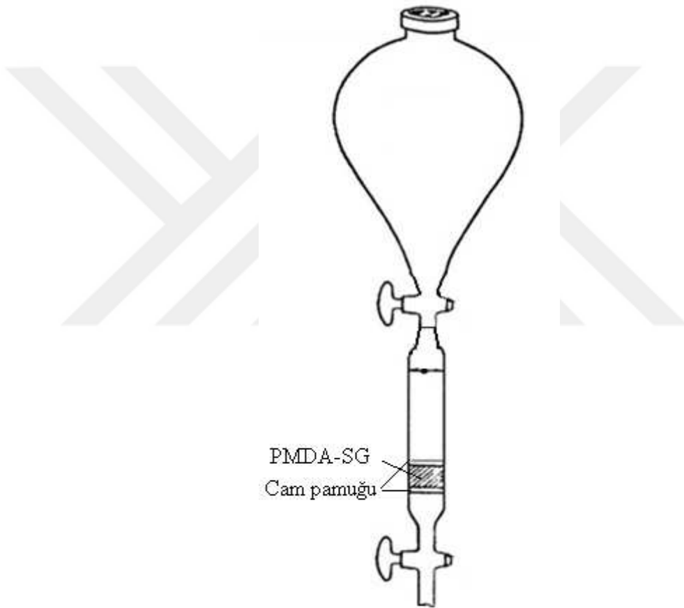
Şekil 3.3. Zenginleştirme çalışmaları sırasında kullanılan düzenek
