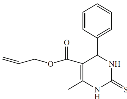
Şekil 2.4. Bağlı olan 6-metil-4-fenil-2-diokso-1,2,3,4-tetrahidropirimidin-5-karboksilat grubu (Sabermahani ve ark., 2012)
