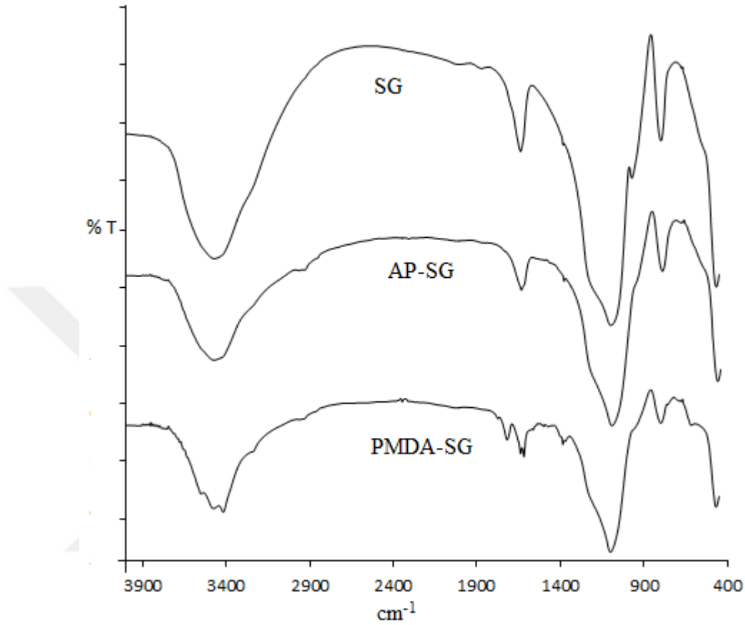
Şekil 4.1. Saf silika jel, amino propil bağlı silika jel ve piromellitik dianhidrit bağlı silika FT-IR Spektrumları
